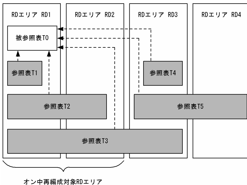
図 2-9 被参照表と参照表の構成例
