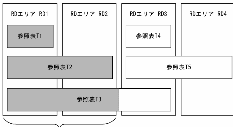
図 2-10 参照表の構成例
