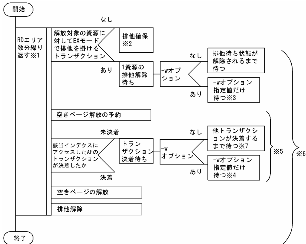
図 11-7 pdreclaim の排他制御の流れ (-a オプションなし)
