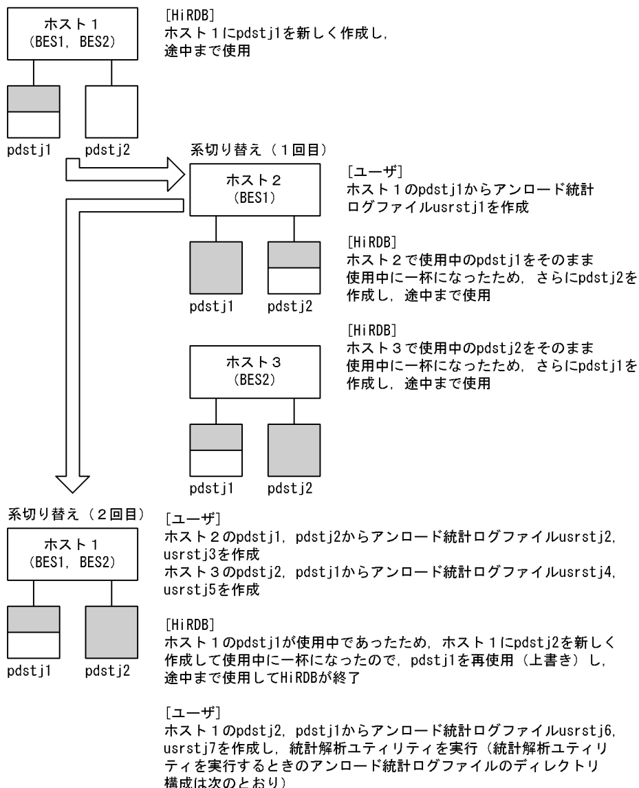
図 26-70 系切り替え機能使用時のアンロード統計ログファイルの作成例（その2）
