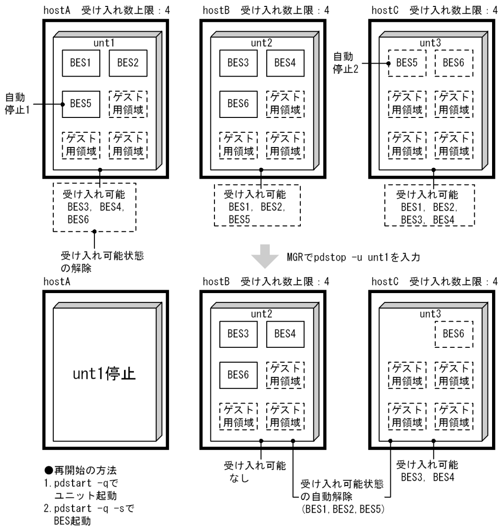
図 26-63 受け入れ中のユニットの停止の例
