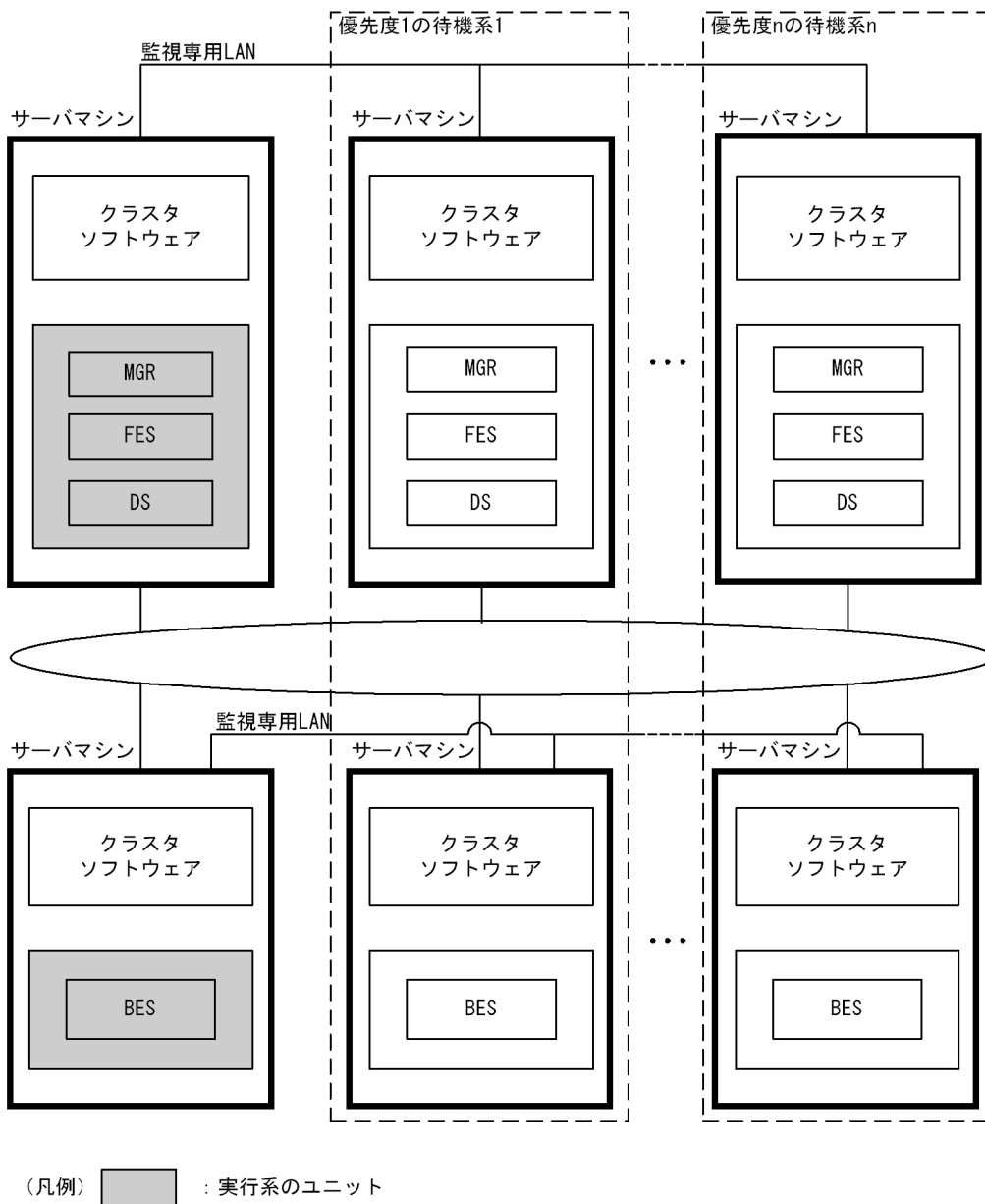
図 26-23 HiRDB/パラレルサーバに対するマルチスタンバイ構成の例
