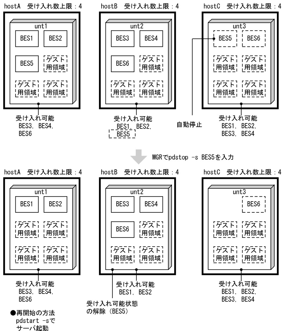
図 26-66 ゲスト BES の停止の例
