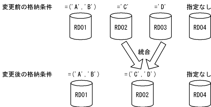
図 13-67 統合できないケース (その 3)
