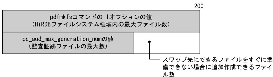
図 24-4 推奨する pd_aud_max_generation_num の値と -l オプションの値の関係
