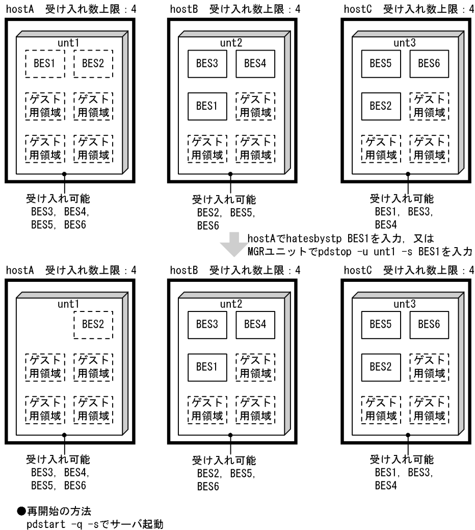
図 26-68 待機系のホスト BES の停止の例
