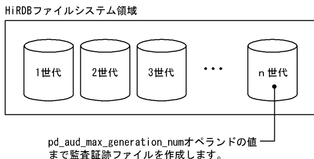
図 24-5 監査証跡ファイルの作成規則
