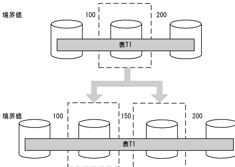
図 13-15 分割機能の概要 (境界値指定の場合)
