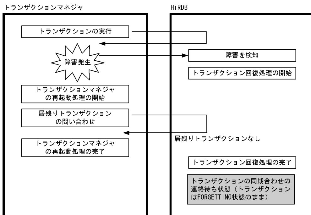
図 20-3 トランザクションマネージャの再起動完了後に FORGETTING 状態のトランザクションが発生する例
