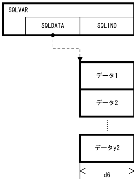
図 24-32 固定長のデータ型で配列を使った入力値（標識変数なし）の構造
