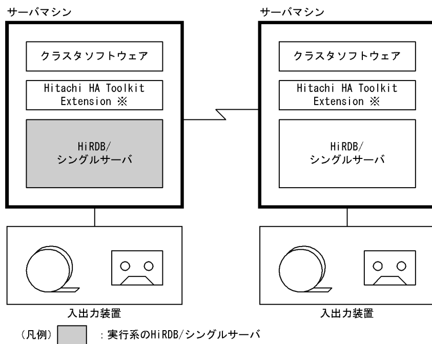
図 26-16 HiRDB/シングルサーバに対する1：1系切り替え構成の例
