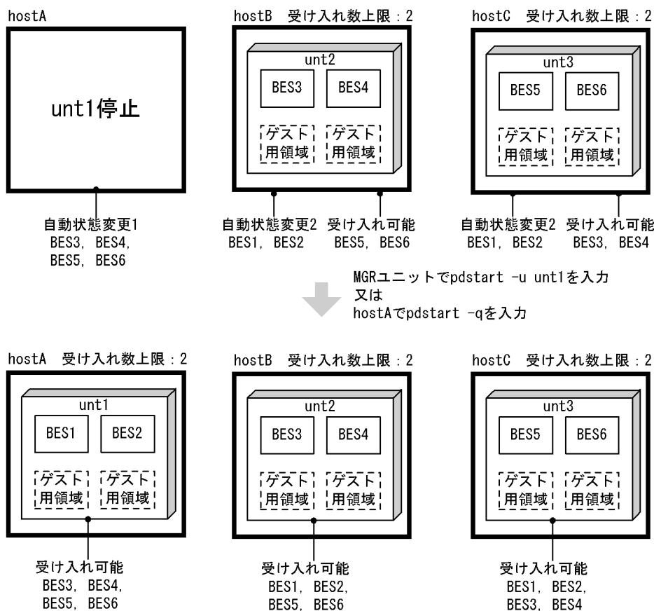
図 26-56 影響分散スタンバイレス型系切り替え機能でのユニット開始の例
