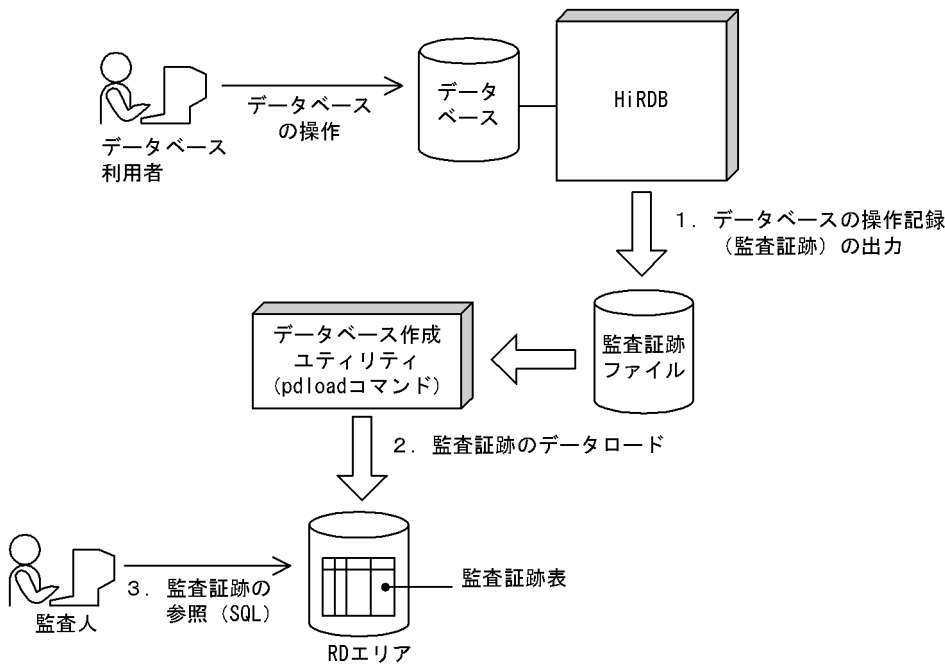
図 24-2 監査証跡の参照方法
