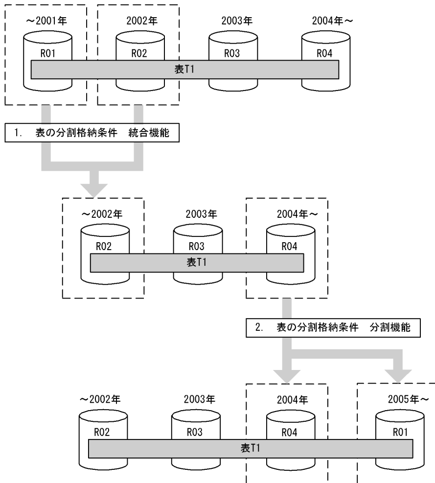
図 13-83 RD エリアを再利用する運用の例
