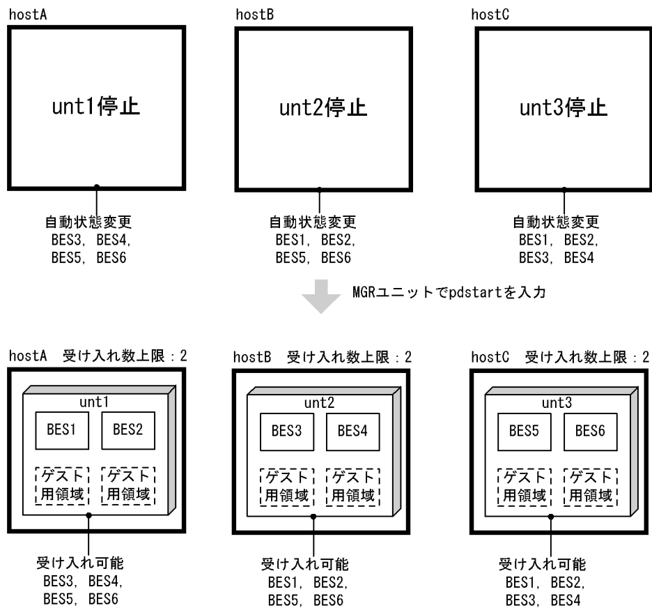
図 26-55 影響分散スタンバイレス型系切り替え機能でのシステム全体開始の例
