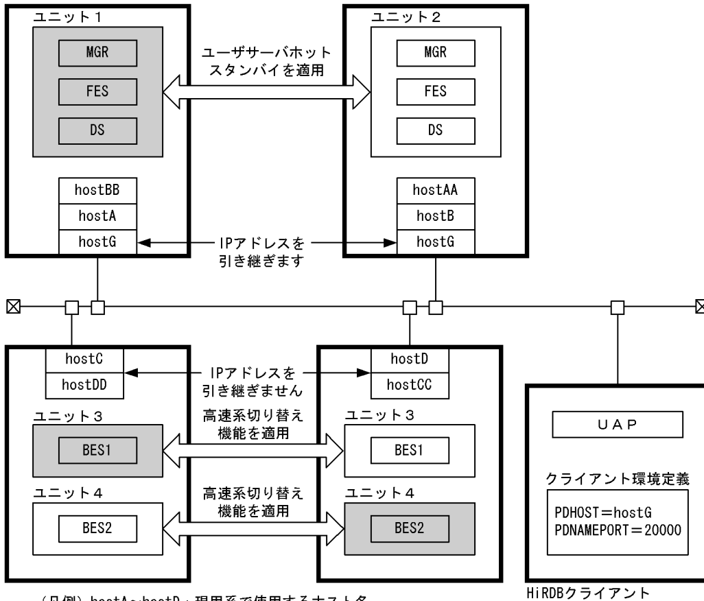
図 26-75 高速系切り替え機能使用時のシステム構成例
