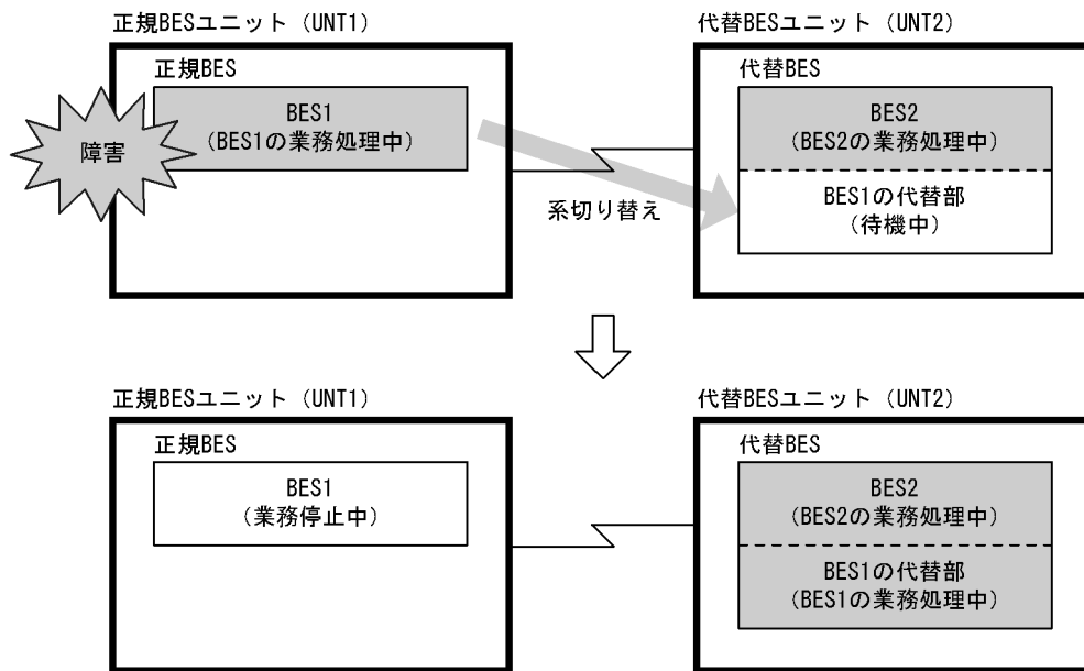
図 26-5 1 : 1 スタンバイレス型系切り替え機能の概要
