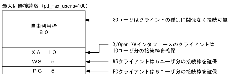
図 9-4 クライアントグループの接続枠保証機能
