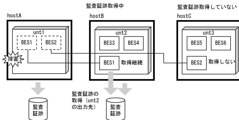
図 26-45 影響分散スタンバイレス型系切り替え機能適用時の監査証跡取得状況の例
