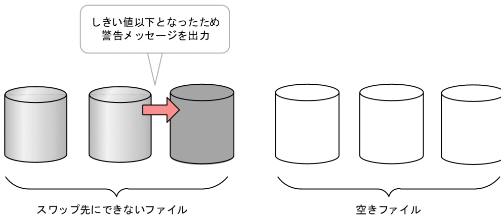
図 3-8 システムログファイルの残量警告機能の概要
