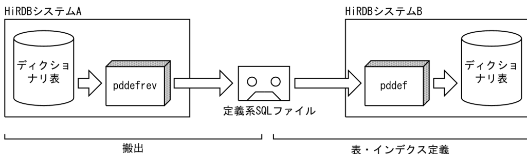
図 12-4 pddefrev（定義系 SQL の生成）を使用した表定義情報の移行
