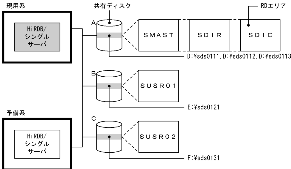
図 26-42 HiRDB/シングルサーバのシステム構成例
