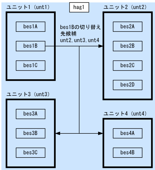
図 26-36 HA グループの構成例 (その 1)
