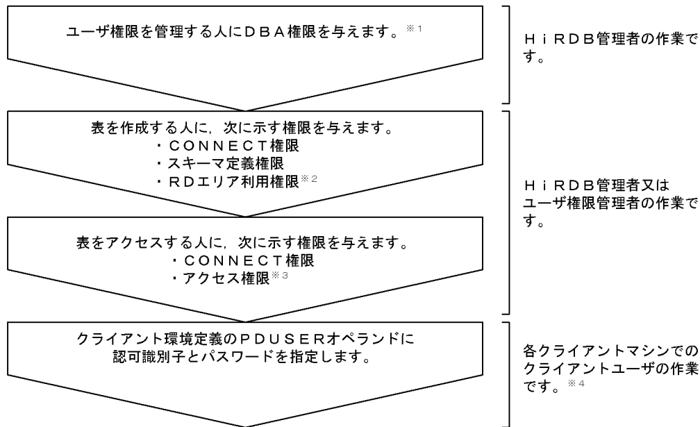
図 2-1 ユーザ権限を設定する手順
