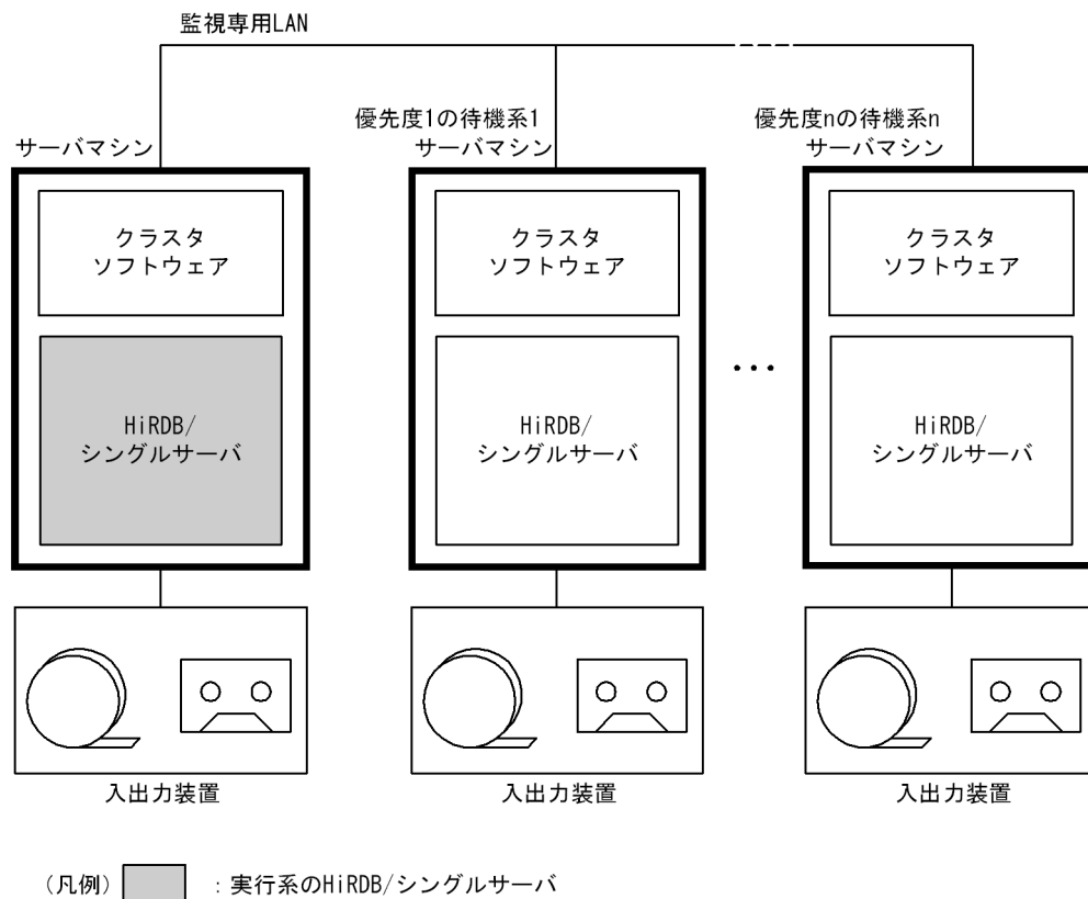
図 26-18 HiRDB/シングルサーバに対するマルチスタンバイ構成の例
