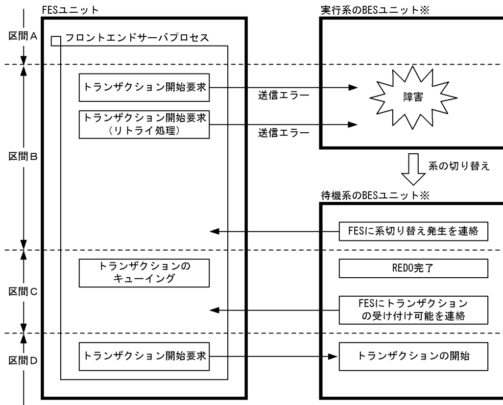
図 26-77 pd_ha_trn_queuing_wait_time オペランドと pd_ha_trn_restart_retry_time オペランドの関係
