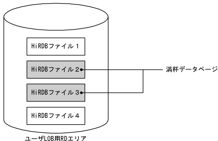
図 6-3 更新凍結コマンドの処理概要
