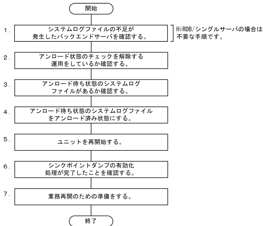
図 20-4 ユニットの再開を最優先する場合の対処手順（フロー）
