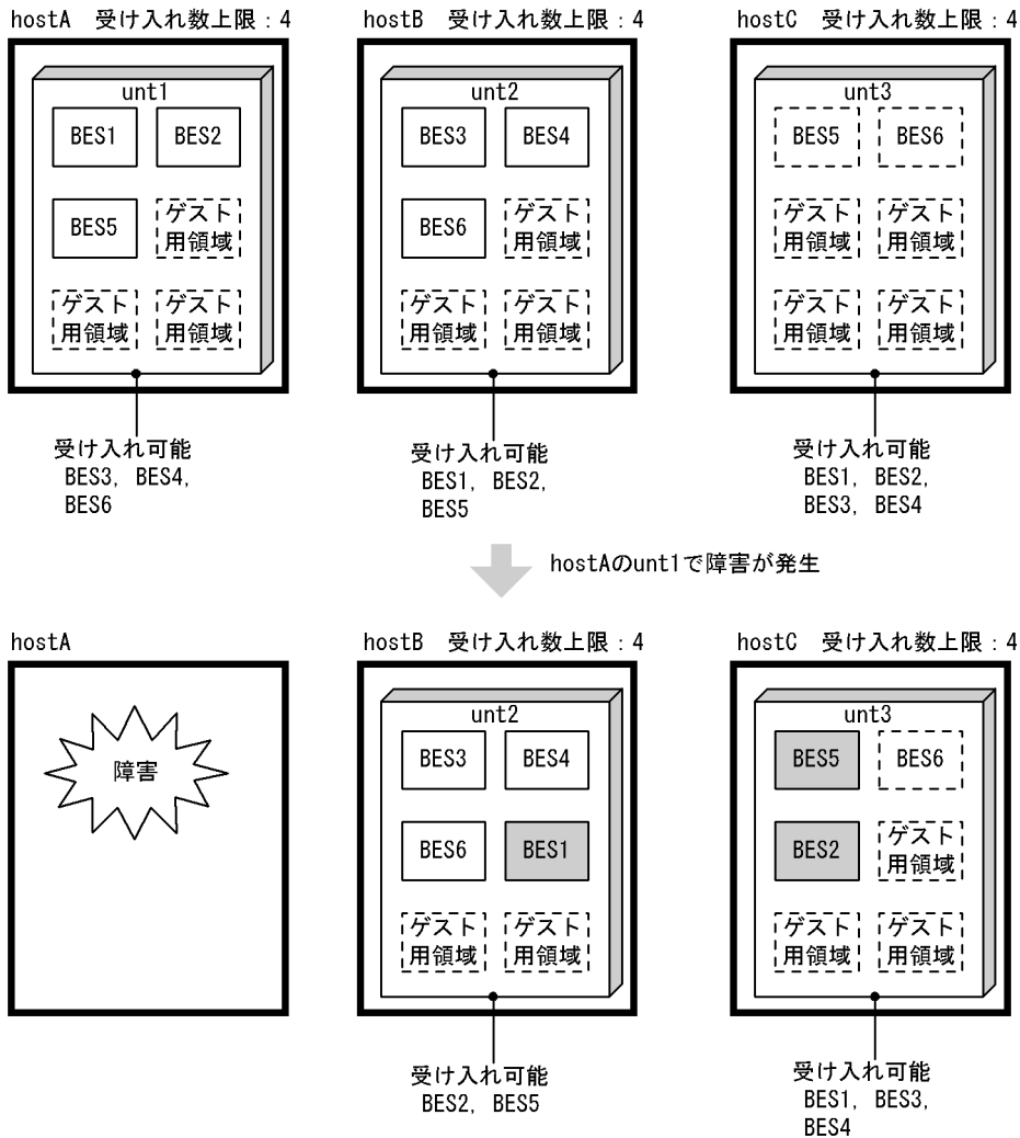
図 26-10 受け入れ中の系切り替えの例
