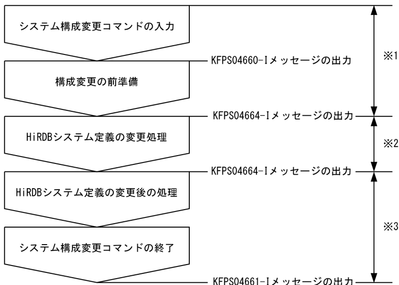
図 9-1 システム構成変更コマンド実行時にエラーが発生した場合の対処方法
