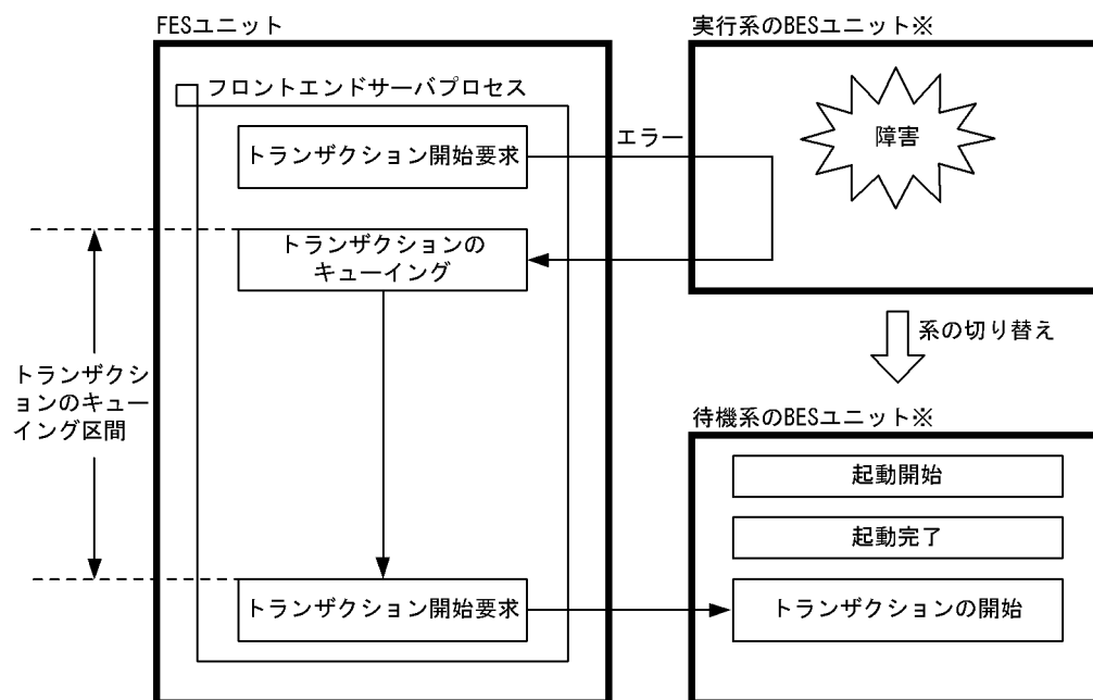
図 26-76 トランザクションキューイング機能の概要
