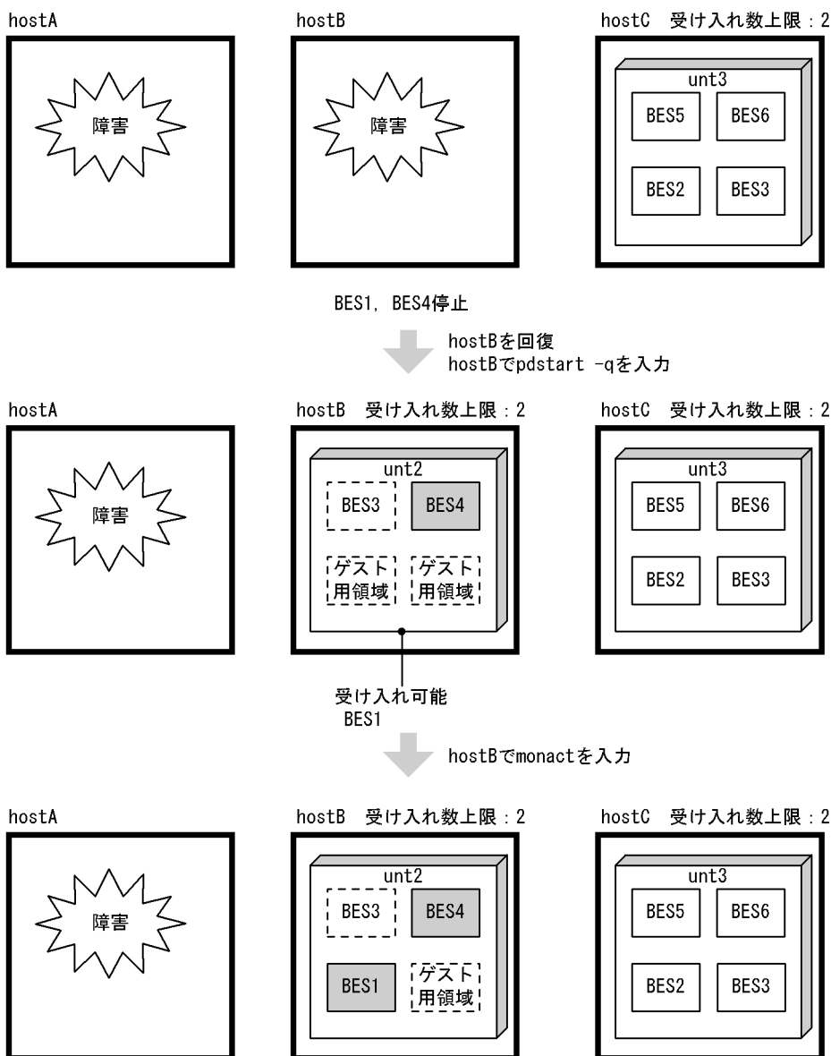
図 26-13 受け入れ数が不足した状態で障害が発生した場合の対処方法の例
