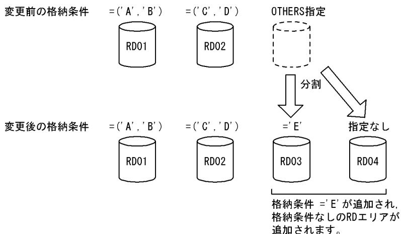
図 13-49 分割できるケース (その 8)
