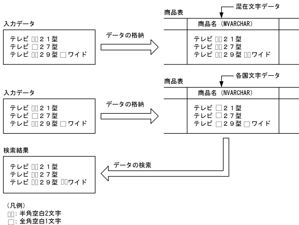
図 13-94 レベル 3 の処理方式
