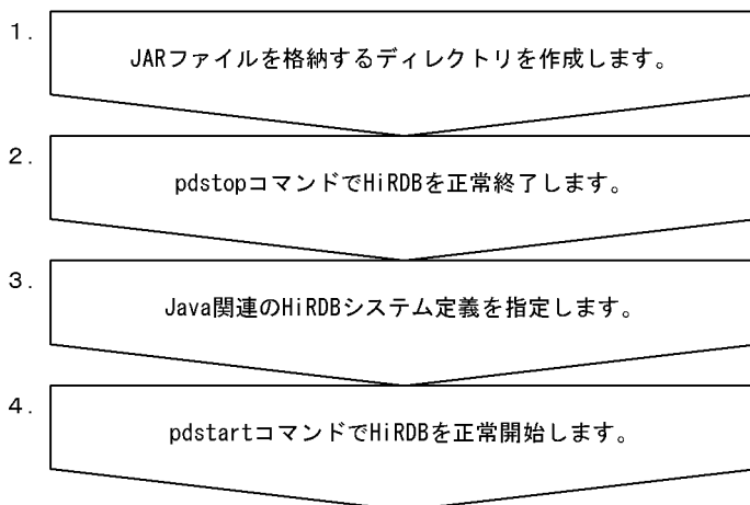
図 17-5 Java ストアドプロシジャ及び Java ストアドファンクションを使用する場合の環境設定手順
