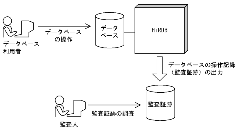
図 24-1 セキュリティ監査機能の概要
