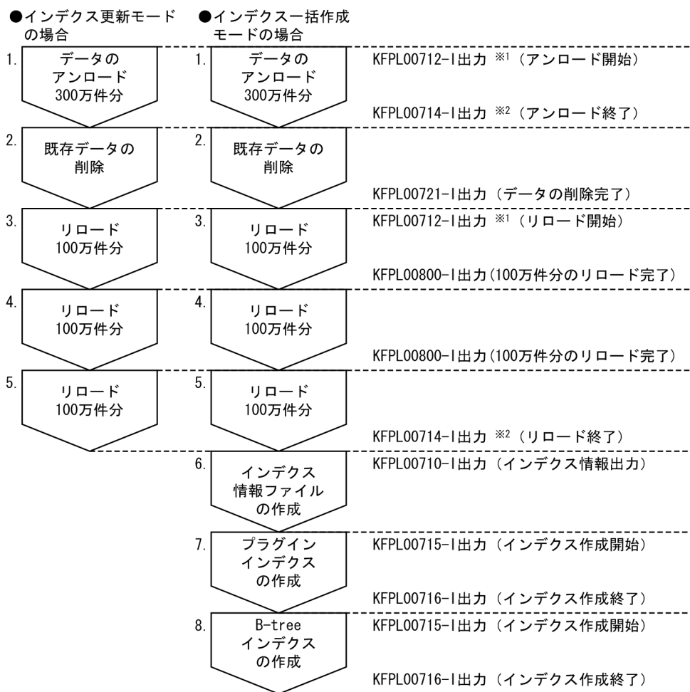
図 20-8 同期点指定の再編成実行中にユティリティが異常終了したときの対処方法
