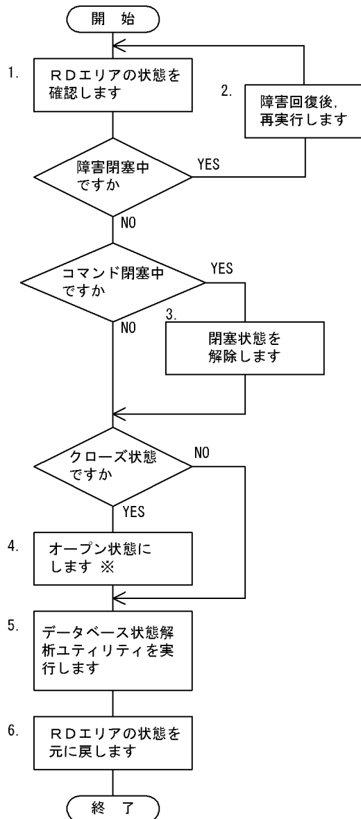
図 22-4 チューニング情報の取得手順（データベース状態解析ユティリティからチューニング情報を取得する場合）
