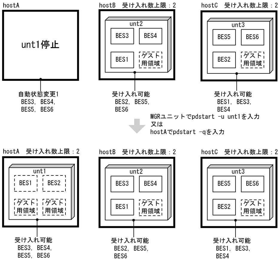
図 26-57 影響分散スタンバイレス型系切り替え機能での実行系のバックエンドサーバがないユニットの開始の例
