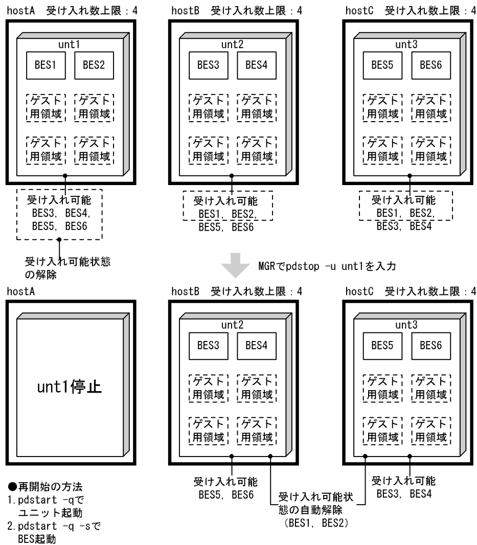
図 26-62 通常時のユニットの停止の例
