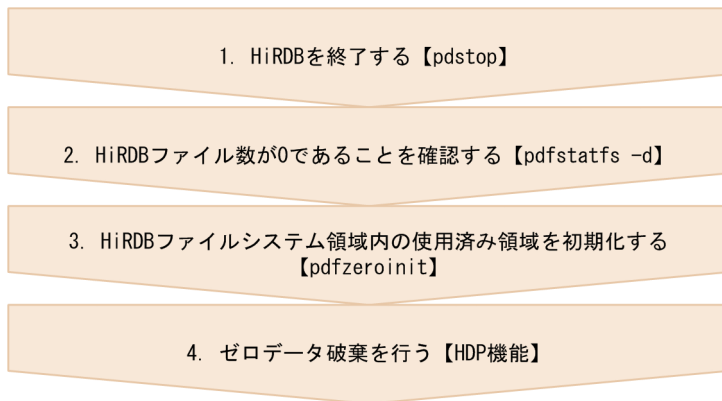
図 10-7 使用済み領域のディスク割り当てを解除する手順（作業表用ファイルを作成する SQL、ユーティリティの実行後）
