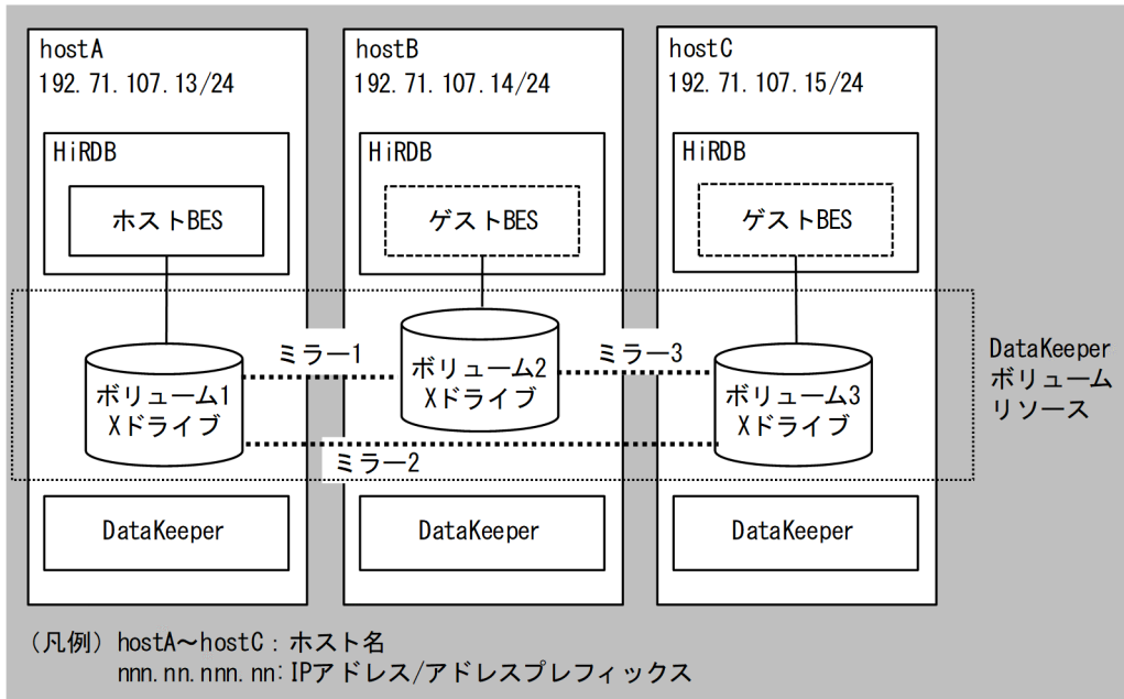
図 26-46 影響分散スタンバイレス構成での DataKeeper ボリュームリソースの例 (hostA のホスト BES に対して、hostB と hostC にゲスト BES を配置)
