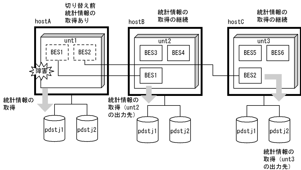
図 26-72 影響分散スタンバイレス型系切り替え機能の場合の系切り替え後の統計ログの取得の例
