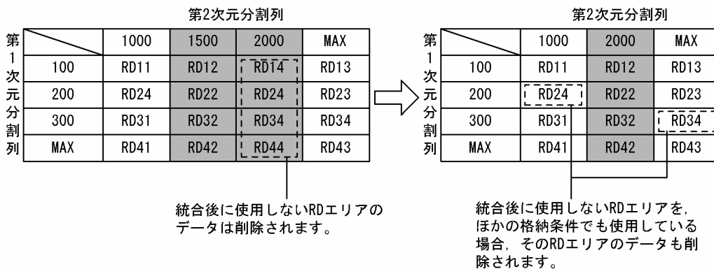
図 13-82 変更対象 RD エリアのデータの扱い（WITHOUT PURGE 指定がある場合）
