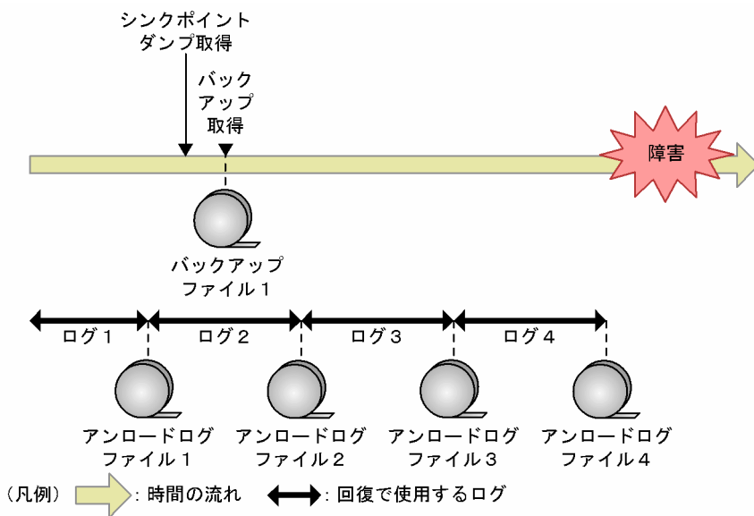
図 3-12 障害が発生した場合の例
