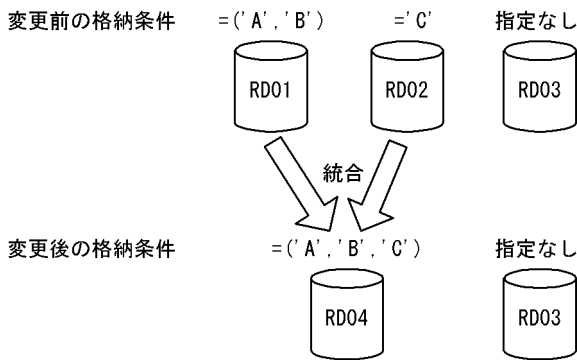
図 13-66 統合できるケース (その 7)
