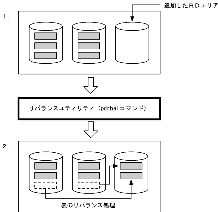
図 13-11 ハッシュ分割表のリバランス機能
