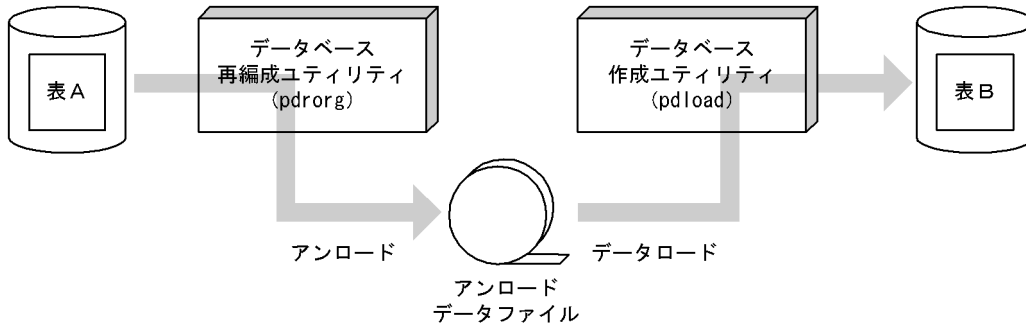
図 13-92 別表へのデータの移行方法
