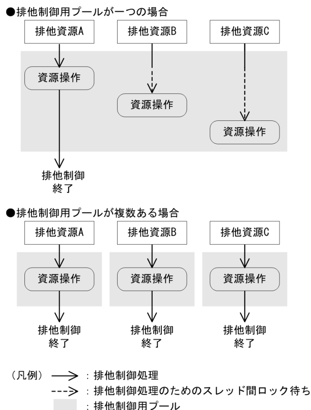
図 9-5 排他制御処理の分散
