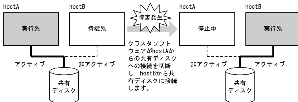
図 26-32 クラスタソフトウェアによる共有ディスクのアクセス制御
