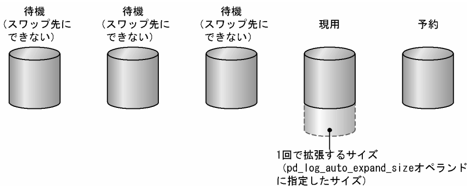
図 3-11 システムログファイルの自動拡張の概要 (契機 2 の場合)
