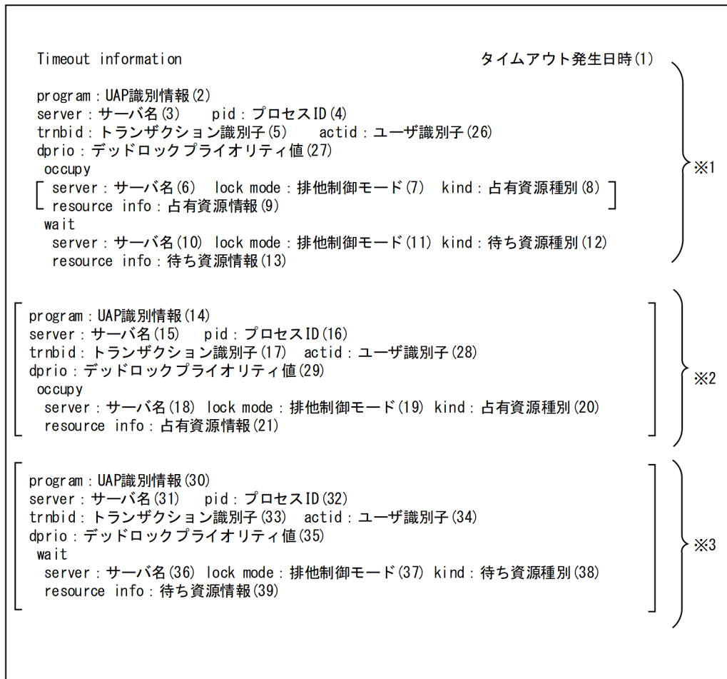
図 8-9 タイムアウト情報の出力内容
