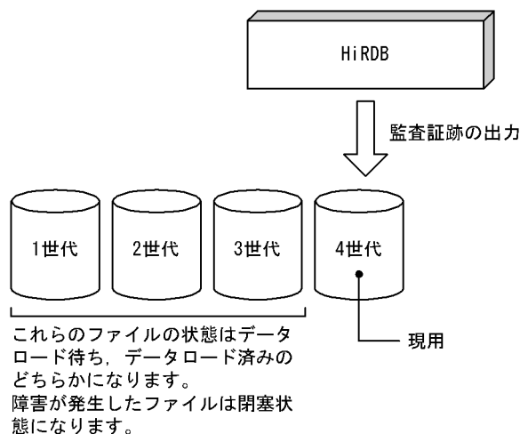
図 24-8 監査証跡ファイルの状態
