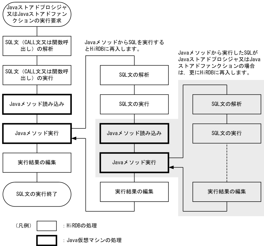
図 17-1 Java ストアドプロシジャ及び Java ストアドファンクションの動作（呼び出し処理の 手順）
