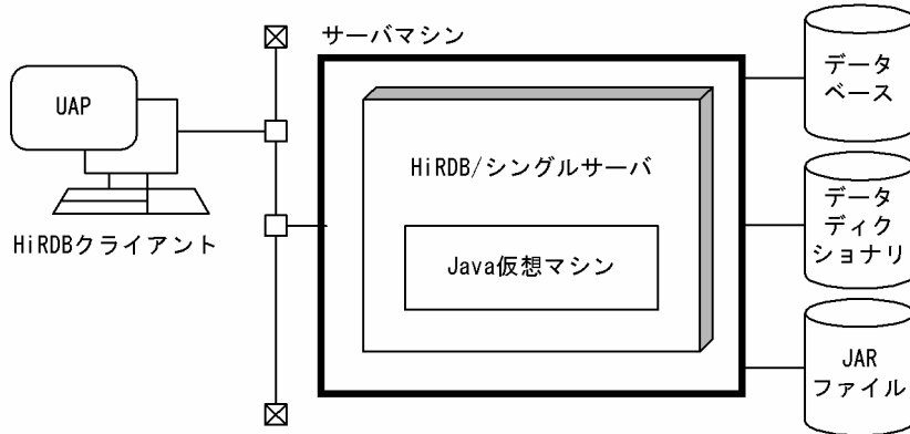
図 17-3 Java ストアドプロシジャ及び Java ストアドファンクション使用時のシステム構成（HiRDB/シングルサーバの場合）
