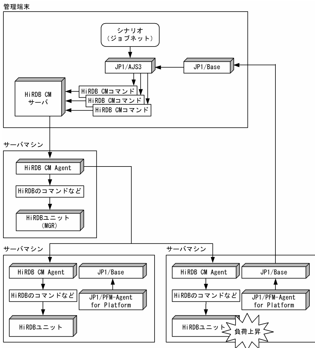
図 11-8 JP1/PFM によるバックエンドサーバの負荷監視と自動シナリオ実行
