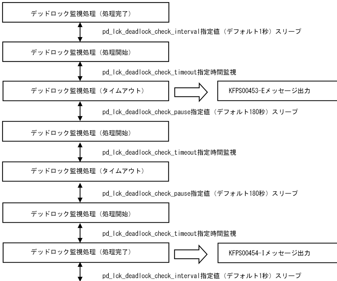
図 9-9 デッドロック監視処理を中断してから再開するまでの動作
