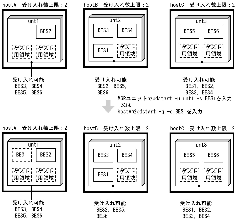
図 26-59 影響分散スタンバイレス型系切り替え機能での待機系サーバの開始の例
