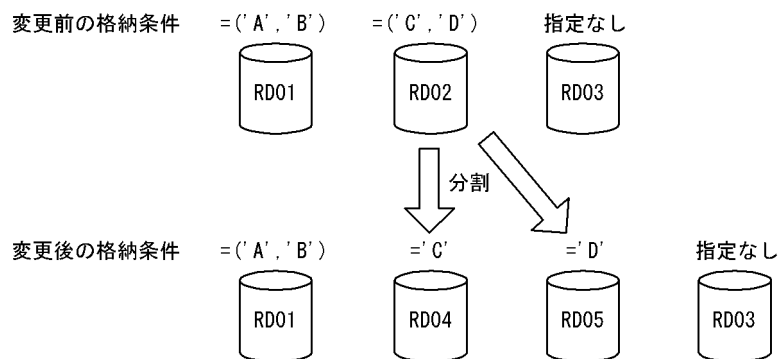
図 13-39 分割できるケース（その 1）
