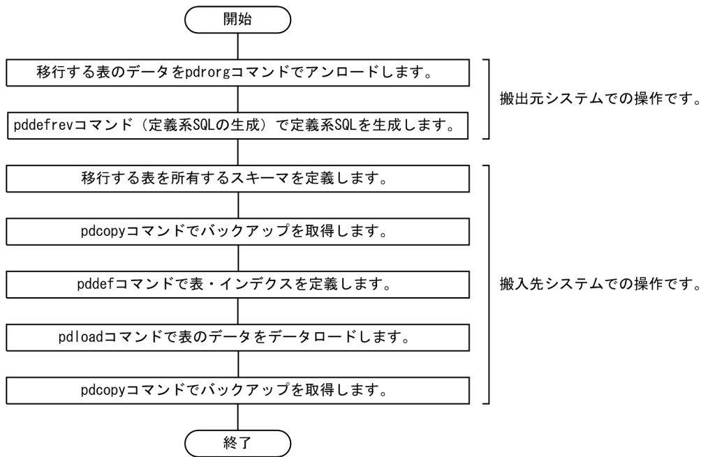
図 12-6 表定義情報と表データを別々にほかの HiRDB システムに移行する手順
