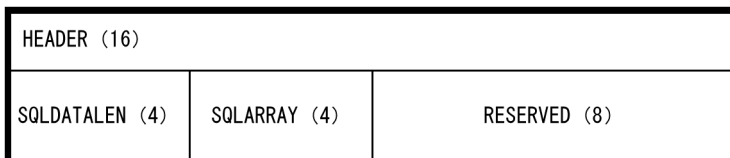
図 24-25 HEADER 領域の構造
