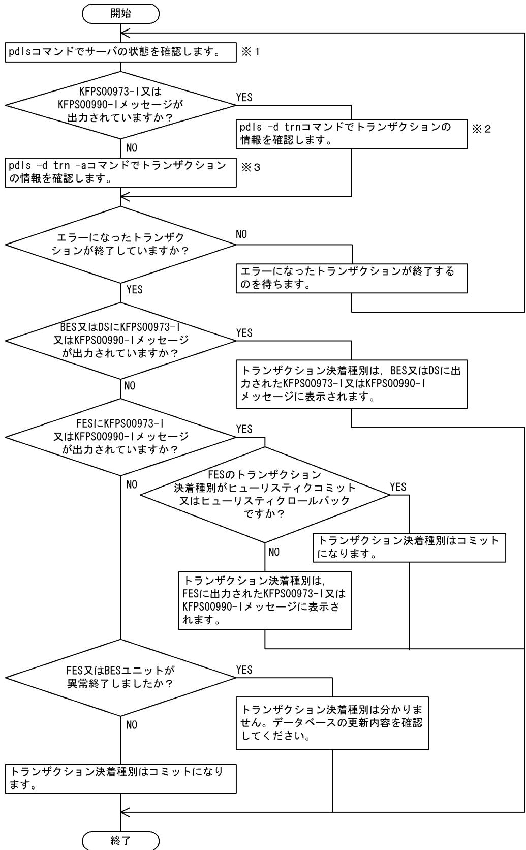
図 20-10 障害が発生したときのトランザクション決着種別の確認方法
