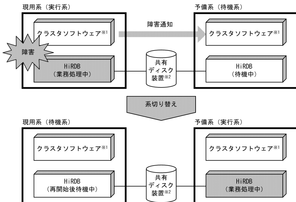
図 26-2 系切り替え機能（スタンバイ型系切り替え機能）の概要
