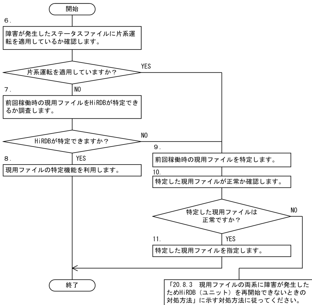
図 20-2 ステータスファイルに障害が発生したときの対処方法
