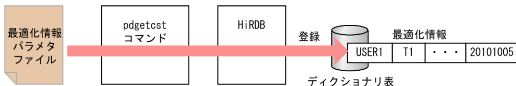
図 19-2 最適化情報パラメタファイルを使用した最適化情報の登録
