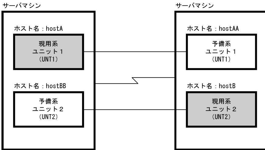
図 26-21 ホスト名の設定例（正しい例）
