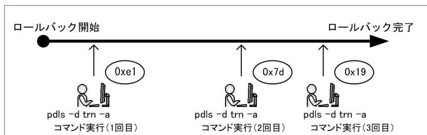
図 8-16 ロールバック処理が進行中の例 (pdls -d trn -a コマンドの場合)
