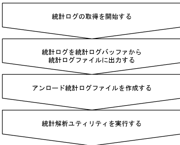
図 22-2 チューニング情報の取得手順（統計ログからチューニング情報を取得する場合）
