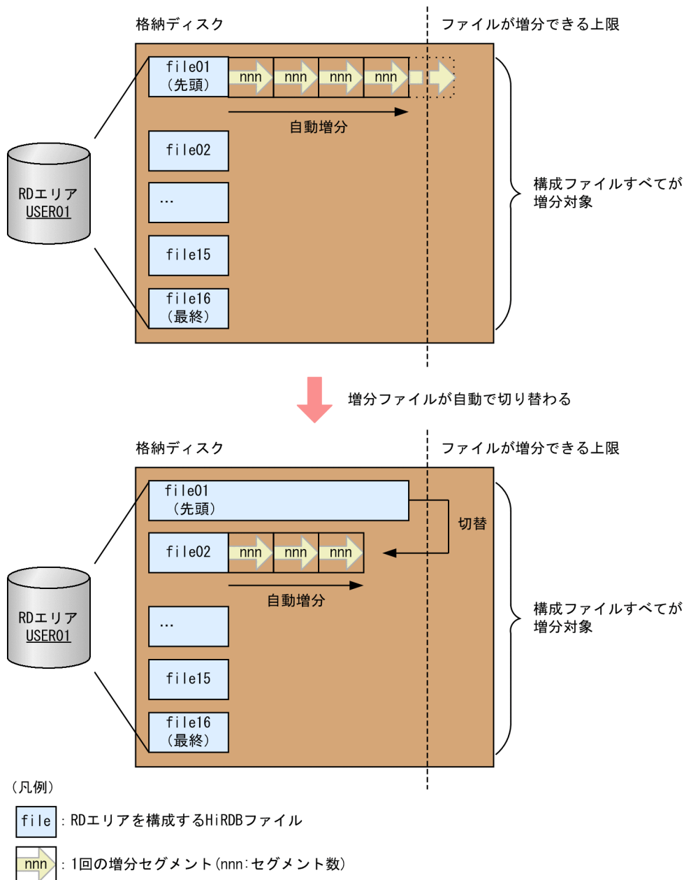
図 15-6 pd_rdarea_extension_file=all を選択した運用例
