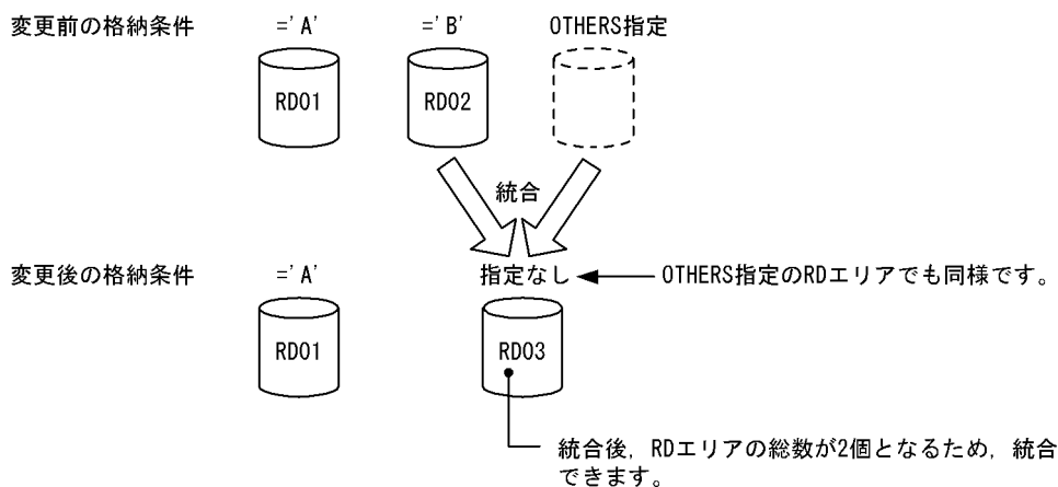
図 13-60 統合できるケース (その 3)
