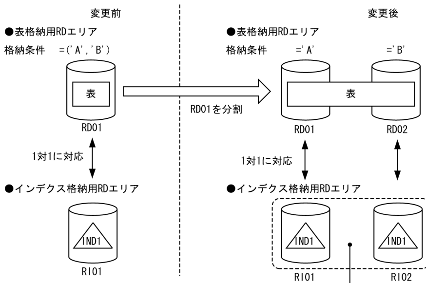
図 13-19 表格納用 RD エリアを分割できないケース (その 1)
