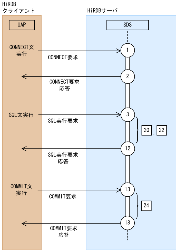
図 28-3 PRF トレースの取得ポイントの概念図 (HiRDB/シングルサーバの場合)
