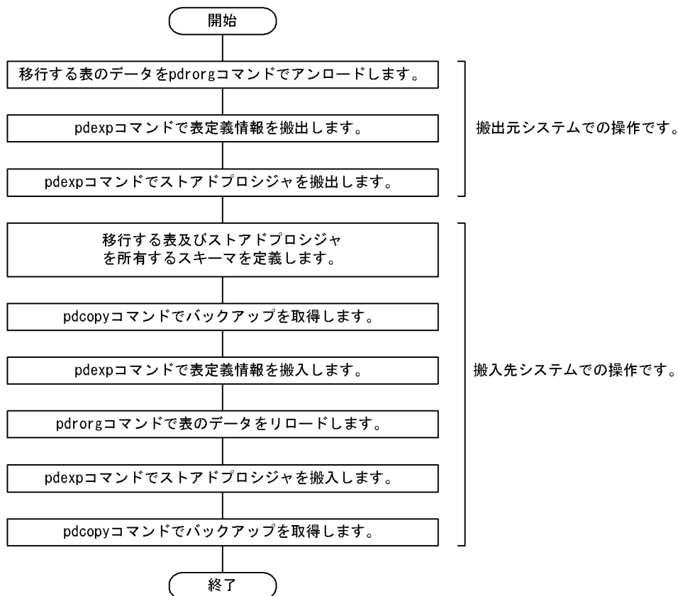
図 12-11 ストアドプロシジャの移行手順
