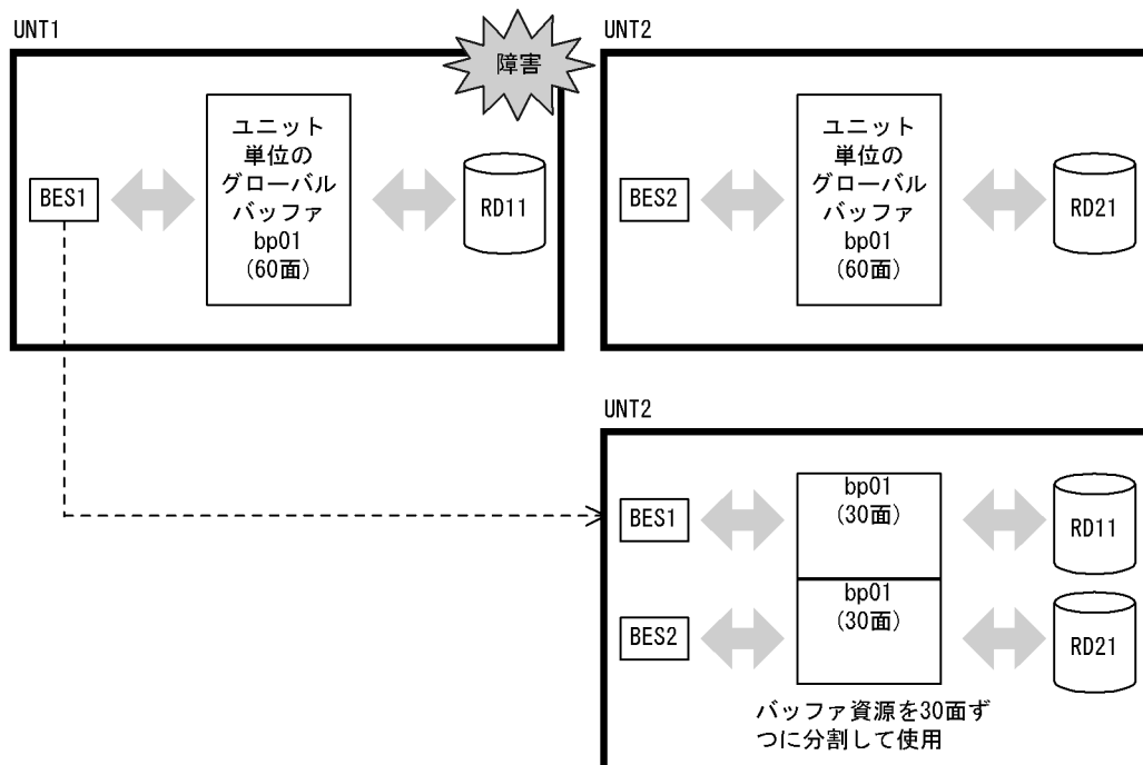
図 26-44 ユニット単位のグローバルバッファの共用イメージ
