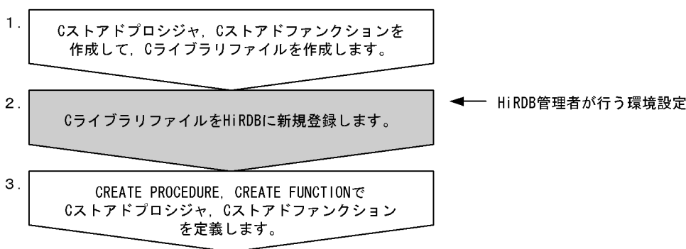
図 18-1 Cストアードプロシジャ又はCストアードファンクションの実行環境を作成するまでの流れ
