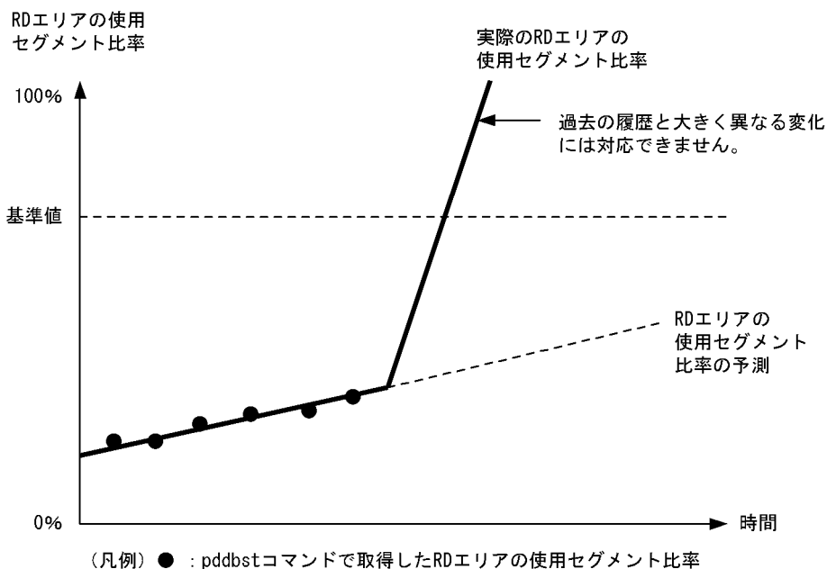
図 13-9 データの格納状態が急激に変化するため正しい予測ができない例
