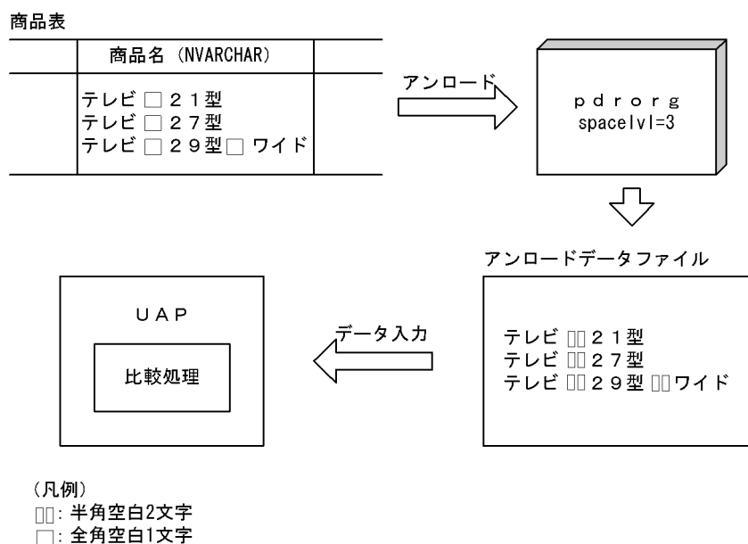
図 13-98 -W オプション指定で出力したアンロードデータを UAP で使用する場合
