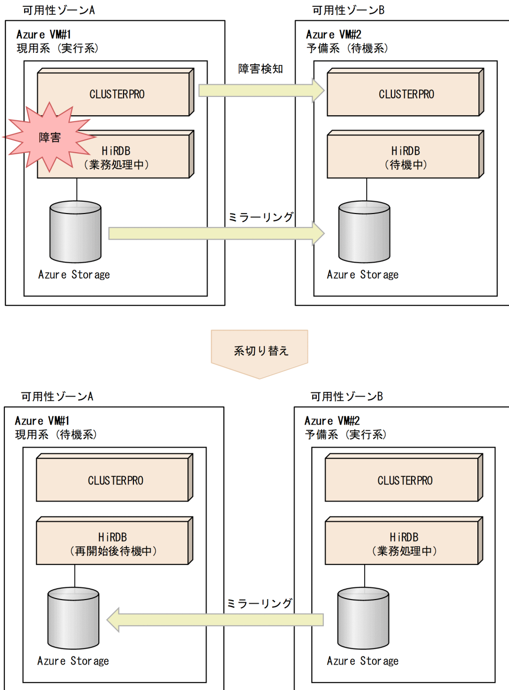
図 26-53 Microsoft Azure 環境上のミラーディスクを使用したクラスタ構成概要図
