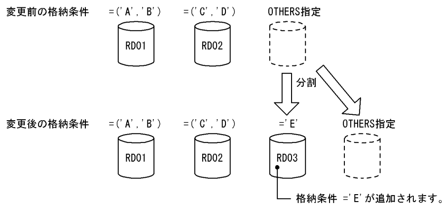
図 13-48 分割できるケース (その 7)
