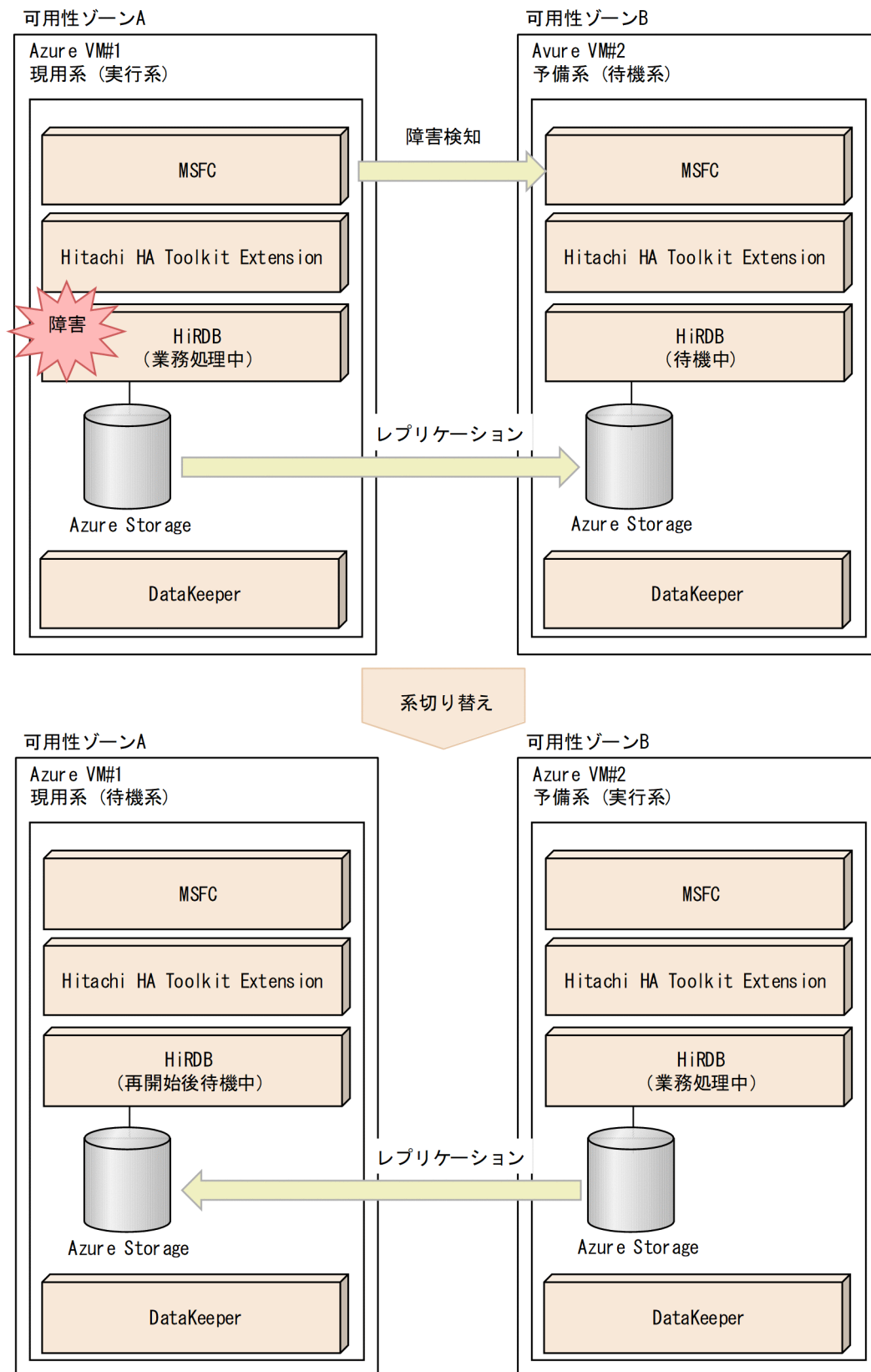
図 26-48 Microsoft Azure 環境上のクラスタ構成概要図
