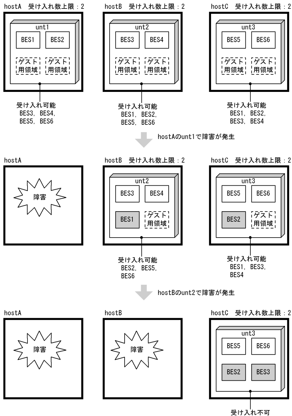
図 26-12 多重障害時の系切り替えで受け入れ数が不足する場合の例
