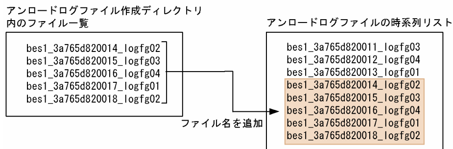
図 3-14 アンロードログファイルの時系列リストの作成方法
