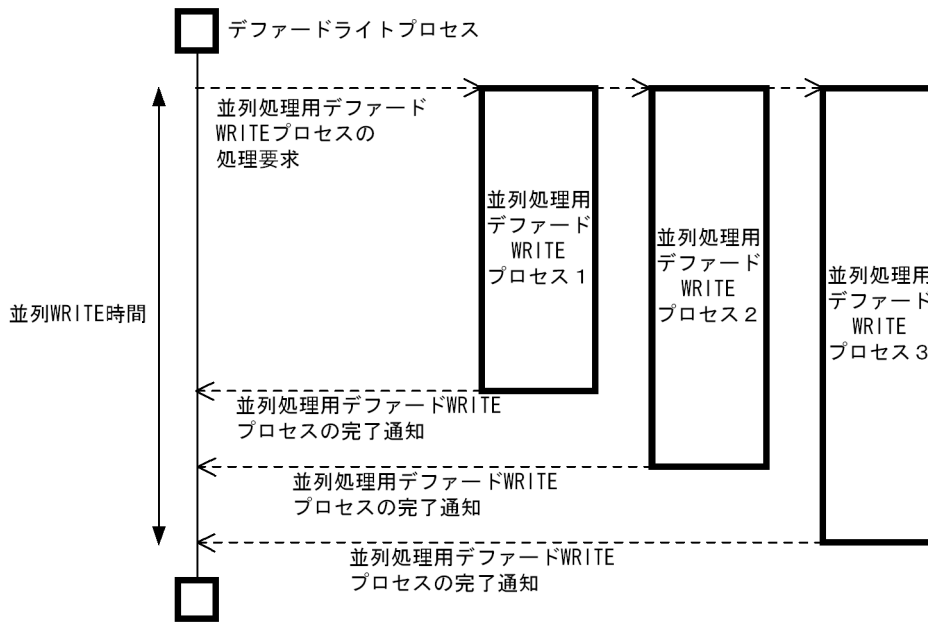
図 23-1 並列 WRITE 時間の概念
