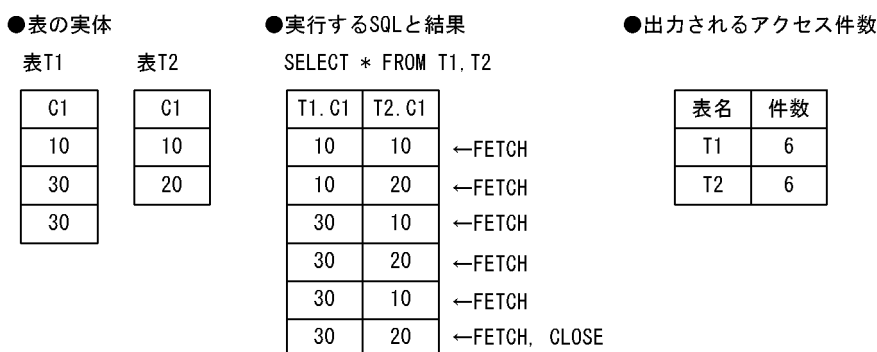
図 24-11 アクセス件数の出力例 (その 2)
