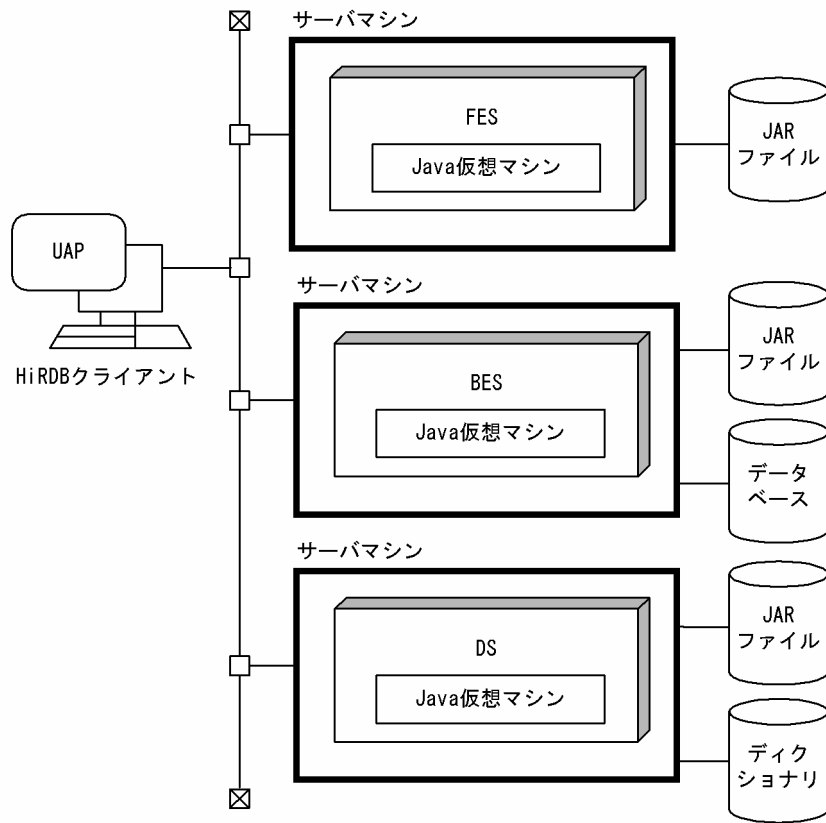
図 17-4 Java ストアドプロシジャ及び Java ストアドファンクション使用時のシステム構成 (HiRDB/パラレルサーバの場合)
