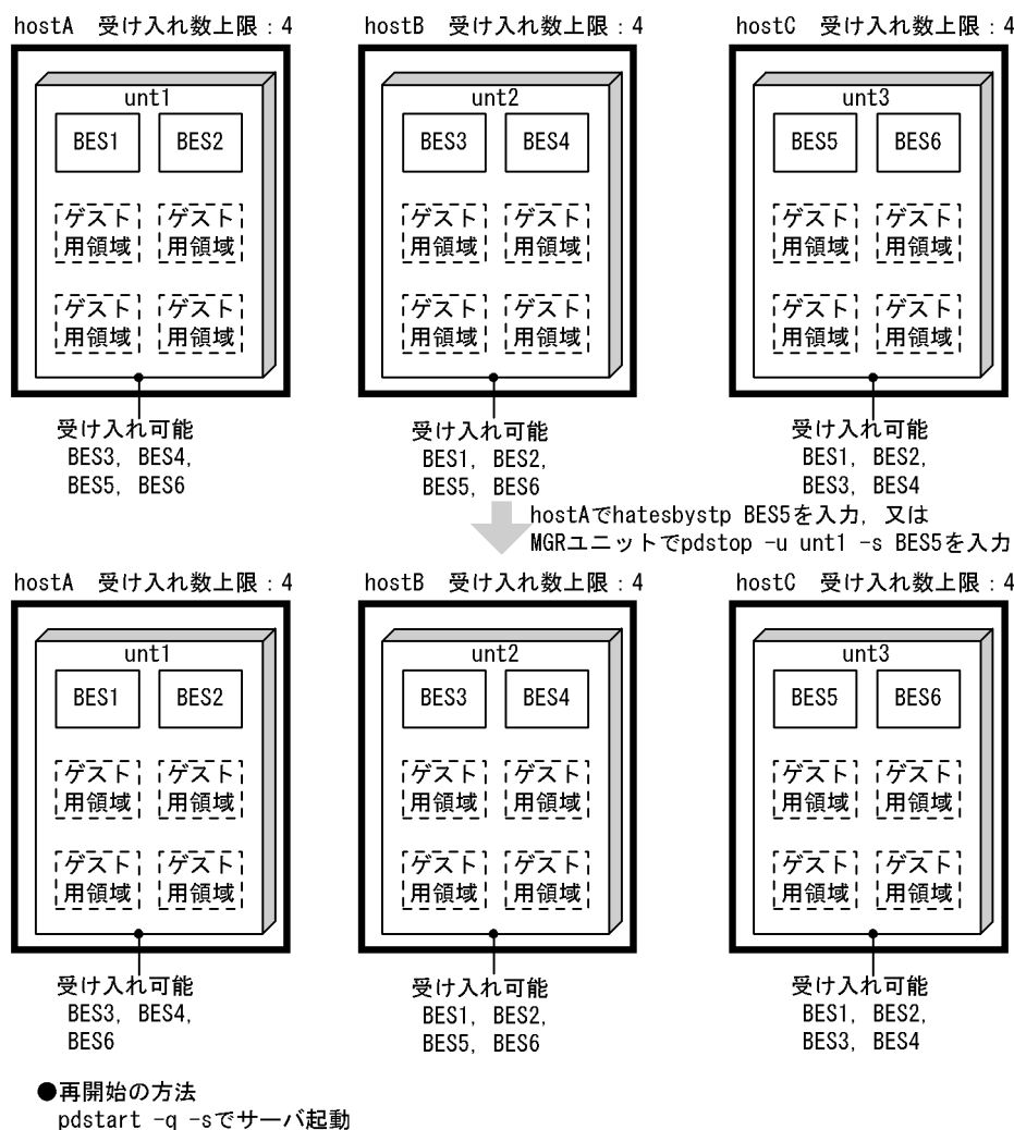
図 26-67 ゲスト BES の受け入れ可能状態の解除の例
