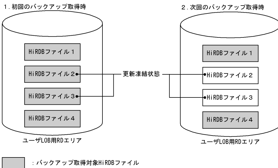
図 6-4 更新凍結コマンドのバックアップ取得への利用方法
