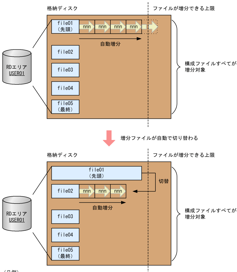
図 15-3 pd_rdarea_extension_file=all の方式
