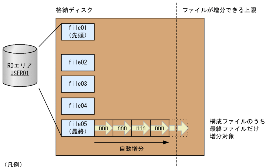
図 15-2 pd_rdarea_extension_file=last の方式
