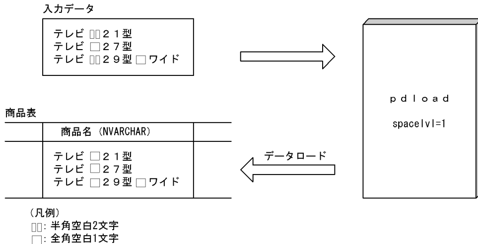
図 13-96 新規データの空白文字を統一する方法
