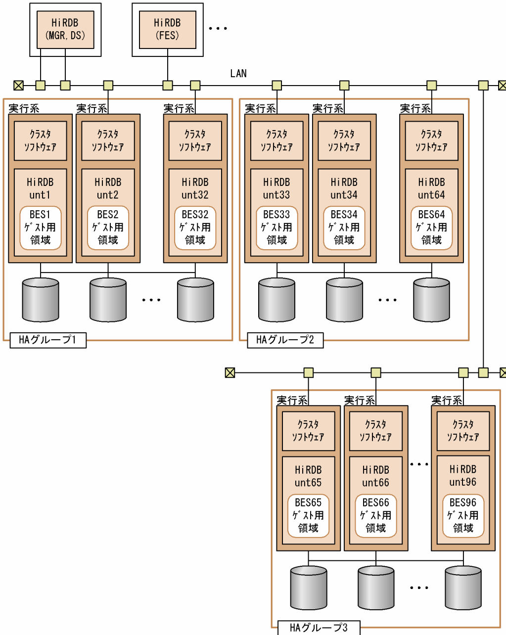
図 26-28 HA グループを複数定義している場合の影響分散スタンバイレス型系切り替えのシステム構成例
