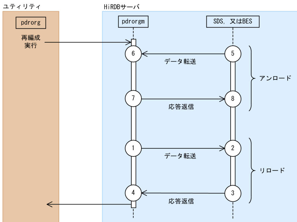
図 28-6 PRF トレースの取得ポイントの概念図 (pdrorg)
