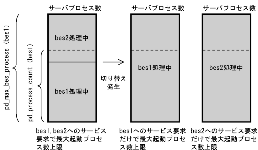
図 26-39 1：1 スタンバイレス型系切り替えでの系切り替え発生後のサーバプロセスの割り当て（その 2）
