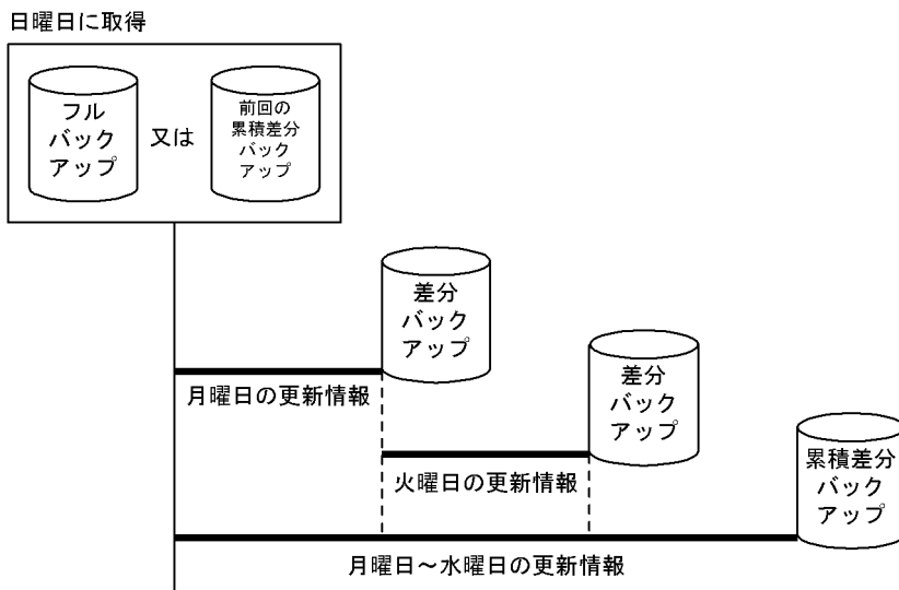
図 6-2 累積差分バックアップの概念
