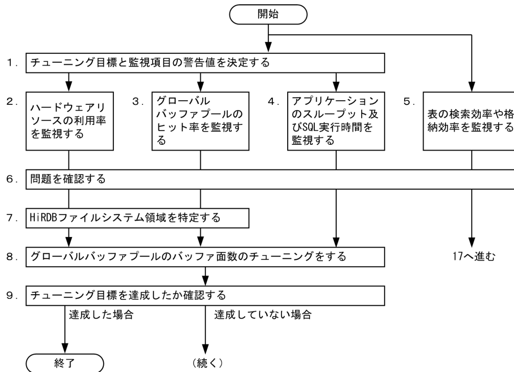
図 23-2 SQL のチューニングの流れ
