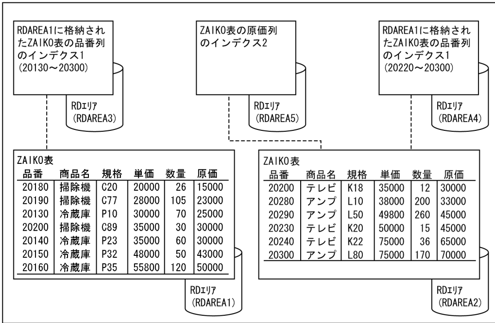
図 11-4 表に非横分割インデクスを定義している場合の移行方法
