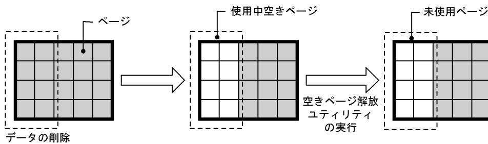
図 15-10 使用中空きページの解放
