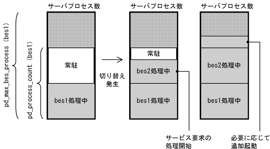
図 26-38 1：1 スタンバイレス型系切り替えでの系切り替え発生後のサーバプロセスの割り当て（その 1）
