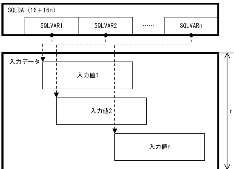
図 24-26 SQLDA 及び入力データ領域の構造
