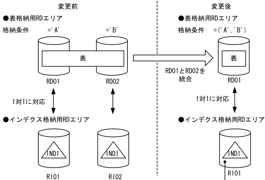
図 13-20 表格納用 RD エリアを分割できないケース (その 2)
