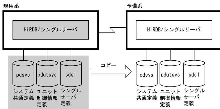
図 26-33 スタンバイ型系切り替え機能使用時の HiRDB システム定義ファイルの構成例 (HiRDB/シングルサーバの場合)
