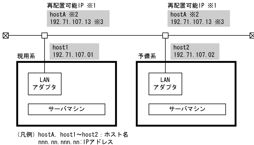
図 26-29 IP アドレスを引き継ぐ場合のネットワーク構成例
