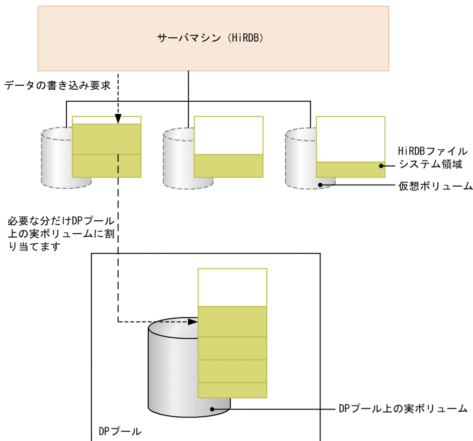
図 10-2 HDP 機能の概要
