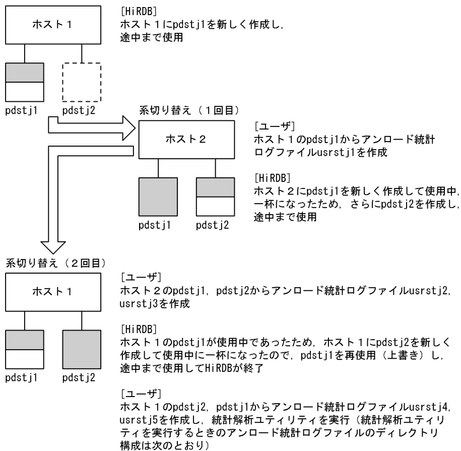
図 26-69 系切り替え機能使用時のアンロード統計ログファイルの作成例（その 1）
