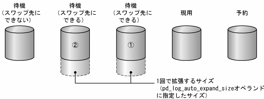
図 3-10 システムログファイルの自動拡張の概要 (契機 1 の場合)
