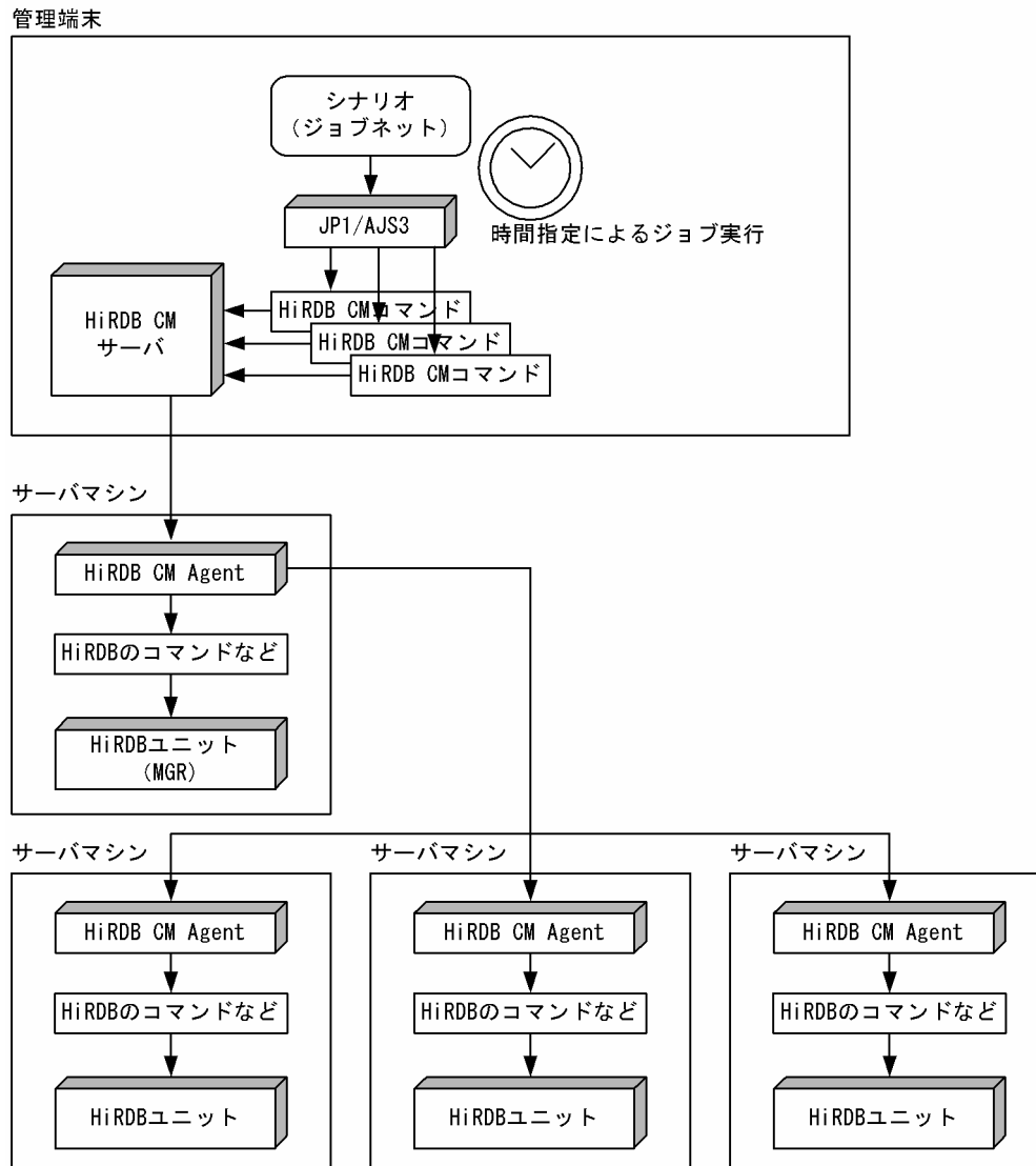
図 11-6 JP1/AJS3 によるシナリオ定期実行
