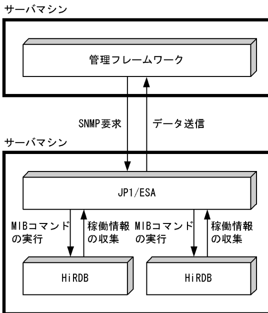
図 27-4 HiRDB/シングルサーバのマルチ HiRDB 構成に適用する場合のシステム構成
