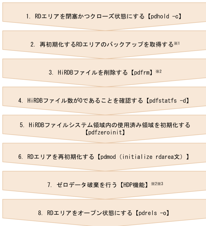
図 10-4 使用済み領域のディスク割り当てを解除する手順 (RD エリアの再初期化時)
