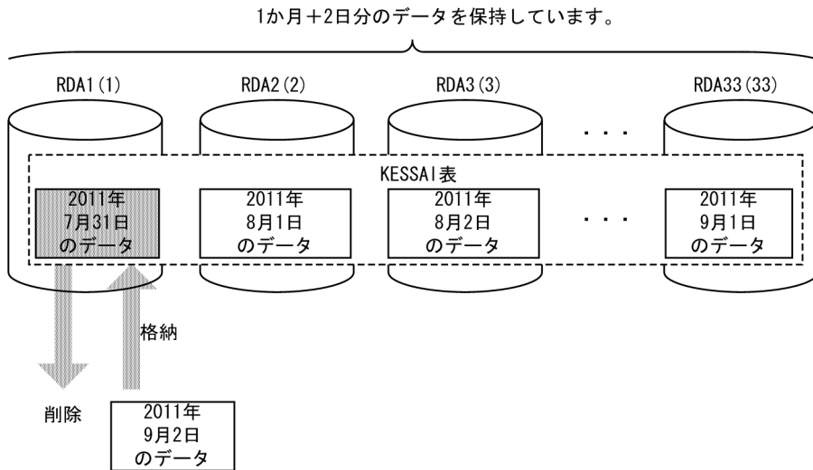
図 13-90 RD エリアを年月日単位に循環させて割り当てる場合（マトリクス分割でない場合）
