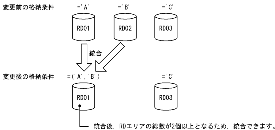
図 13-62 統合できるケース (その 5)
