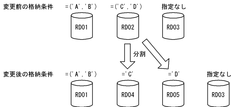
図 13-36 格納条件を指定していない RD エリアを分割する例
