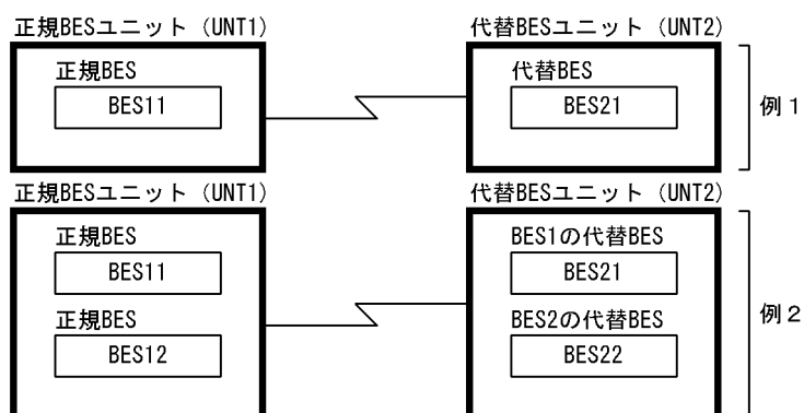
図 26-6 正規 BES ユニット及び代替 BES ユニットの正しい構成例
