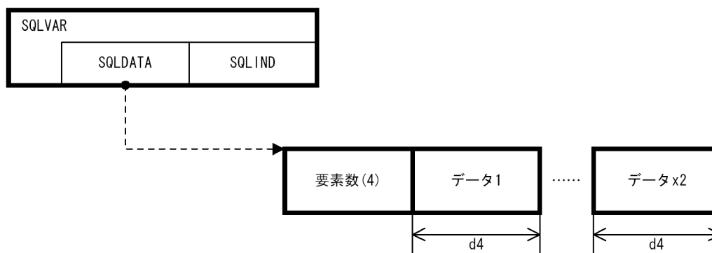
図 24-30 繰返し構造の入力値 (標識変数なし) の構造
