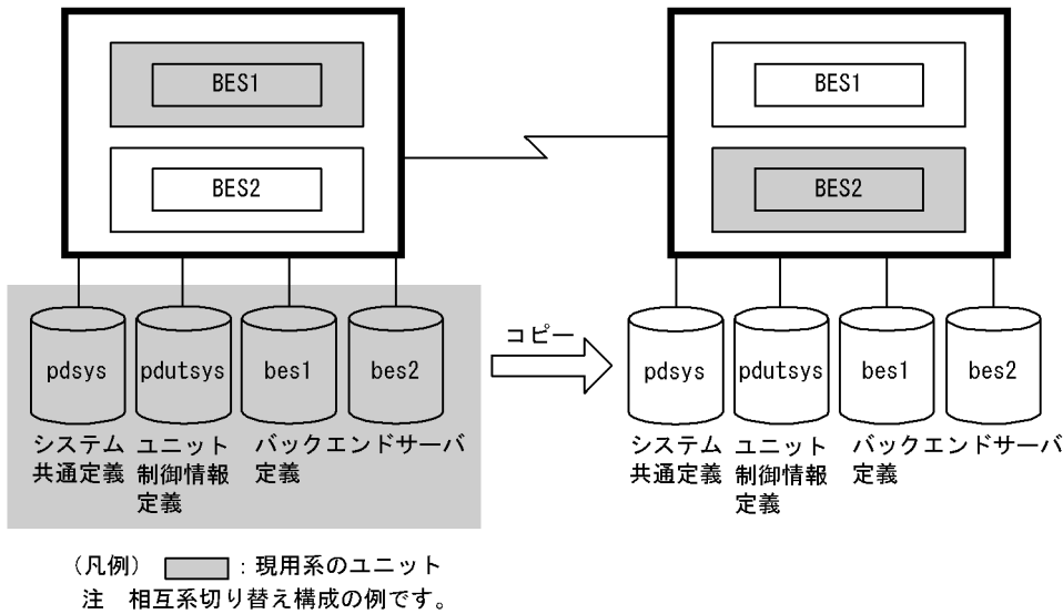
図 26-34 スタンバイ型系切り替え機能使用時の HiRDB システム定義ファイルの構成例 (HiRDB/ 平行サーバの場合)
