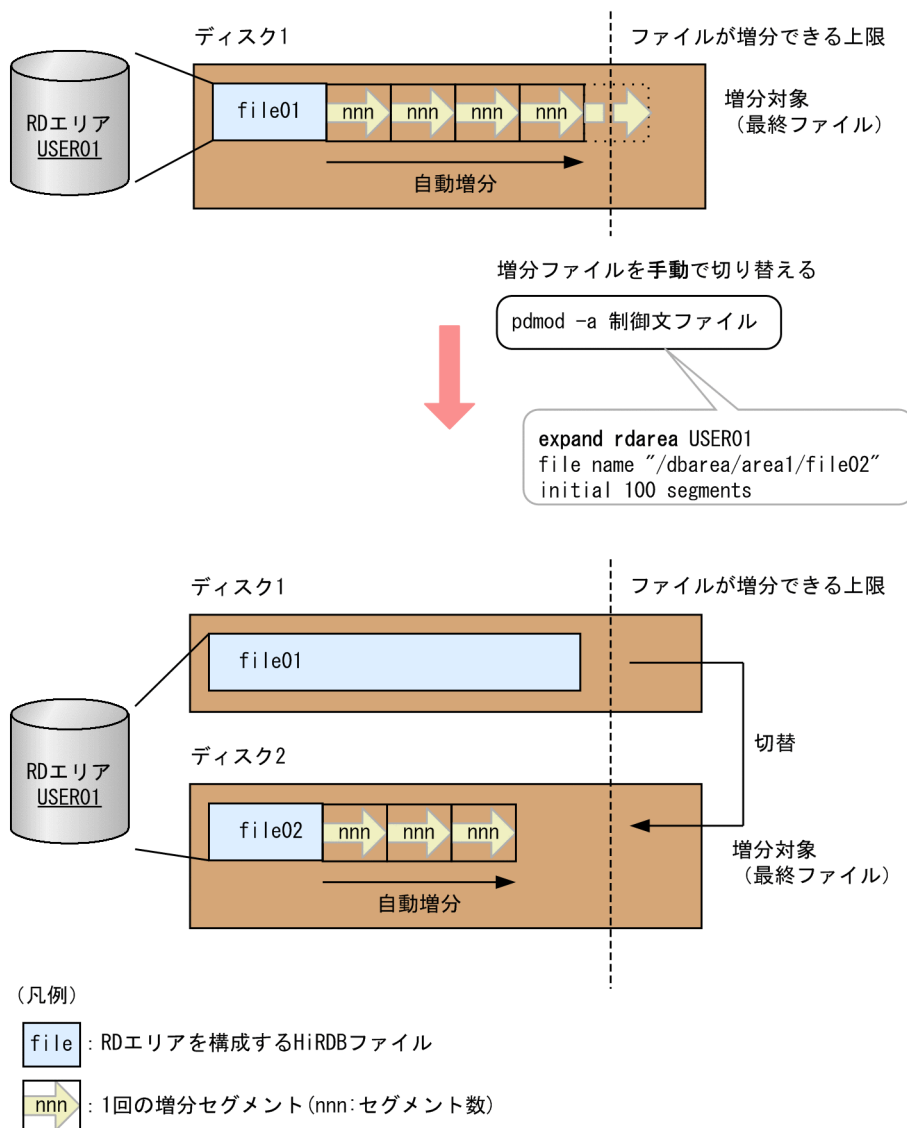
図 15-5 pd_rdarea_extension_file=last を選択した運用例
