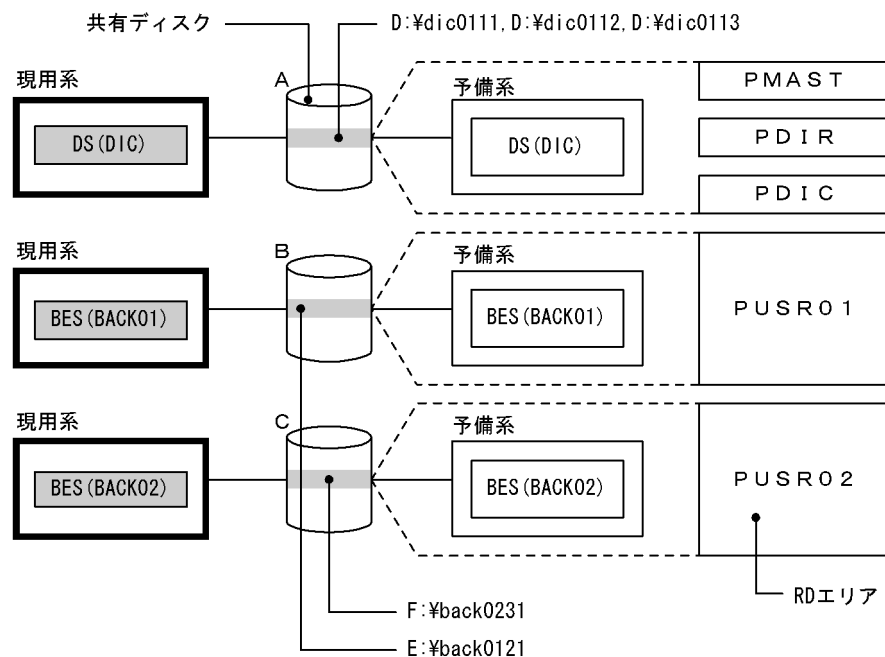
図 26-43 HiRDB/パラレルサーバのシステム構成例
