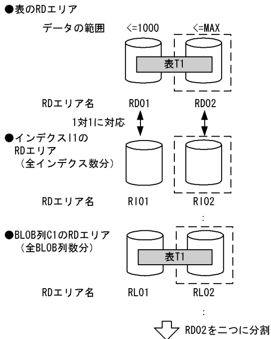
図 13-27 WITHOUT PURGE 指定なしの場合のデータの削除対象 RD エリアの例
