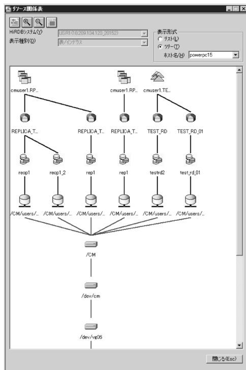
図 23-3 HiRDB CM による関係情報の取得例
