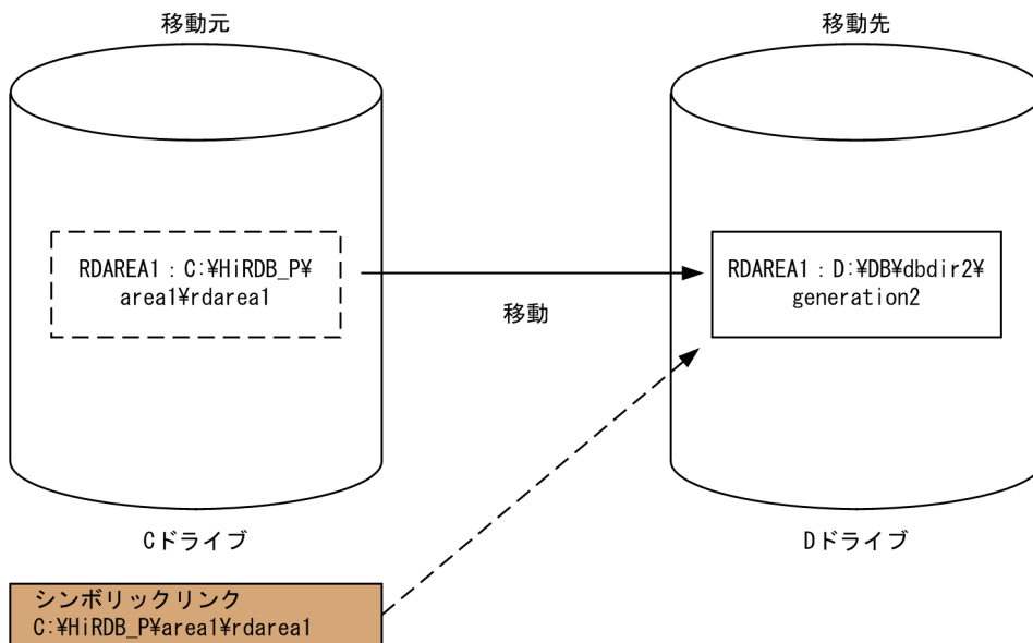
図 15-7 シンボリックリンクを使用した HiRDB ファイルシステム領域の移動
