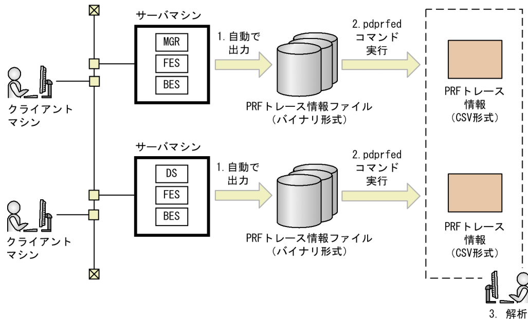
図 28-1 PRF トレース機能の概要（HiRDB/パラレルサーバの場合）
