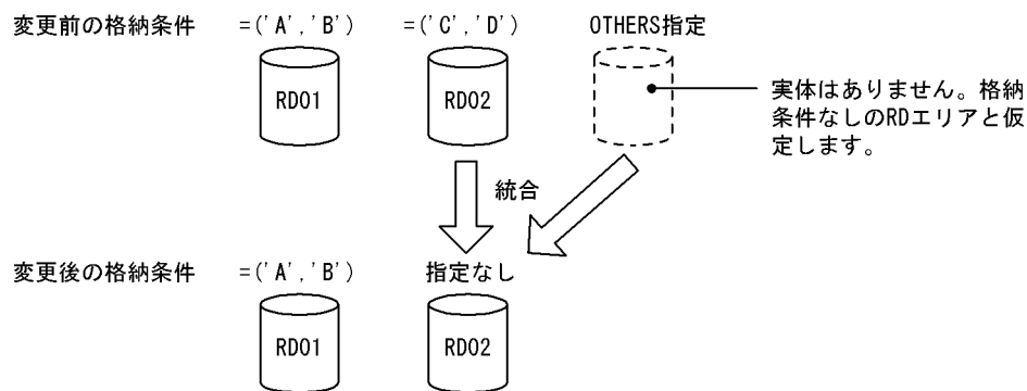
図 13-57 OTHERS 指定の RD エリアを統合できない例
