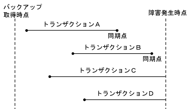
図 21-2 回復の対象になるトランザクション (障害発生直前の最新の同期点に回復する場合)
