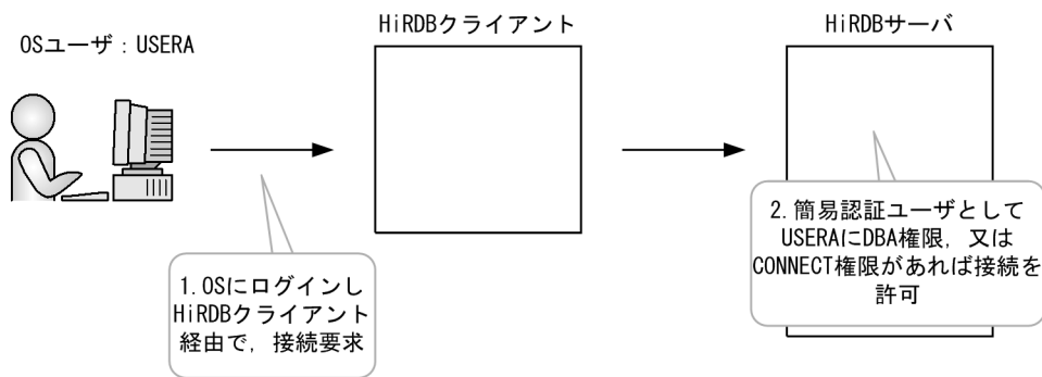
図 2-2 OS ログインユーザの簡易認証機能を使用した際の HiRDB サーバへの接続時の流れ
