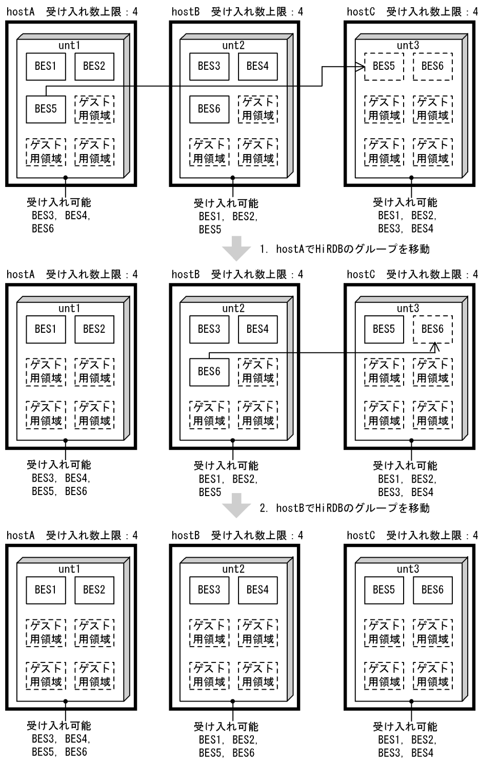
図 26-74 ゲスト BES に対する計画系切り替え (系の切り戻し) の例
