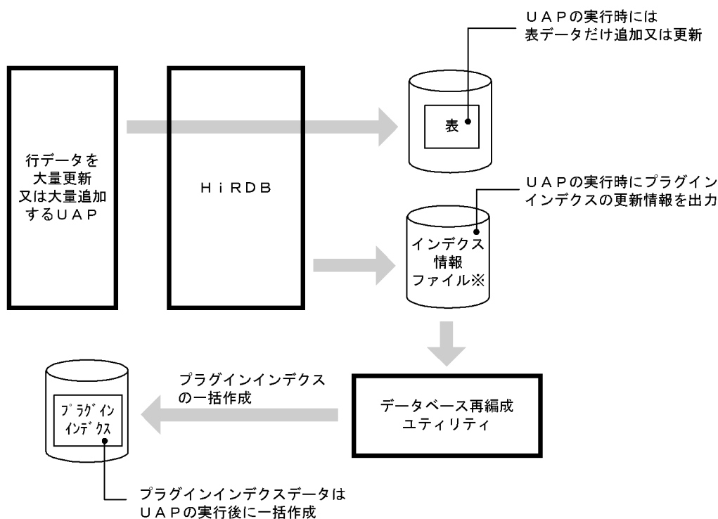
図 14-5 プラグインインデックスの遅延一括作成
