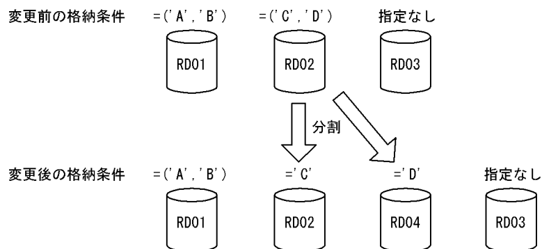
図 13-41 分割できないケース (その 1)
