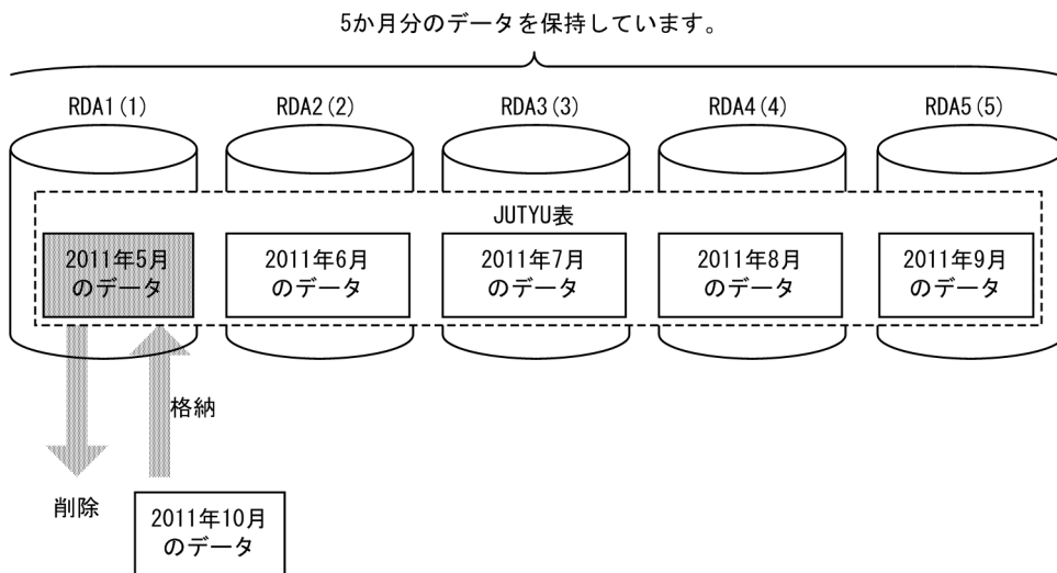
図 13-88 RD エリアを年月単位に循環させて割り当てる方法 (マトリクス分割ではない場合)
