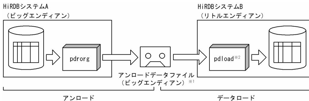
図 12-7 エンディアンが異なるシステム間の表データの移行
