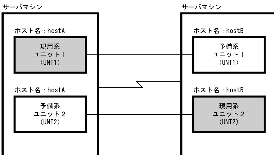
図 26-22 ホスト名の設定例（間違っただ例）
