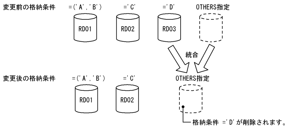
図 13-72 統合できるケース (その 12)
