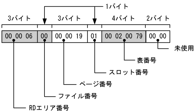
図 8-11 資源情報の出力例 (資源種別 0007 の場合)
