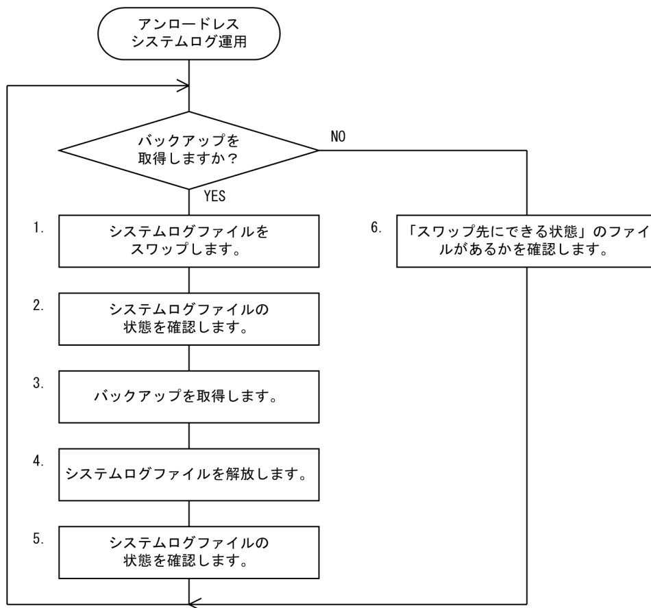
図 3-4 アンロードレスシステムログ運用の手順 (HiRDB/シングルサーバの場合)
