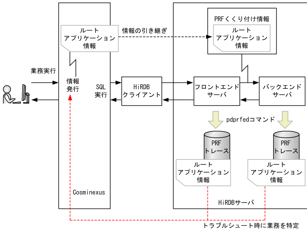
図 28-2 Cosminexus と連携した PRF トレース情報の取得例
