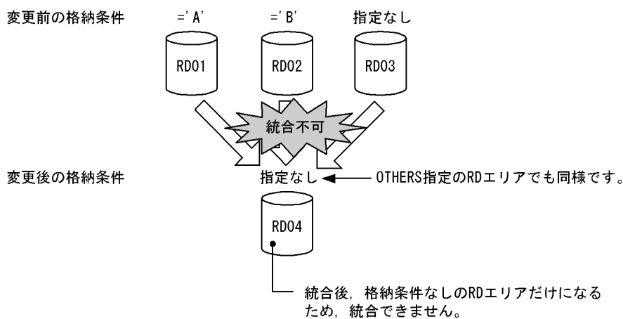
図 13-63 統合できないケース (その 1)
