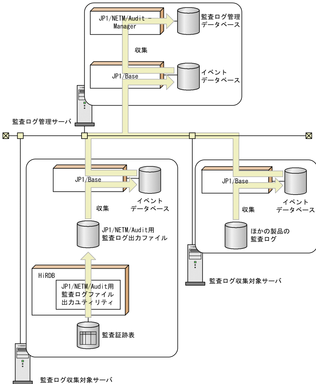
図 24-35 JP1/NETM/Audit との連携の概要
