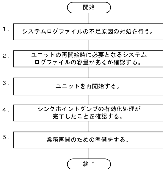
図 20-6 システムログファイルの不足原因が特定されている場合の対処手順（フロー）
