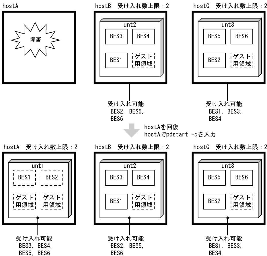
図 26-14 受け入れ数の不足を回避する方法の例
