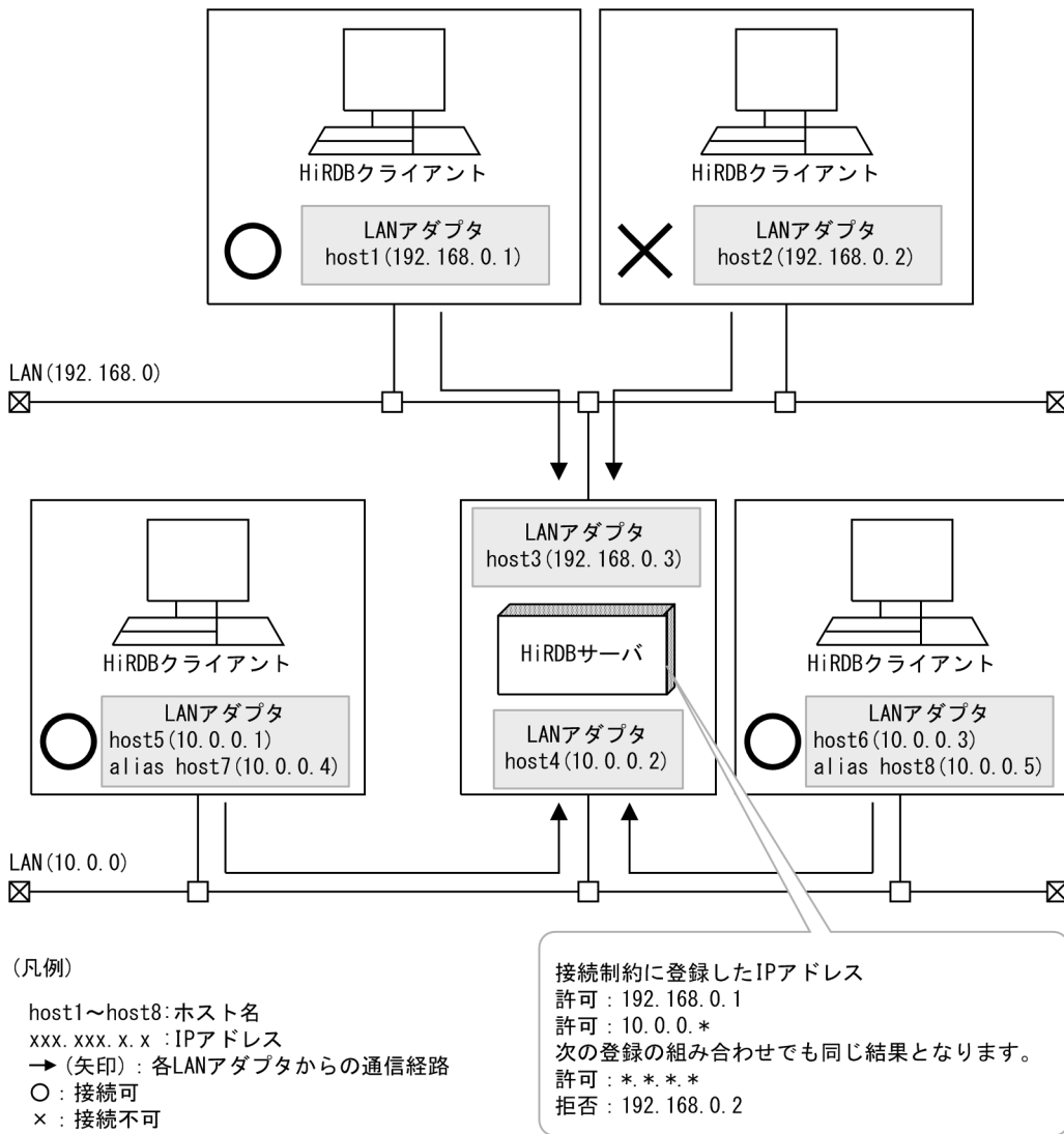
図 25-1 IP アドレスによる接続制限機能の概要
