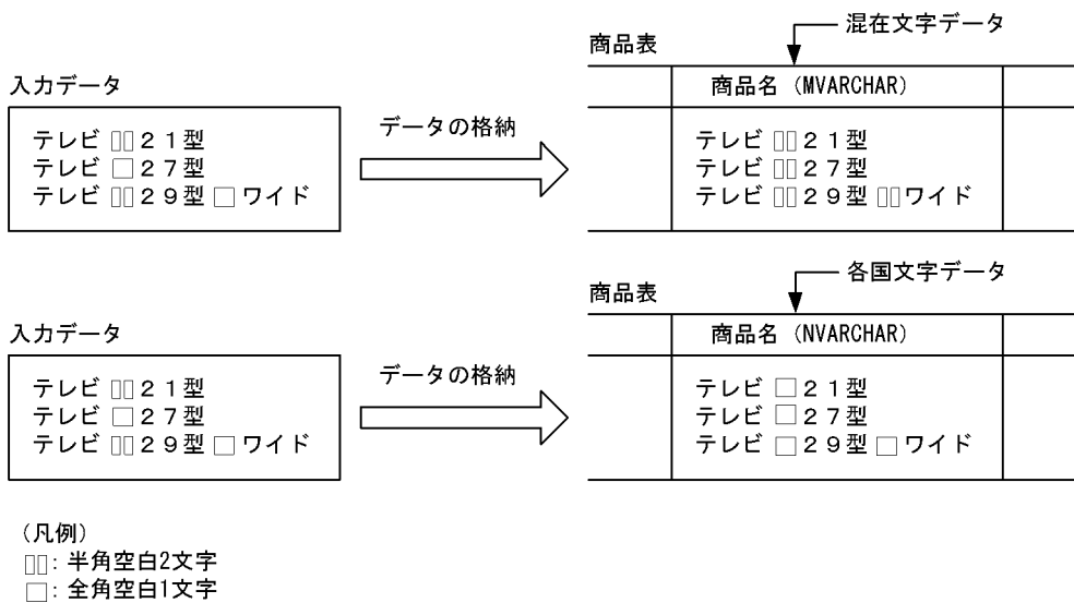
図 13-93 レベル 1 の処理方式
