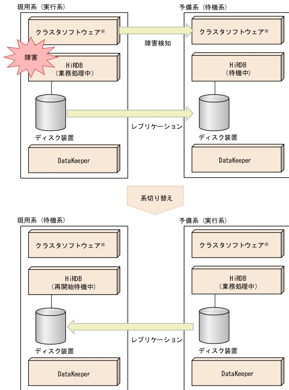
図 26-3 DataKeeper による複製ディスク使用時の系切り替え機能（スタンバイ型系切り替え機能）の概要
