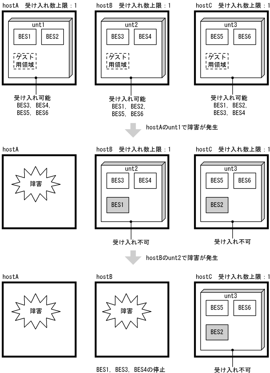
図 26-15 多重障害時に系切り替えができなくなる場合の例
