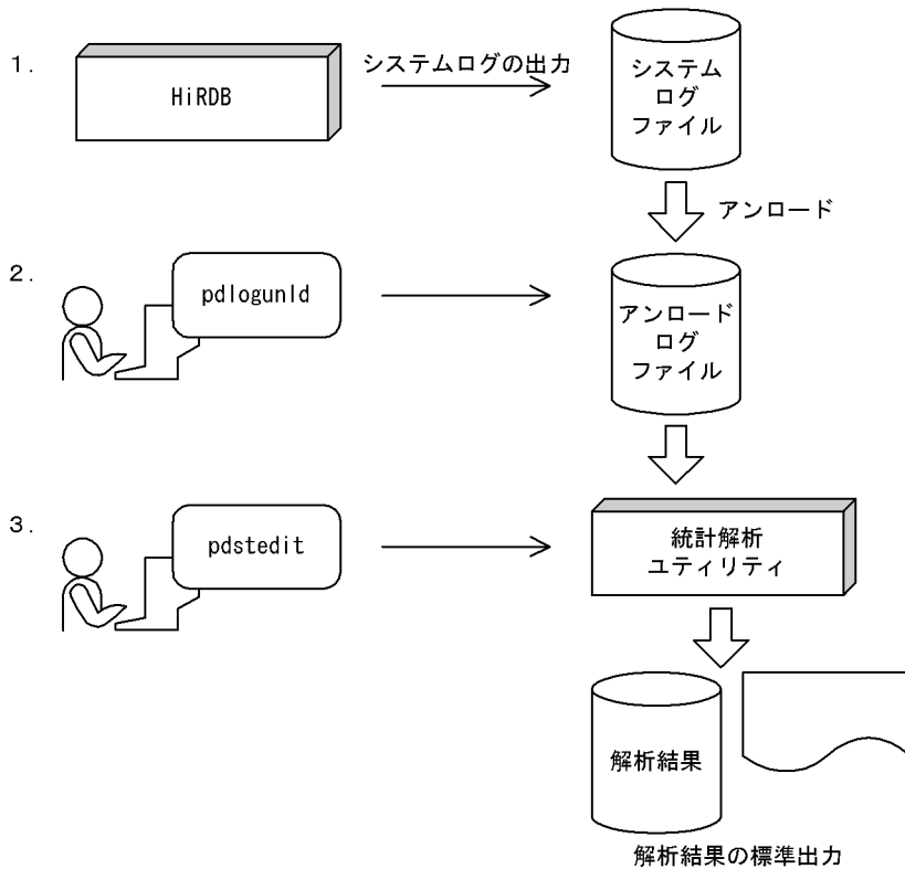
図 22-3 チューニング情報の取得手順（システムログからチューニング情報を取得する場合）
