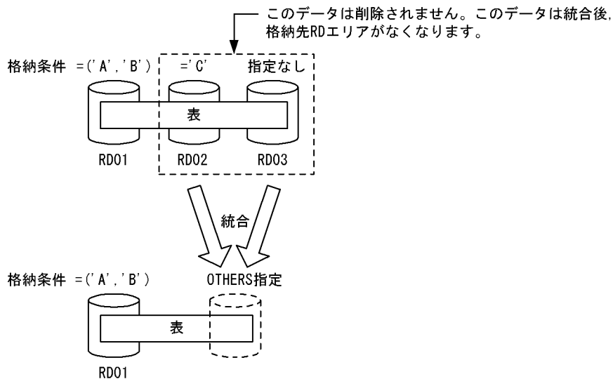
図 13-76 統合後にデータを格納する RD エリアがなくなるケース (その 1)
