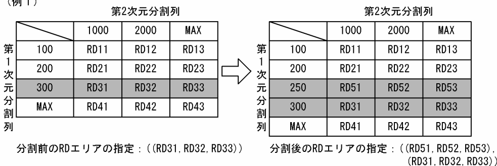
図 13-79 RD エリアの分割後の RD エリアの指定 (マトリクス分割の場合)
