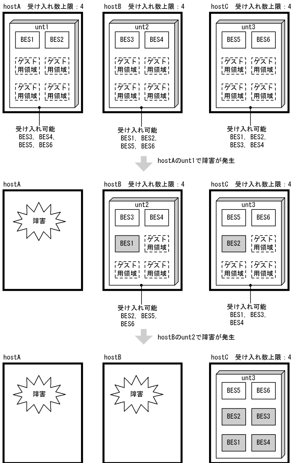
図 26-11 多重障害時の系切り替えの例
