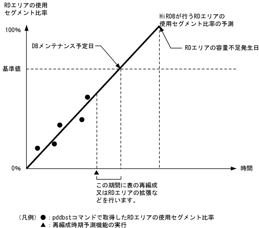
図 13-10 HiRDB が行う予測データの解析方法の概要
