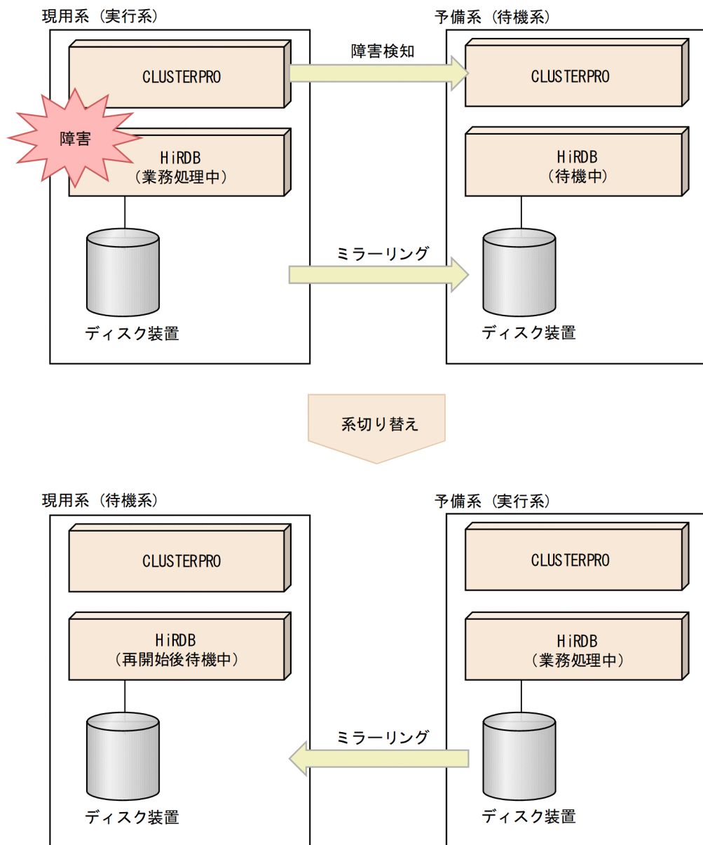
図 26-4 CLUSTERPRO によるミラーディスク使用時の系切り替え機能（スタンバイ型系切り替え機能）の概要
