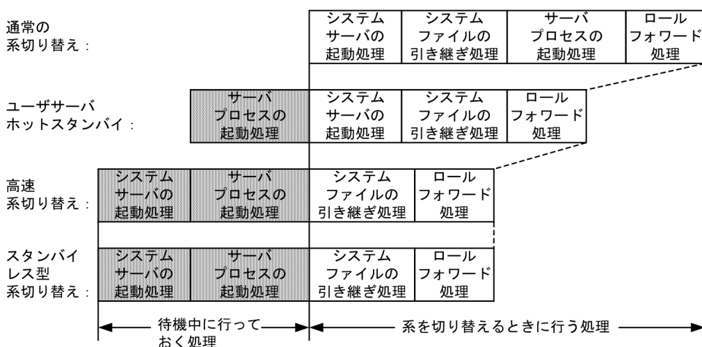
図 26-1 系の切り替え時間の比較
