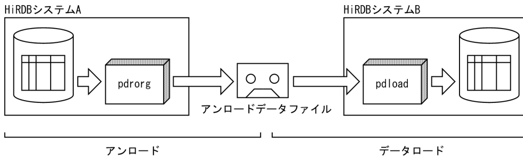
図 12-5 データベース再編成ユーティリティ及びデータベース作成ユーティリティを使用した表データの移行
