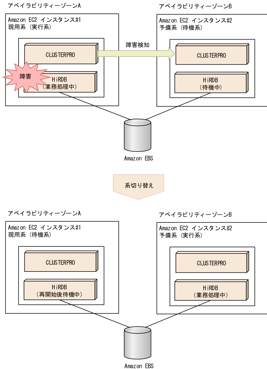
図 26-49 Amazon Web Services 環境上の共有ディスクを使用したクラスタ構成概要図
