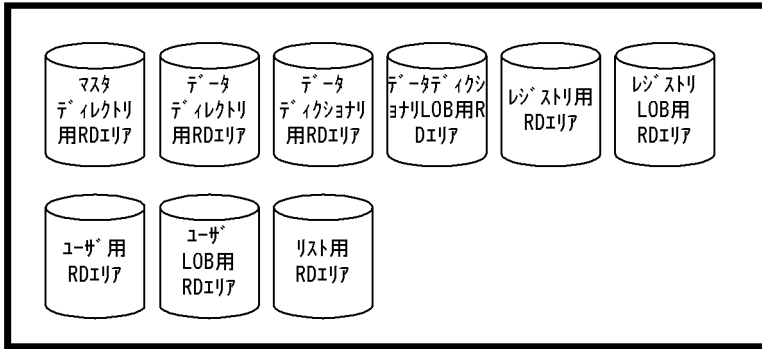
図 11-1 データベース構成変更ユーティリティによる RD エリアの移行
