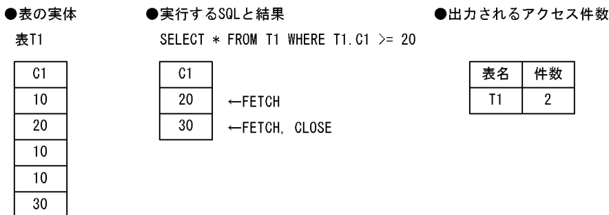
図 24-11 アクセス件数の出力例 (その 2)
