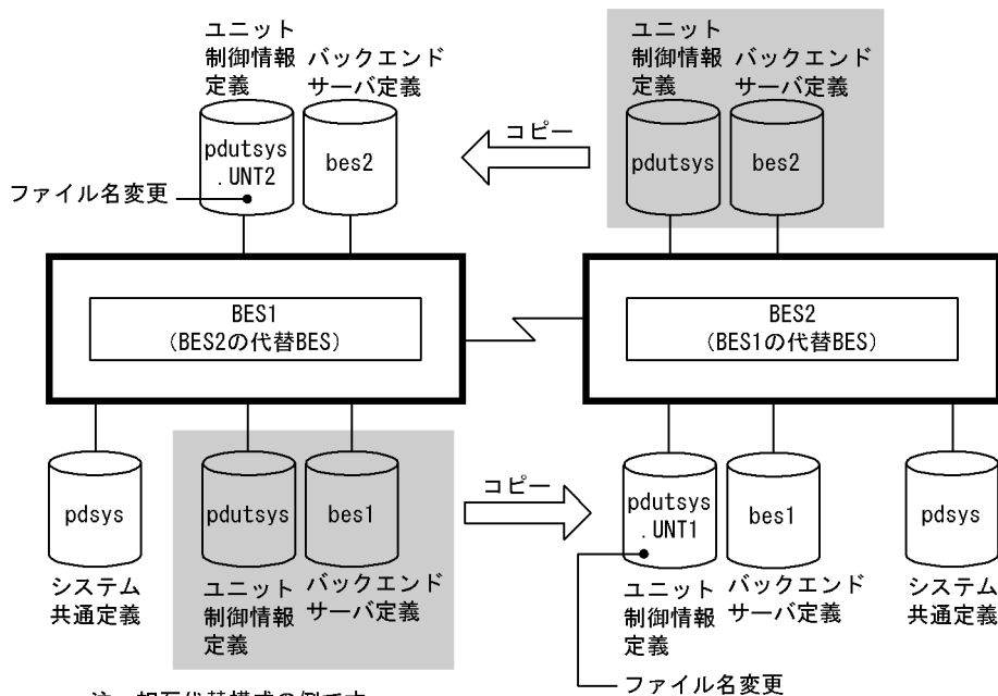
図 26-35 スタンバイレス型系切り替え機能使用時の HiRDB システム定義ファイルの構成例（相互代替構成の場合）
