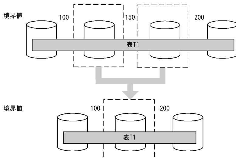
図 13-17 統合機能の概要（境界値指定の場合）
