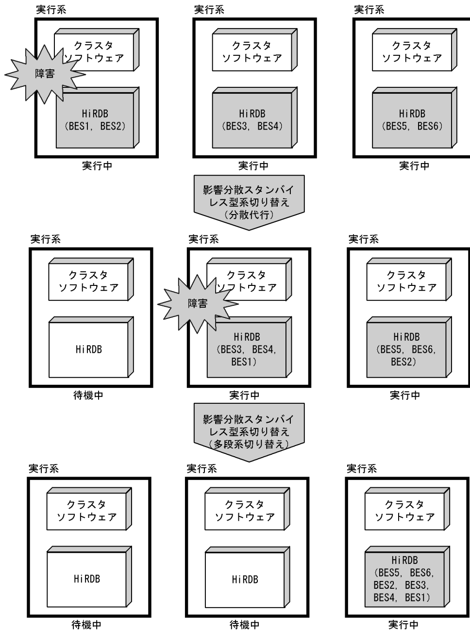
図 26-8 影響分散スタンバイレス型系切り替え機能の概要（分散代行，多段系切り替え）
