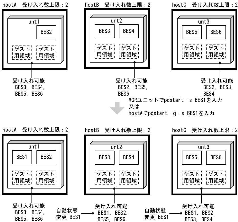
図 26-58 影響分散スタンバイレス型系切り替え機能での実行系サーバの開始の例
