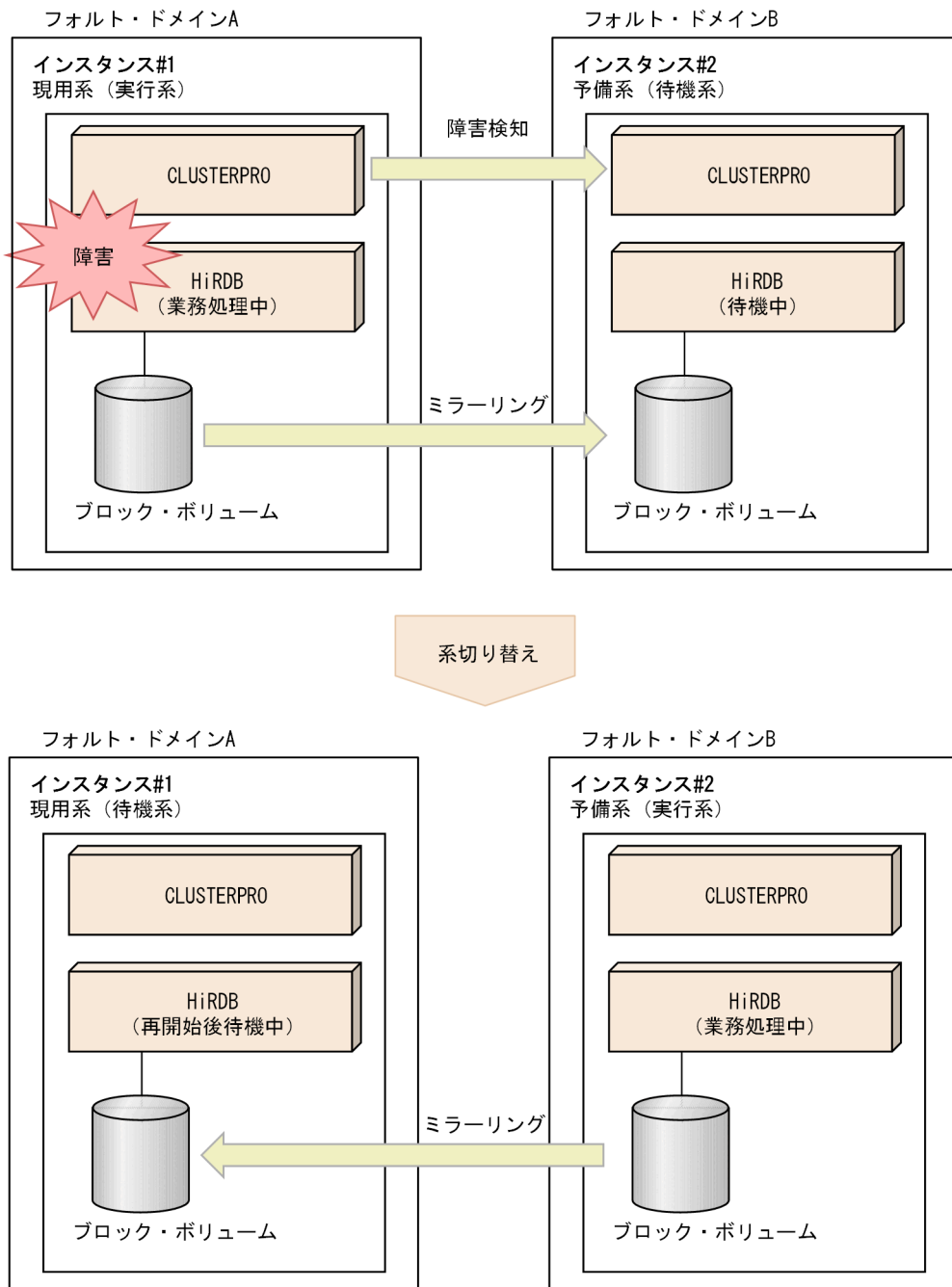
図 26-54 Oracle Cloud Infrastructure 環境上のミラーディスクを使用したクラスタ構成概要図
