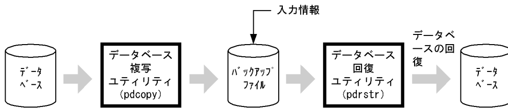
図 21-1 データベース回復の概要 (バックアップ取得時点に回復する場合)
