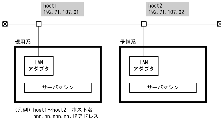
図 26-30 IP アドレスを引き継がない場合のネットワーク構成例
