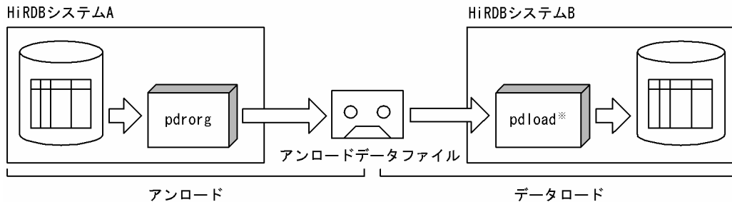
図 12-8 固定長文字データの列の定義長を拡張する表データの移行
