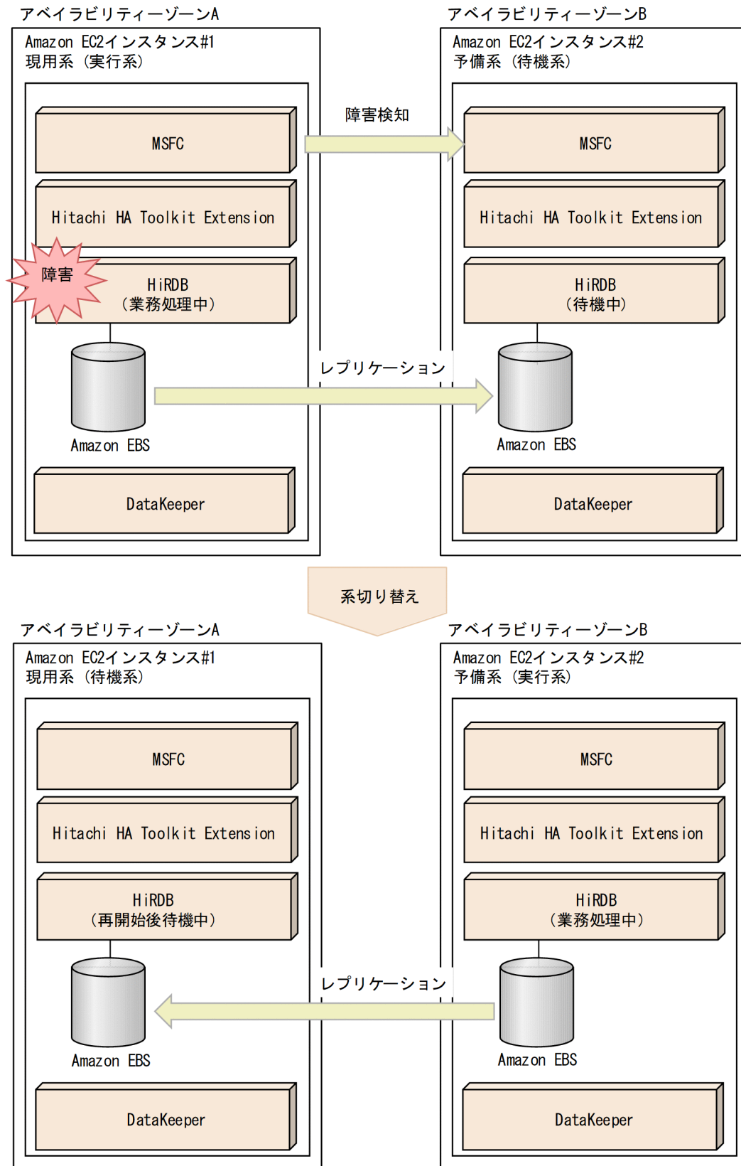
図 26-47 Amazon Web Services 環境上のクラスタ構成概要図
