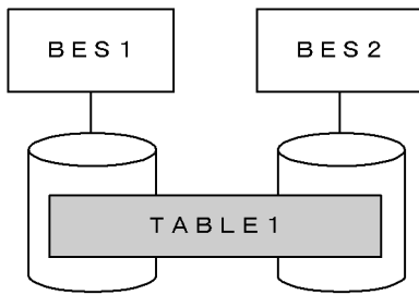
図 20-9 表を複数のバックエンドサーバに横分割している場合の例
