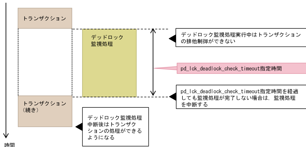
図 9-8 トランザクションとデッドロック監視処理の関係
