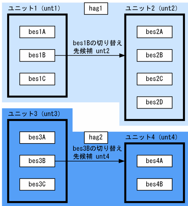
図 26-37 HA グループの構成例 (その 2)
