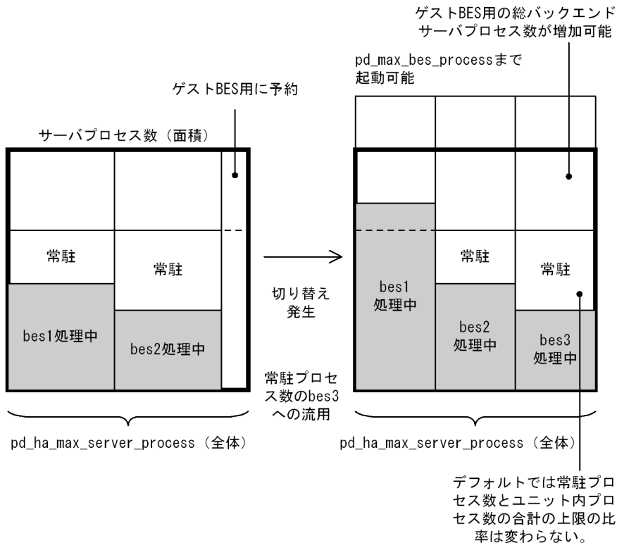
図 26-40 影響分散スタンバイレス型系切り替えでの系切り替え発生後のサーバプロセス割り当て (その 1)
