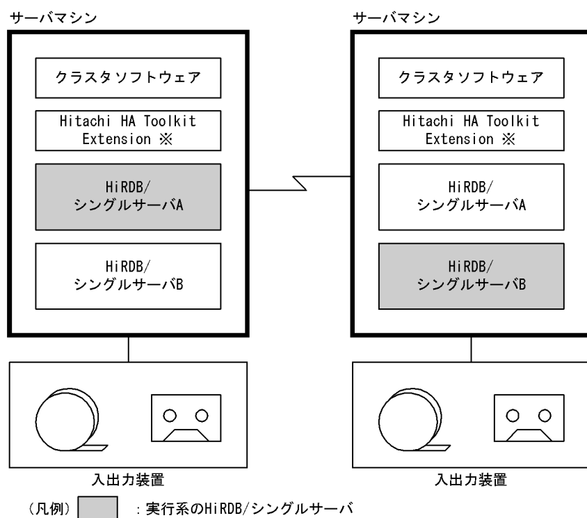
図 26-17 HiRDB/シングルサーバに対する相互系切り替え構成の例
