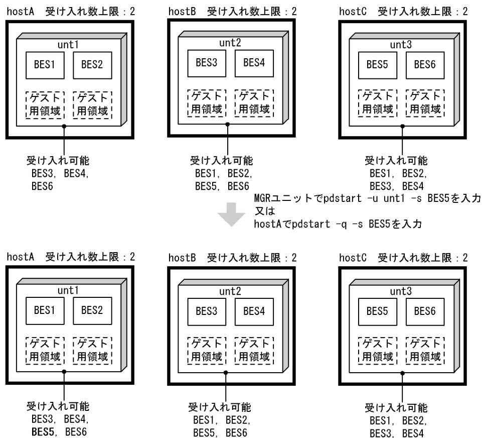
図 26-60 影響分散スタンバイレス型系切り替え機能でのゲストサーバの状態変更の例
