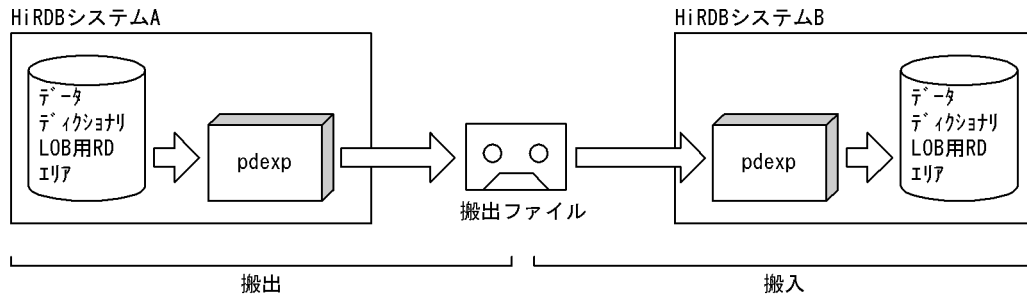
図 12-10 デイクショナリ搬出入ユーティリティを使用したストアプロシジャの移行
