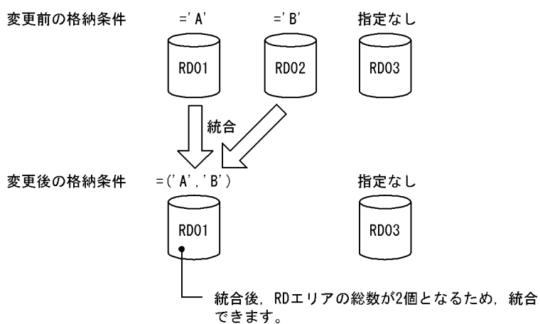
図 13-59 統合できるケース (その 2)
