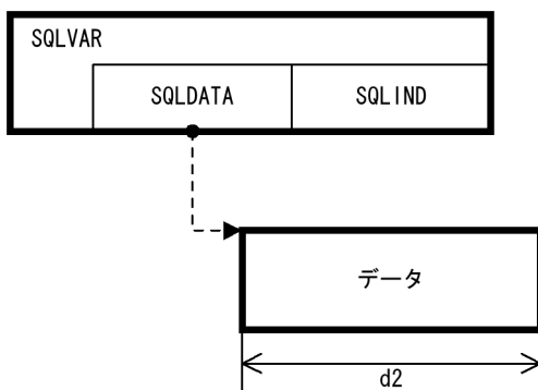
図 24-28 単純構造の入力値（標識変数なし）の構造
