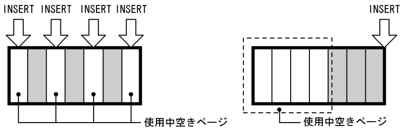
図 15-11 インデクスページに使用中空きページが作成される処理
