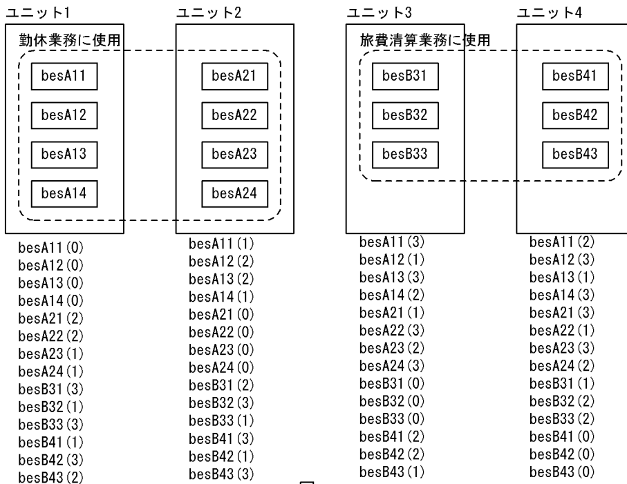
図 11-10 負荷均等化を行うときのバックエンドサーバの構成例 2 (2 業務, 4 ユニット, 14 バックエンドサーバの場合)
