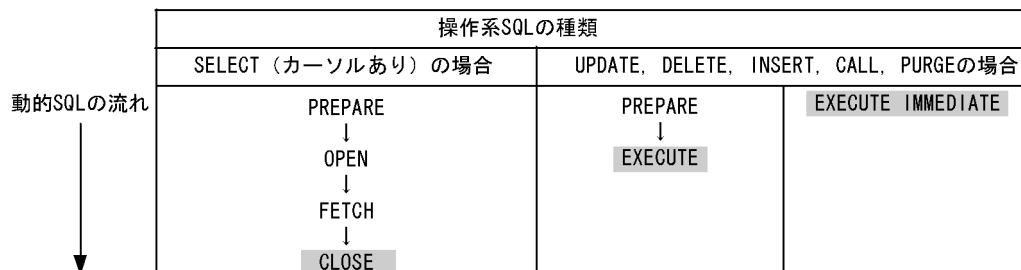
図 24-3 操作系 SQL の種類による動的 SQL の流れ
