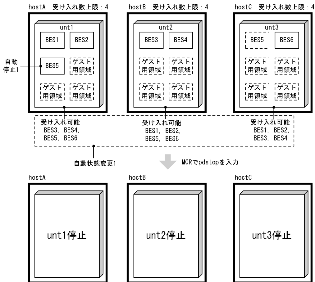
図 26-61 システム停止の例
