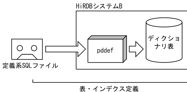
図 12-9 データベース定義ユーティリティを使用した表・インデクス定義
