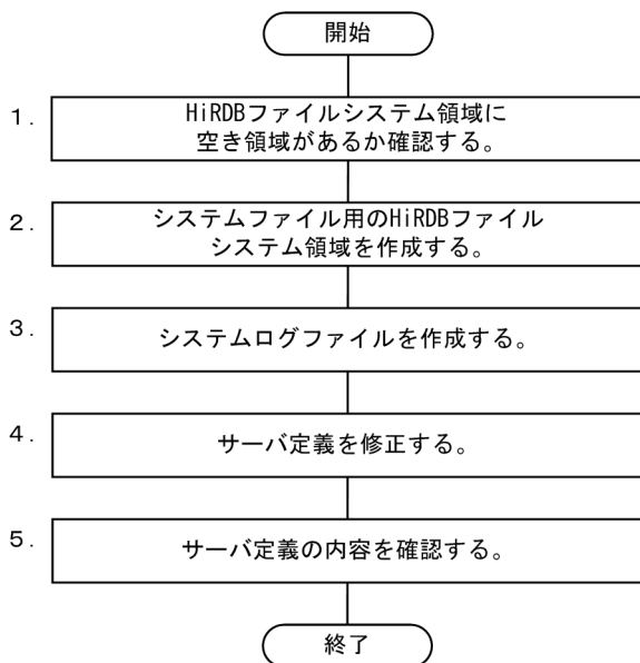
図 20-7 システムログファイルの追加手順（フロー）
