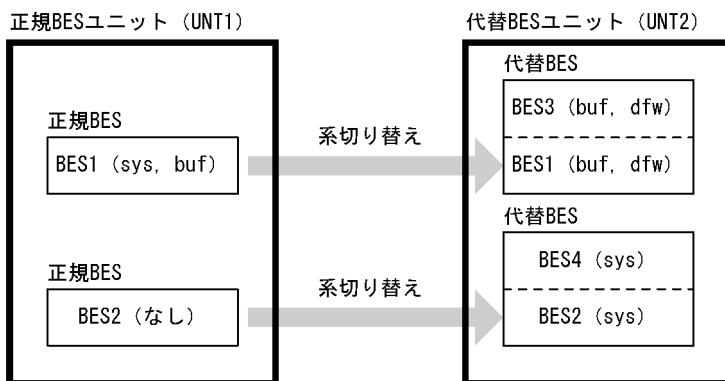
図 26-71 代替中の統計情報の取得処理
