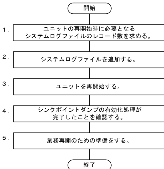
図 20-5 システムログファイルを追加してからユニットを再開始する手順（フロー）
