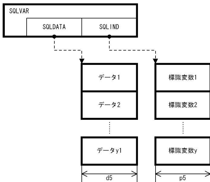
図 24-31 固定長のデータ型で配列を使った入力値 (標識変数あり) の構造
