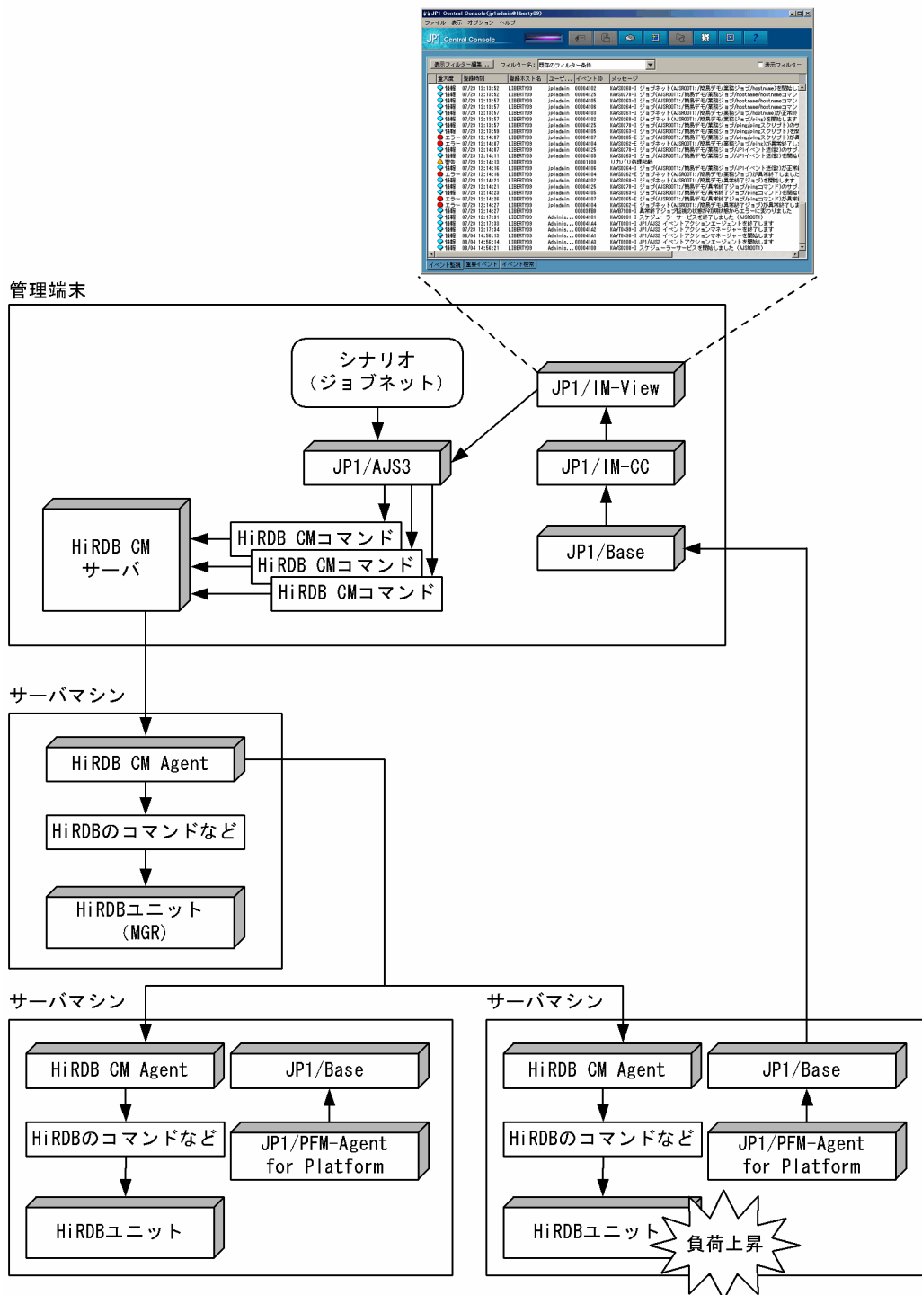
図 11-7 JP1/PFM によるバックエンドサーバの負荷監視とユーザ操作によるシナリオ実行
