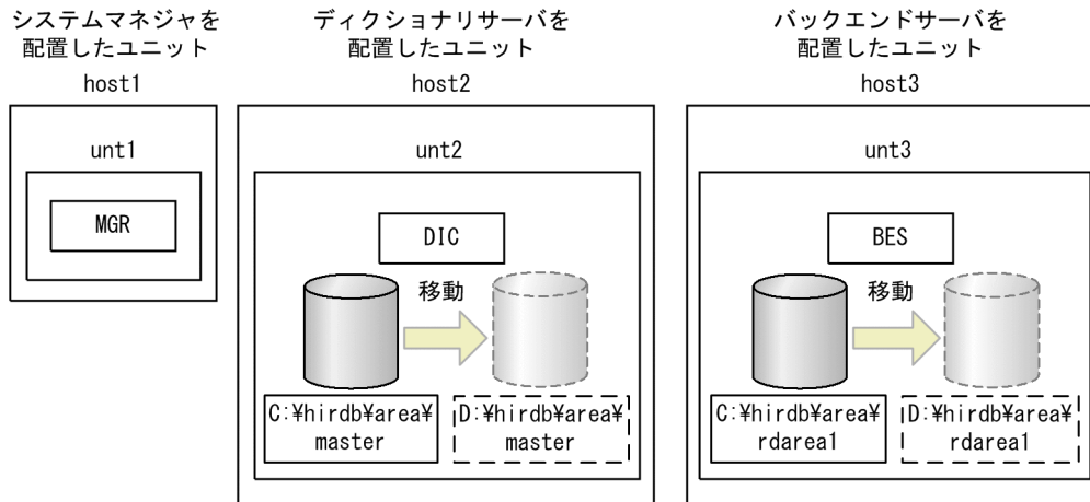
図 15-8 ユニットの變更のない移動
