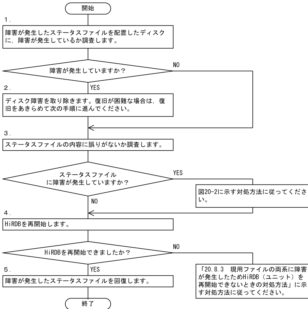
図 20-1 障害が発生したステータスファイルがある状態で HiRDB (ユニット) を開始するときの対処方法
