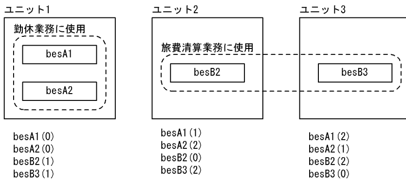
図 11-9 負荷均等化を行うときのバックエンドサーバの構成例 1 (2 業務, 3 ユニット, 4 バックエンドサーバの場合)
