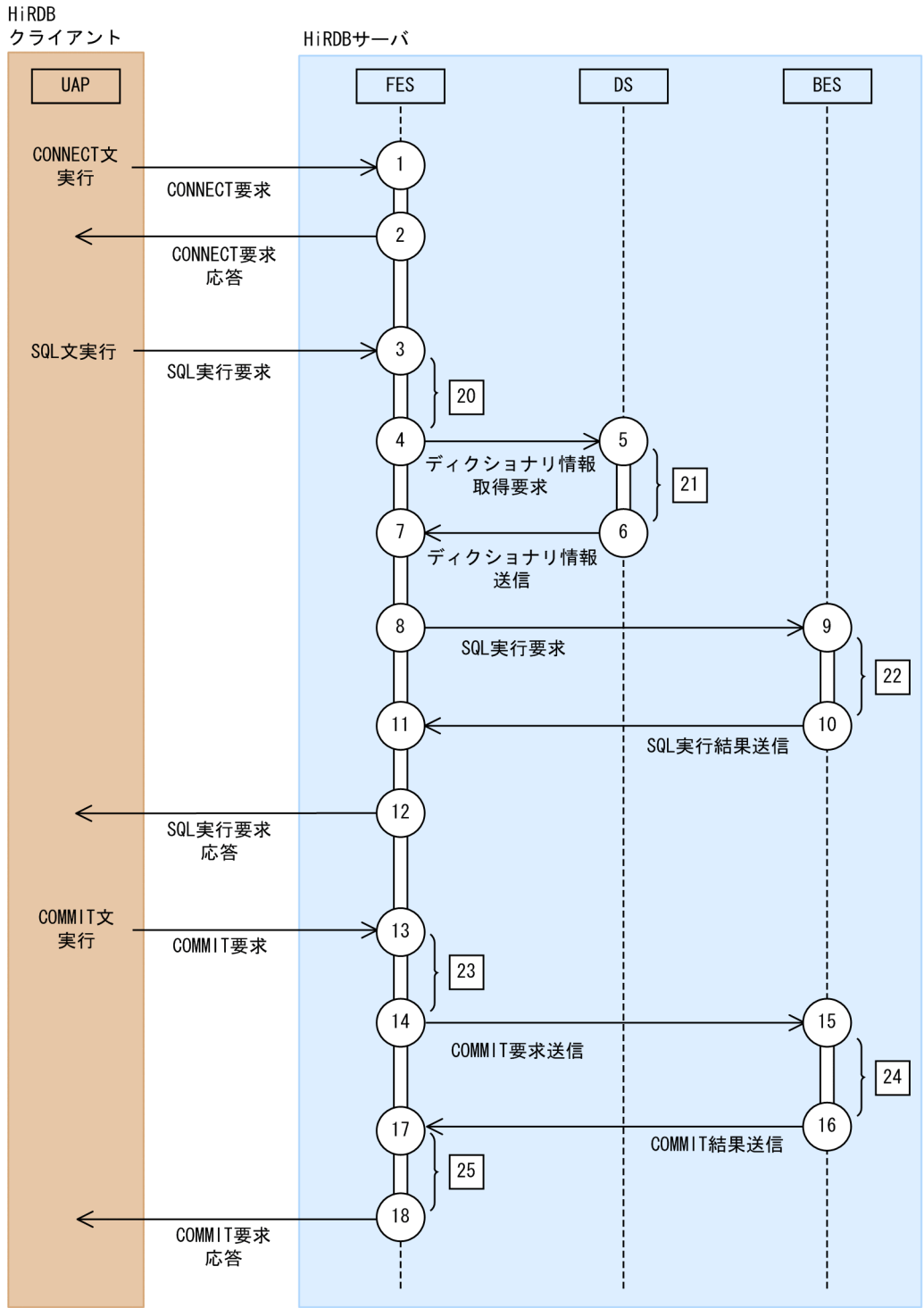
図 28-4 PRF トレースの取得ポイントの概念図 (HiRDB/パラレルサーバの場合)
