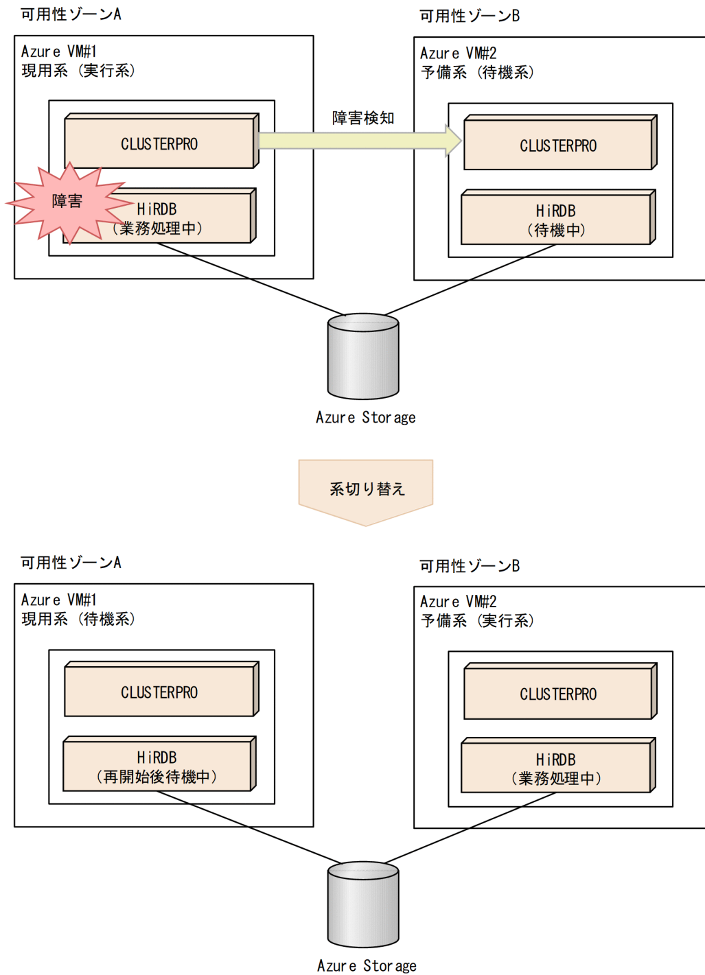
図 26-50 Microsoft Azure 環境上の共有ディスクを使用したクラスタ構成概要図
