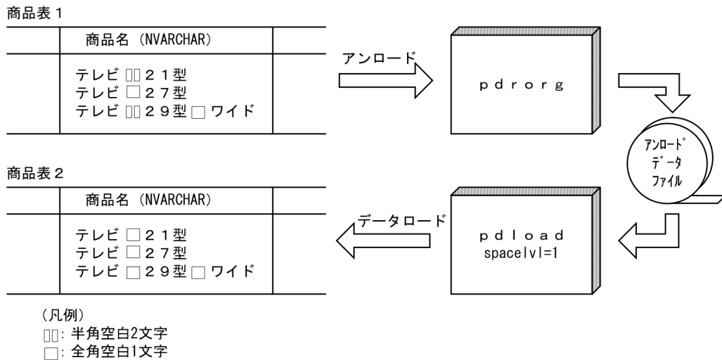
図 13-97 別システムに表データを移行する場合の空白文字の統一方法
