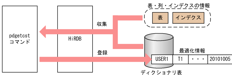
図 19-1 データベースからの最適化情報の収集
