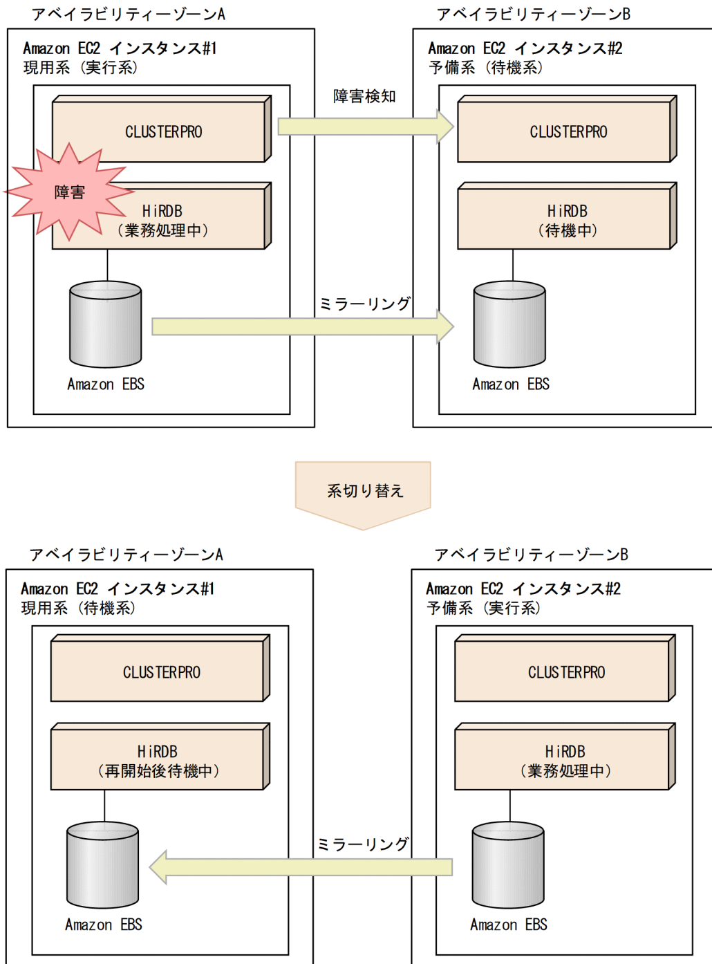
図 26-52 Amazon Web Services 環境上のミラーディスクを使用したクラスタ構成概要図
