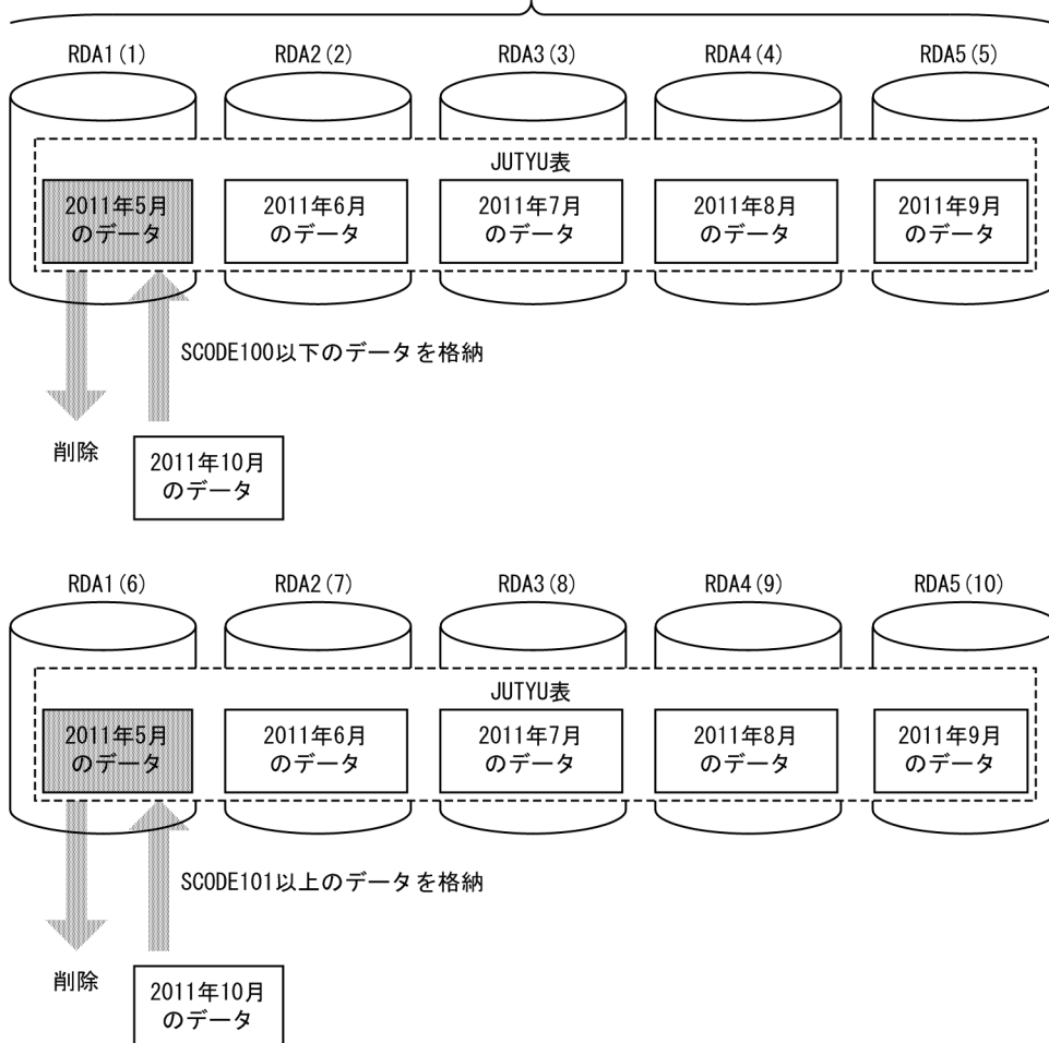
図 13-89 RD エリアを年月単位に循環させて割り当てる場合 (マトリクス分割の場合)
