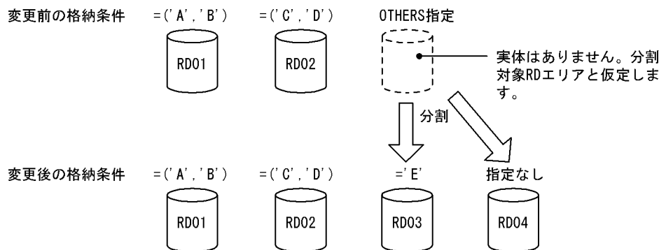
図 13-37 OTHERS 指定の RD エリアを分割する例
