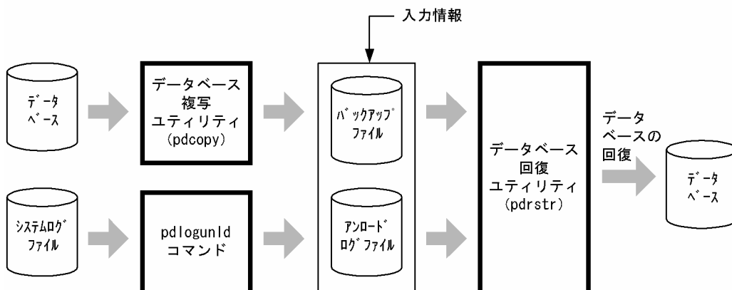
図 21-3 データベース回復の概要（障害発生直前の最新の同期点に回復する場合）
