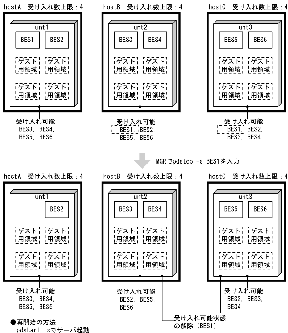
図 26-65 ホスト BES の停止の例
