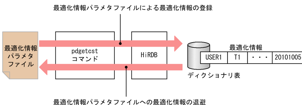
図 19-3 最適化情報パラメタファイルの概要
