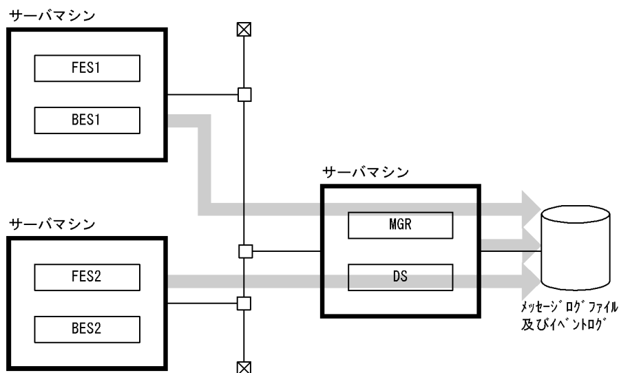
図 8-2 通常のメッセージログの出力方式（1の方式の場合）
