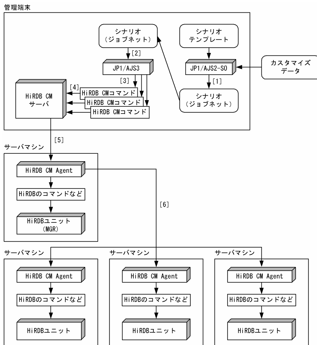
図 11-5 バックエンドサーバの負荷均等化のシナリオ運用形態
