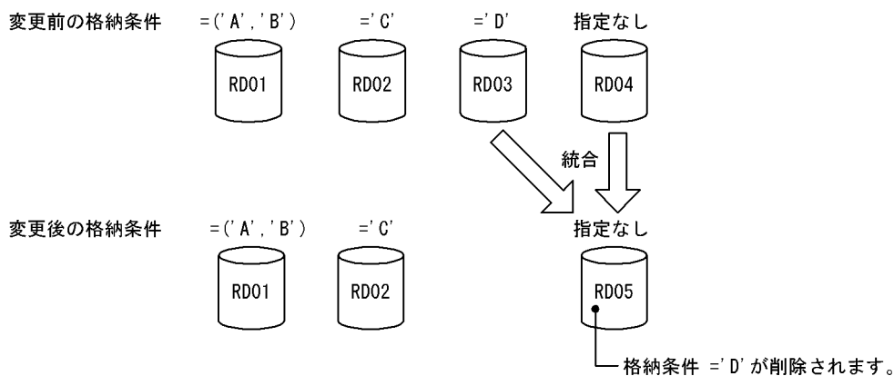
図 13-68 統合できるケース（その 8）
