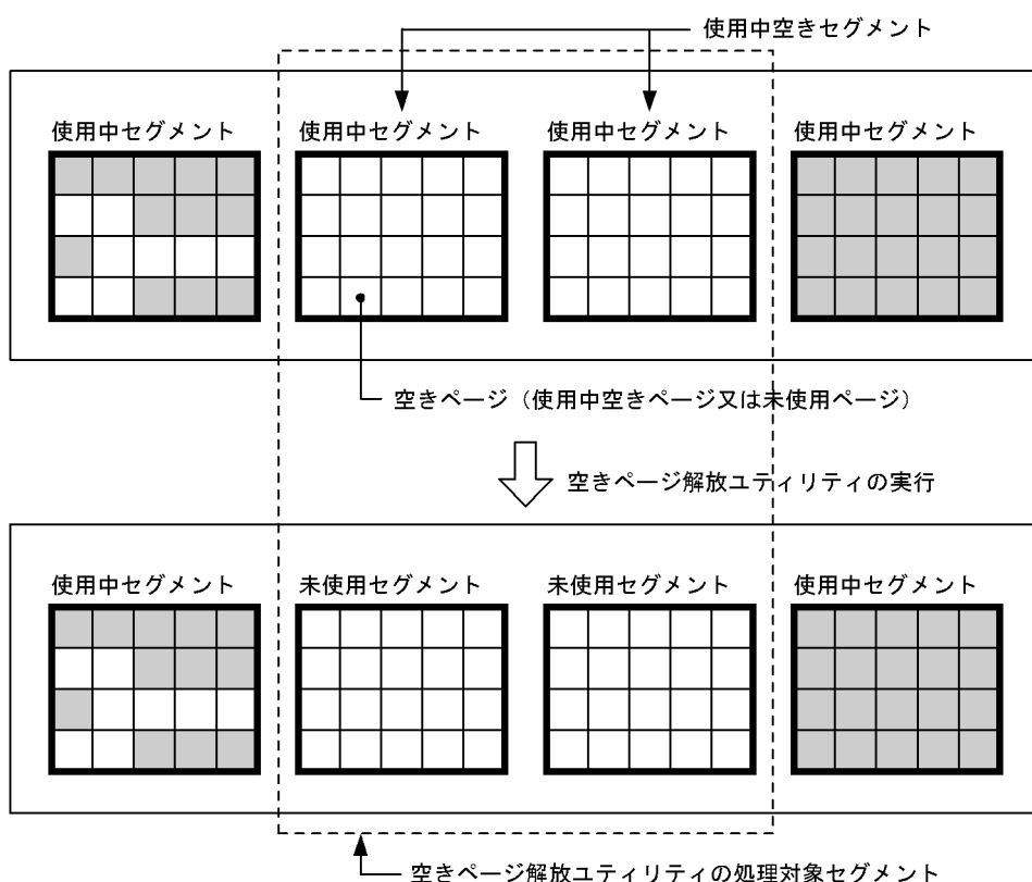
図 15-12 使用中空きセグメントの解放
