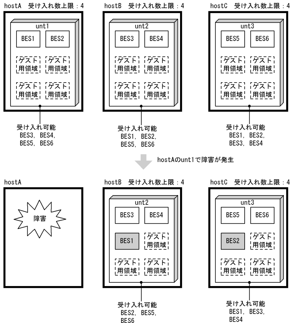
図 26-9 通常時の系切り替えの例
