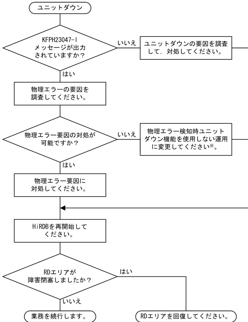
図 15-13 物理エラーが発生した場合の対処方法
