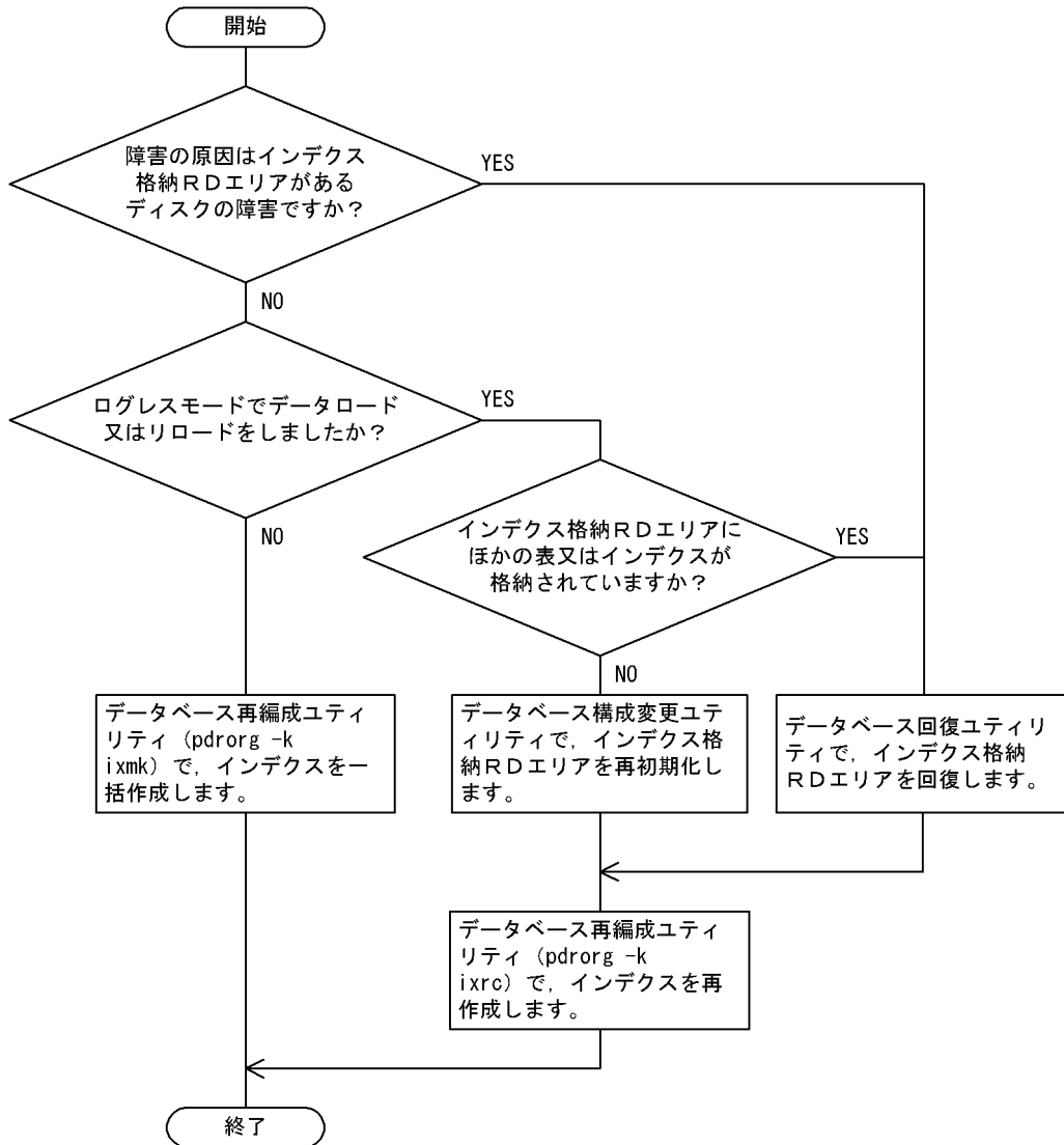
図 14-4 インデクスデータの回復方法の流れ
