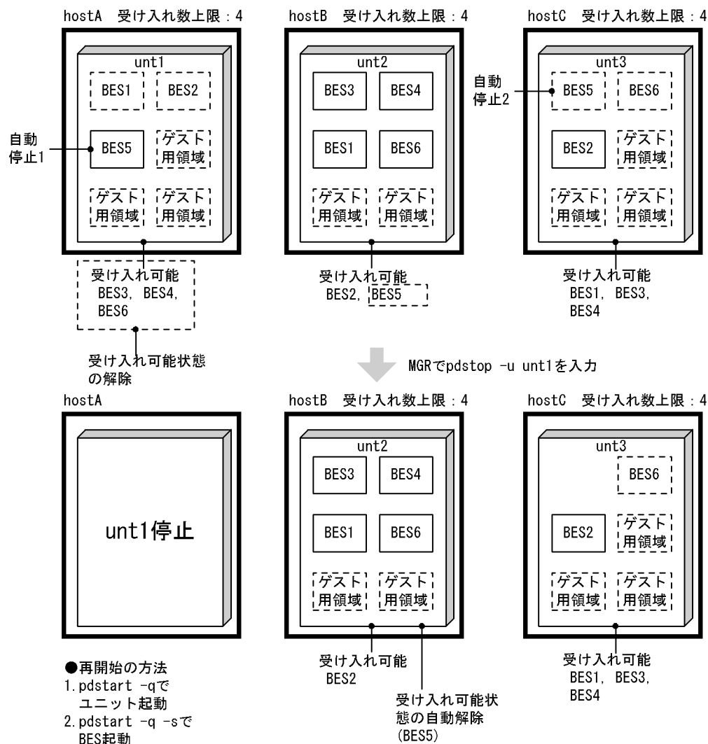
図 26-64 ゲスト BES だけのユニットの停止の例
