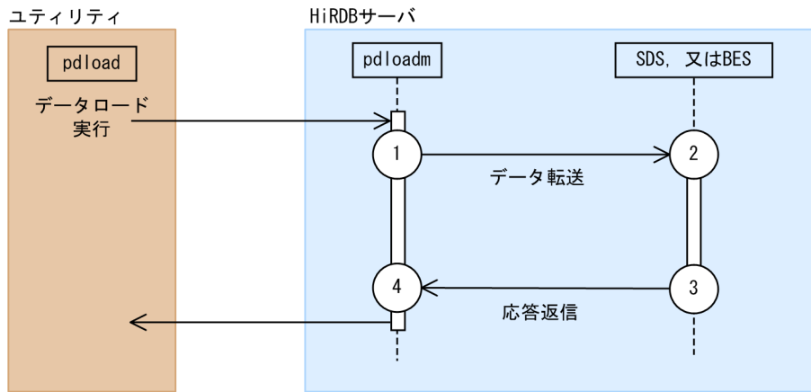
図 28-5 PRF トレースの取得ポイントの概念図 (pdload)
