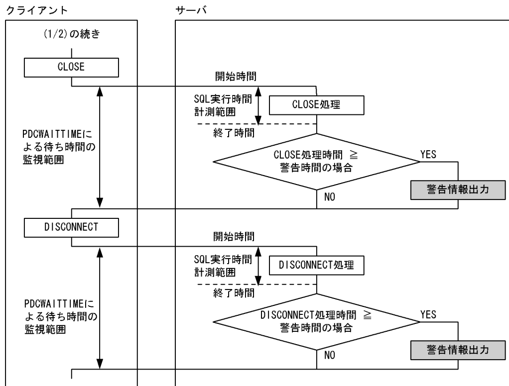
図 8-15 PDCWAITTIME と SQL 実行時間警告出力機能の関係 (2/2)
