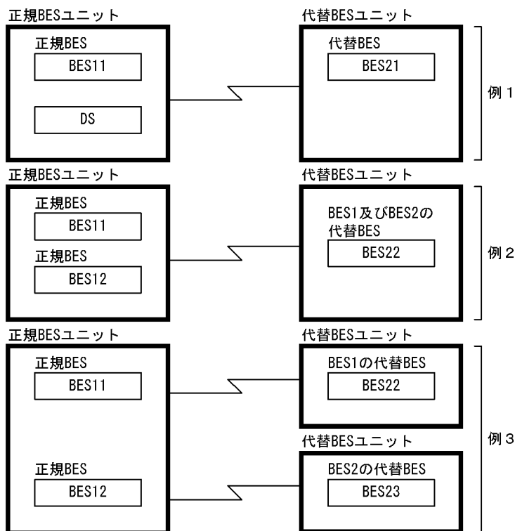
図 26-7 正規 BES ユニット及び代替 BES ユニットの間違っ構成例
