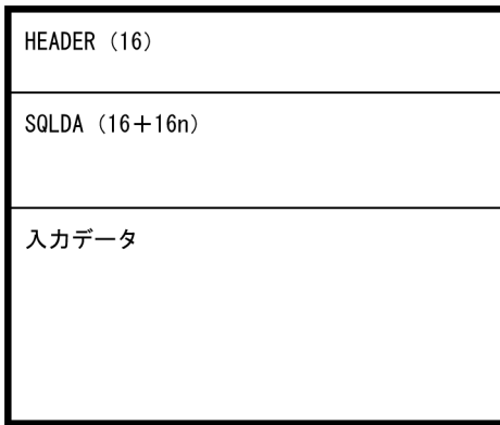
図 24-24 SQL データの構造
