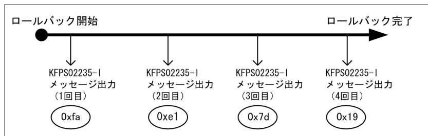
図 8-17 ロールバック処理が進行中の例 (KFPS02235-I メッセージの場合)
