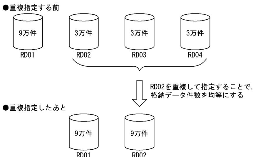
図 12-4 ハッシュ分割で表格納用 RD エリアを重複指定する例
