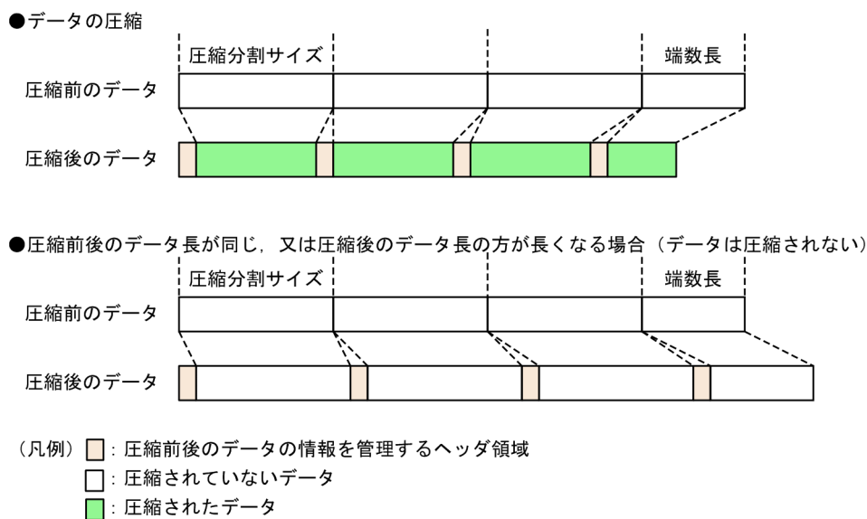
図 12-44 圧縮前後のデータ
