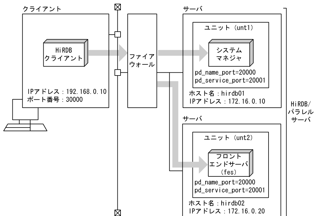
図 21-10 ファイアウォールが HiRDB/パラレルサーバ側に設置されているネットワーク構成例
