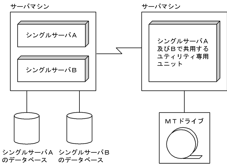
図 9-2 マルチ HiRDB でのユティリティ専用ユニットの設置例（複数の HiRDB でユティリティ専用ユニットを共用するシステム構成）
