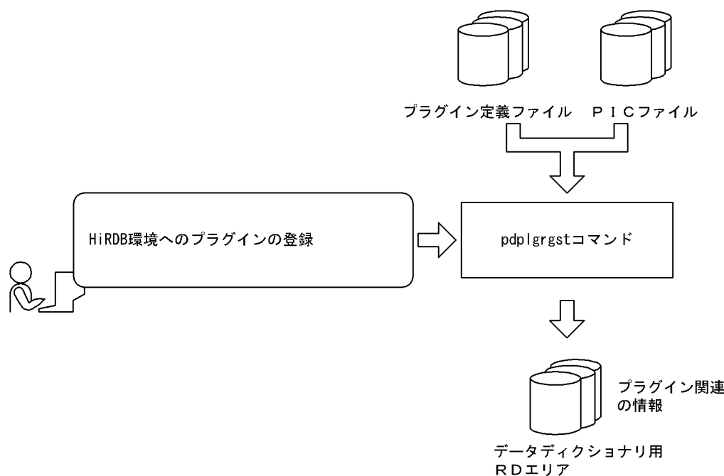
図 4-2 プラグインの登録の流れ
