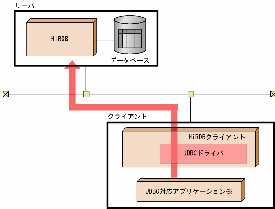
図 1-13 JDBC 対応のアプリケーションからデータベースにアクセスする形態
