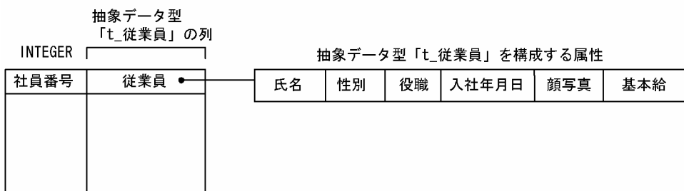
図 3-36 抽象データ型を定義した社員表
