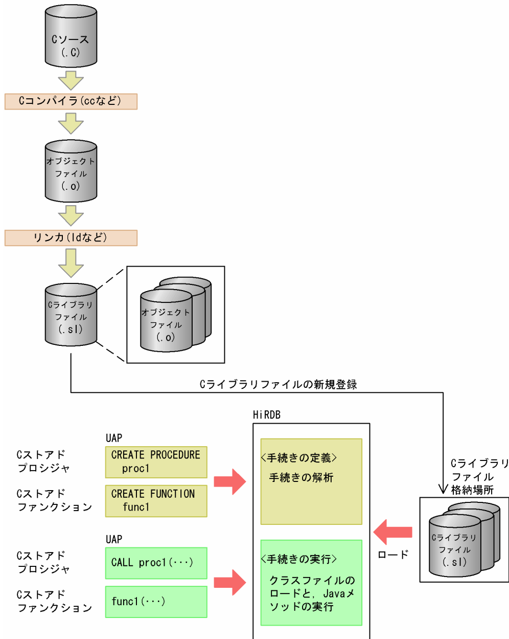
図 5-6 外部 C スタドルーチンの作成から実行までの流れ
