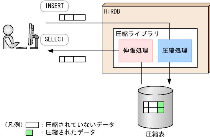
図 3-21 データ圧縮の概要
