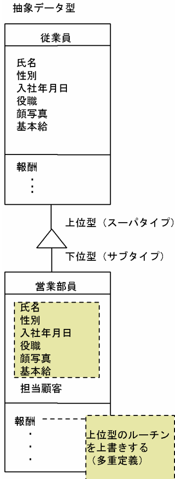
図 3-42 多重定義
