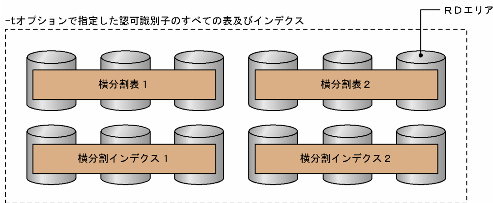
図 7-12 スキーマ単位の再編成
