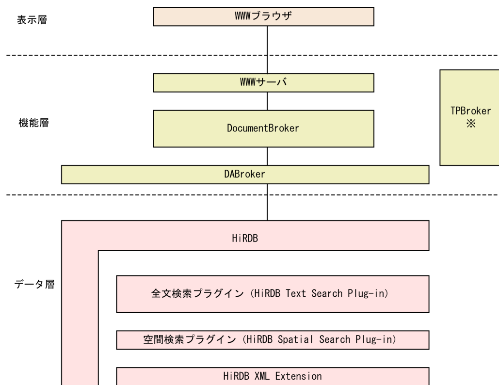
図 2-14 HiRDB の関連製品のシステム構成
