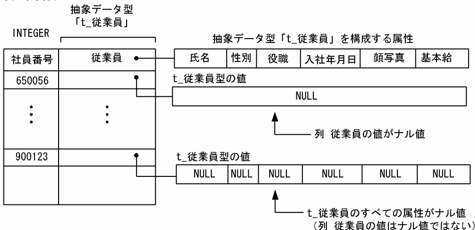
図 3-39 抽象データ型を定義した社員表でのナル値の扱い
