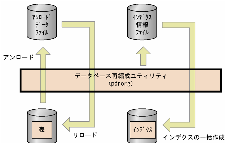
図 7-9 表の再編成
