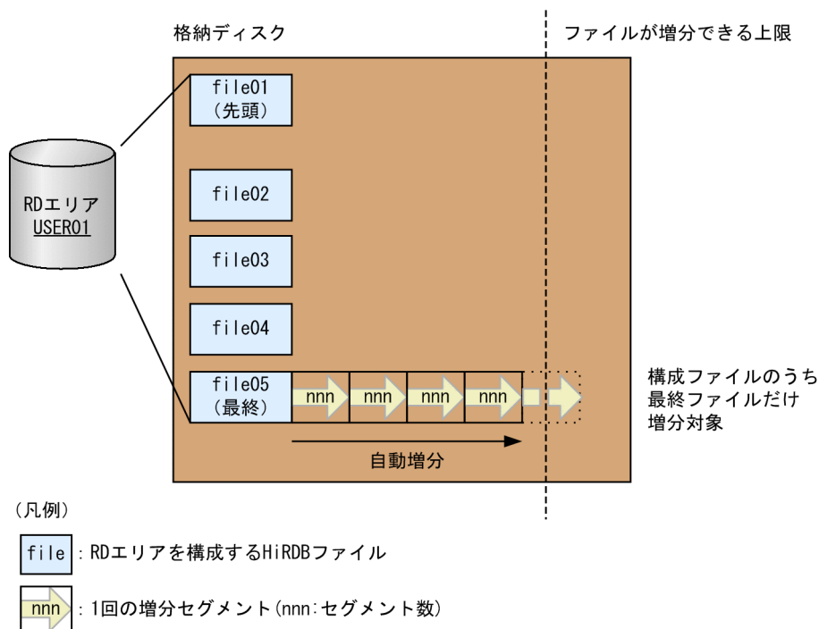
図 7-19 pd_rdarea_extension_file=last の方式
