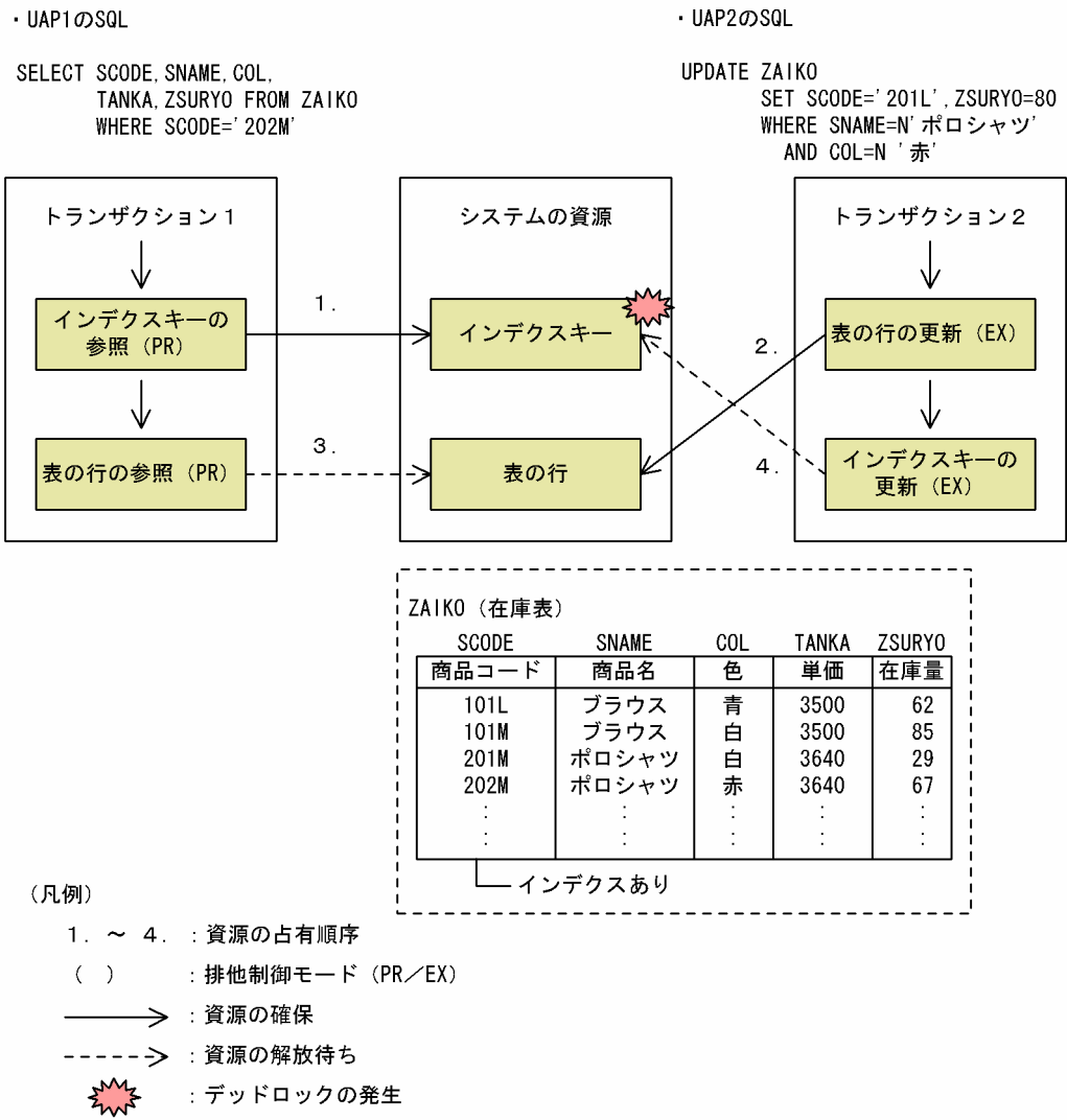
図 3-33 デッドロックの例（インデクスキー値無排他を使用しない場合）
