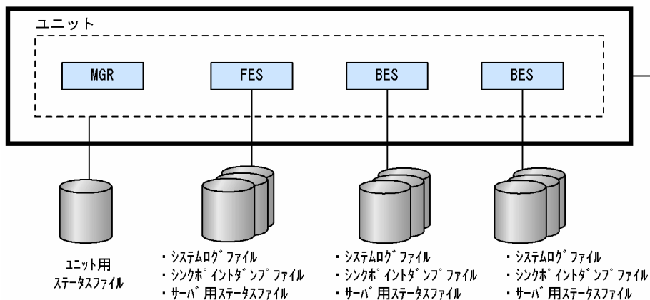
図 6-6 システムファイルの構成 (HiRDB/パラレルサーバの場合)
