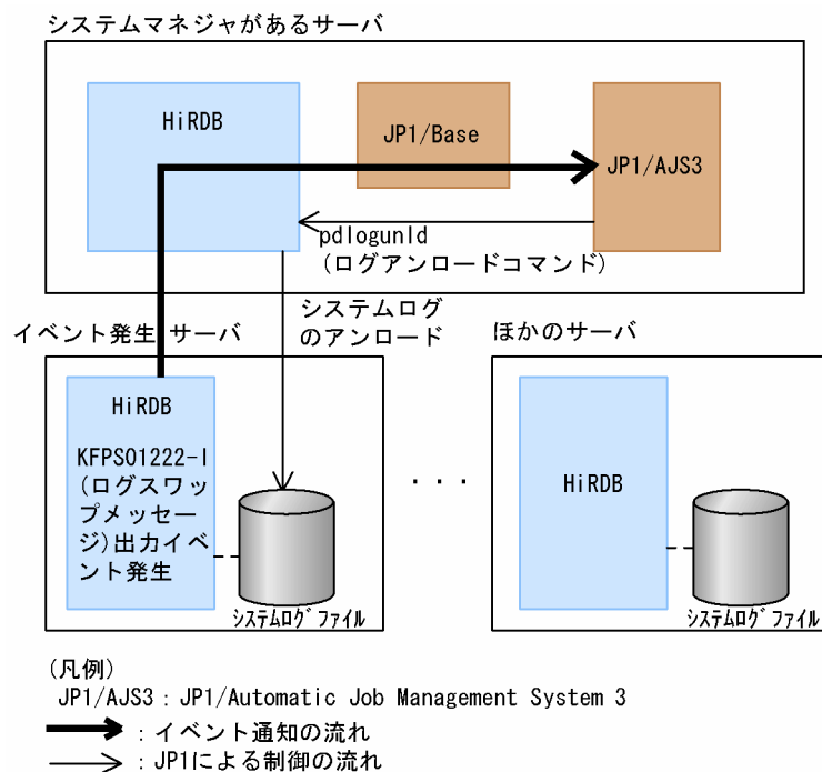
図 2-11 JP1 との連携によるシステムログファイルのアンロード時の自動制御
