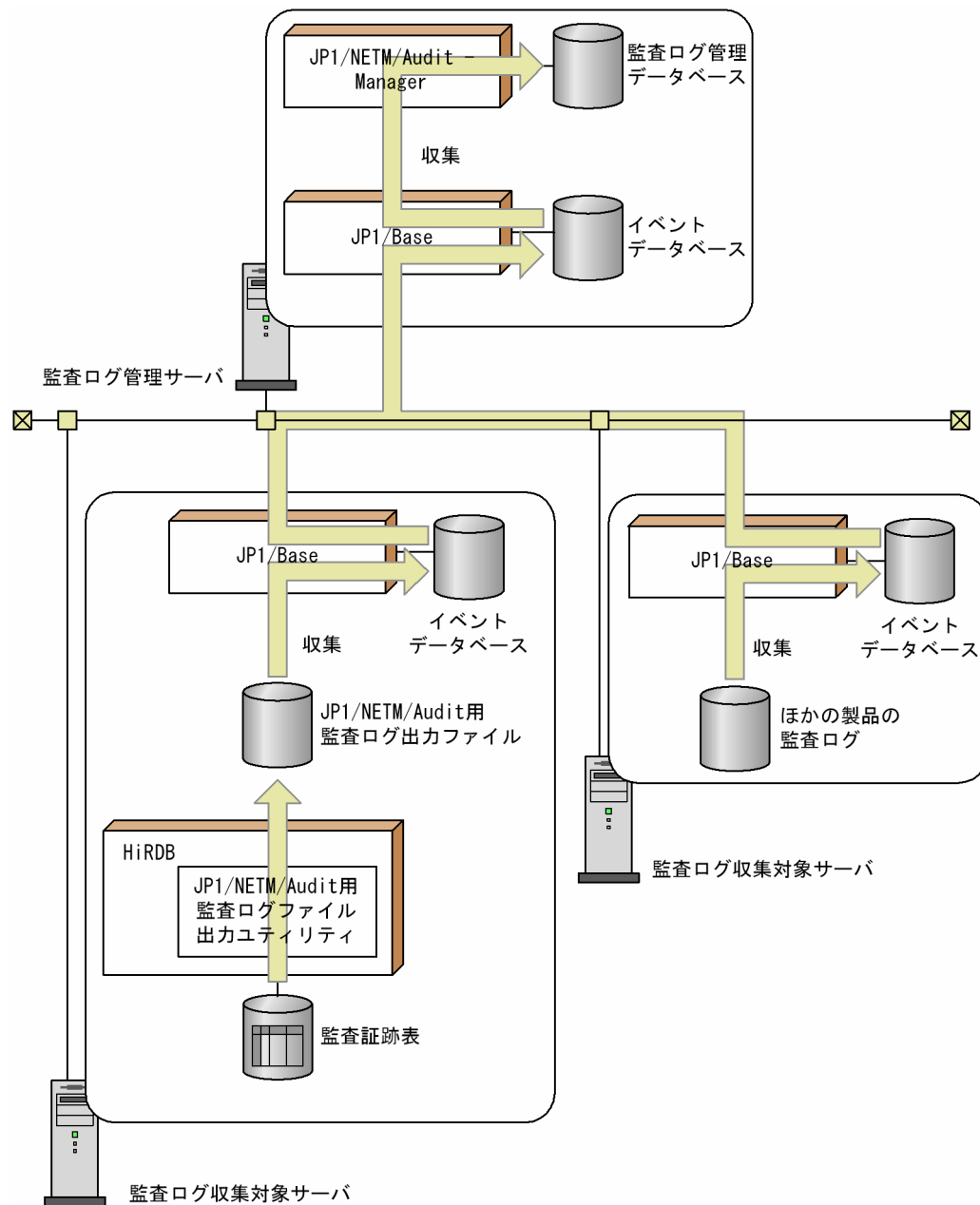
図 2-12 JP1/NETM/Audit との連携の概要
