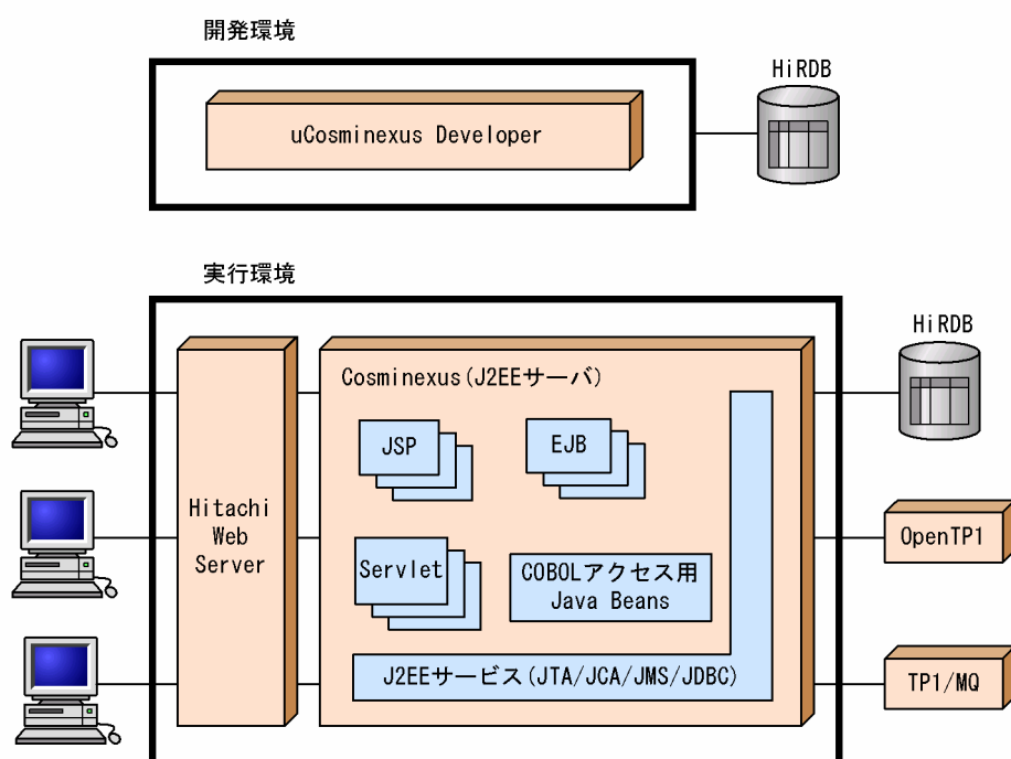
図 2-15 Cosminexus との連携
