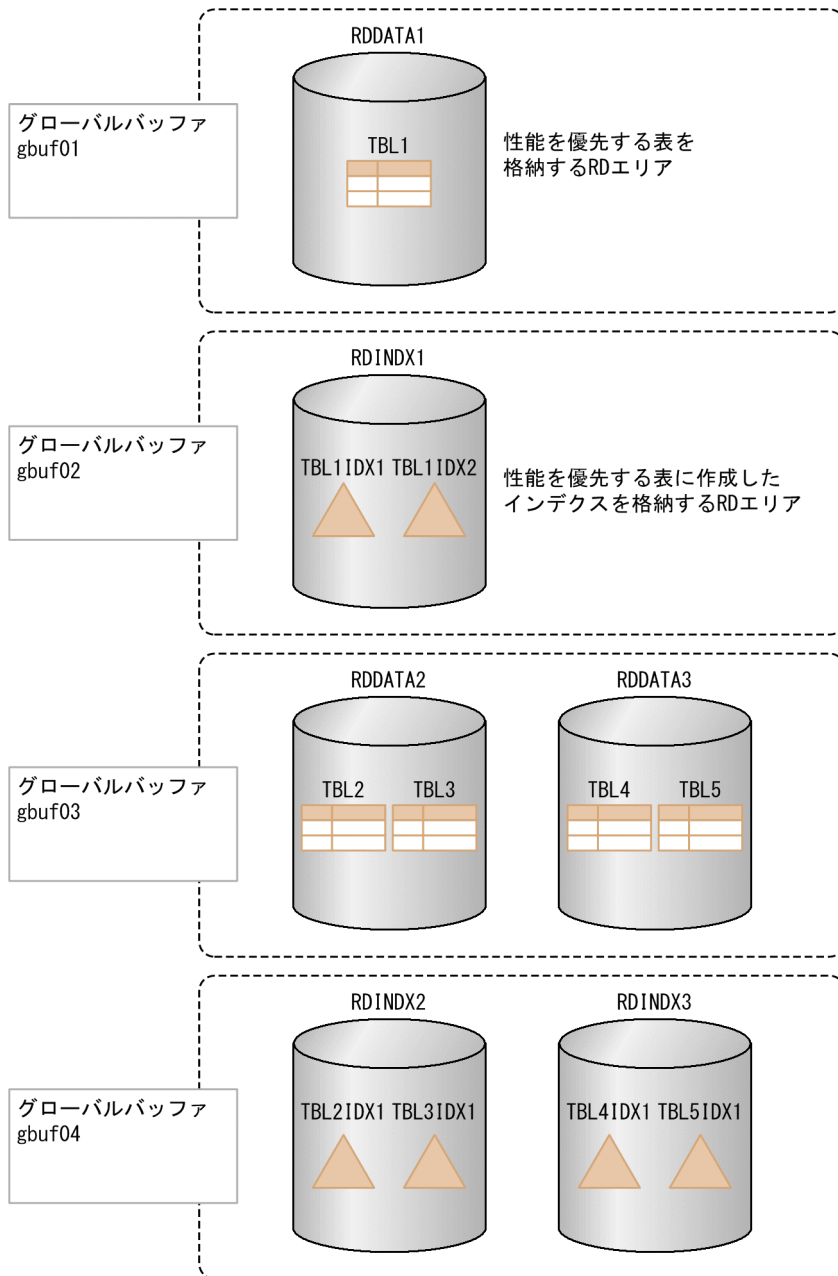
図 11-1 グローバルバッファの構成例
