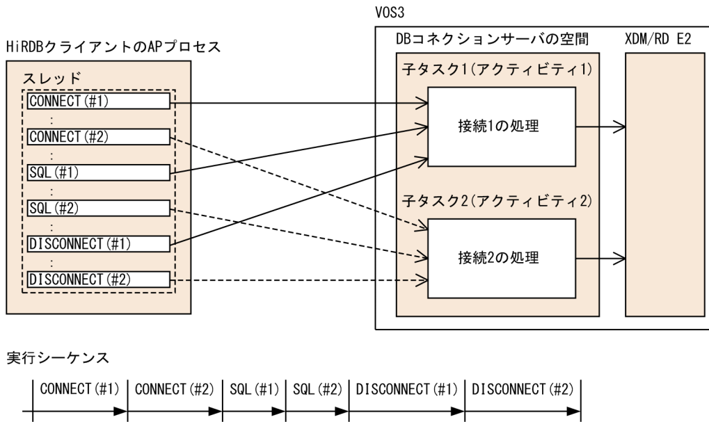
図 3-2 複数接続機能の処理概要 (マルチスレッドを使用しない場合)
