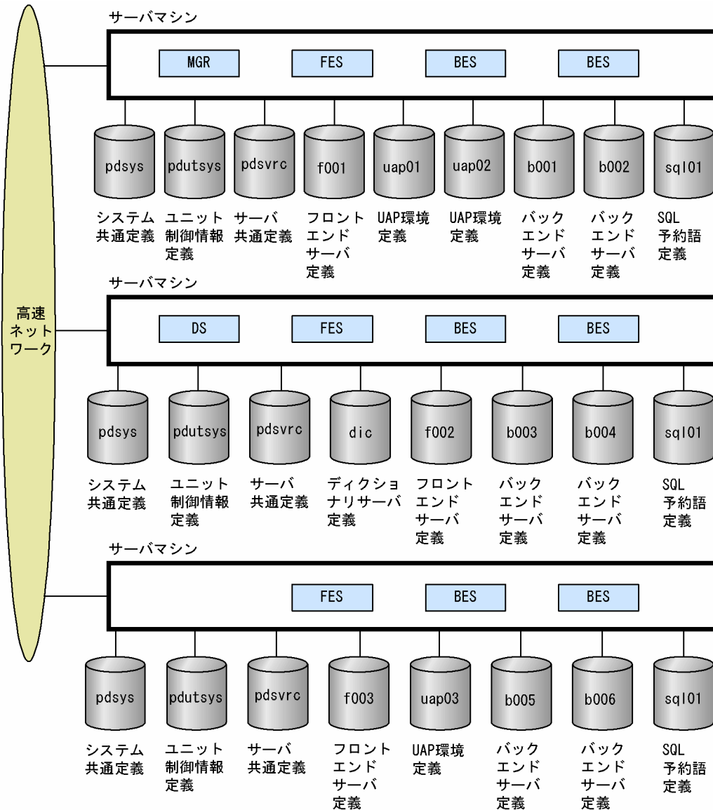
図 6-8 HiRDB システム定義ファイルの構成例 (HiRDB/パラレルサーバの場合)
