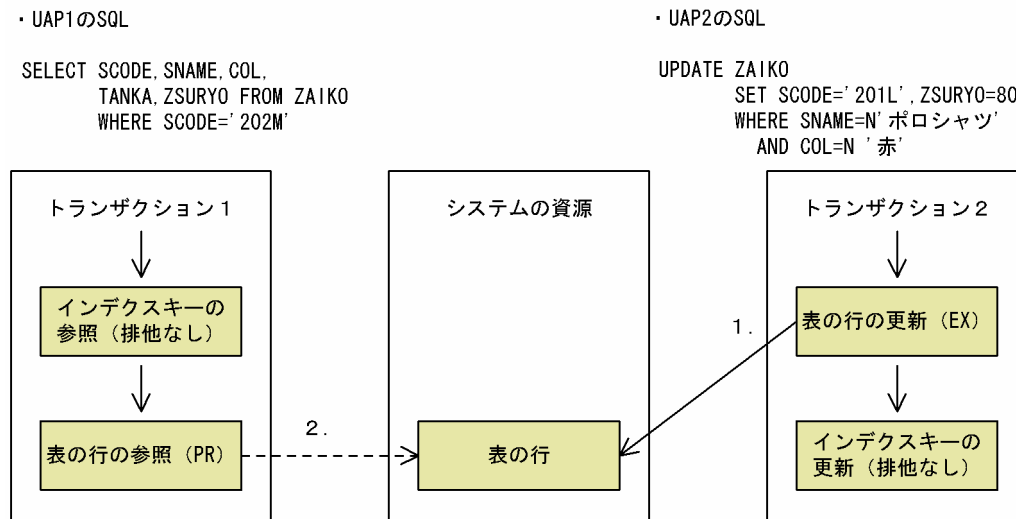
図 3-34 インデクスキー値無排他を使用した場合のデッドロック回避の例
