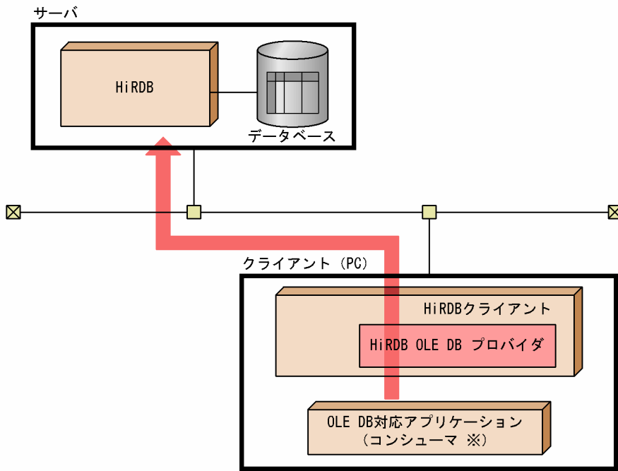
図 1-12 OLE DB 対応のアプリケーションからデータベースにアクセスする形態
