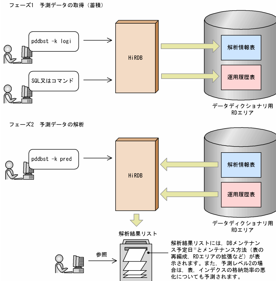
図 7-13 再編成時期予測機能の概要
