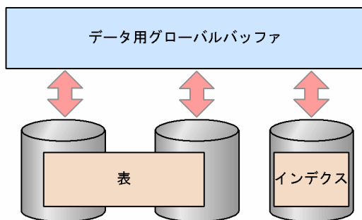
図 6-10 グローバルバッファの概念
