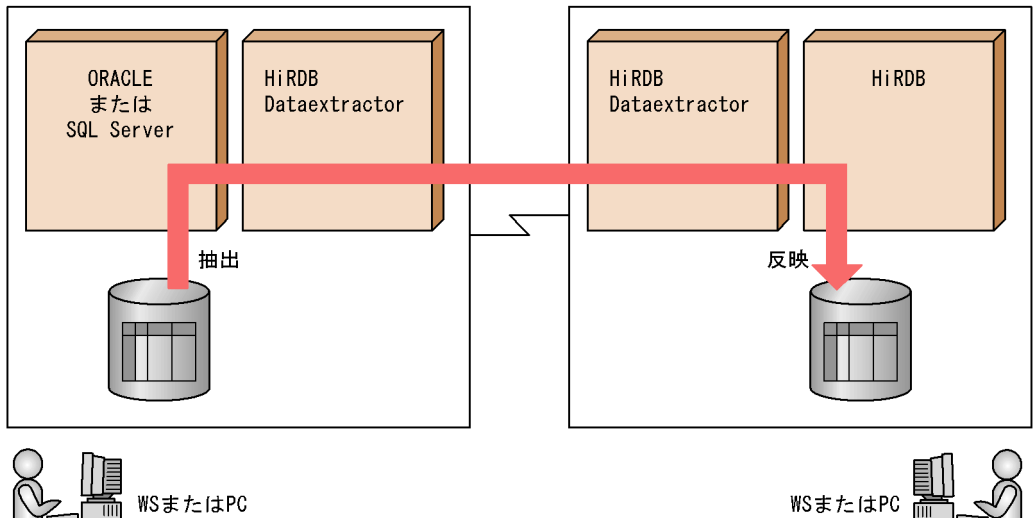
図 1-4 ORACLE , または SQL Server のデータの抽出の概要
