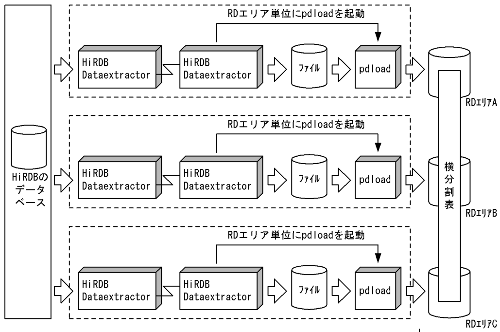
図 3-11 RD エリア単位の格納の概要
