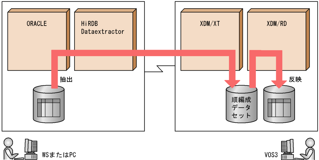
図 1-6 ORACLE からメインフレーム側の DB へのデータの反映の概要
