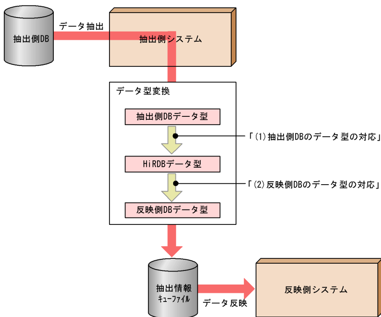
図 4-1 データ型の変換
