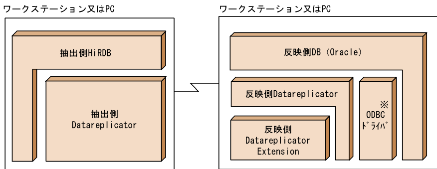
図 1-3 HiRDB から Oracle へデータ連動する場合のソフトウェア構成
