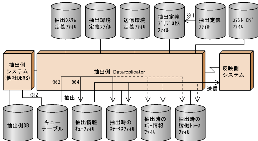
図 3-1 抽出処理の概要
