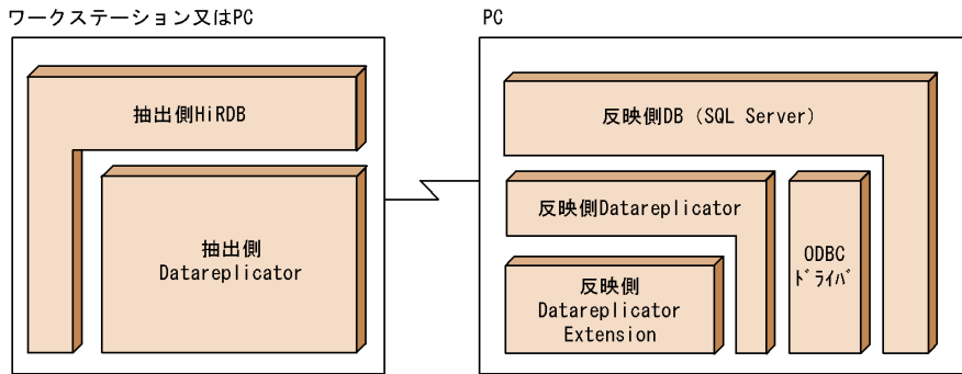
図 1-4 HiRDB から ODBC ドライバを使用して SQL Server へデータ連動する場合のソフトウェア構成
