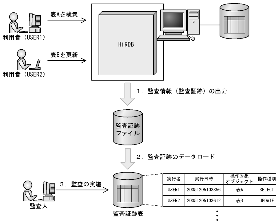
図 1-3 監査情報の出力と参照方法の概要
