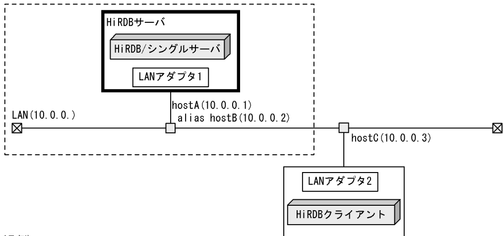
図 7-1 pd_security_host_group オペランドの指定例 (HiRDB/ シングルサーバの場合)
