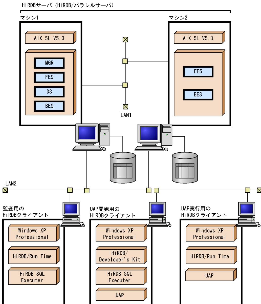
図 2-4 ISO/IEC 15408 の評価構成システム (HiRDB/パラレルサーバの場合)
