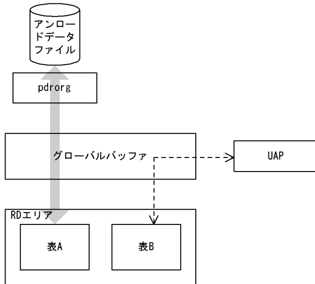
図 8-20 pdrorg とバッファの関係
