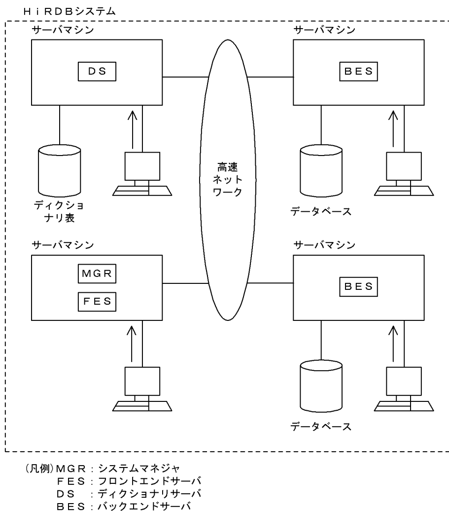
図 1-2 コマンドの実行形態 (HiRDB/パラレルサーバの場合)
