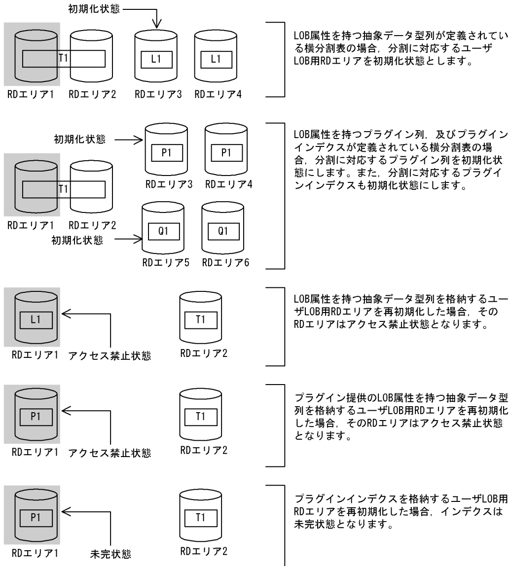
図 7-6 再初期化した後の表、LOB 属性の抽象データ型列、プラグインが提供する抽象データ型列、及びプラグインインデックスの状態
