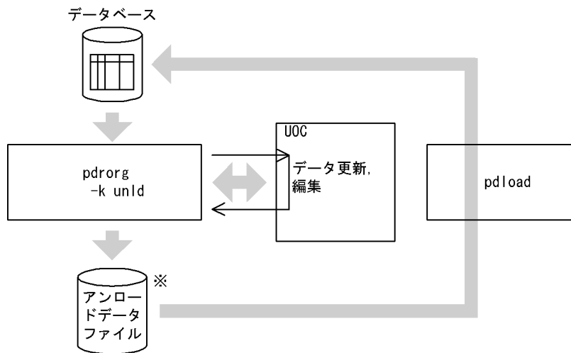
図 8-24 UOC を利用した再編成の概要 (アプリケーション向けデータ更新)
