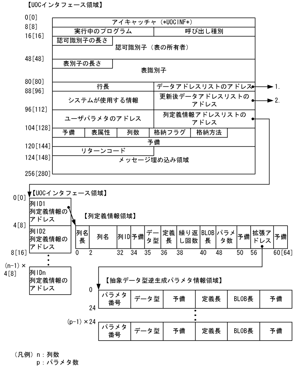
図 8-27 UOC インタフェース領域の構造 (1/2)
