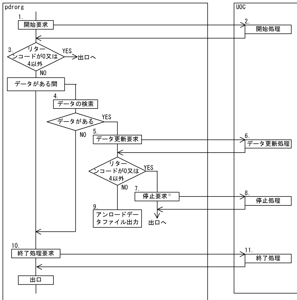
図 8-26 pdrorg, UOC 間の呼び出しシーケンス
