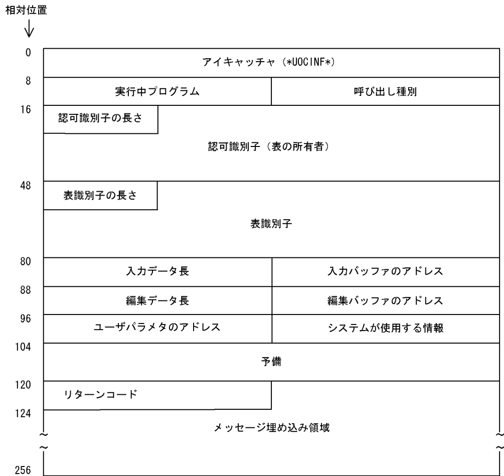
図 5-29 UOC インタフェース領域の構造 (32 ビットモードの場合)
