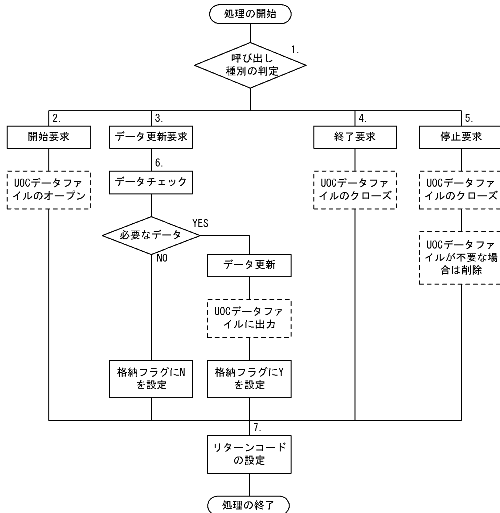
図 8-25 UOC の処理概要
