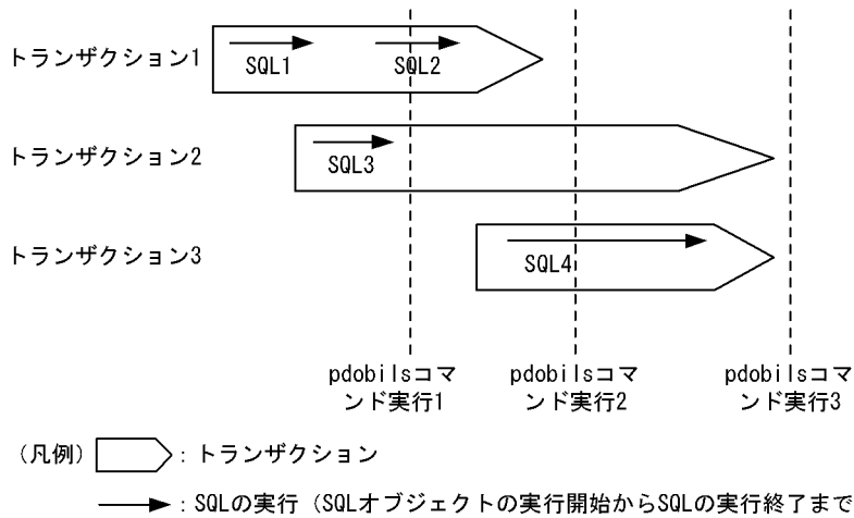
図 2-5 pdobils コマンド実行時に表示される SQL オブジェクトの実行時間
