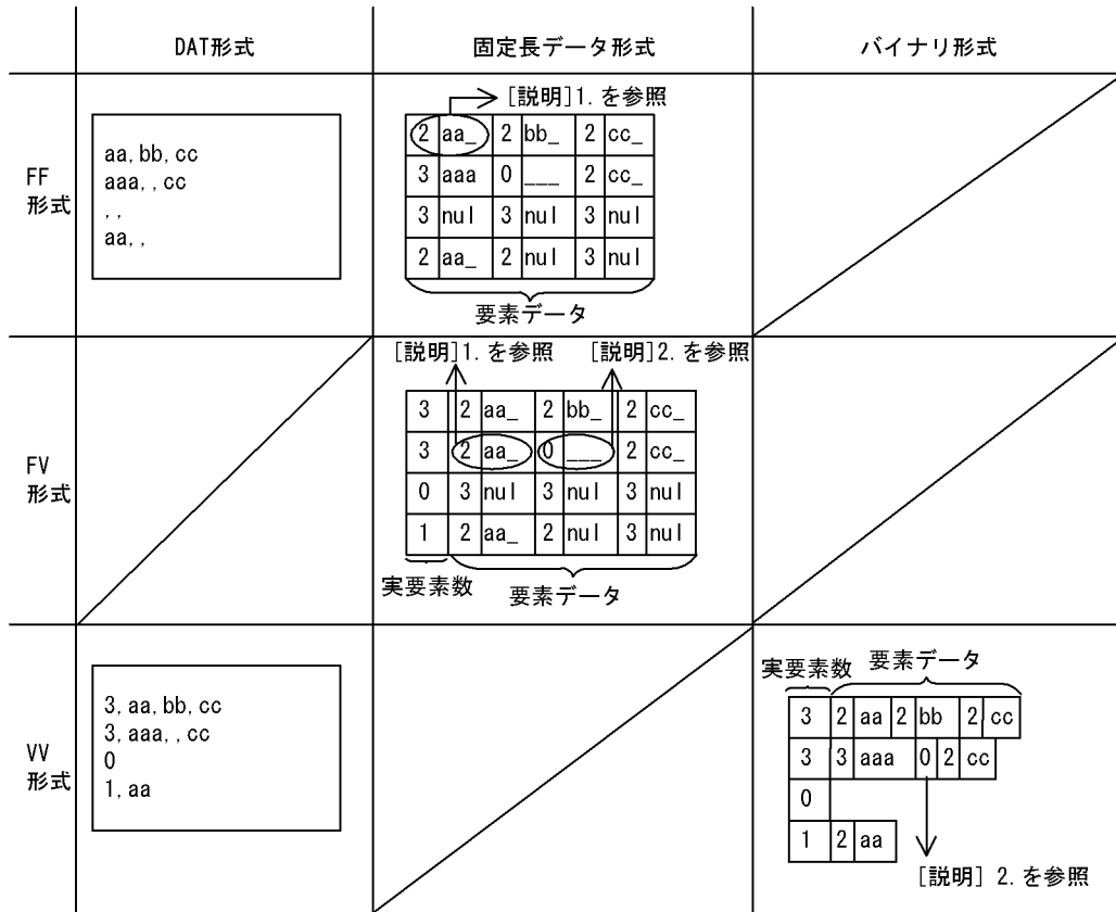
図 5-18 可変長データ型の場合の配列データの指定例
