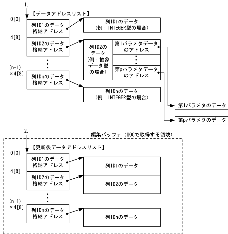
図 8-28 UOC インタフェース領域の構造 (2/2)
