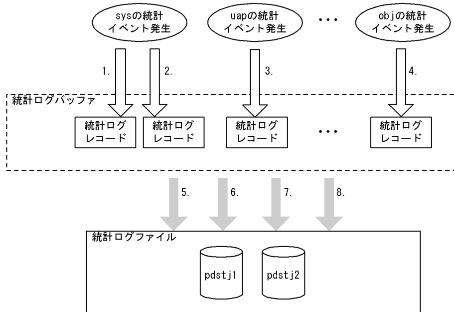
図 2-8 統計レコード出力タイミング、及び統計ログファイルへの出力タイミング
