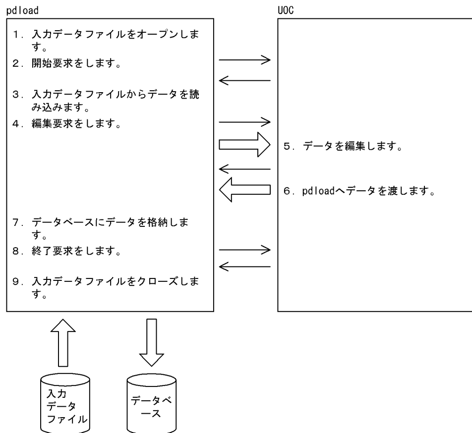
図 5-27 UOC を利用した場合の表の作成方法 (ユーティリティが入力データファイルを入力する方法)
