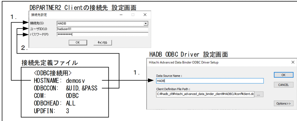
図 2-8 DBPARTNER2 Client, ODBC ドライバの指定値の関係 (HADB の場合)
