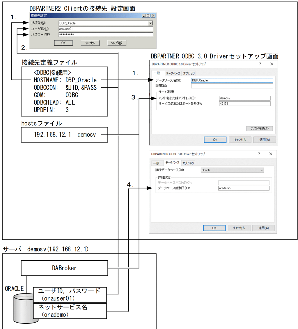
図 2-5 DBPARTNER2 Client, ODBC ドライバの指定値の関係 (ORACLE の場合)
