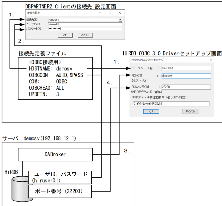
図 2-6 DBPARTNER2 Client, ODBC ドライバの指定値の関係 (HiRDB の場合)
