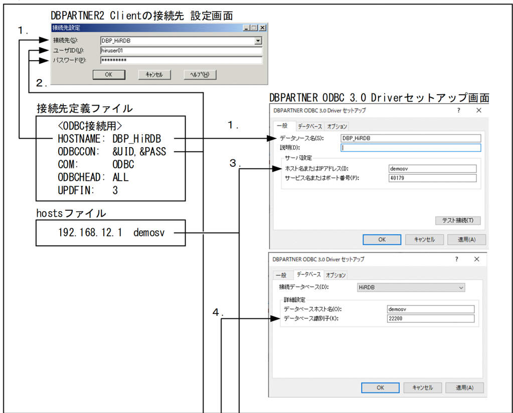
図 2-4 DBPARTNER2 Client, ODBC ドライバの指定値の関係 (HIRDB の場合)
