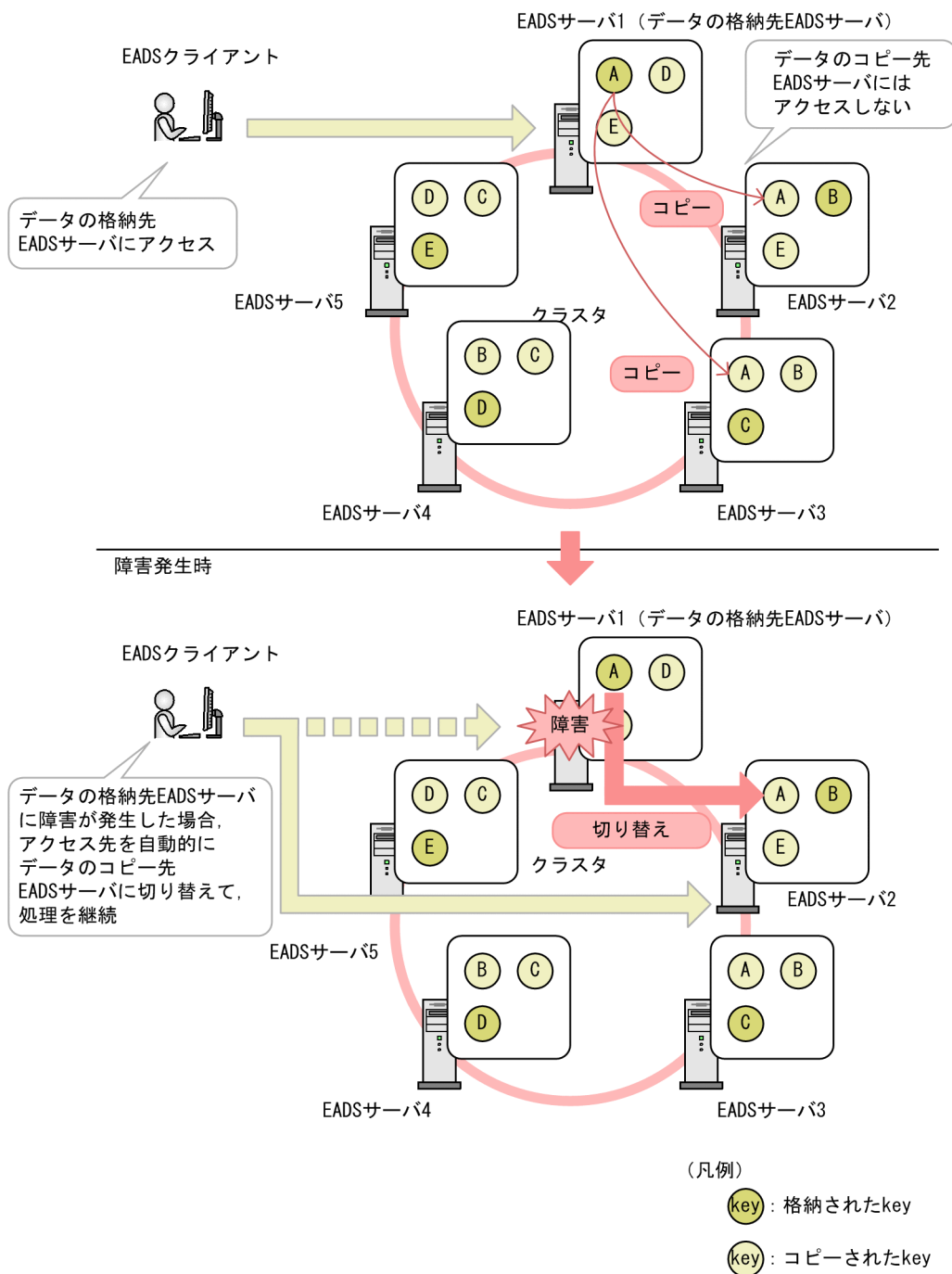
図 2-27 データを多重化している場合のデータアクセスと障害発生時のアクセス先の切り替え
