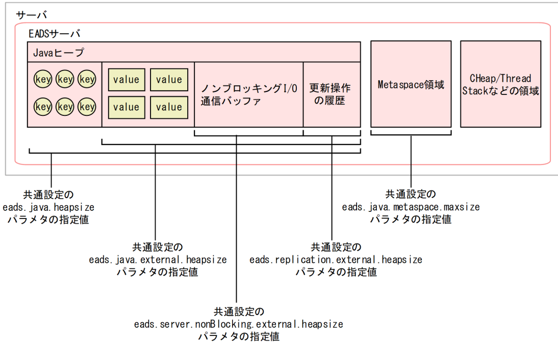
図 4-1 メモリ構成
