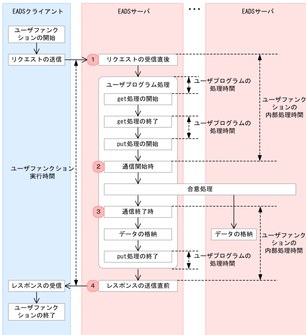
図 11-2 統計情報が取得される箇所（ユーザファンクションの統計情報）
