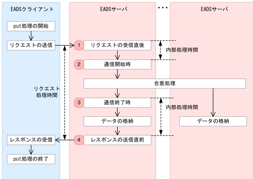
図 11-1 EADS サーバの性能測定に使用する統計情報が取得される箇所 (put 処理の例)
