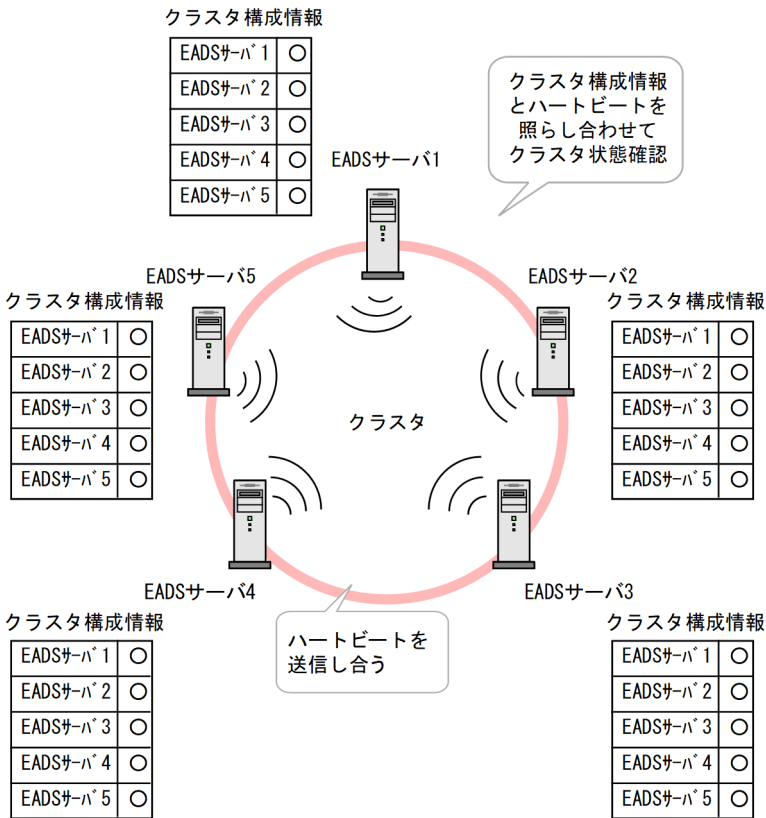
図 2-28 クラスタ監視の概要
