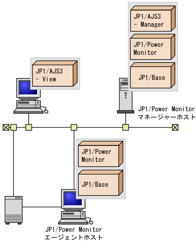
図 4-4 JP1/AJS3 と連携して他ホストを起動・終了する場合のシステム構成例
