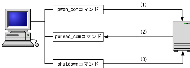
図 6-2 次回電源投入時刻を随時設定できる電源制御装置の場合のコマンドの処理
