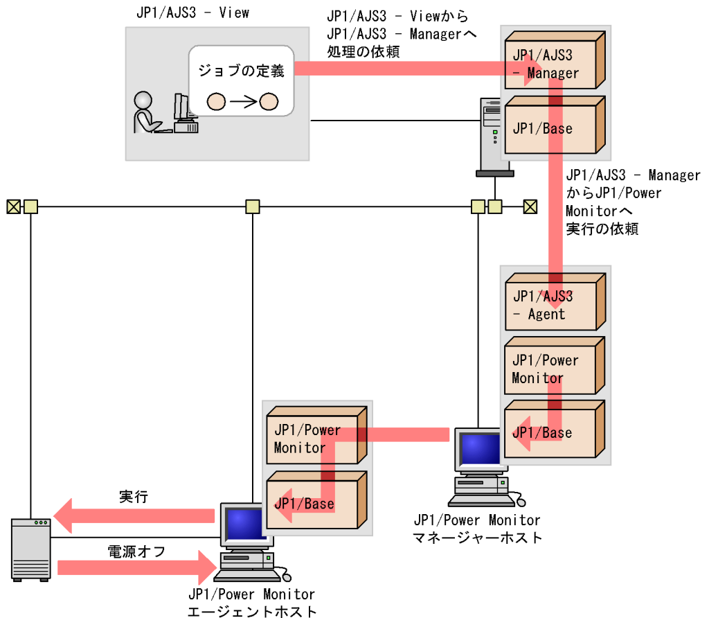
図 1-18 JP1/AJS3 が組み込まれたホストから別のホストを終了する
