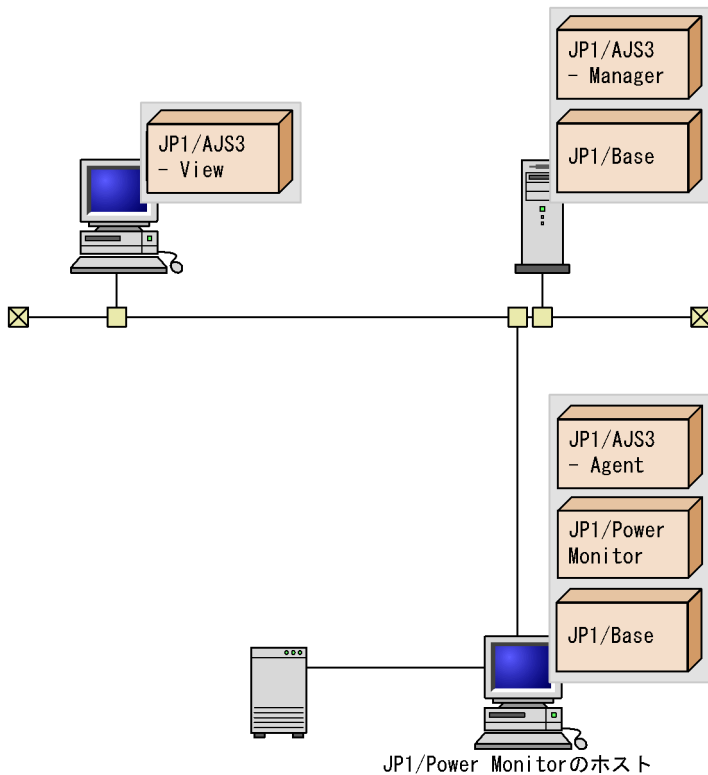
図 4-3 JP1/AJS3 と連携して自ホストを起動・終了する場合のシステム構成例
