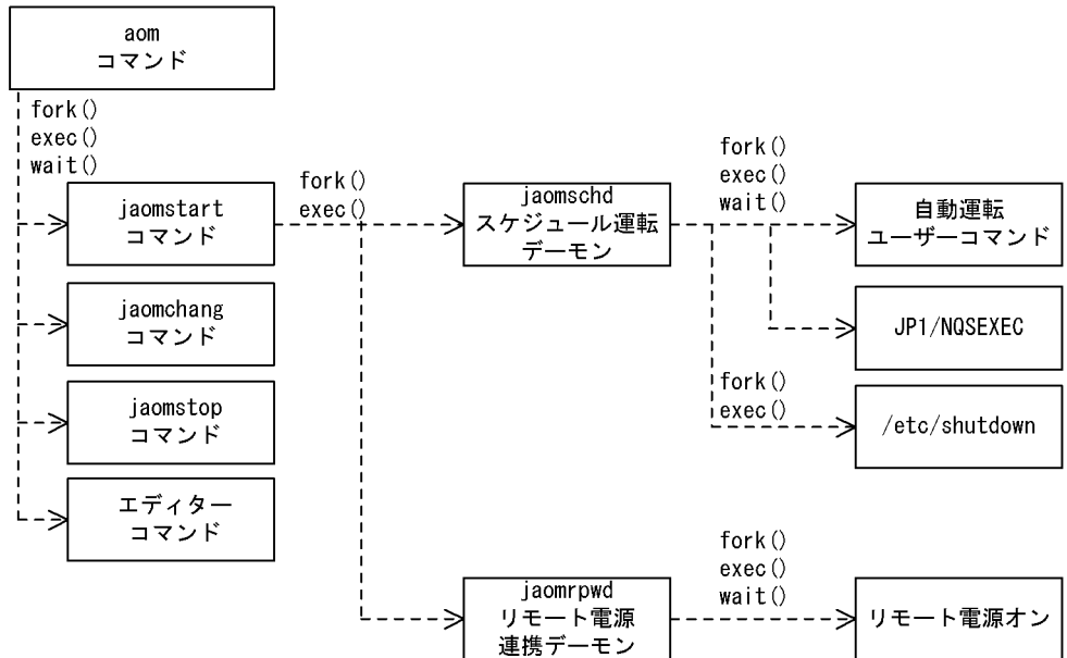
図 B-4 UNIX ホストで JP1/Power Monitor を実行する際のプロセス構成
