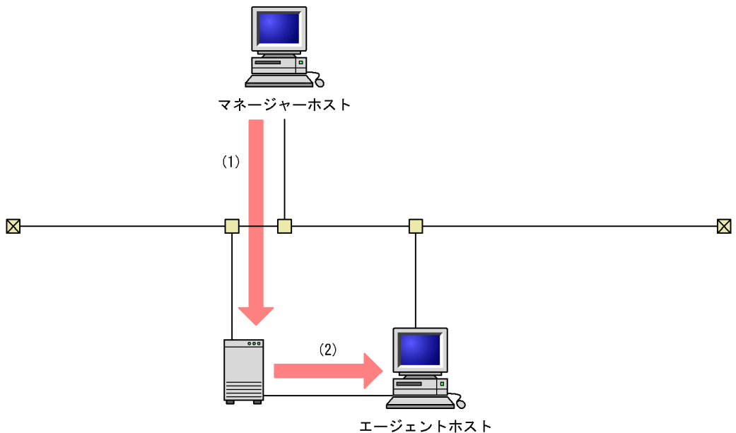
図 1-4 エージェントホストに接続されている電源制御装置を直接制御してホストの電源をオン・オフする流れ
