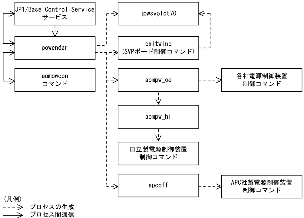
図 B-1 Windows ホストで自ホストを起動・終了する場合のプロセス構成
