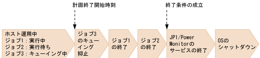
図 1-9 計画終了の流れ
