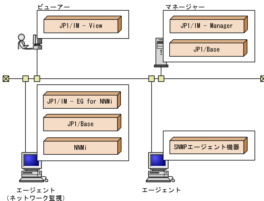
図 1-2 JP1/IM - EG for NNMi のシステム構成の例
