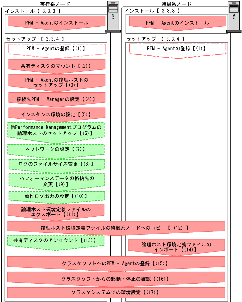
図 3-3 クラスタシステムで論理ホスト運用する PFM - Agent for DB2 のインストールおよびセットアップの流れ
