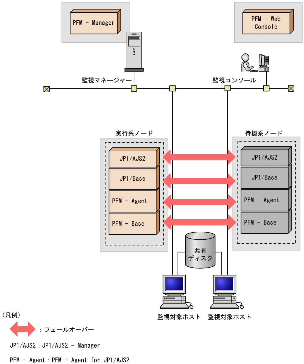
図 4-1 HA クラスタシステムでの PFM - Agent for JP1/AJS2 の構成例
