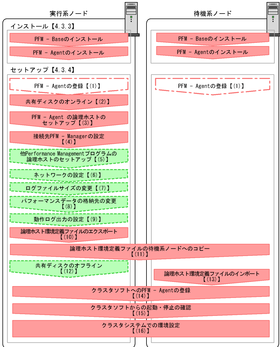
図 4-3 クラスタシステムで論理ホストとして運用する PFM - Agent for JP1/AJS2 のインストールおよびセットアップの流れ (Windows の場合)
