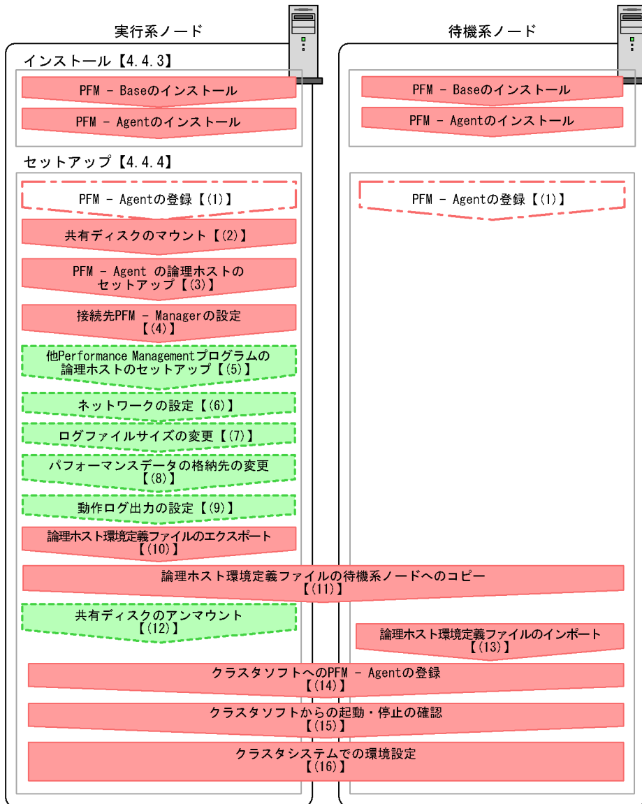
図 4-4 クラスタシステムで論理ホストとして運用する PFM - Agent for JP1/AJS2 のインストールおよびセットアップの流れ (UNIX の場合)
