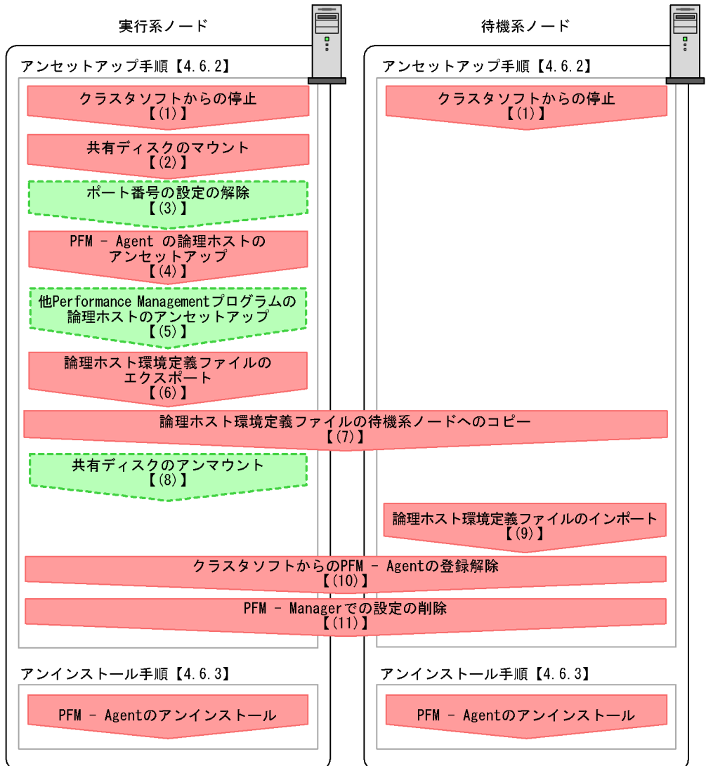
図 4-6 クラスタシステムで論理ホストとして運用する PFM - Agent for JP1/AJS2 のアンインストールおよびアンセットアップの流れ (UNIX の場合)
