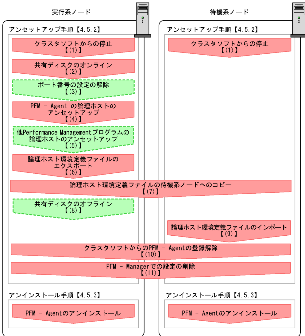
図 4-5 クラスタシステムで論理ホストとして運用する PFM - Agent for JP1/AJS2 のアンインストールおよびアンセットアップの流れ (Windows の場合)
