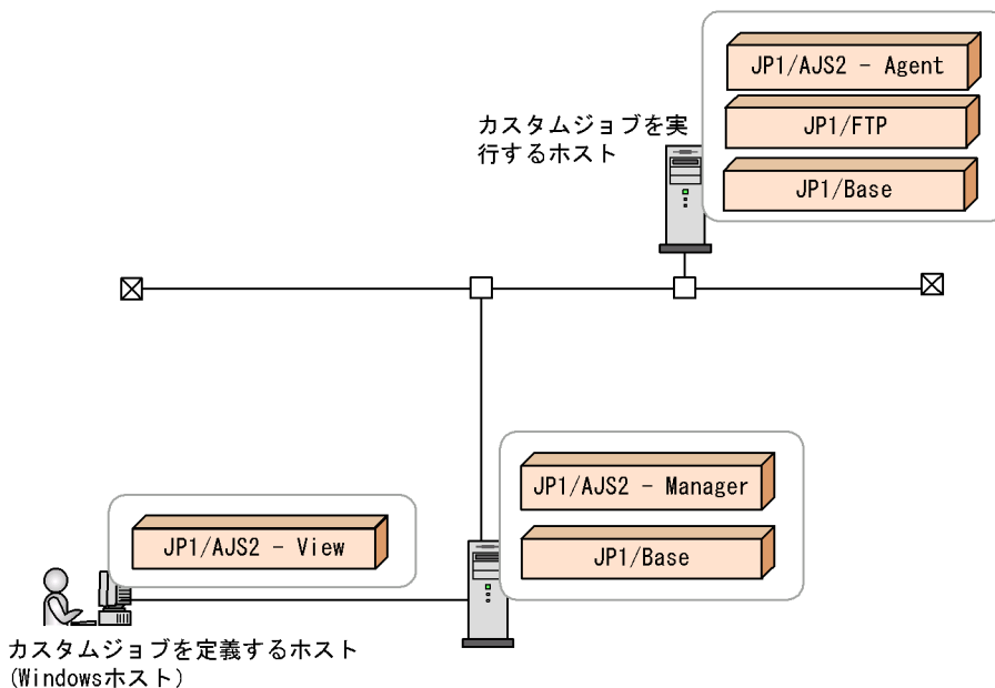
図 5-1 JP1/AJS2 と連携する場合のシステム構成例
