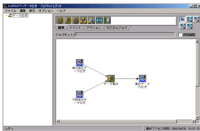
図 5-6 ジョブネット設定例
