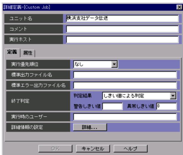
図 5-4 [ 詳細定義 - [ Custom Job ] ] ダイアログボックス設定例
