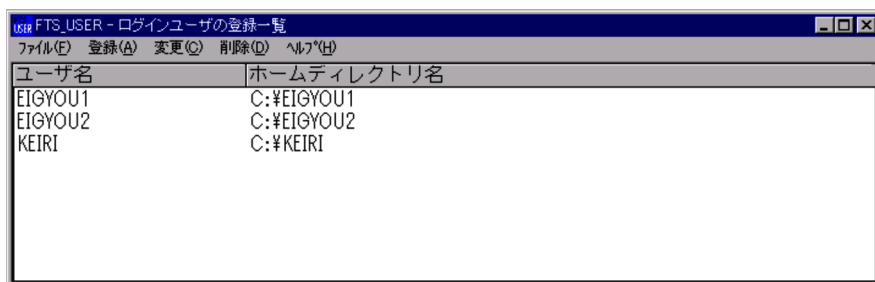
図 3-2 [ ログインユーザの登録一覧 ] ウィンドウ
