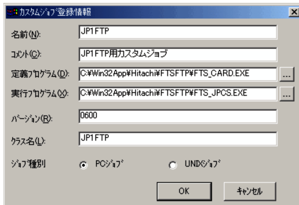
図 5-2 [ カスタムジョブ登録情報 ] ダイアログボックス
