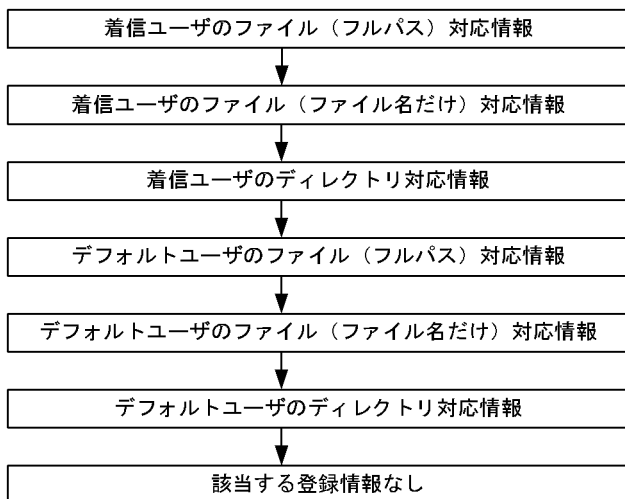
図 3-7 自動起動プログラム起動時の優先順位
