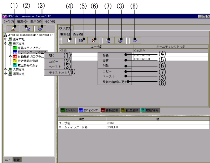
図 4-4 ログインユーザの登録画面
