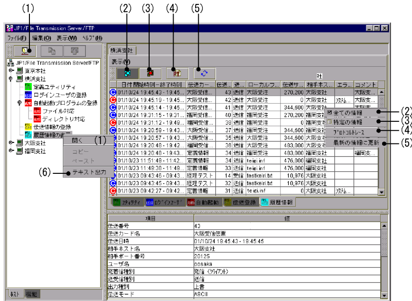
図 4-7 履歴情報の表示画面
