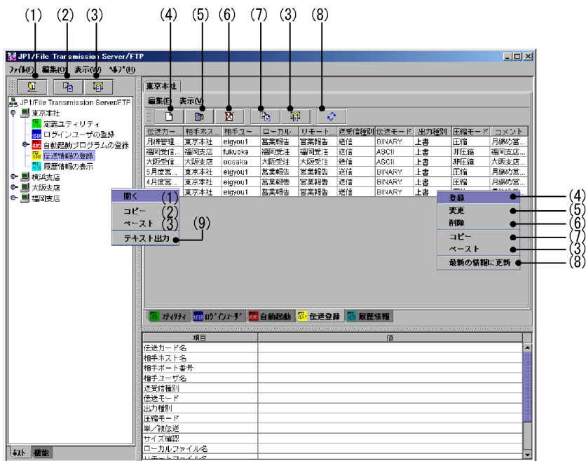
図 4-6 伝送情報の登録画面
