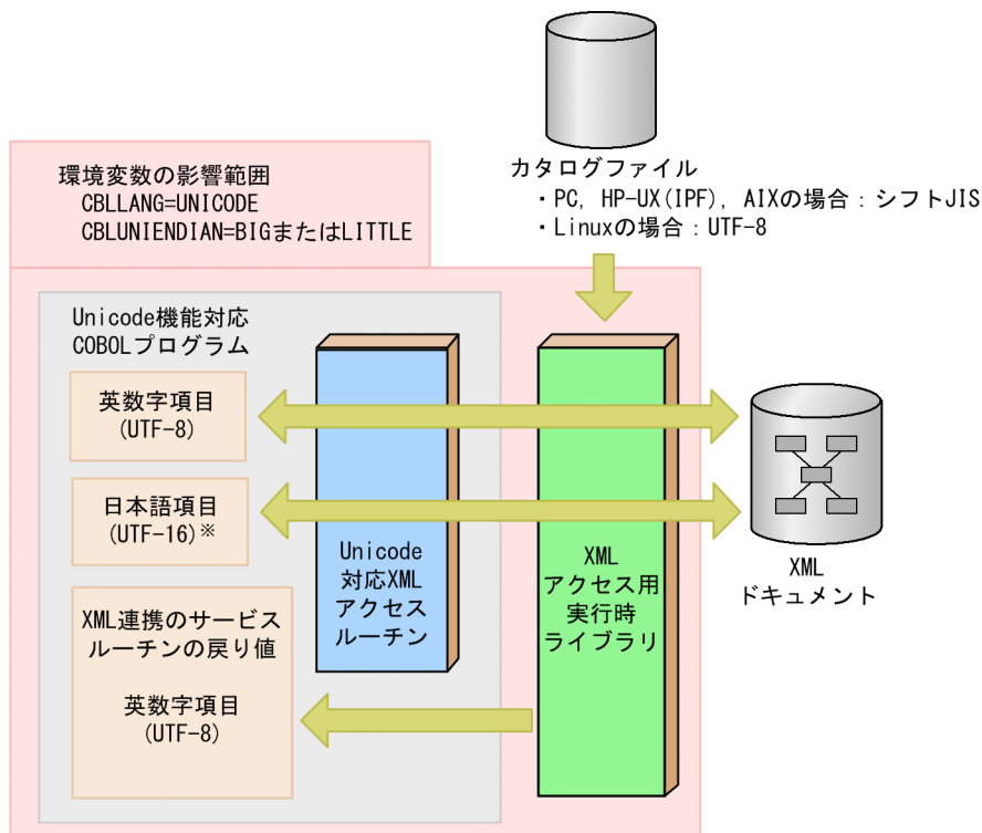
図 H-2 Unicode 機能に対応した XML 連携機能を使用する COBOL プログラムでの文字コード
