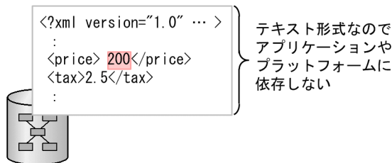
図 1-1 XML の特長
