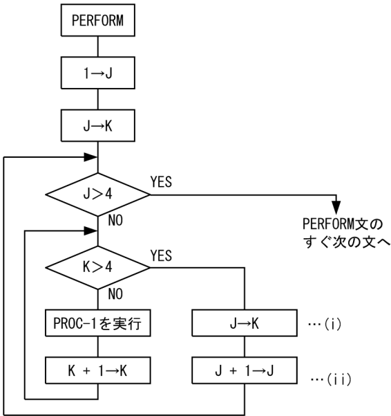
図 25-1 PERFORM 文の流れ
