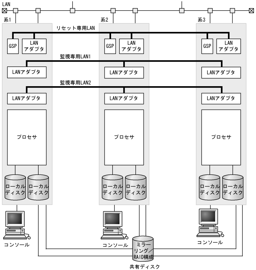
図 5-19 複数スタンバイ構成時のハードウェア構成例 (H9000V)
