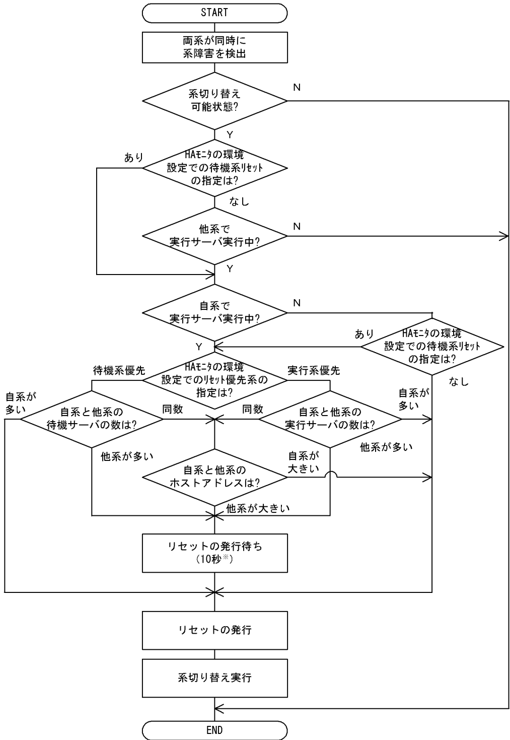
図 4-11 HA モニタリセット優先系を決定する方法
