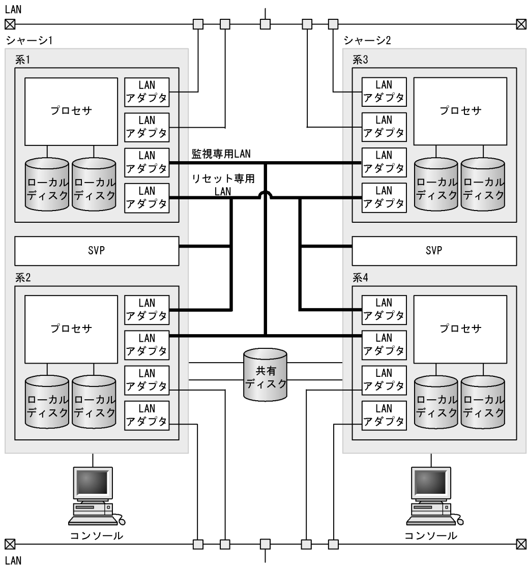
図 5-16 クラスタ型系切り替え構成時のハードウェア構成例 (BladeSymphony)
