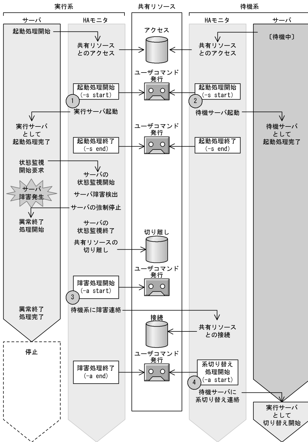
図 6-27 ユーザコマンドのコーディング例で示す発行タイミング
