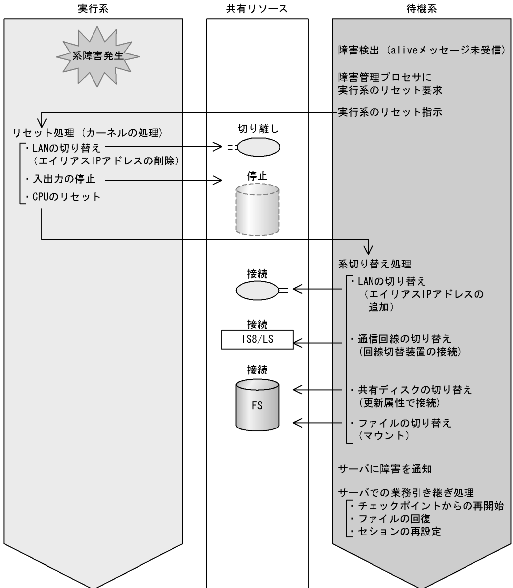
図 2-8 系障害時の系切り替えの概要
