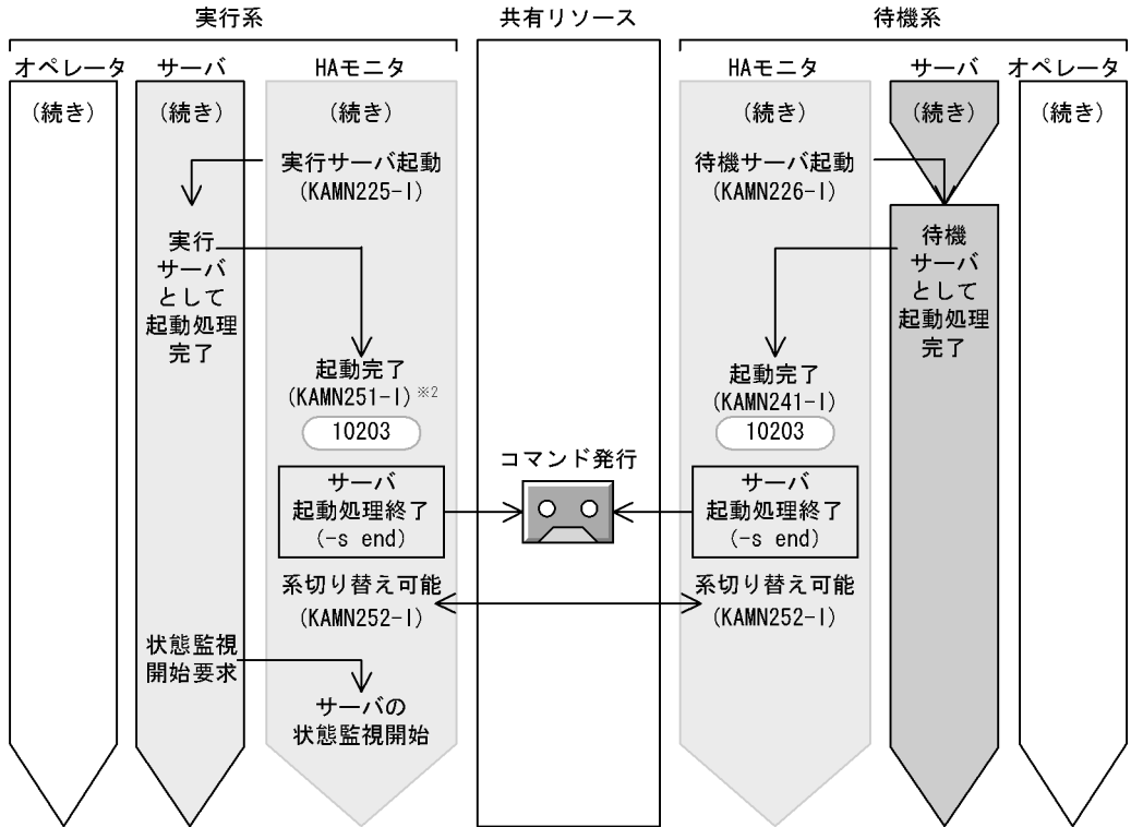
図 4-36 サーバの起動処理の流れ (サーバの起動処理完了からサーバの状態監視開始まで) (サーバモード)
