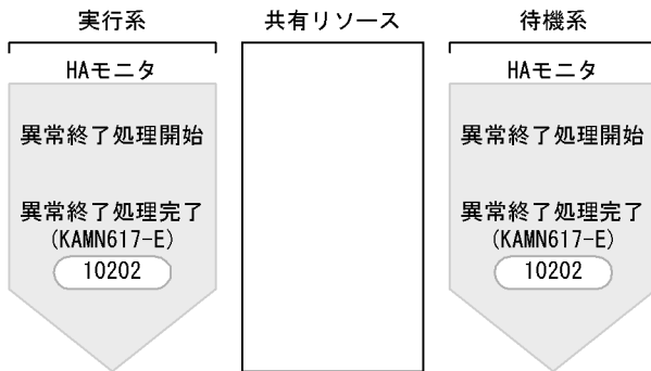
図 A-6 HA モニタ異常終了時のイベント発行タイミング
