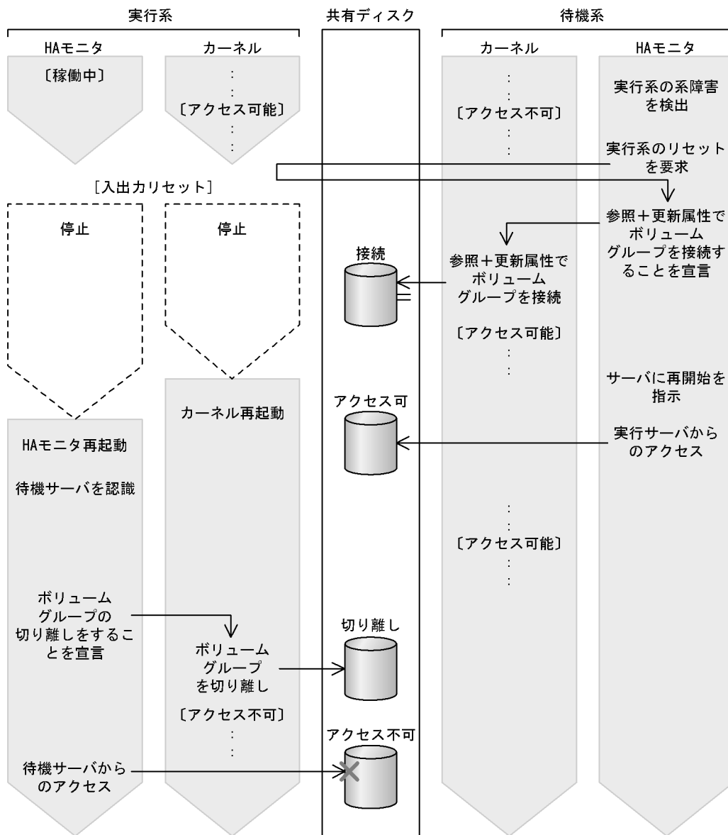
図 4-17 系障害時の共有ディスクの切り替えの流れ
