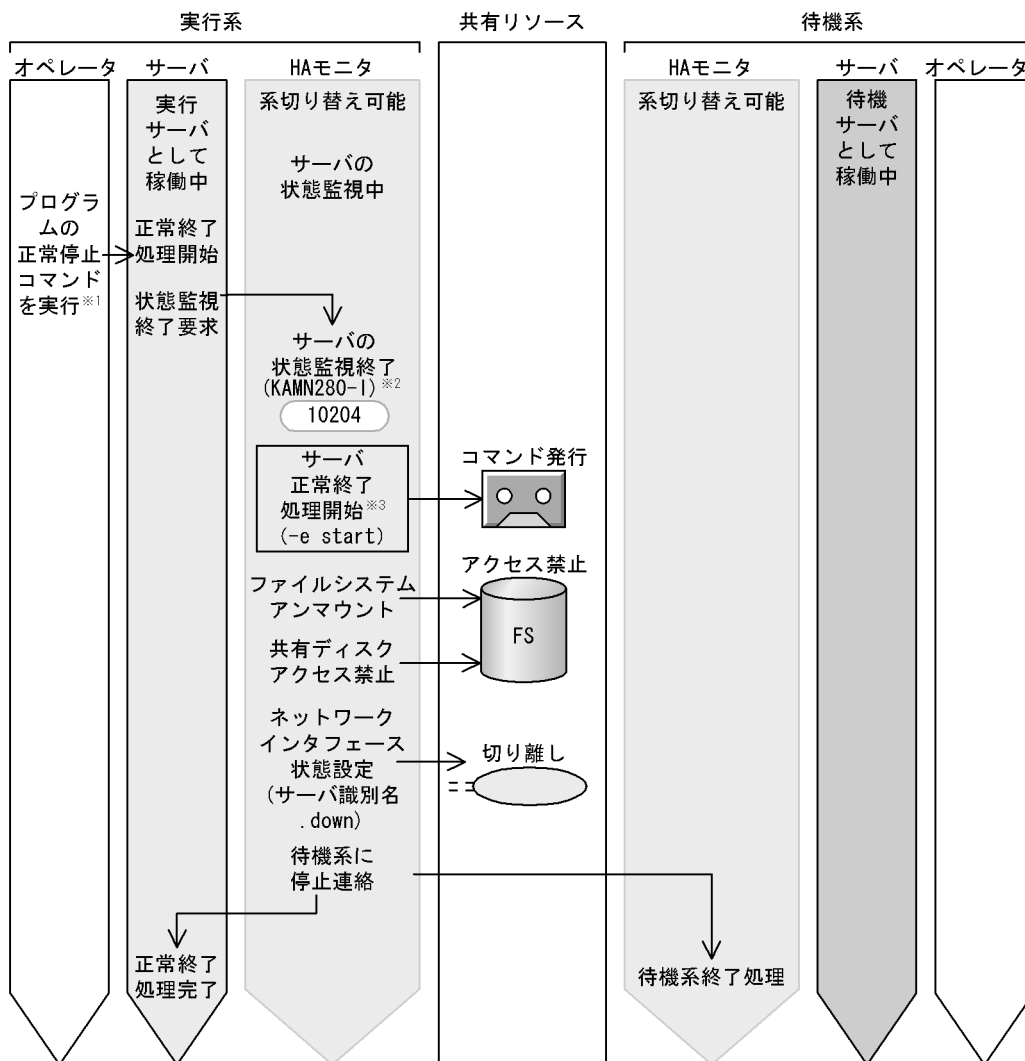
図 4-53 共有リソースの切り離しを接続時と逆順にする場合の、サーバの停止処理の流れ（サーバの状態監視終了から共有リソースの切り離しまで）（サーバモード：実行サーバの停止処理終了時に待機サーバを停止する）
