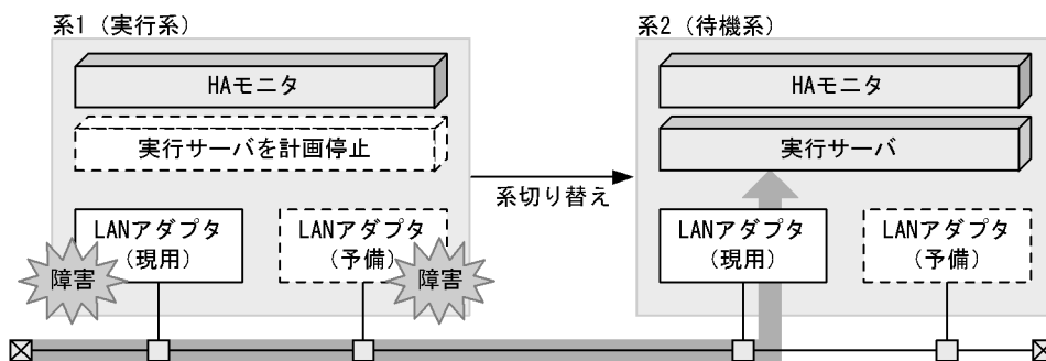
図 3-16 LAN アダプタ二重障害時の系切り替えの流れ
