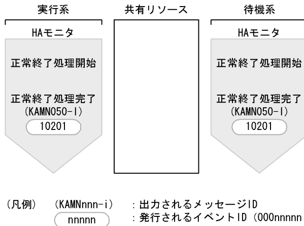
図 A-4 HA モニタ正常終了時のイベント発行タイミング
