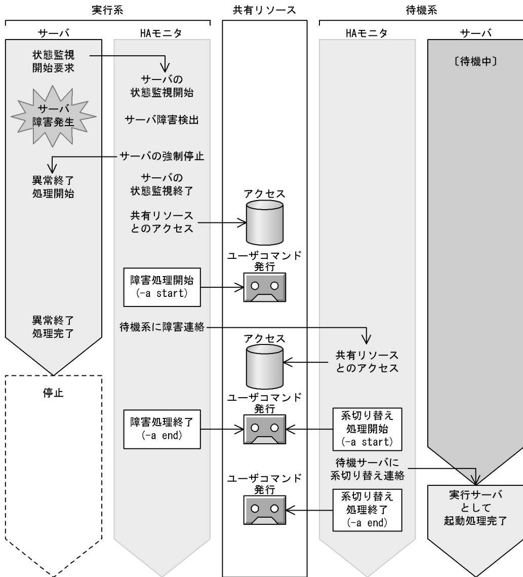
図 6-17 実行サーバ障害時に渡されるパラメタと発行タイミング
