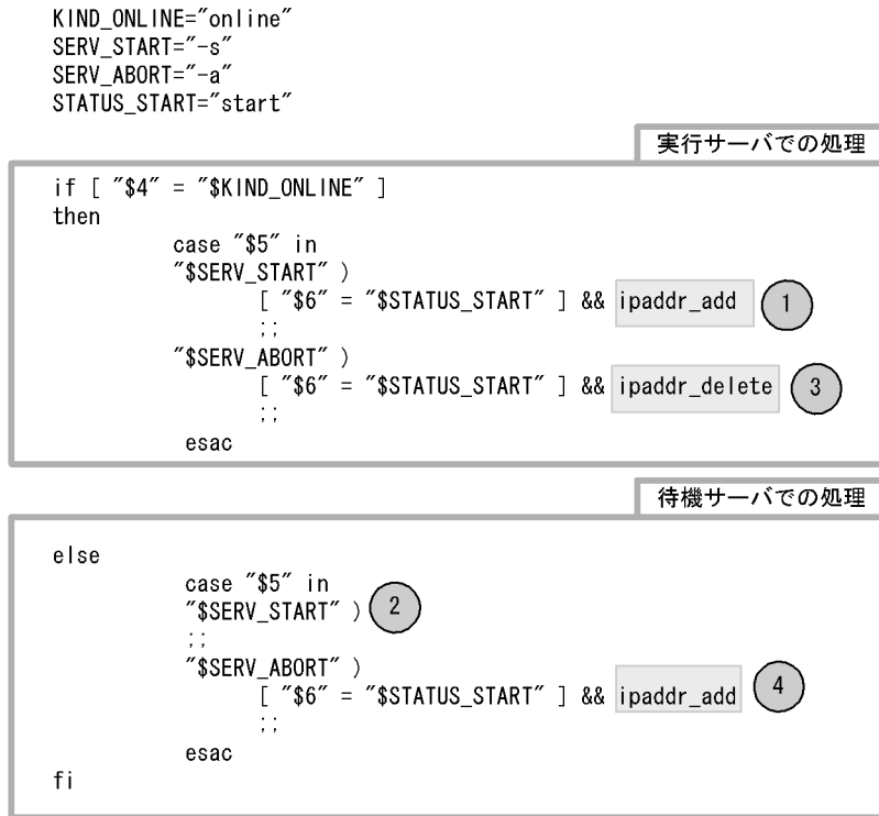
図 6-28 ユーザコマンドのコーディング例と発行タイミングの対応
