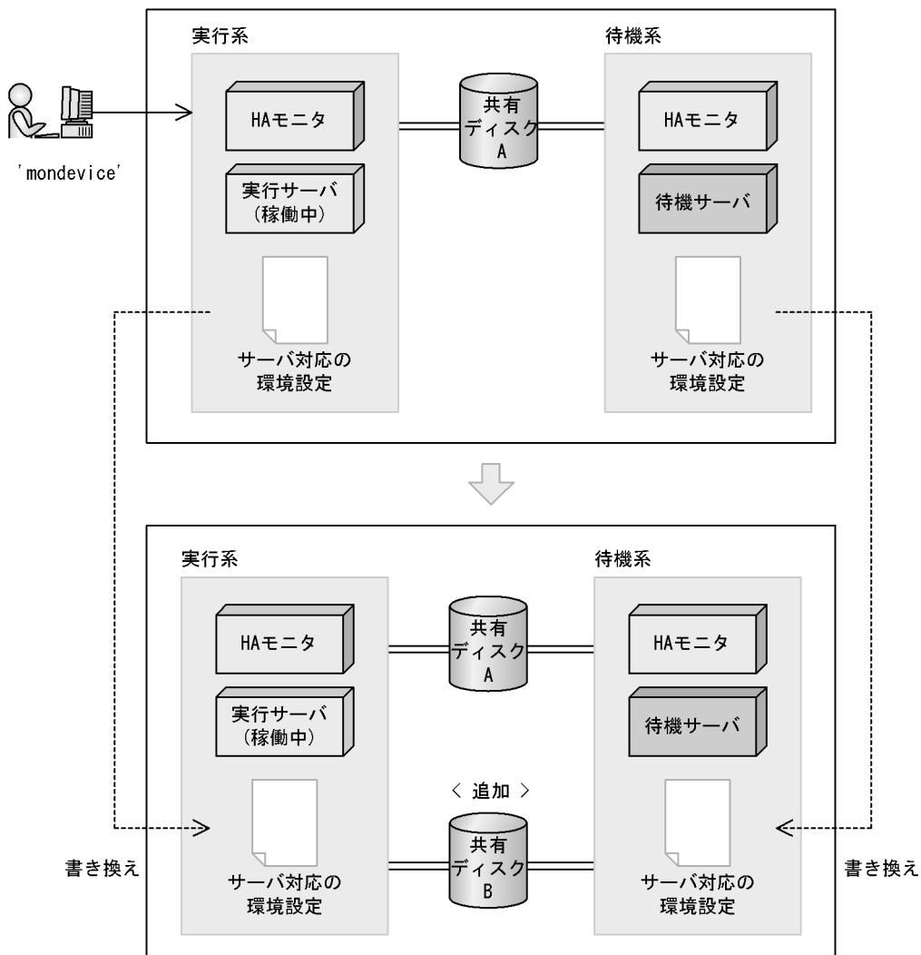
図 3-11 HA モニタの mondevice コマンドを使用した共有リソースの動的変更の概要
