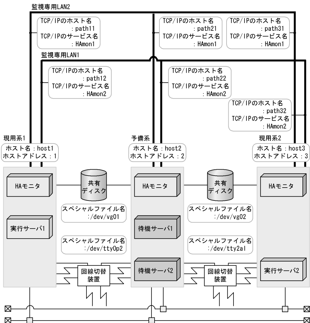
図 8-9 2:1 系切り替え構成時のシステム構成
