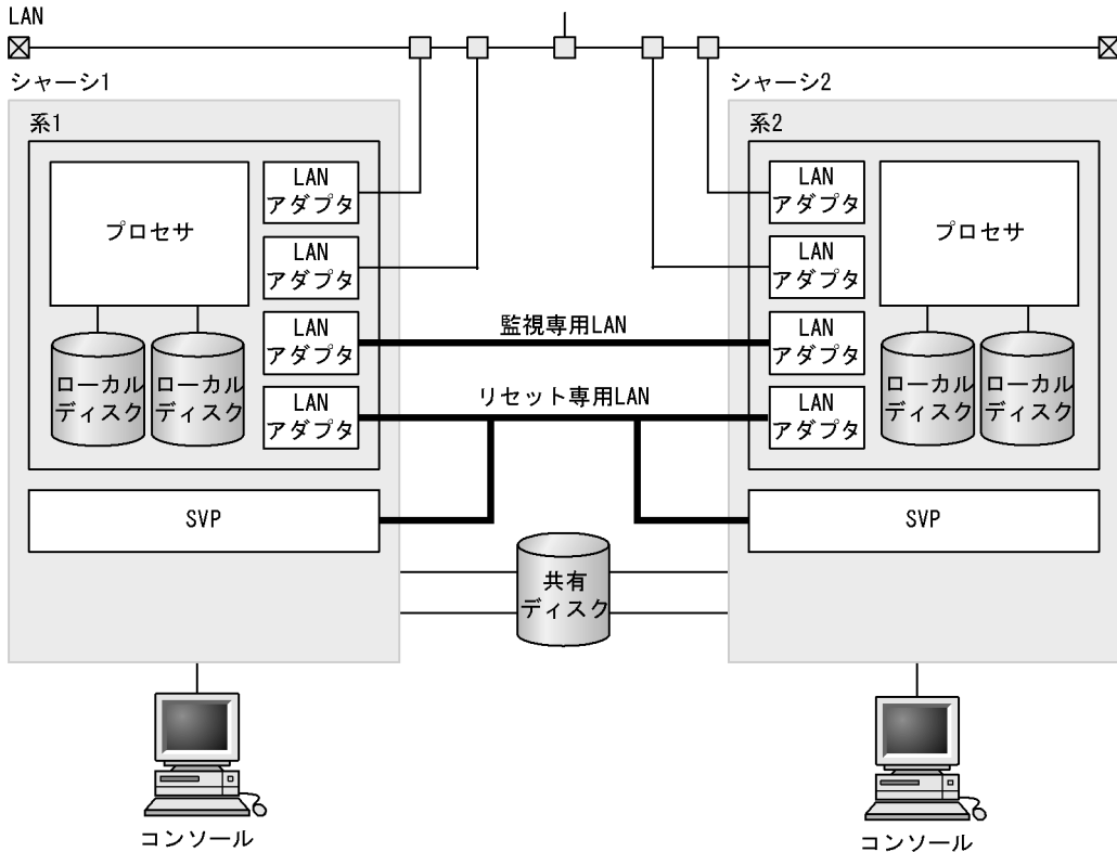
図 5-14 二つのシャーシ間での 1:1 系切り替え構成時のハードウェア構成例 (BladeSymphony)
