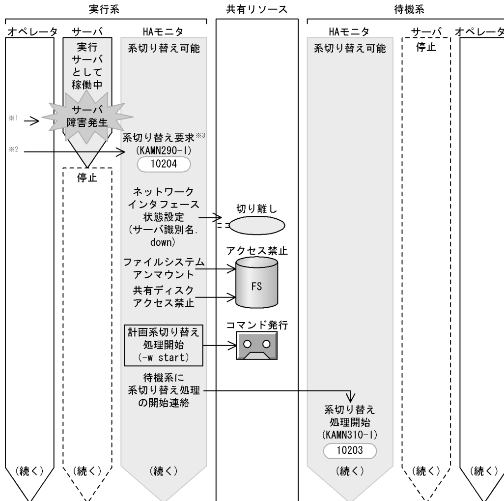
図 4-47 サーバ障害時の系切り替え処理の流れ (共有リソースの切り離しから系切り替え開始まで)(モニタモード)
