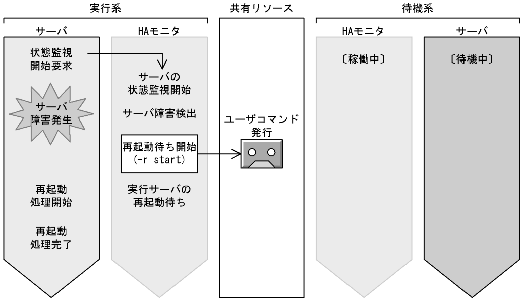
図 6-20 実行サーバ再起動待ち時に渡されるパラメタと発行タイミング
