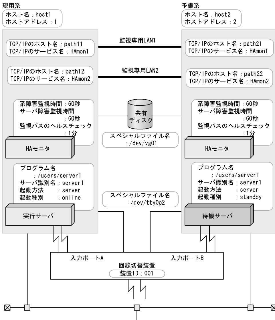
図 8-2 HT-4990-KIRIKV または HT-4990-KIRIKX の回線切替装置使用時のシステム構成 (H9000V)
