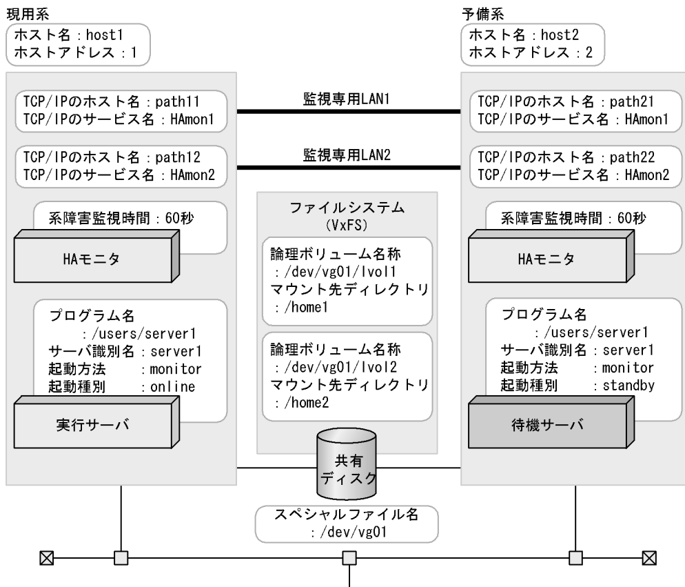
図 8-6 ファイルシステム使用時のシステム構成
