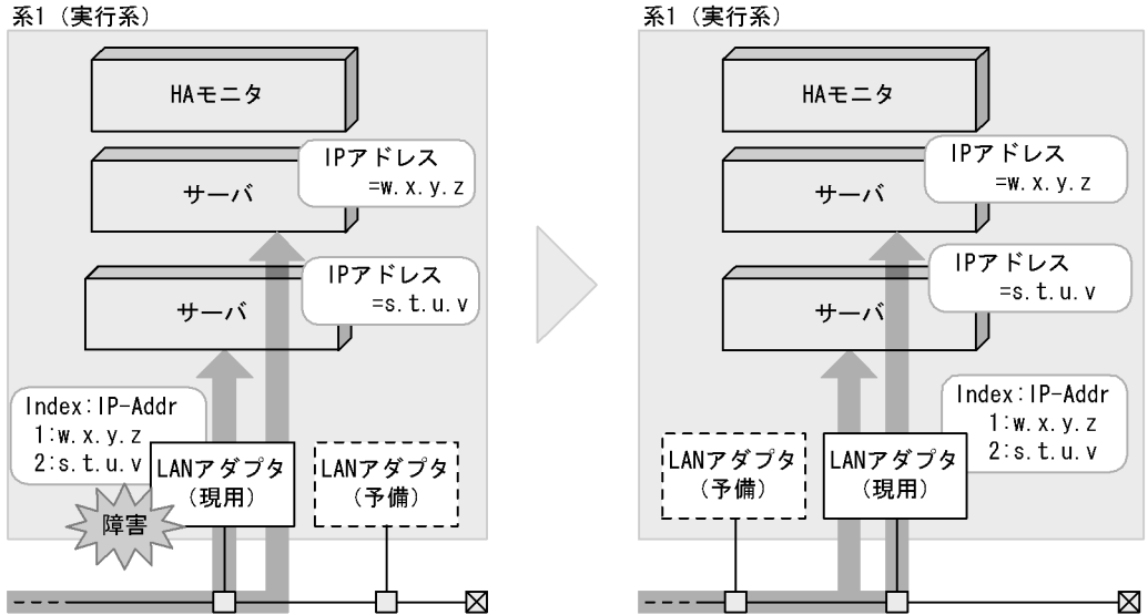
図 3-15 複数の IP アドレスが設定されている場合の LAN アダプタの切り替え
