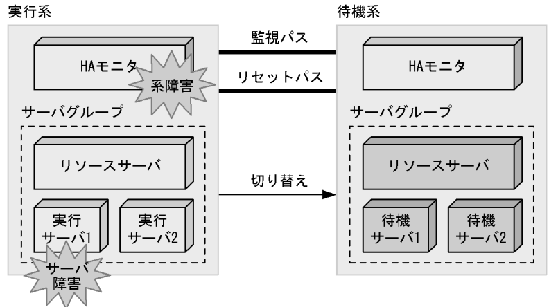
図 4-31 リソースサーバを使用した場合の系切り替え
