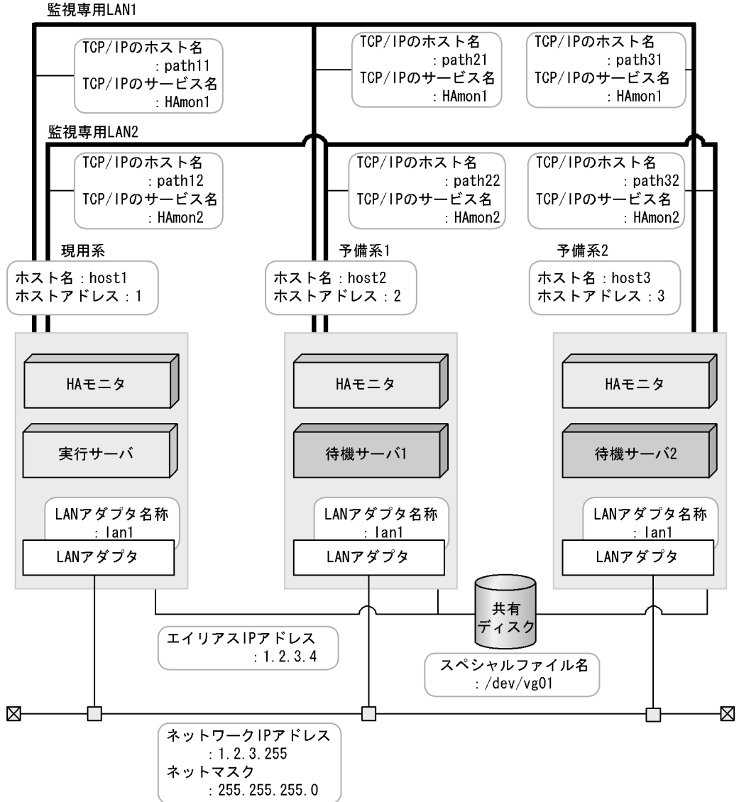
図 8-10 複数スタンバイ構成時のシステム構成
