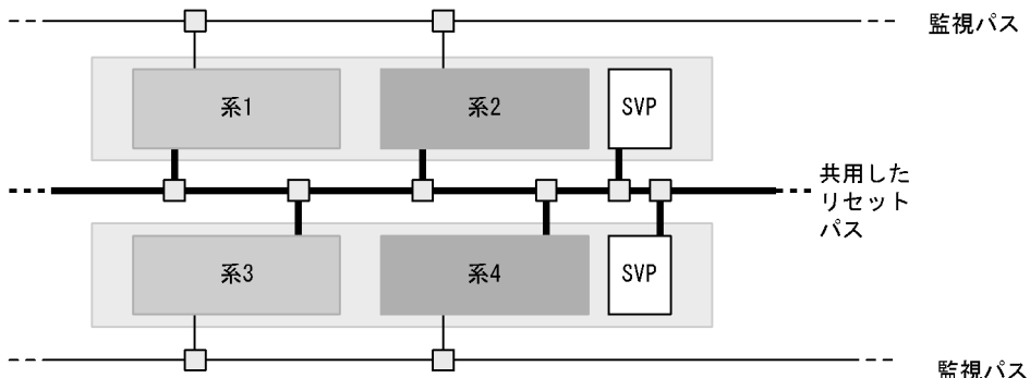
図 5-3 系切り替え構成間でリセットパスを共用したネットワーク構成 (SVP を共用する場合)
