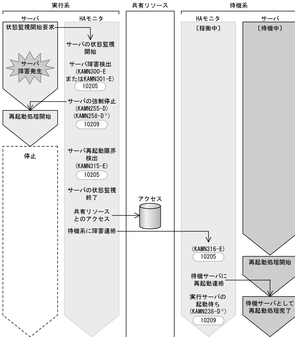
図 A-17 サーバ再起動限界時 (switchtype = manual) のイベント発行タイミング
