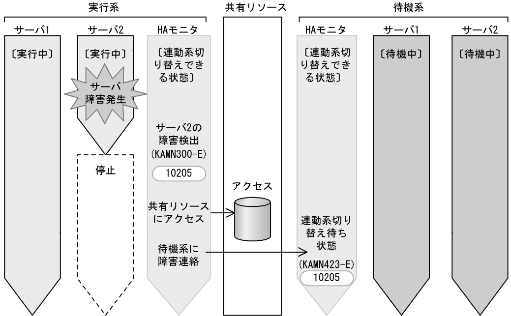
図 A-22 サーバ障害時 (group = no_exchange) のイベント発行タイミング
