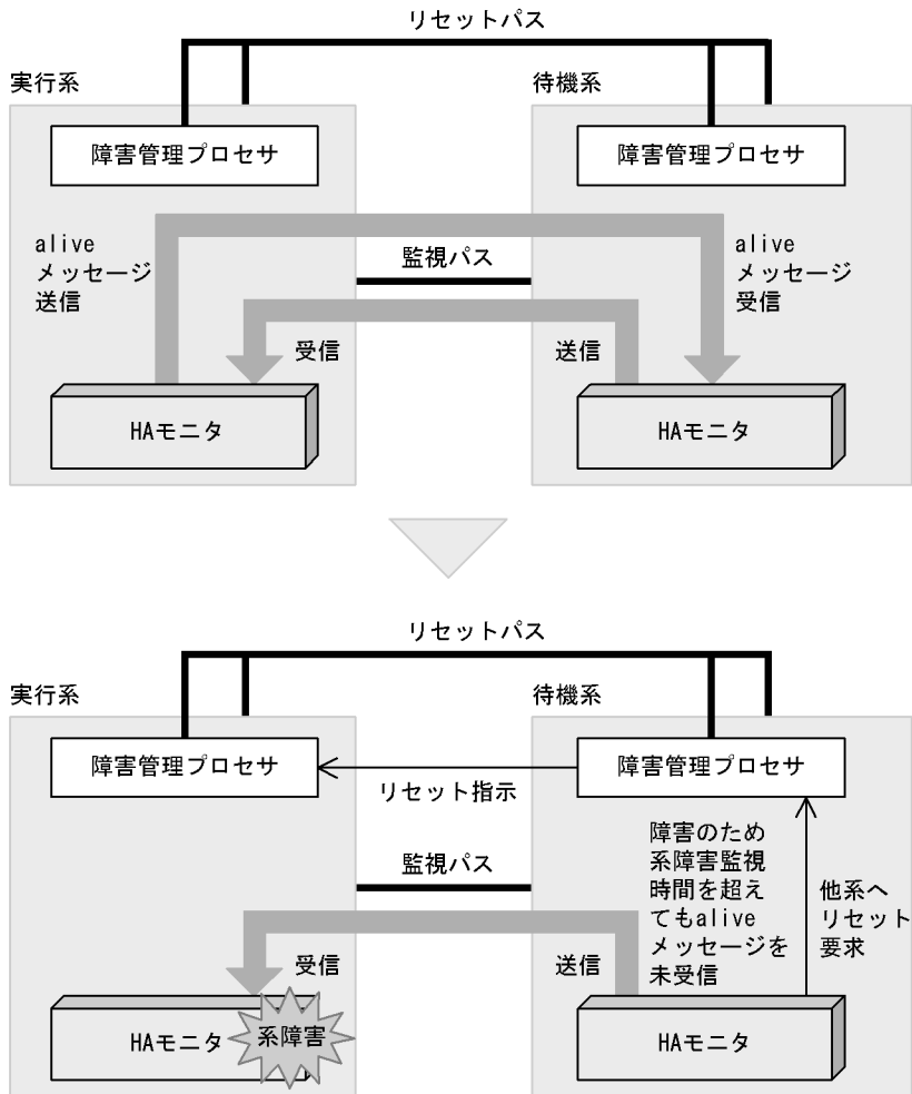
図 2-10 系の状態監視と系のリセット
