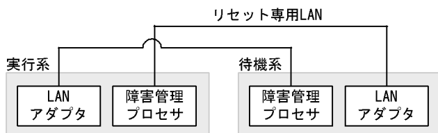
図 5-10 リセット専用 LAN の接続構成（相互に直接接続する場合）
