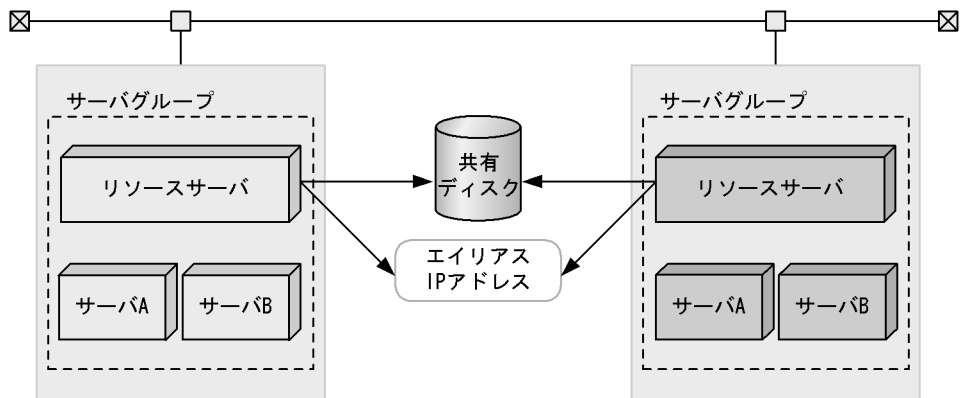
図 5-5 一つのリソースサーバから、複数の共有リソースを共用する構成
