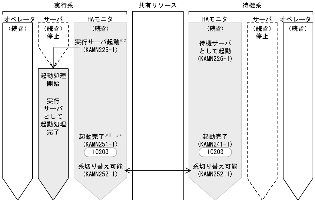
図 4-38 サーバの起動処理の流れ (サーバの起動処理完了) (モニタモード)
