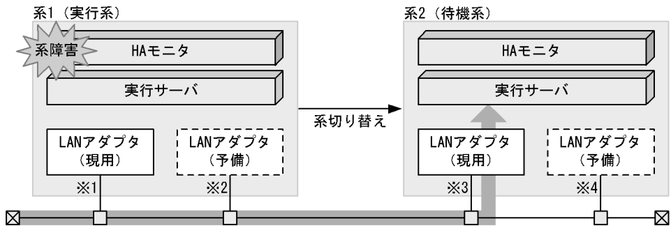
図 3-14 系障害による系切り替え発生後の LAN アダプタの状態
