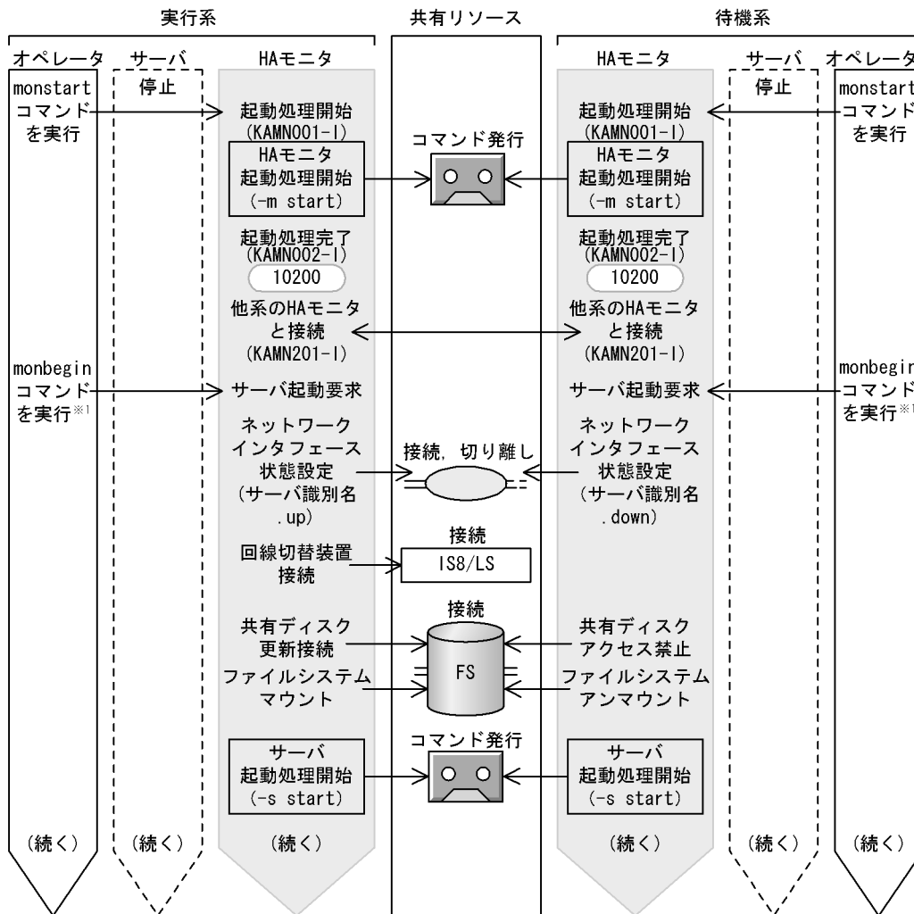
図 4-37 サーバの起動処理の流れ (HA モニタの起動からサーバの起動処理開始まで) (モニターモード)
