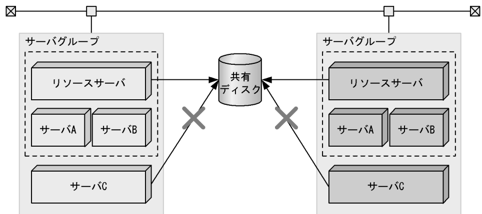
図 5-7 リソースサーバを使用して共有リソースの共用を実現できない構成
