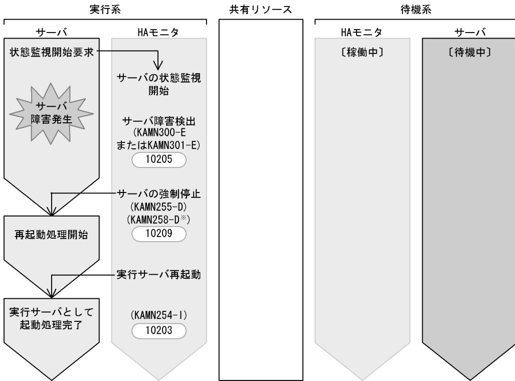
図 A-15 サーバ障害時 (switchtype = manual) のイベント発行タイミング
