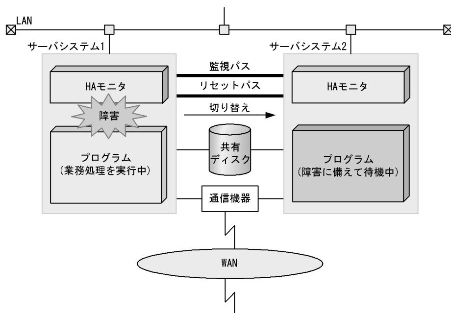
図 1-1 HA モニタの概要
