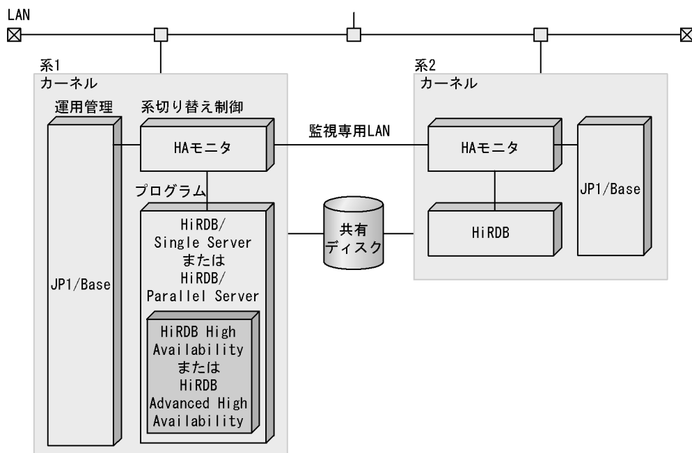
図 1-11 プログラムに HiRDB を使用する場合のソフトウェア構成例
