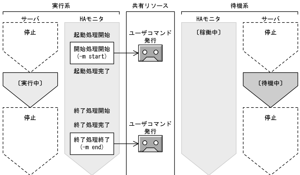
図 6-25 HA モニタ開始・終了時に渡されるパラメタと発行タイミング
