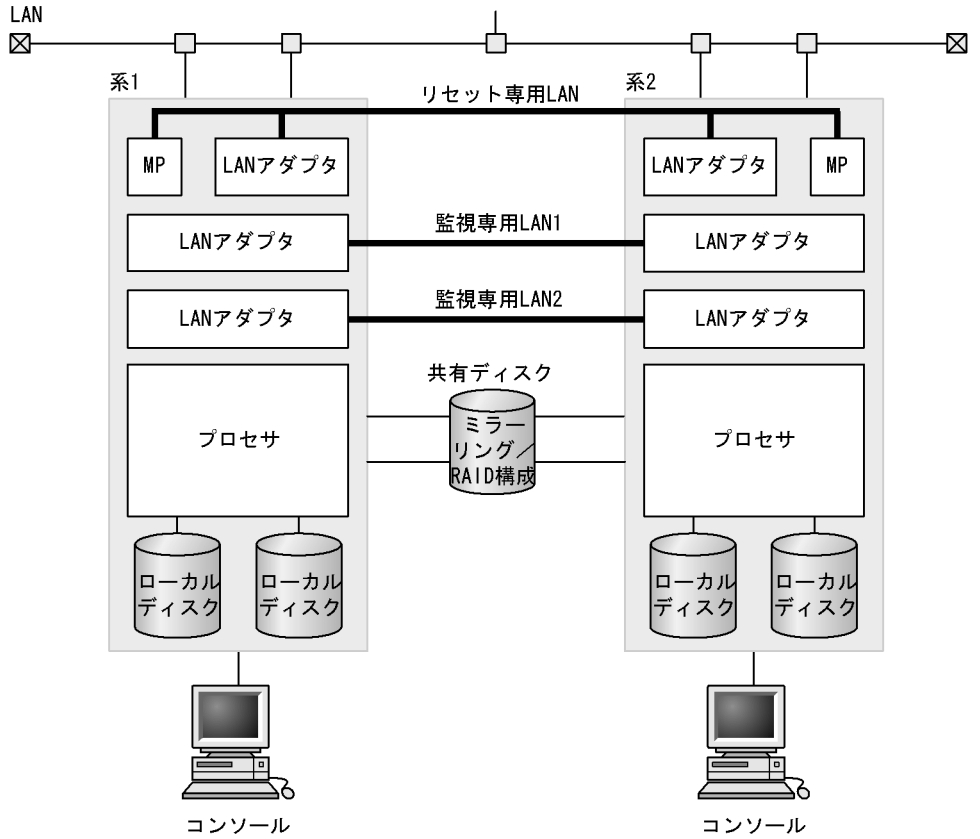
図 5-21 1:1 系切り替え構成時のハードウェア構成例 (HA8500)
