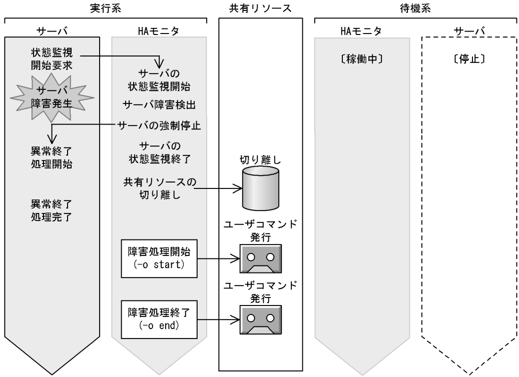
図 6-18 系切り替え不可能時に渡されるパラメタと発行タイミング
