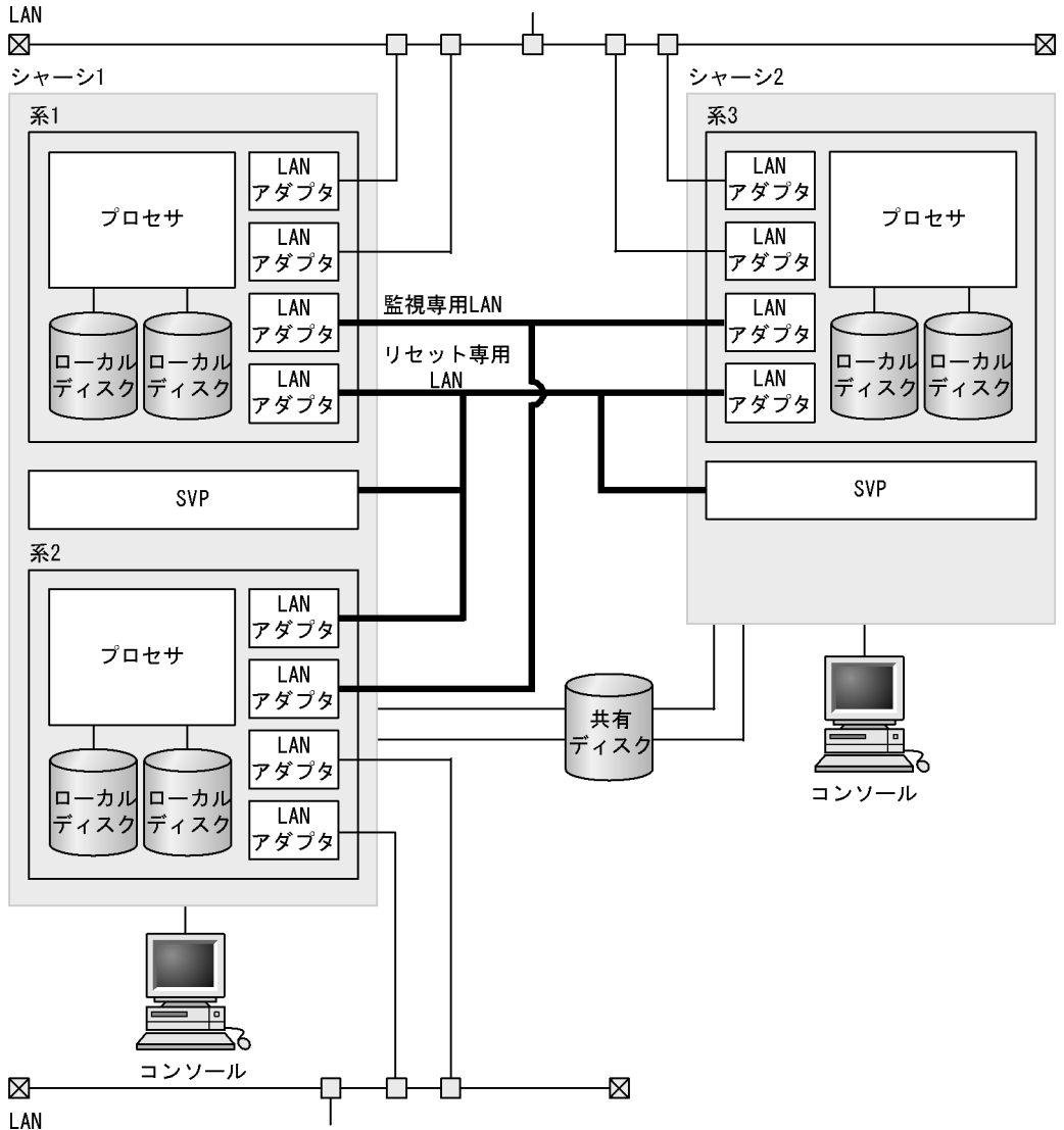
図 5-15 2:1 系切り替え構成時のハードウェア構成例 (BladeSymphony)
