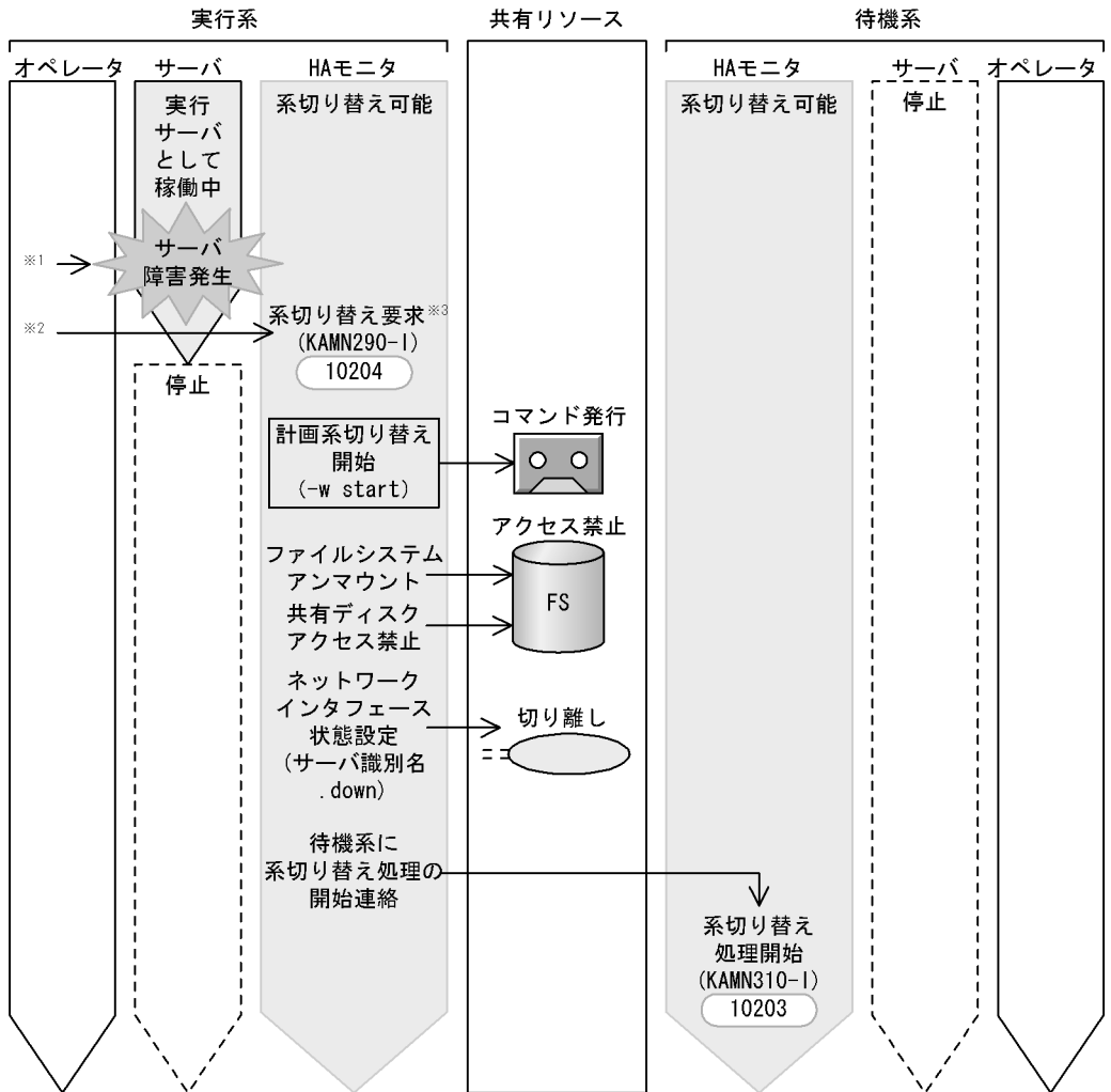
図 4-57 共有リソースの切り離しを接続時と逆順にする場合の、サーバ障害時の系切り替え処理の流れ（共有リソースの切り離しから系切り替え開始まで）（モニターモード）
