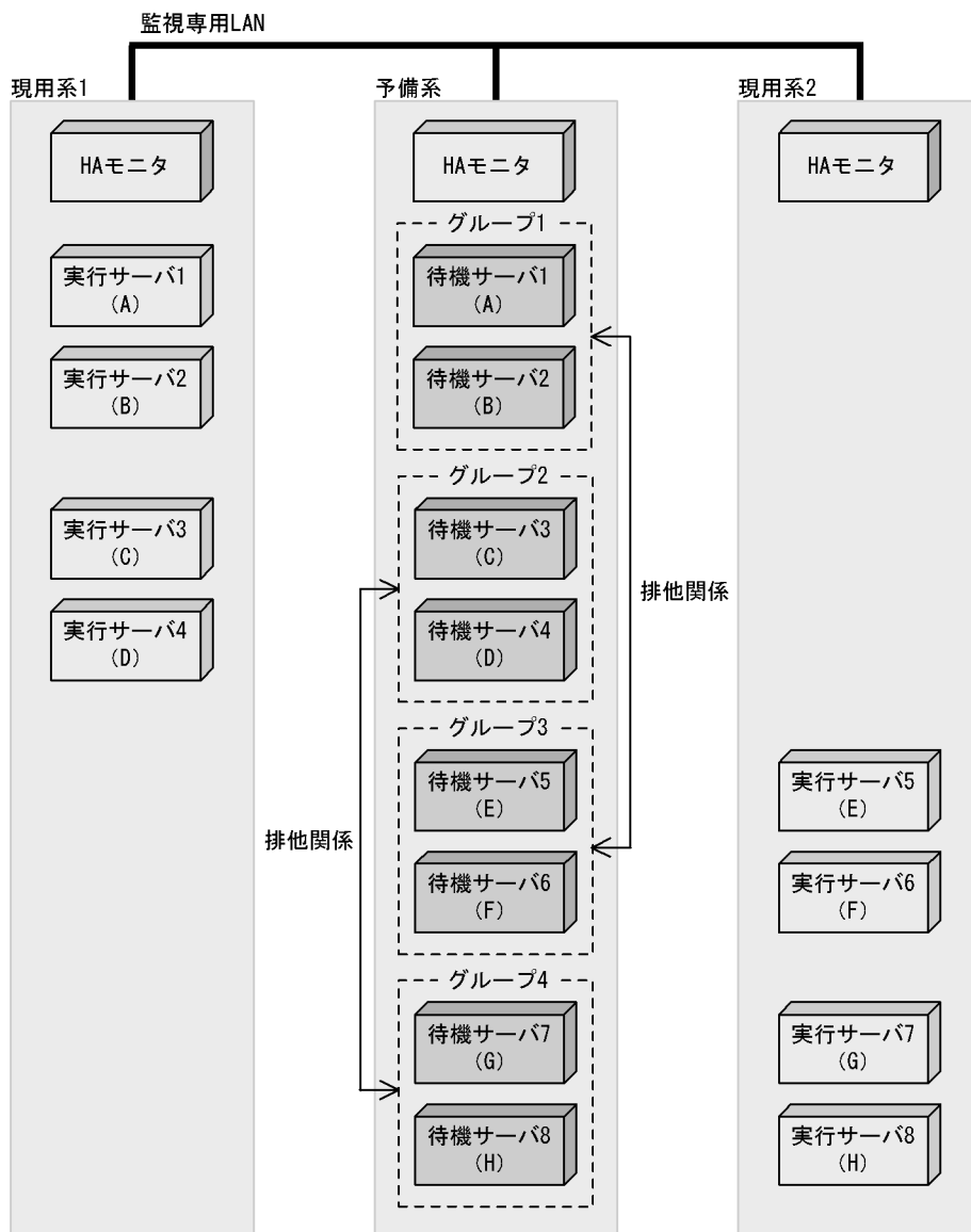
図 8-16 グループ単位に排他関係（複数）にある場合の環境設定の定義例
