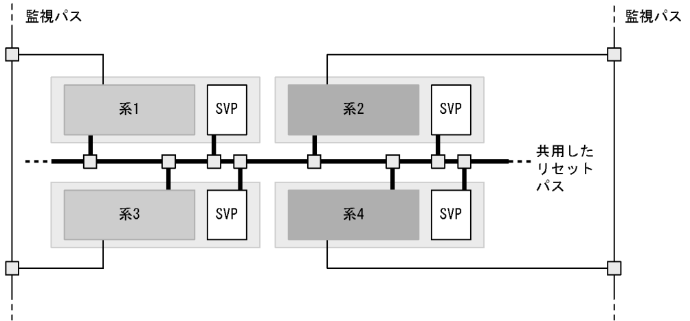
図 5-4 系切り替え構成間でリセットパスを共用したネットワーク構成 (SVP を共用しない場合)
