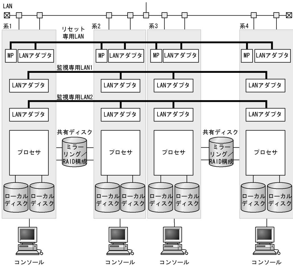
図 5-24 クラスタ型系切り替え構成時のハードウェア構成例 (HA8500)
