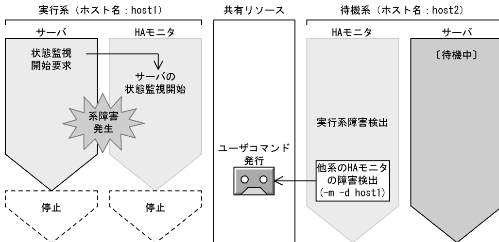
図 6-26 他系の HA モニタ障害検出時に渡されるパラメタと発行タイミング
