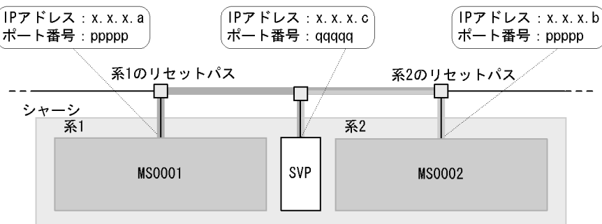
図 6-5 リセットパスの設定例 2 (BladeSymphony)
