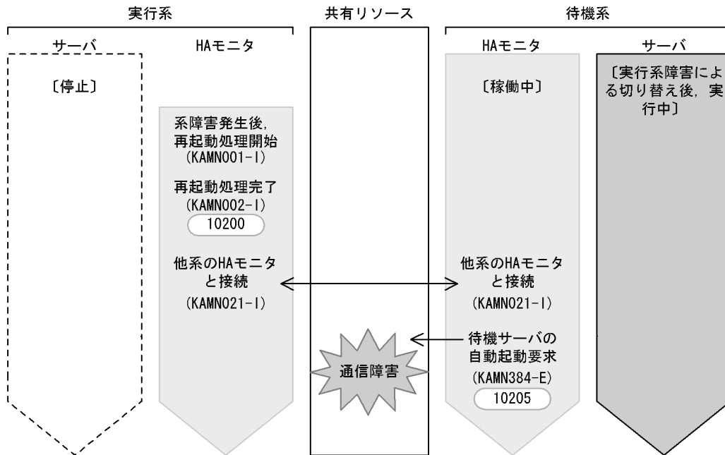
図 A-21 モニタモードのサーバでの待機サーバ自動起動要求失敗時のイベント発行タイミング
