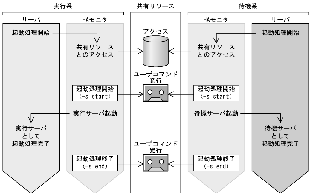
図 6-13 サーバ起動時に渡されるパラメタと発行タイミング
