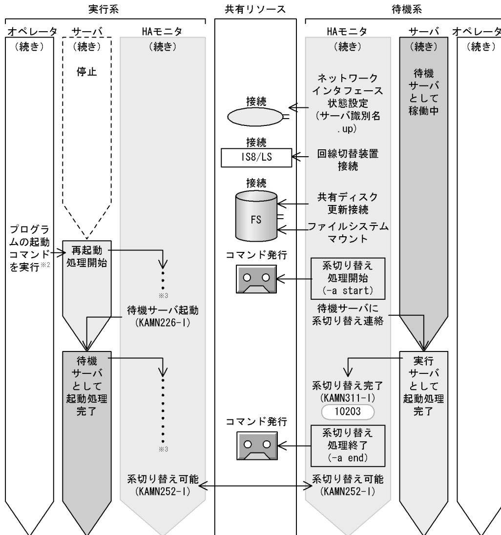
図 4-46 サーバ障害時の系切り替え処理の流れ (共有リソースの接続からサーバの起動まで)(サーバモード)
