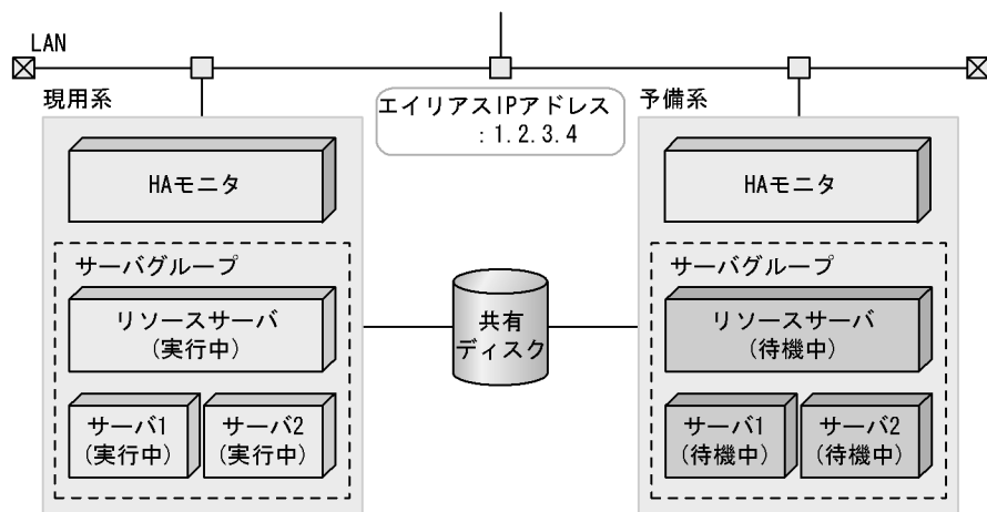
図 3-10 リソースサーバを使用した構成例
