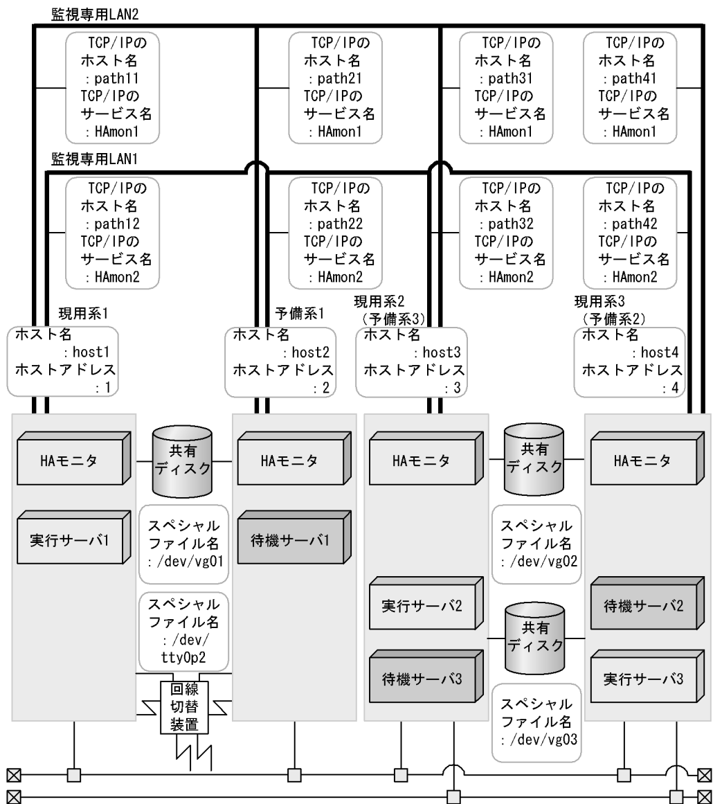
図 8-11 クラスタ型系切り替え構成時のシステム構成
