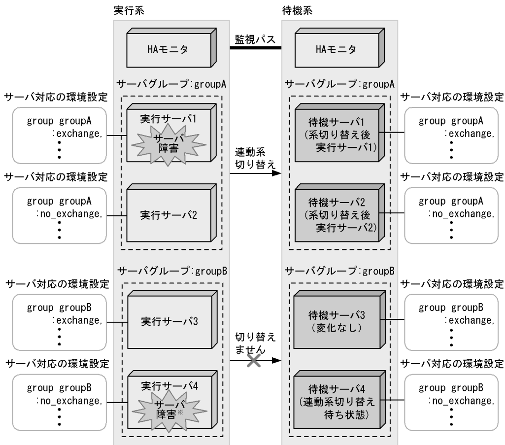
図 4-27 サーバの切り替え種別の指定と連動系切り替えの関係
