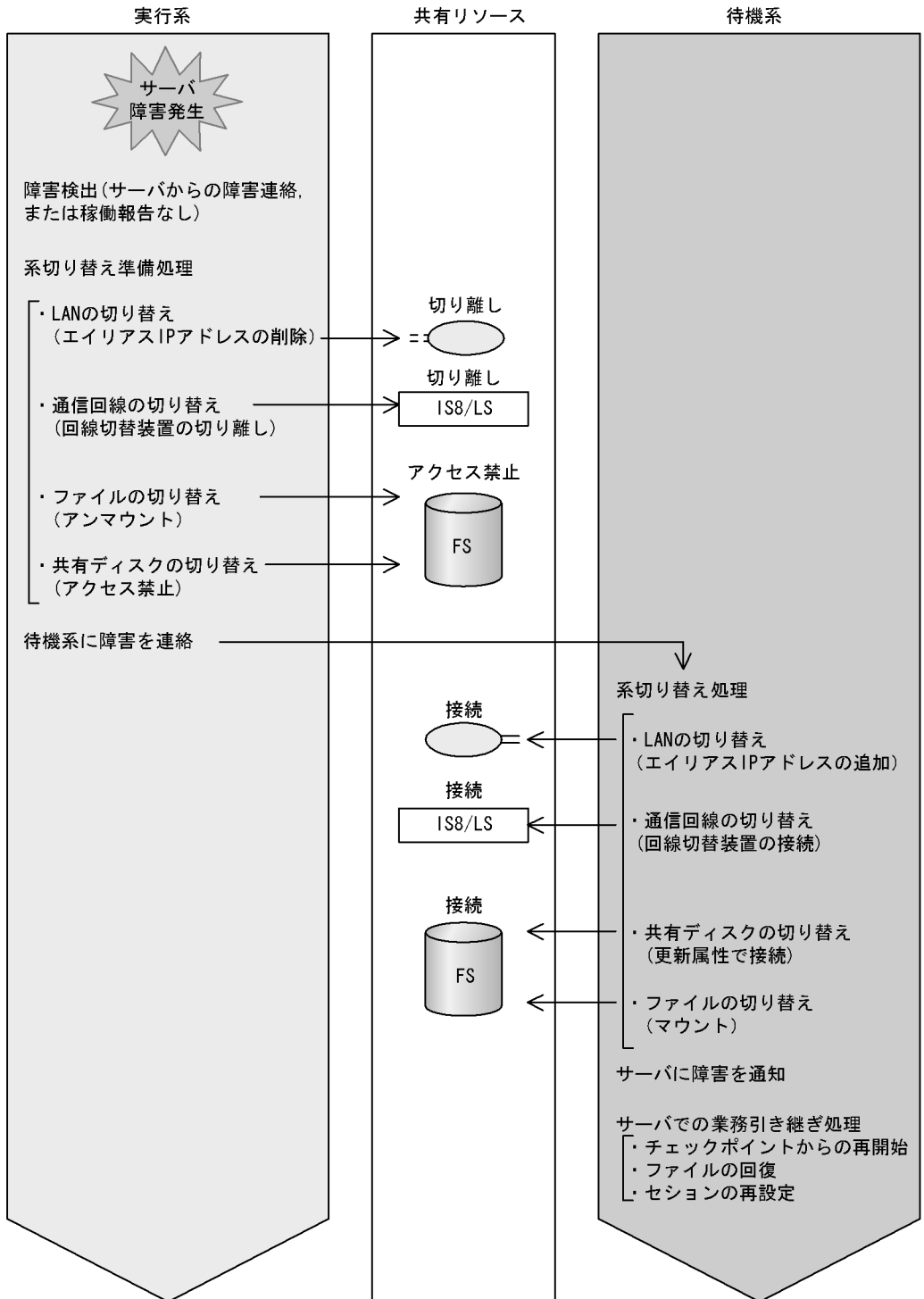
図 2-7 サーバ障害時の系切り替えの概要
