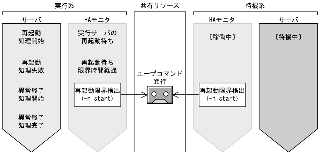
図 6-21 実行サーバの再起動待ち限界時間経過時に渡されるパラメタと発行タイミング
