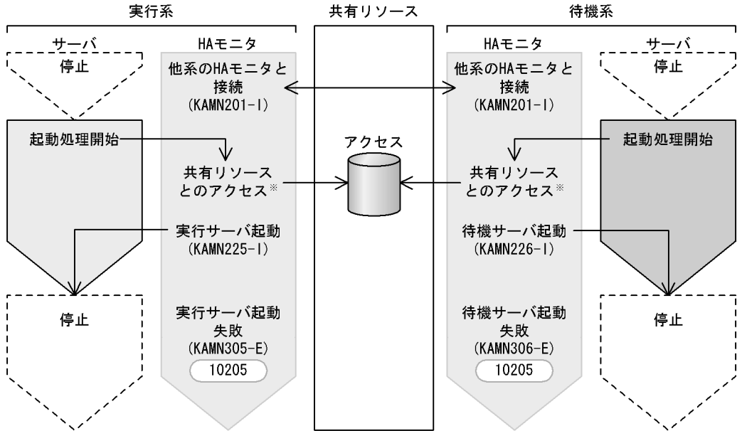
図 A-12 サーバ起動失敗時のイベント発行タイミング
