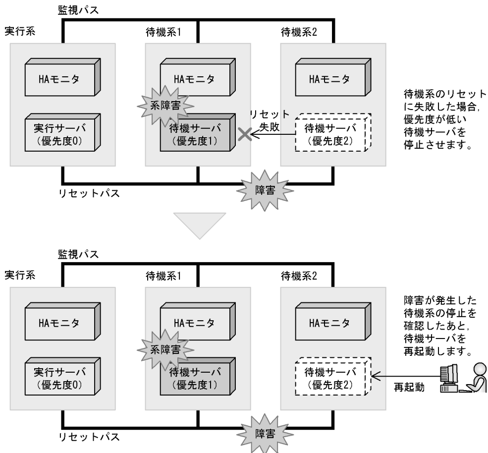
図 4-30 待機系のリセットが失敗した場合の流れ (マルチスタンバイ機能使用時)
