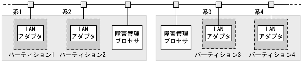
図 5-11 リセット専用 LAN の接続構成（パーティション間で系切り替え構成にする場合）
