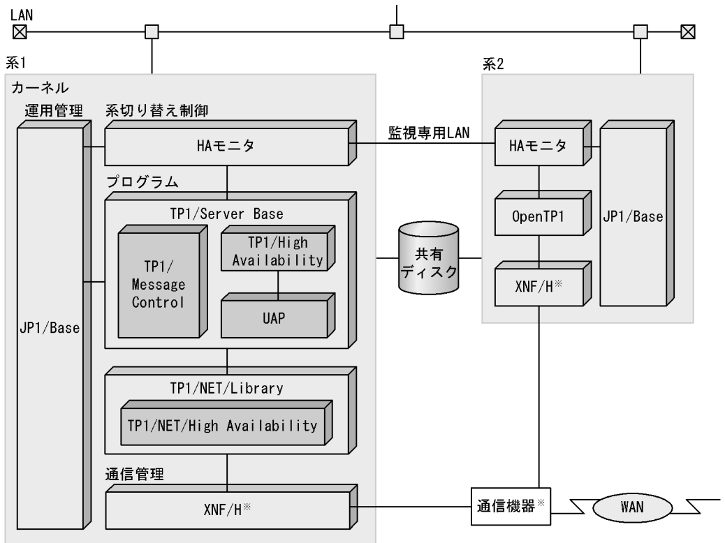
図 1-10 プログラムに OpenTP1 を使用する場合のソフトウェア構成例
