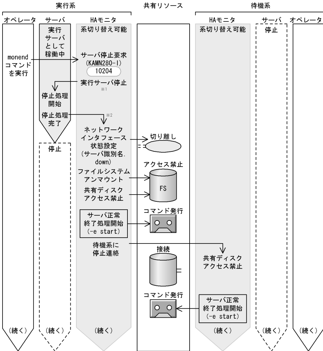
図 4-43 サーバの停止処理の流れ (共有リソースの切り離し)(モニタモード)
