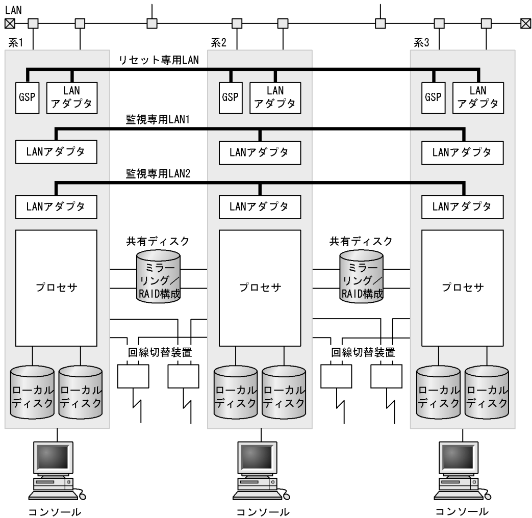
図 5-18 2:1 系切り替え構成時のハードウェア構成例 (H9000V)
