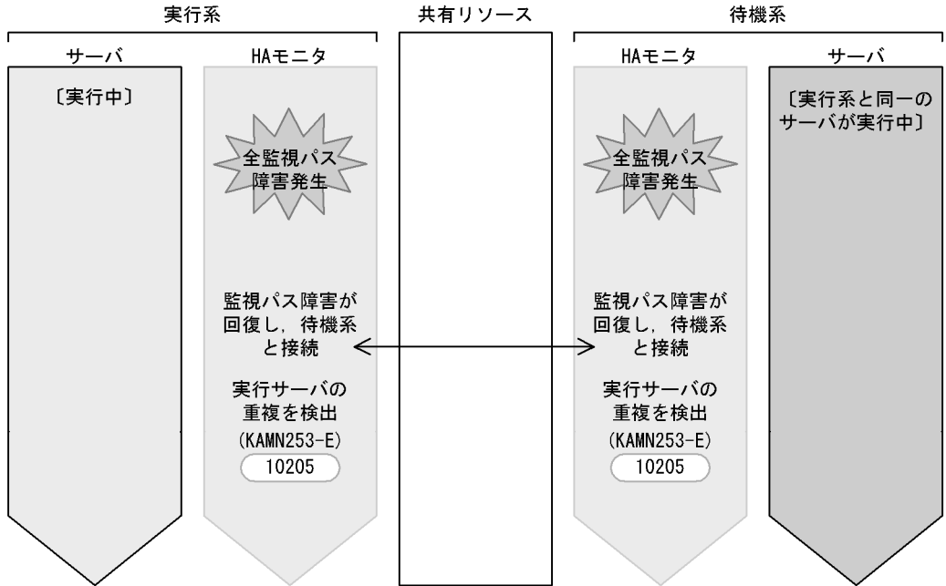
図 A-20 実行サーバ重複起動時のイベント発行タイミング
