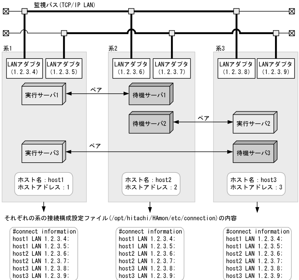
図 6-11 すべての系が互いに監視し合う場合の HA モニタの接続構成設定ファイルの作成例
