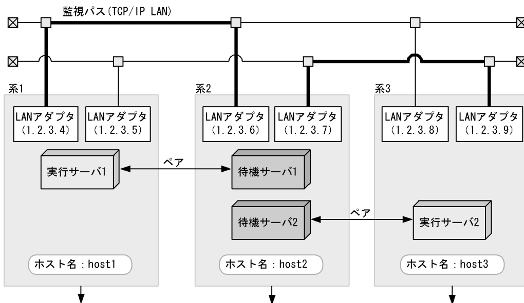
図 6-12 監視し合わない系がある場合の HA モニタの接続構成設定ファイルの作成例
