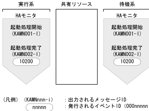
図 A-3 HA モニタ開始時のイベント発行タイミング
