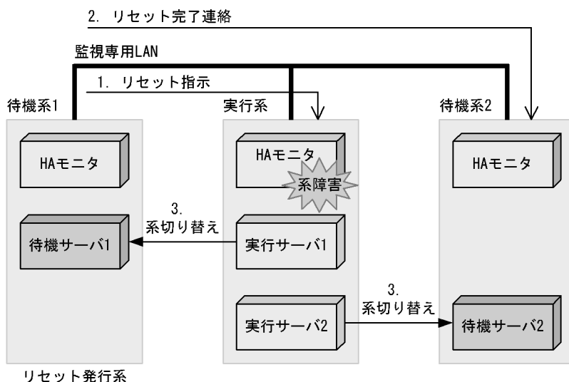
図 4-9 系障害発生時のリセット発行系の動作
