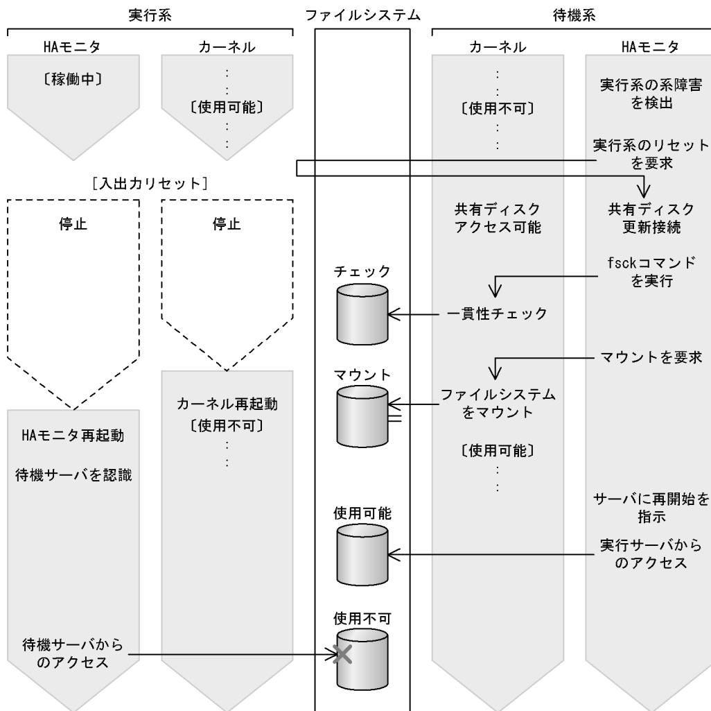
図 4-20 系障害時のファイルシステムの切り替えの流れ
