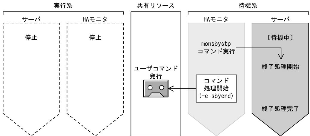
図 6-16 待機サーバ終了時に渡されるパラメタと発行タイミング
