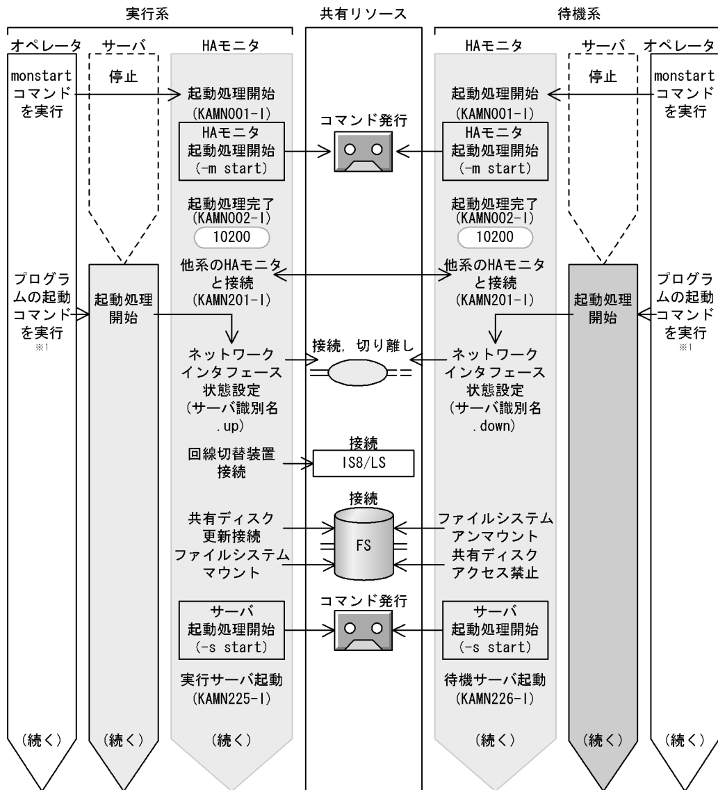
図 4-35 サーバの起動処理の流れ (HA モニタの起動からサーバの起動処理開始まで) (サーバモード)
