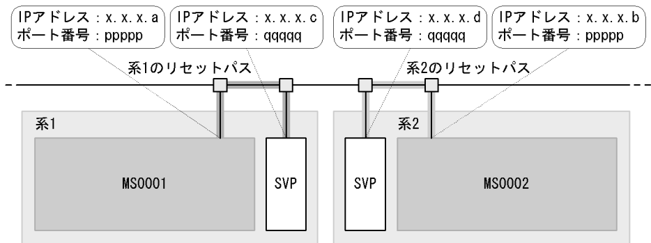
図 6-4 リセットパスの設定例 1 (BladeSymphony)
