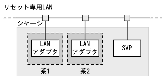
図 5-9 リセット専用 LAN の接続構成（同一シャーシ内での 1:1 系切り替え構成の場合） （BladeSymphony）
