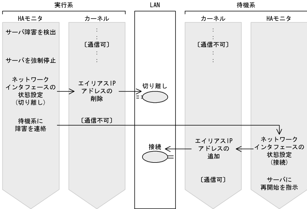
図 4-22 サーバ障害時の LAN の切り替えの流れ
