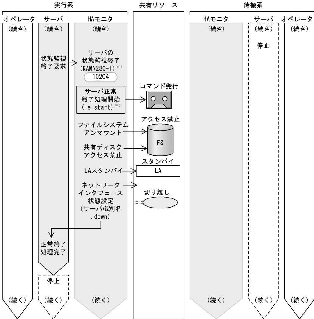
図 4-54 共有リソースの切り離しを接続時と逆順にする場合の、サーバの停止処理の流れ（サーバの状態監視終了から HA モニタの停止まで）（サーバモード：実行サーバの停止処理開始時に待機サーバを停止する）
