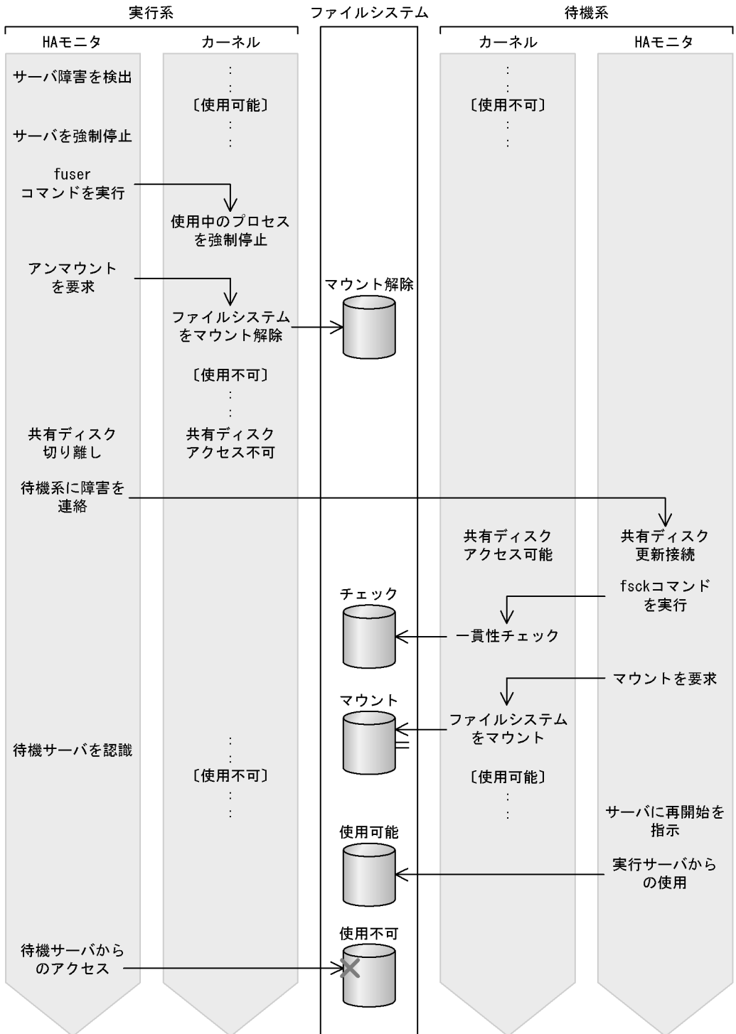
図 4-19 サーバ障害時のファイルシステムの切り替えの流れ
