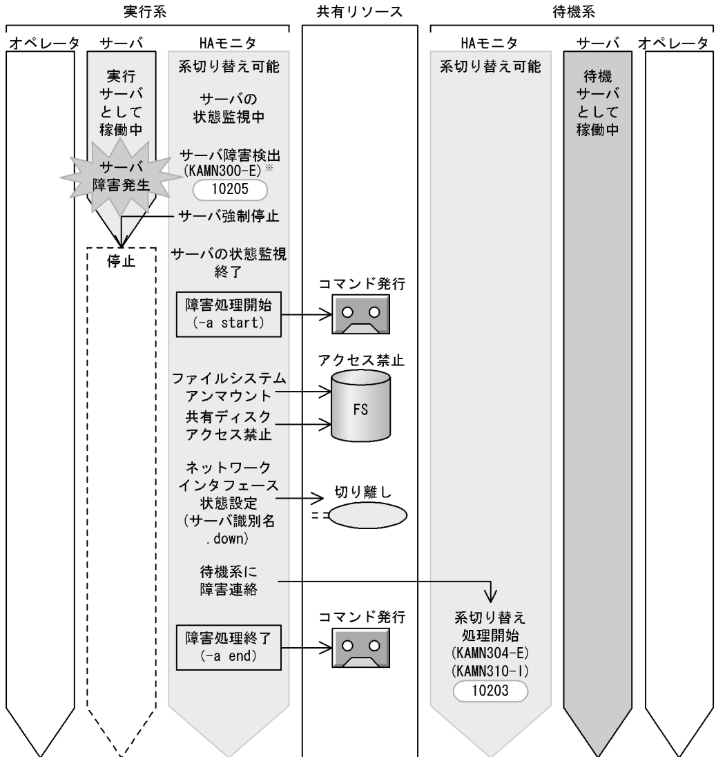
図 4-56 共有リソースの切り離しを接続時と逆順にする場合の、サーバ障害時の系切り替え処理の流れ（サーバ障害の検出から系切り替え開始まで）（サーバモード）
