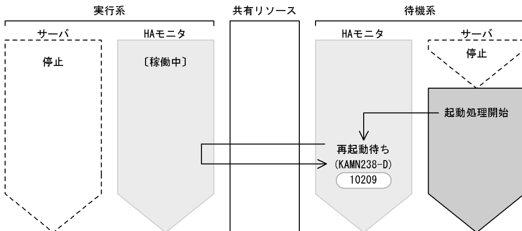
図 A-28 実行サーバ未起動によるオペレータ介入待ち時のイベント発行タイミング
