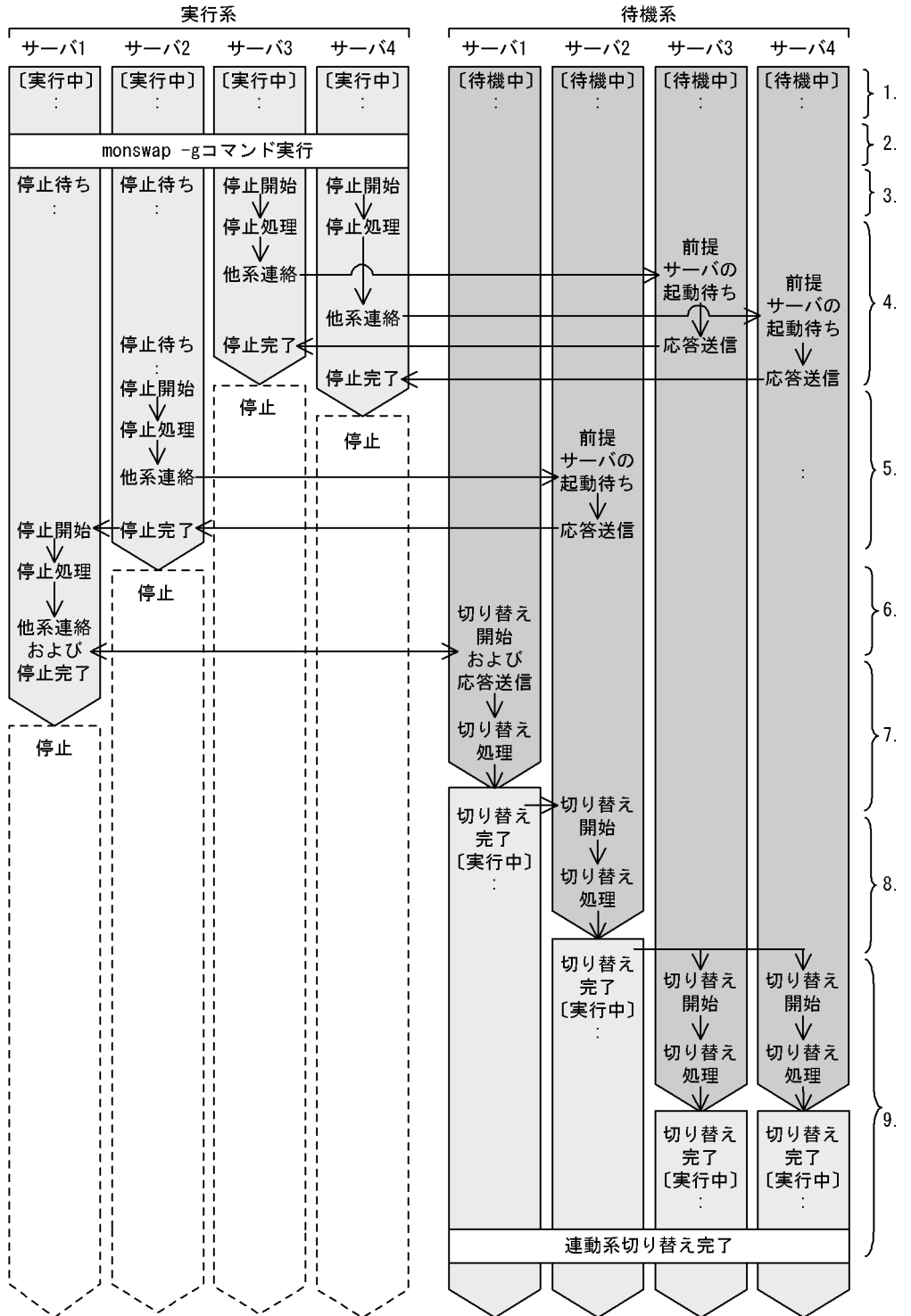
図 4-4 計画系切り替え時の順序制御の流れ
