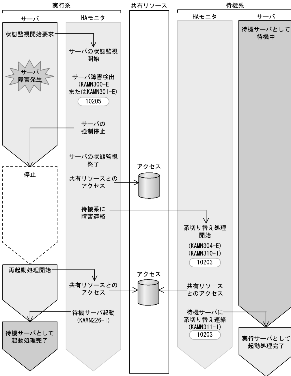
図 A-13 サーバ障害時 (switchtype = switch) のイベント発行タイミング
