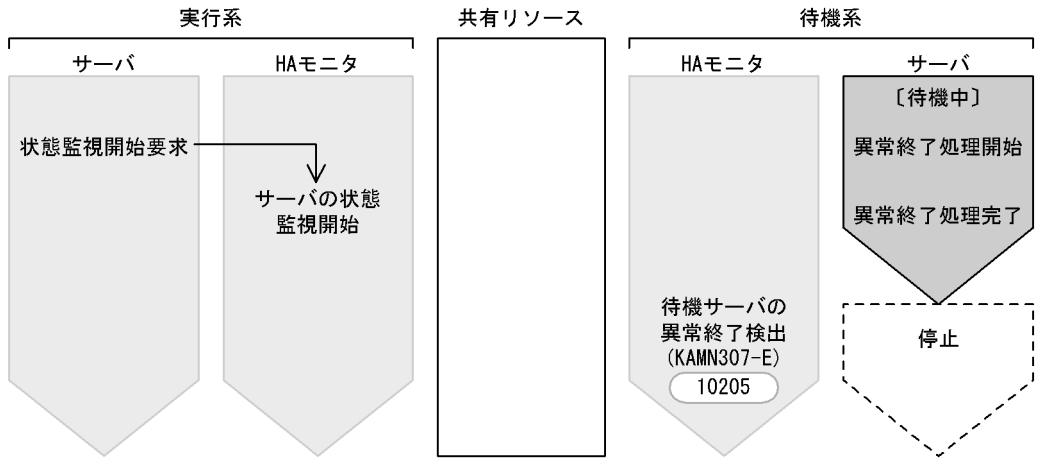
図 A-18 待機サーバ異常終了時のイベント発行タイミング
