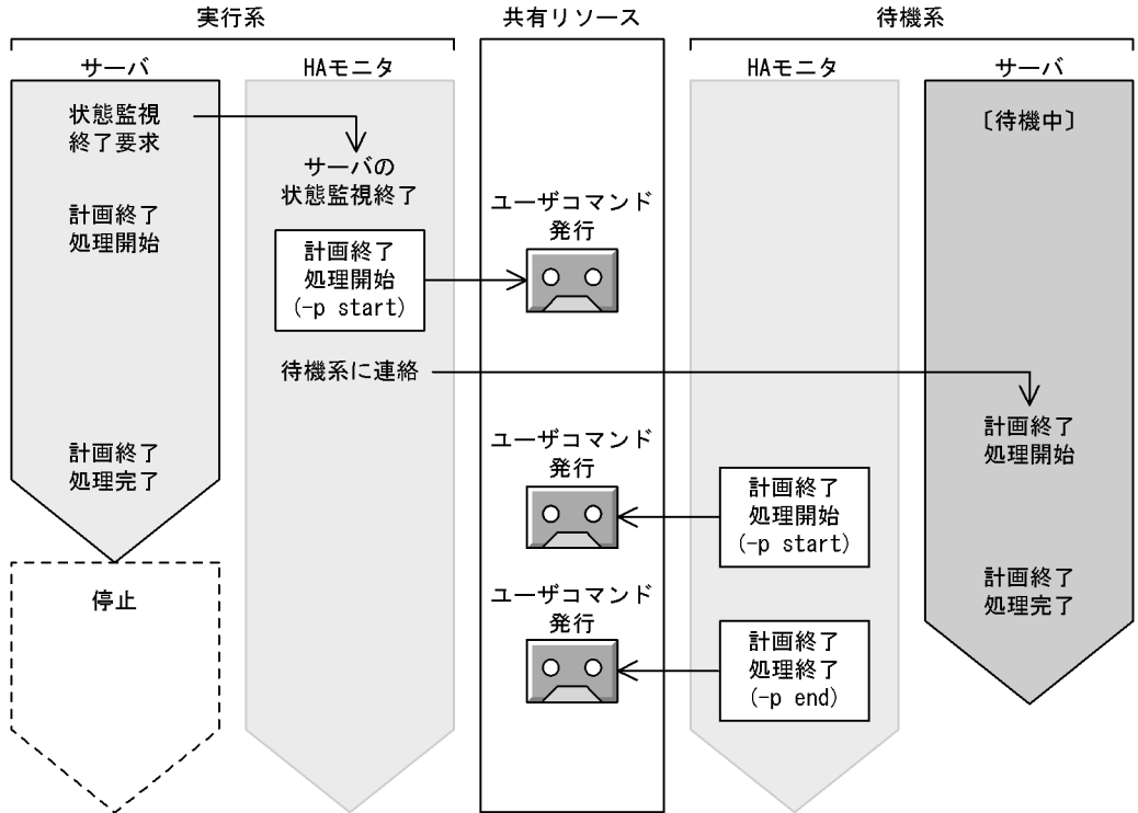
図 6-15 サーバ計画終了時に渡されるパラメタと発行タイミング
