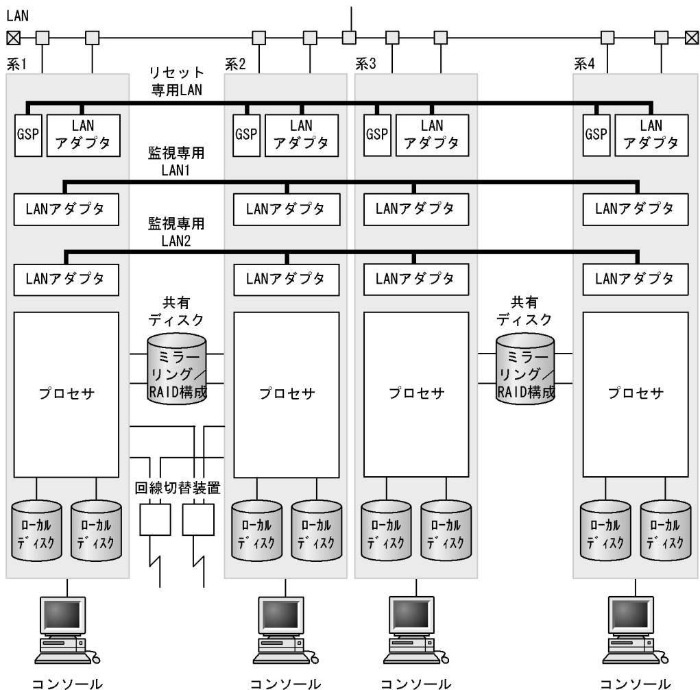
図 5-20 クラスタ型系切り替え構成時のハードウェア構成例 (H9000V)
