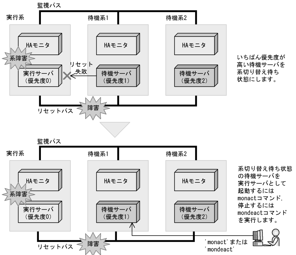
図 4-29 実行系のリセットが失敗した場合の流れ（マルチスタンバイ機能使用時）
