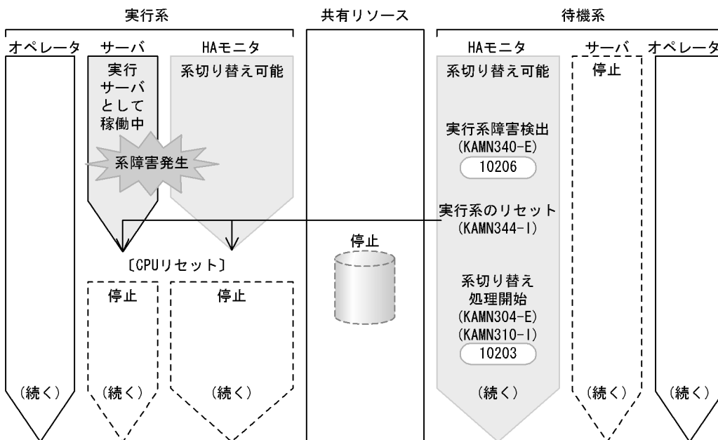
図 4-51 系障害時の系切り替えの流れ (系障害の検出からサーバの起動まで)(モニタモード)
