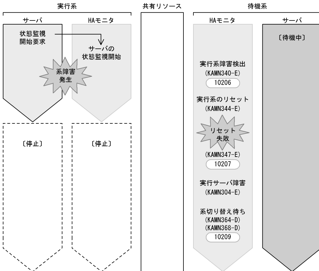
図 A-25 系のリセット失敗時のイベント発行タイミング
