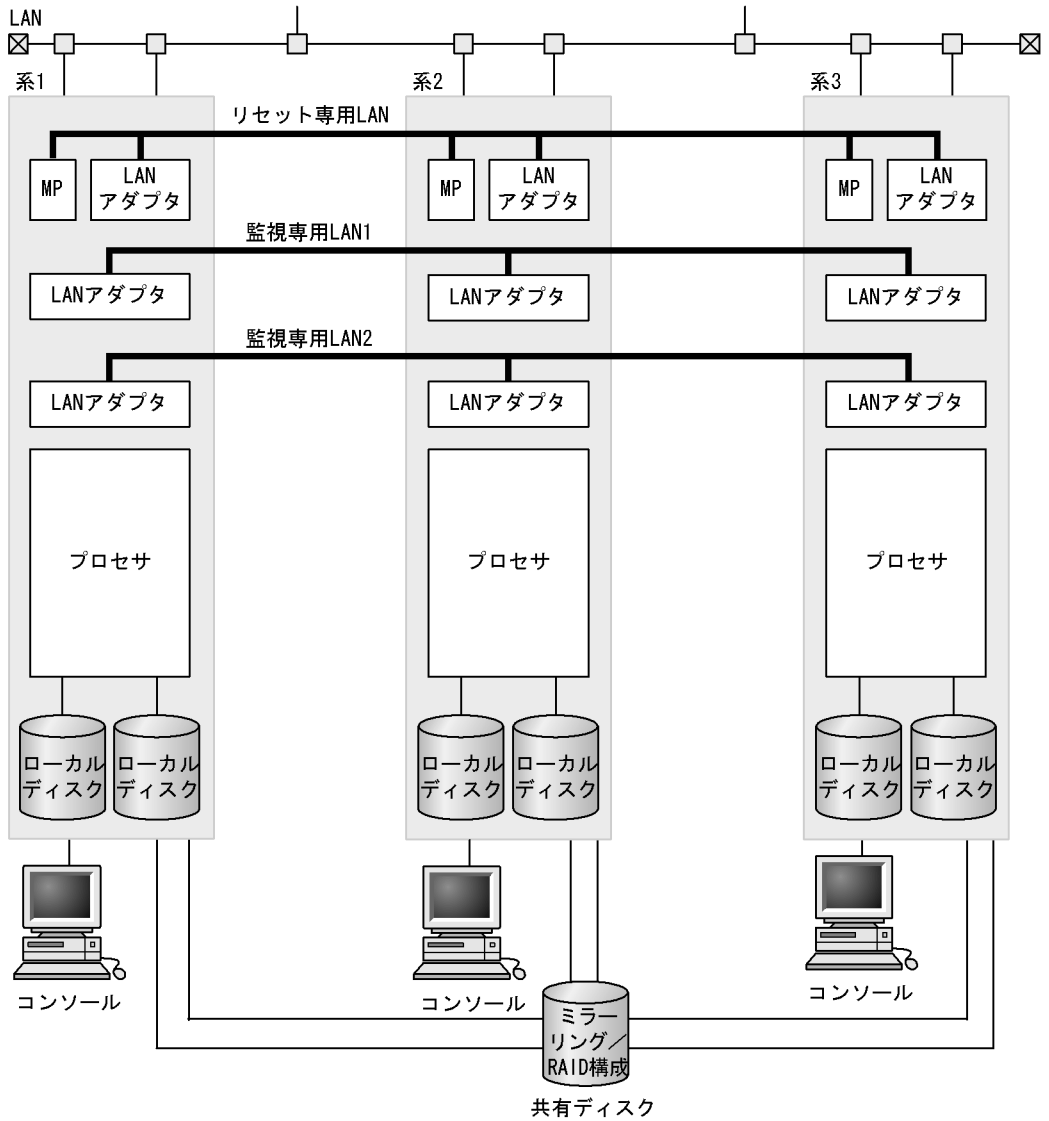
図 5-23 複数スタンバイ構成時のハードウェア構成例 (HA8500)
