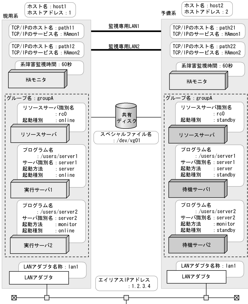
図 8-8 複数サーバで共有リソースを共用する場合のシステム構成
