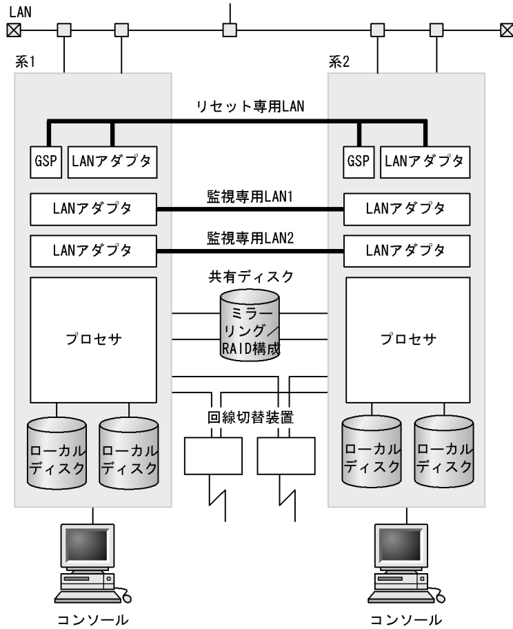
図 5-17 1:1 系切り替え構成時のハードウェア構成例 (H9000V)
