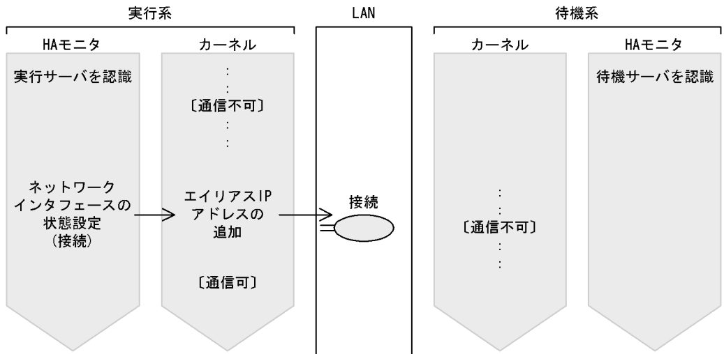
図 4-21 LAN との接続の流れ
