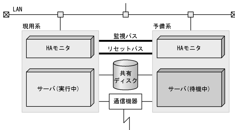
図 2-1 1:1 系切り替え構成例
