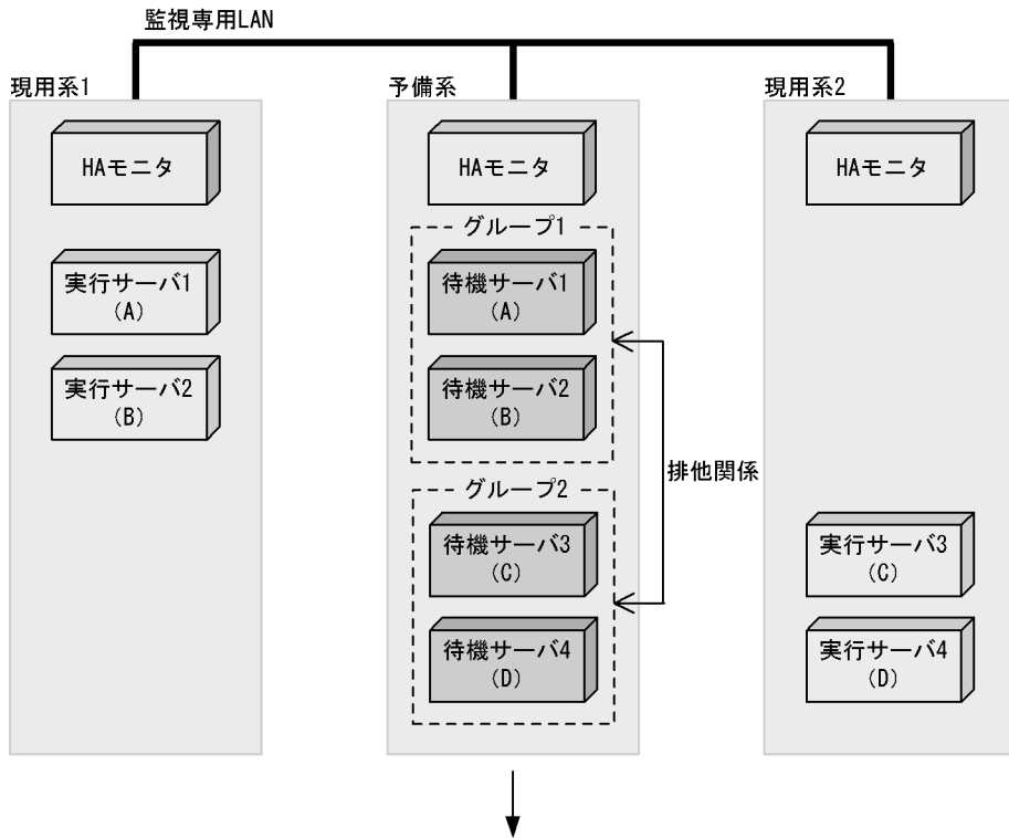
図 8-13 グループ単位に排他関係にある場合の環境設定の定義例
