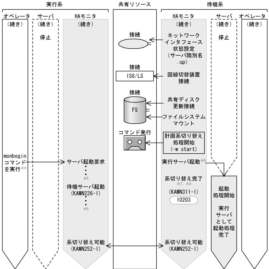
図 4-48 サーバ障害時の系切り替え処理の流れ（共有リソースの接続からサーバの起動まで）(モニターモード)
