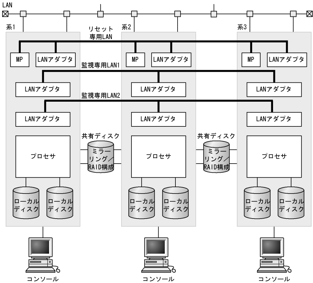
図 5-22 2:1 系切り替え構成時のハードウェア構成例 (HA8500)
