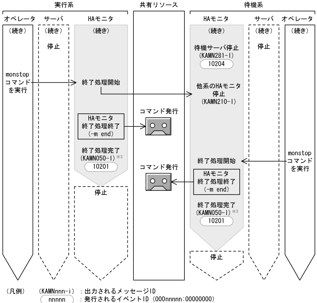
図 4-44 サーバの停止処理の流れ (待機サーバの停止から HA モニタの停止まで) (モニタモード)
