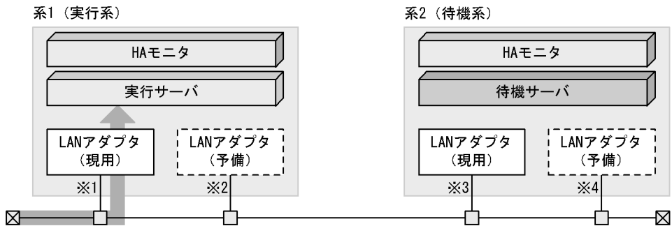
図 3-12 LAN アダプタを二重化した場合の構成
