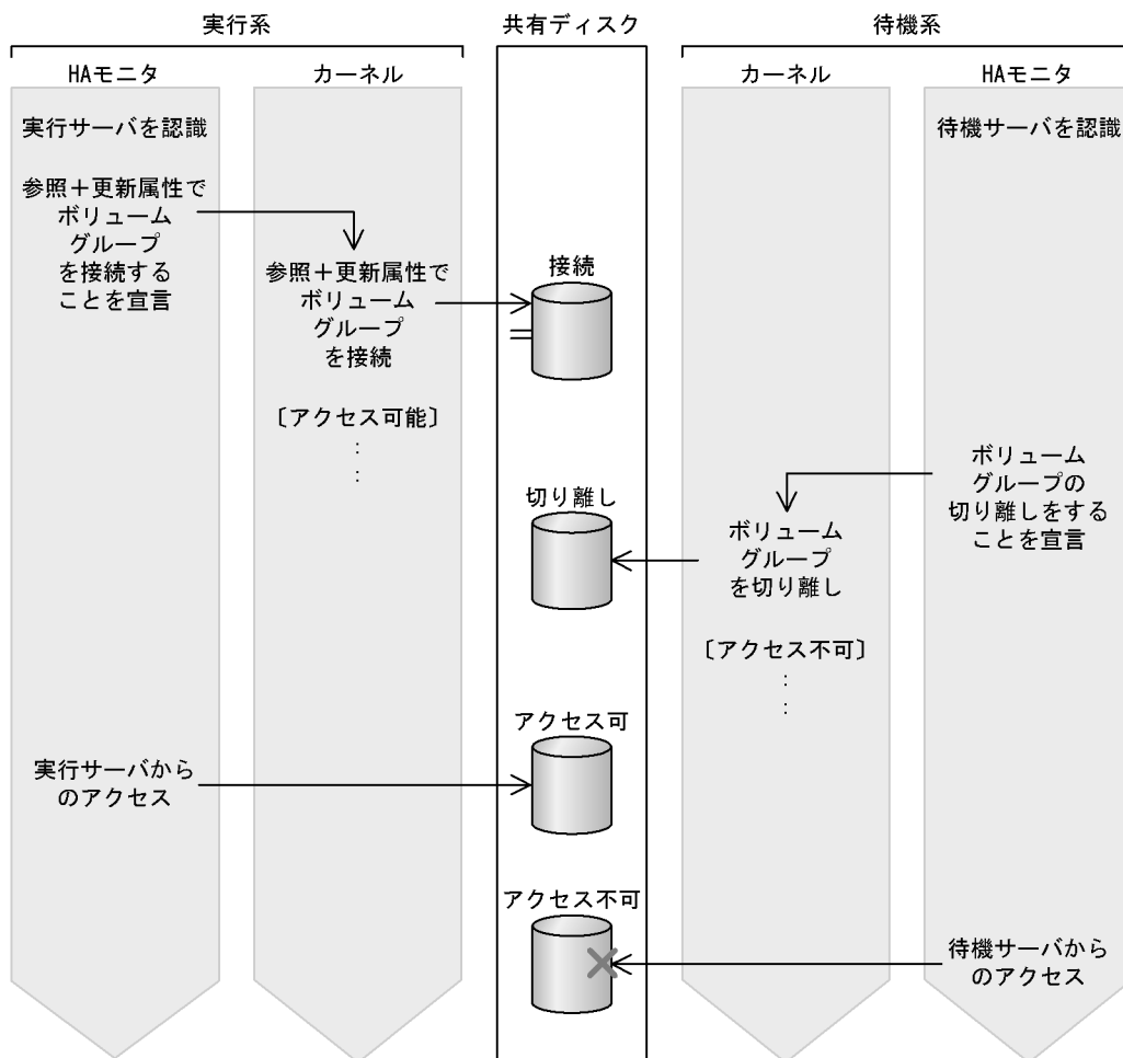
図 4-15 共有ディスクとの接続の流れ
