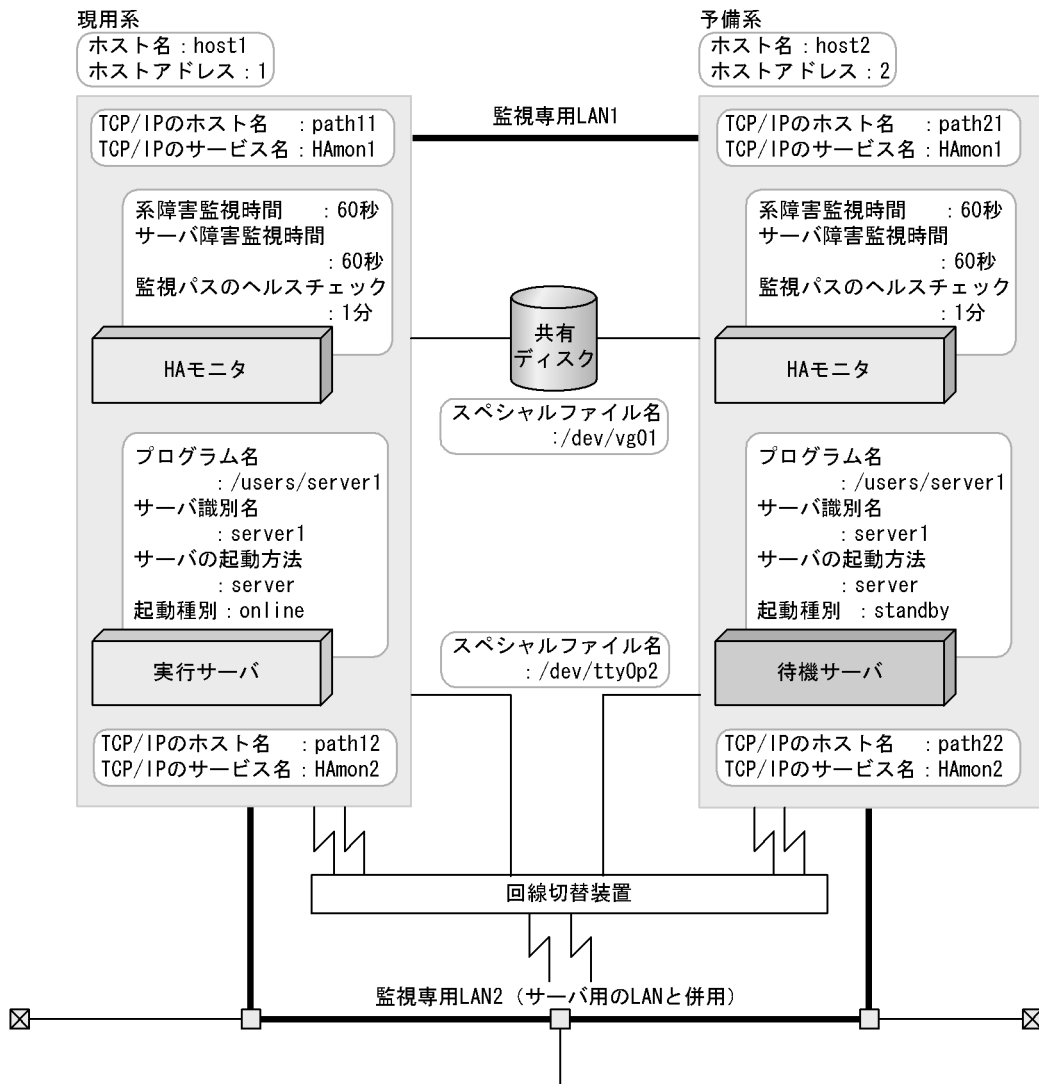
図 8-1 HN-7601-8V または HN-7601-8X の回線切替装置使用時のシステム構成 (H9000V)
