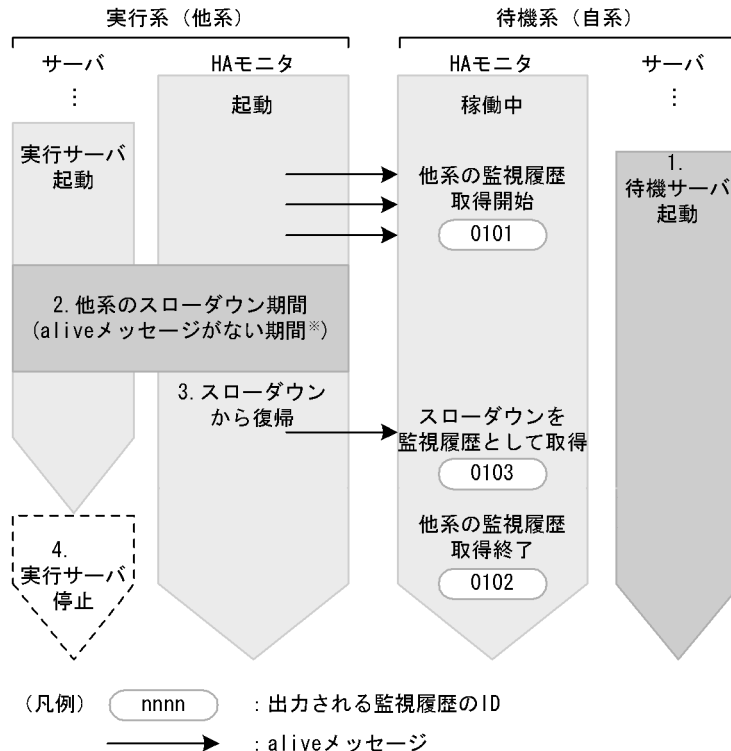
図 B-2 他系の監視履歴が出力されるタイミング
