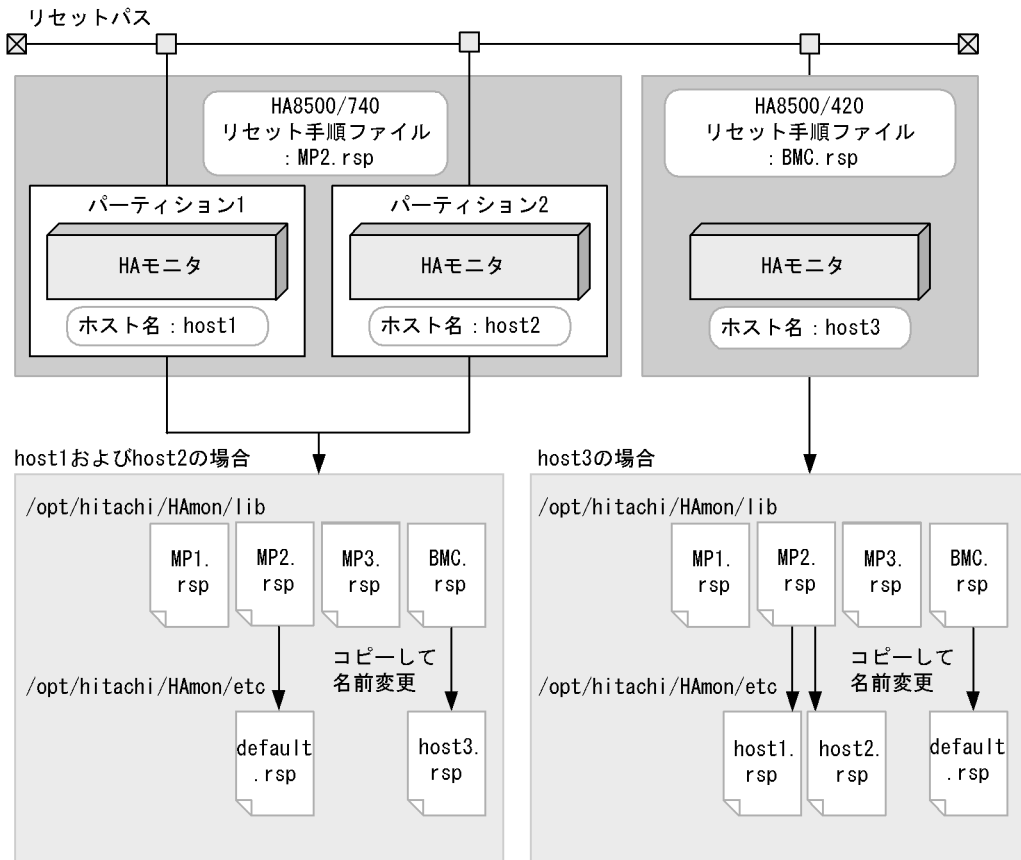
図 6-9 リセット手順ファイルの作成例 (HA8500)
