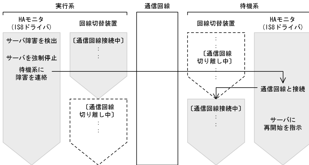
図 4-25 サーバ障害時の、回線切替装置を使用した通信回線の切り替えの流れ (H9000V)
