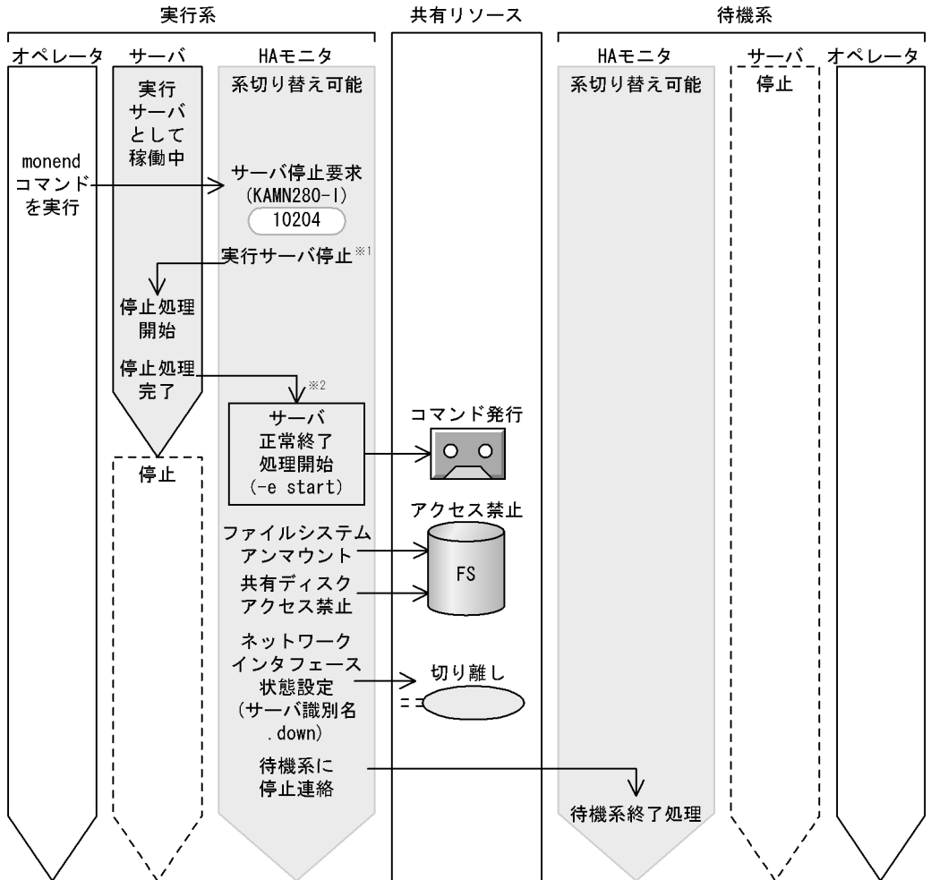
図 4-55 共有リソースの切り離しを接続時と逆順にする場合の、サーバの停止処理の流れ (共有リソースの切り離し) (モニタモード)
