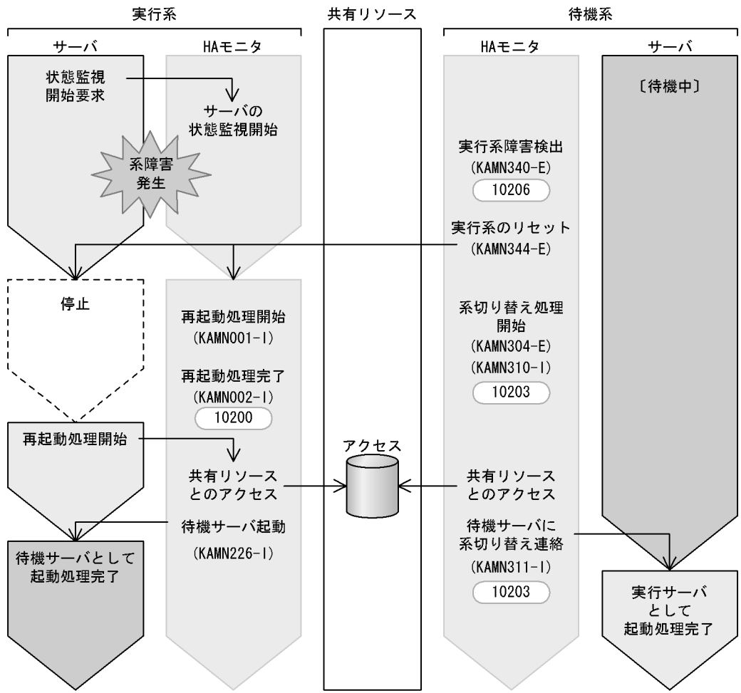
図 A-23 系障害時のイベント発行タイミング
