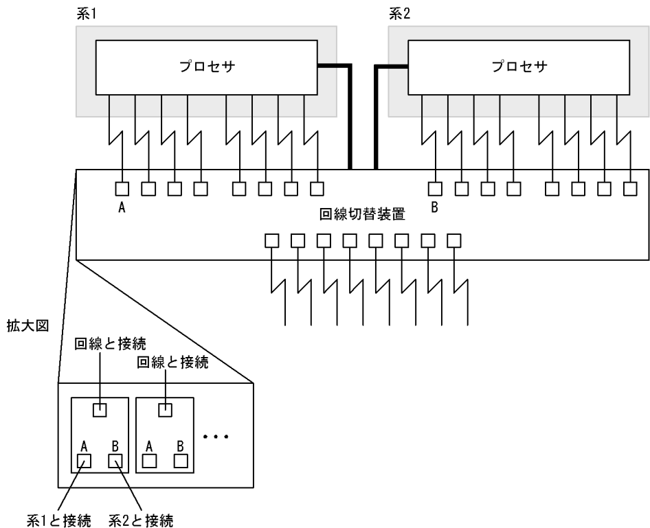
図 5-12 回線切替装置を使用した通信回線との接続例
