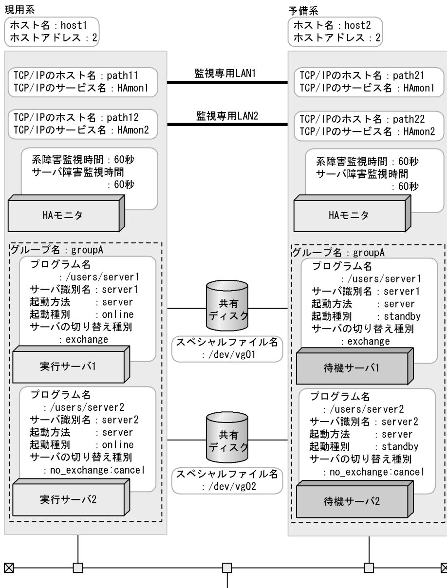
図 8-3 サーバをグループ化する場合のシステム構成
