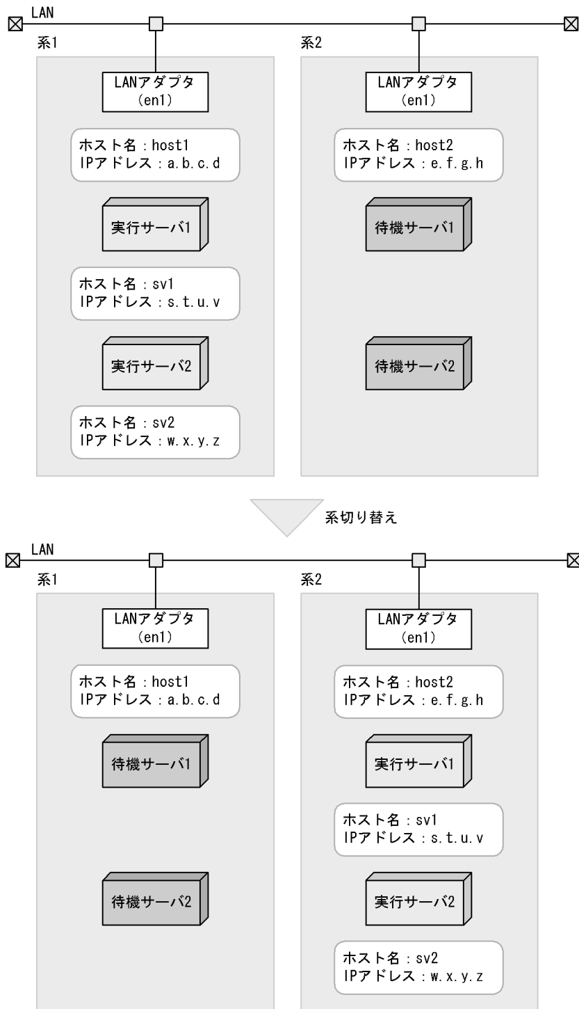
図 2-11 エイリアス IP アドレスの引き継ぎ例
