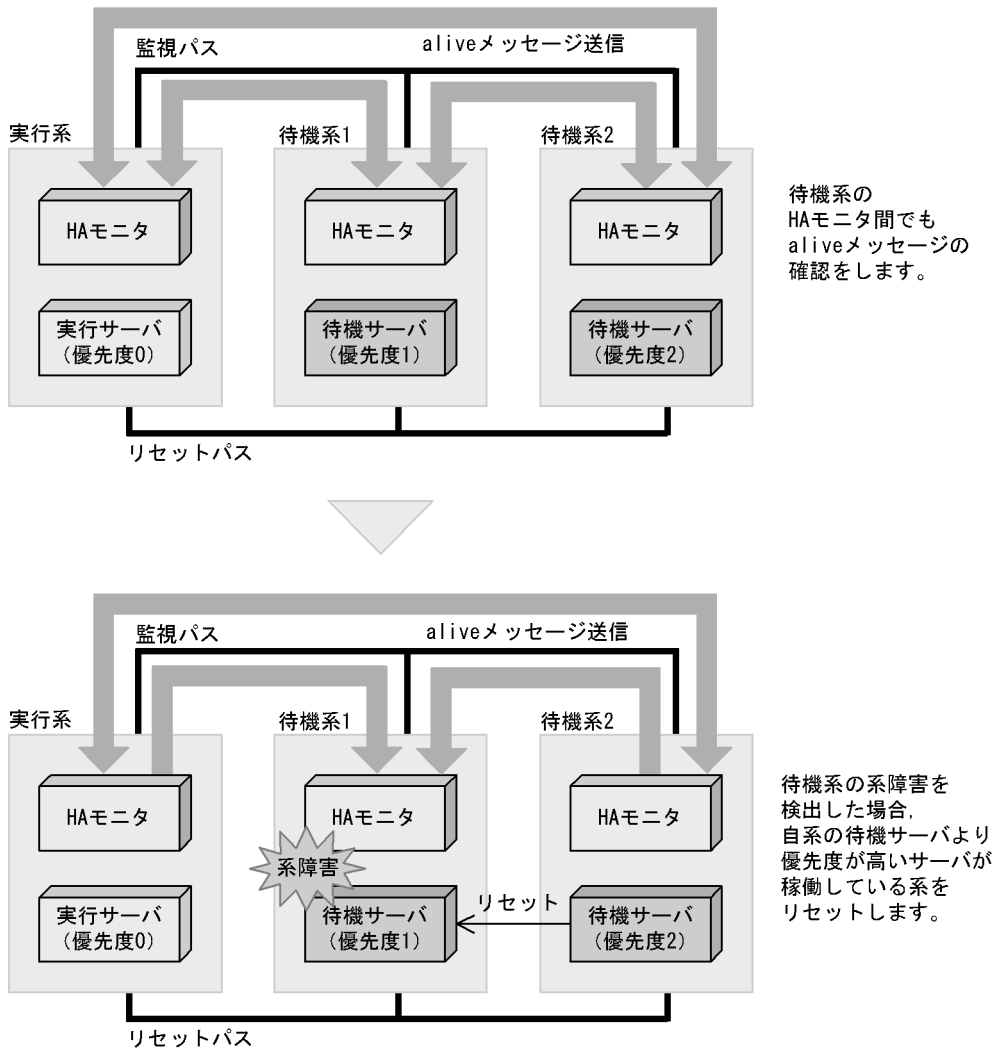
図 4-28 系の状態監視と系のリセット（マルチスタンバイ機能使用時）
