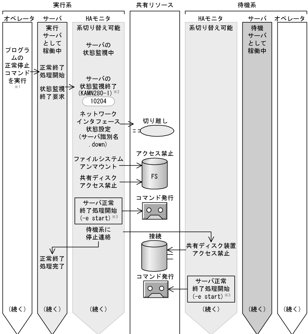
図 4-39 サーバの停止処理の流れ (サーバの状態監視終了から共有リソースの切り離しまで) (サーバモード: 実行サーバの停止処理終了時に待機サーバを停止する)
