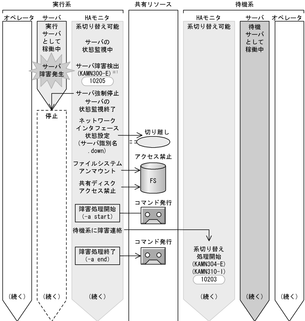
図 4-45 サーバ障害時の系切り替え処理の流れ (サーバ障害の検出から系切り替え開始まで)(サーバモード)
