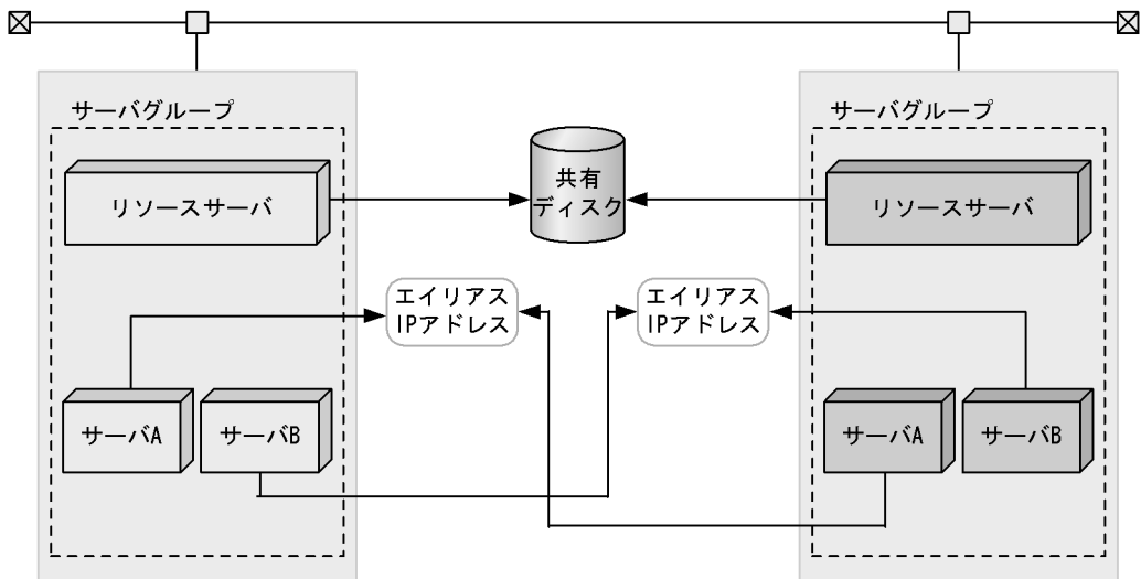
図 5-6 複数の共有リソースのうち一つを共用し、残りはサーバ単位で使用する構成
