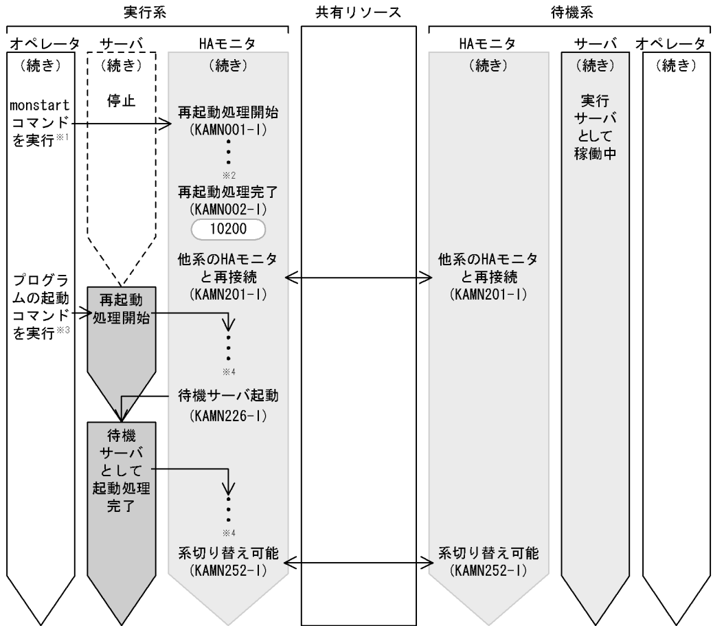
図 4-50 系障害時の系切り替えの流れ(系の再起動)(サーバモード)
