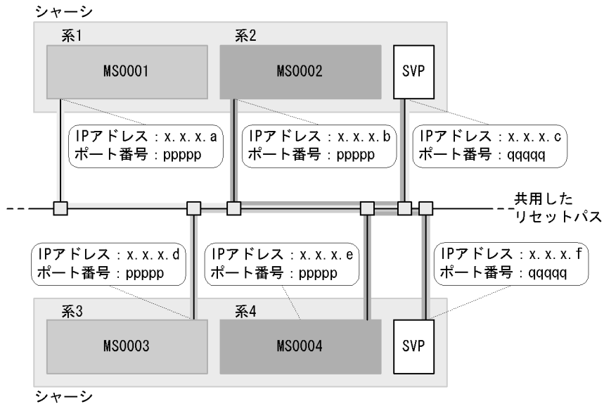
図 6-6 リセットパスの設定例 3 (BladeSymphony)
