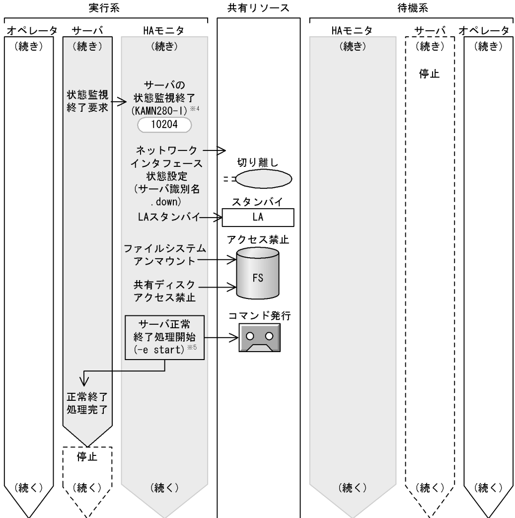
図 4-42 サーバの停止処理の流れ (サーバの状態監視終了から HA モニタの停止まで) (サーバモード：実行サーバの停止処理開始時に待機サーバを停止する)
