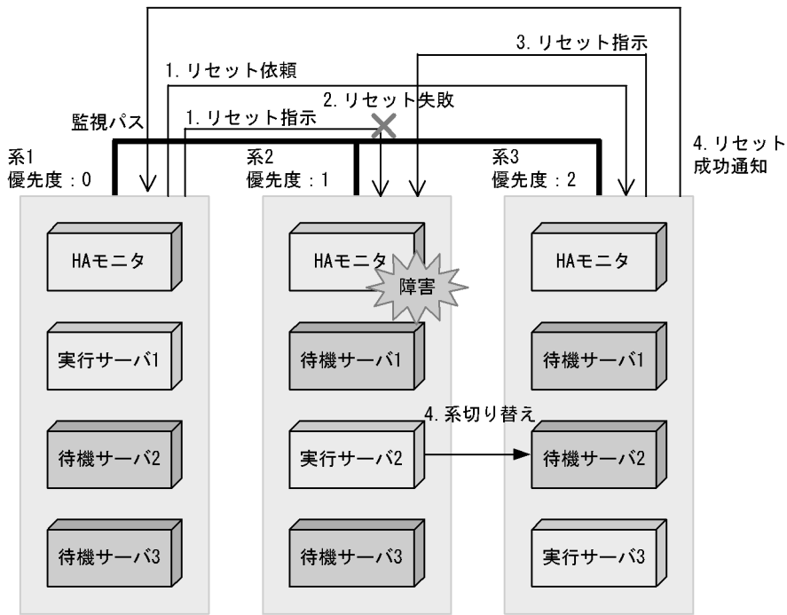
図 4-13 複数の待機系がある系切り替え構成で、系のリセットが失敗した場合の系のリセット
