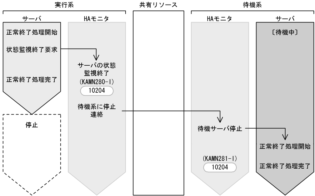
図 A-10 サーバ正常終了時のイベント発行タイミング
