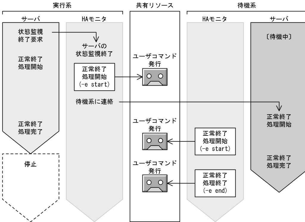
図 6-14 サーバ正常終了時に渡されるパラメタと発行タイミング
