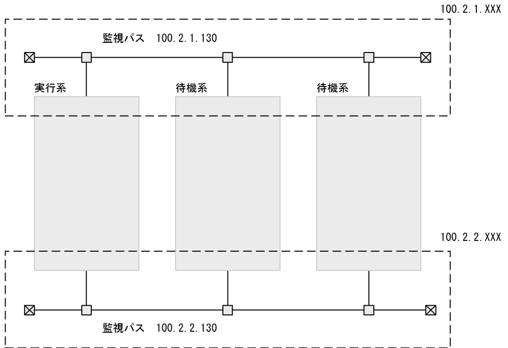
図 5-2 監視パスを複線化したネットワーク構成
