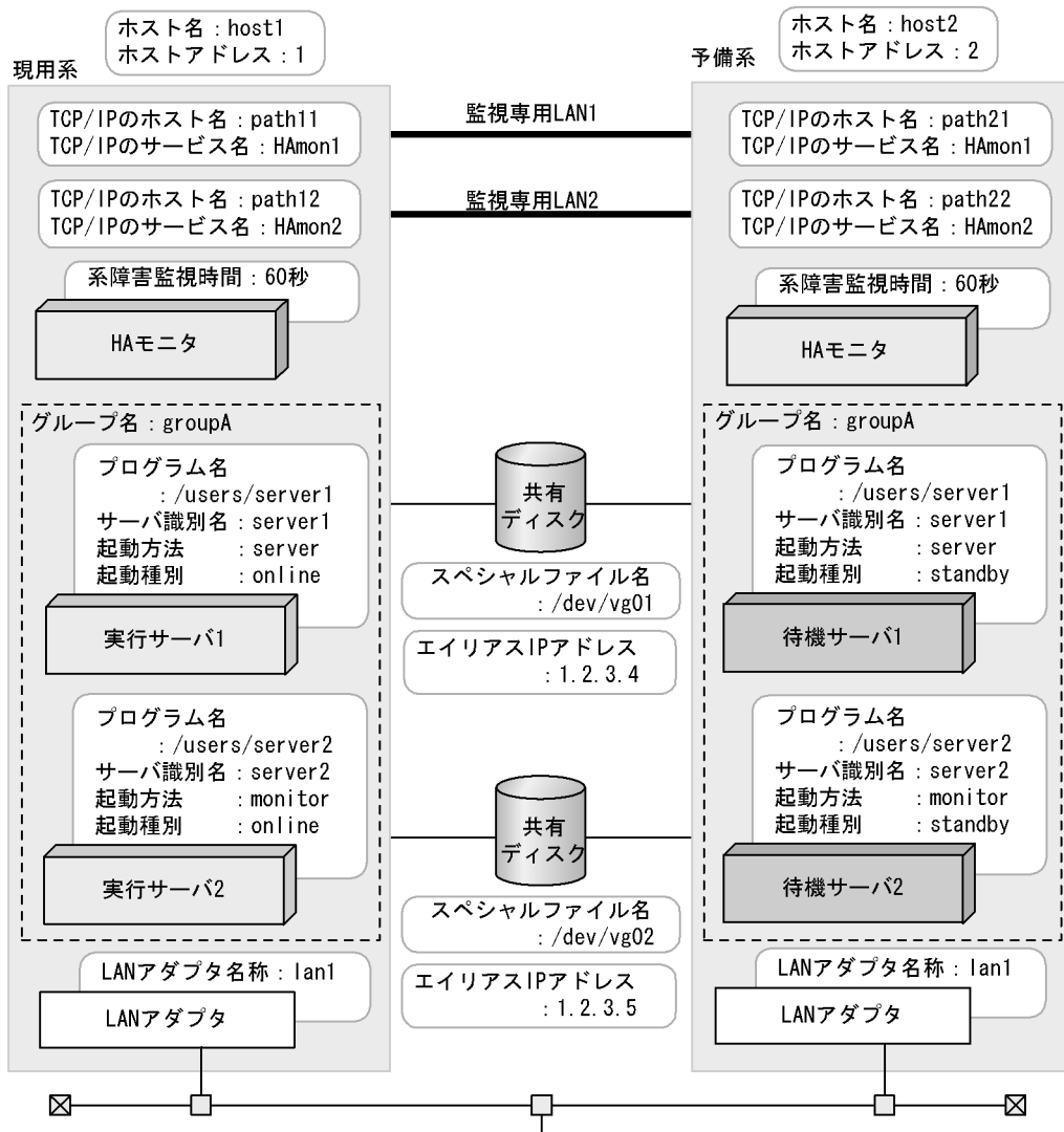
図 8-7 サーバの切り替え順序を制御する場合のシステム構成
