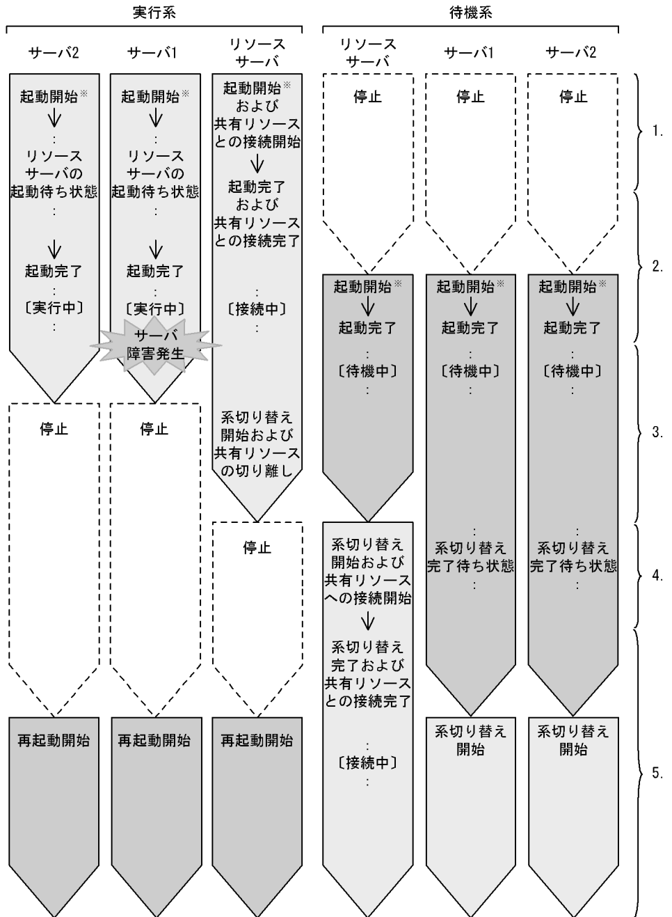
図 4-33 共有リソースとの接続および切り離しの流れ（リソースサーバ使用時）
