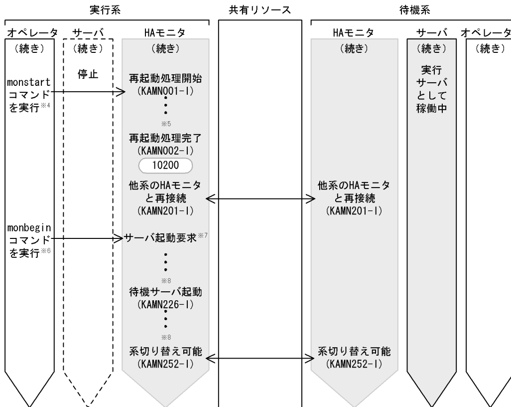
図 4-52 系障害時の系切り替えの流れ (系の再起動)(モニタモード)
