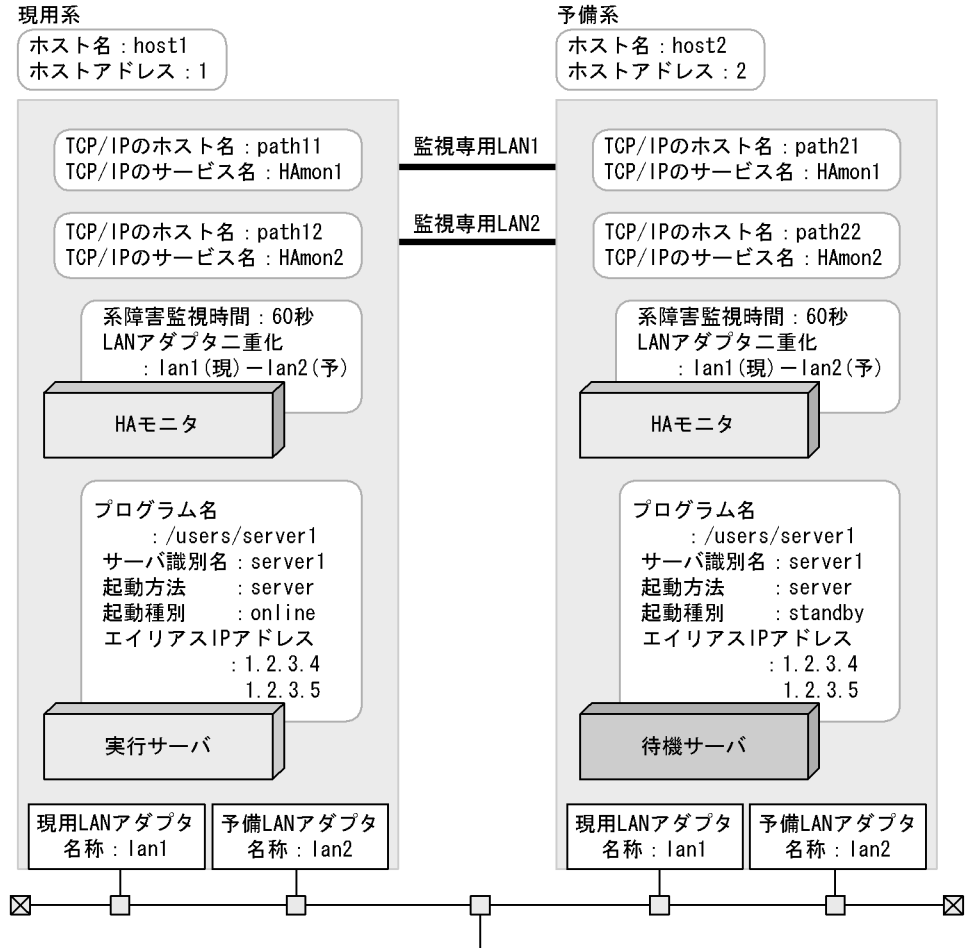
図 8-5 LAN アダプタ二重化時のシステム構成
