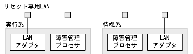
図 5-8 リセット専用 LAN の接続構成（1:1 系切り替え構成の場合）
