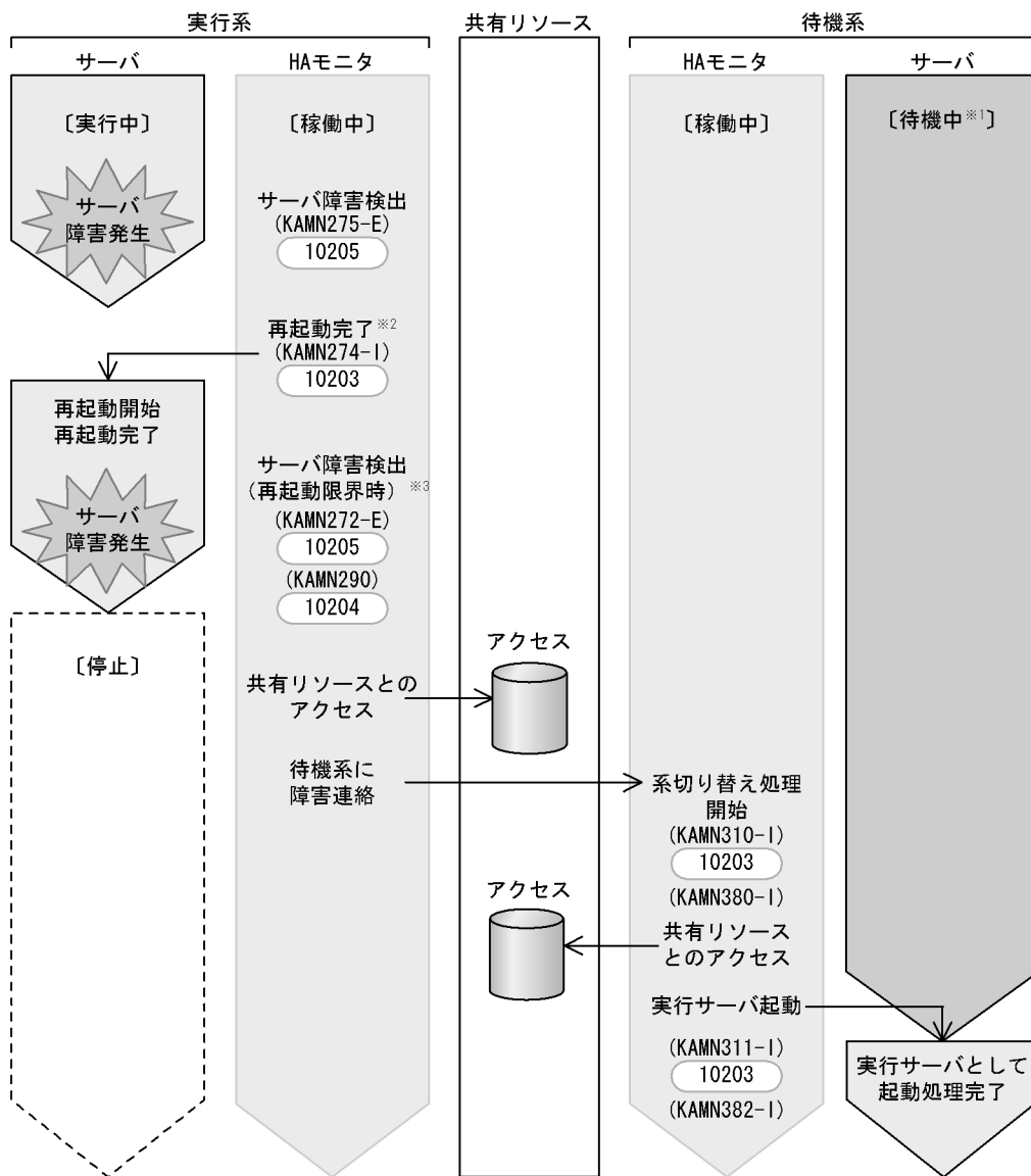
図 A-19 モニタモードのサーバでの障害検出時のイベント発行タイミング
