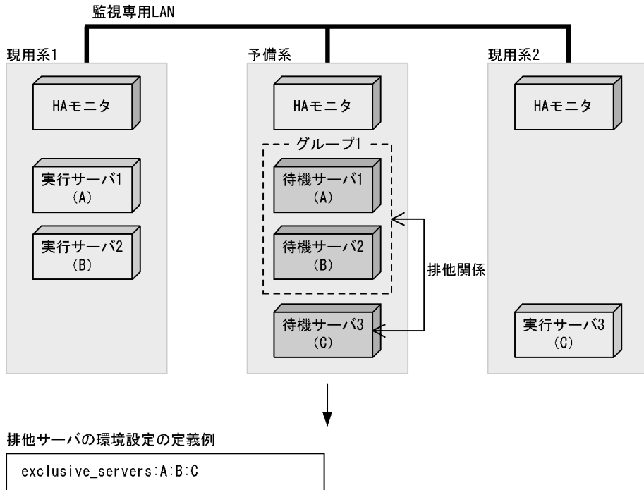
図 8-17 グループとサーバ単体で排他関係にある場合の環境設定の定義例
