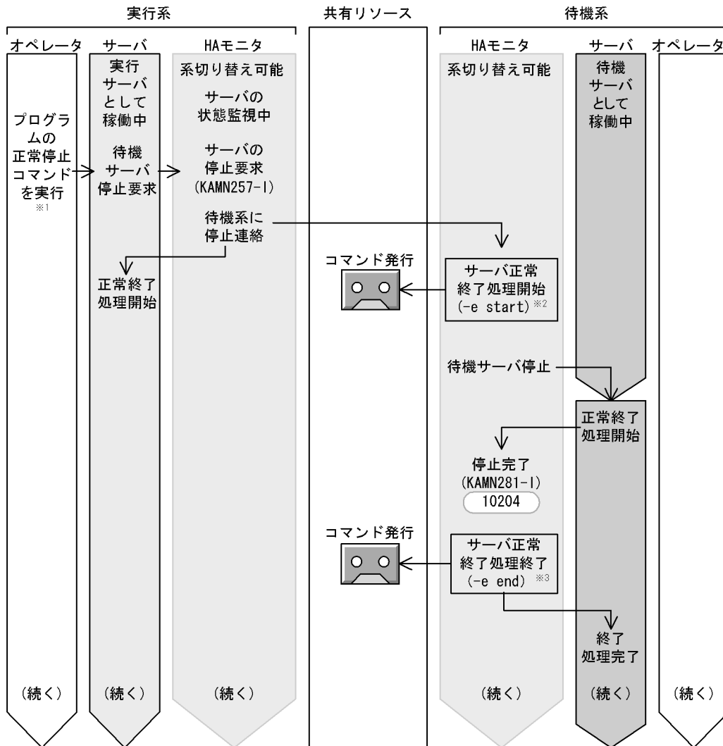
図 4-41 サーバの停止処理の流れ (待機サーバの停止) (サーバモード：実行サーバの停止処理開始時に待機サーバを停止する)
