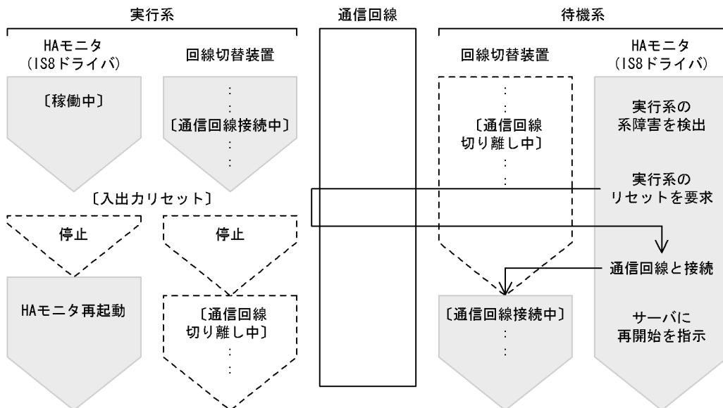
図 4-26 系障害時の、回線切替装置を使用した通信回線の切り替えの流れ (H9000V)
