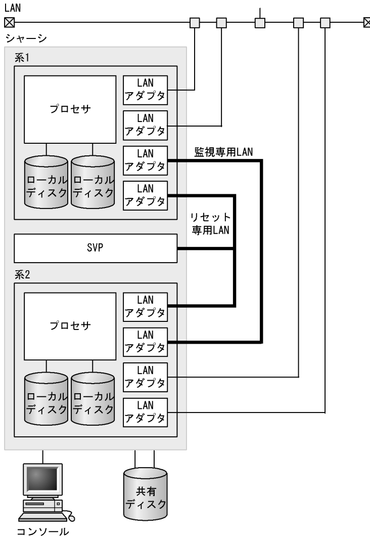
図 5-13 同一シャーシ内での 1:1 系切り替え構成時のハードウェア構成例 (BladeSymphony)
