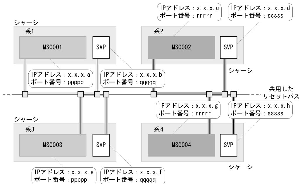
図 6-7 リセットパスの設定例 4 (BladeSymphony)
