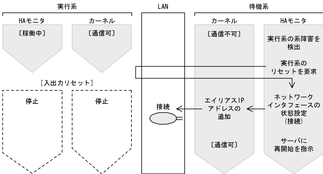
図 4-23 系障害時の LAN の切り替えの流れ
