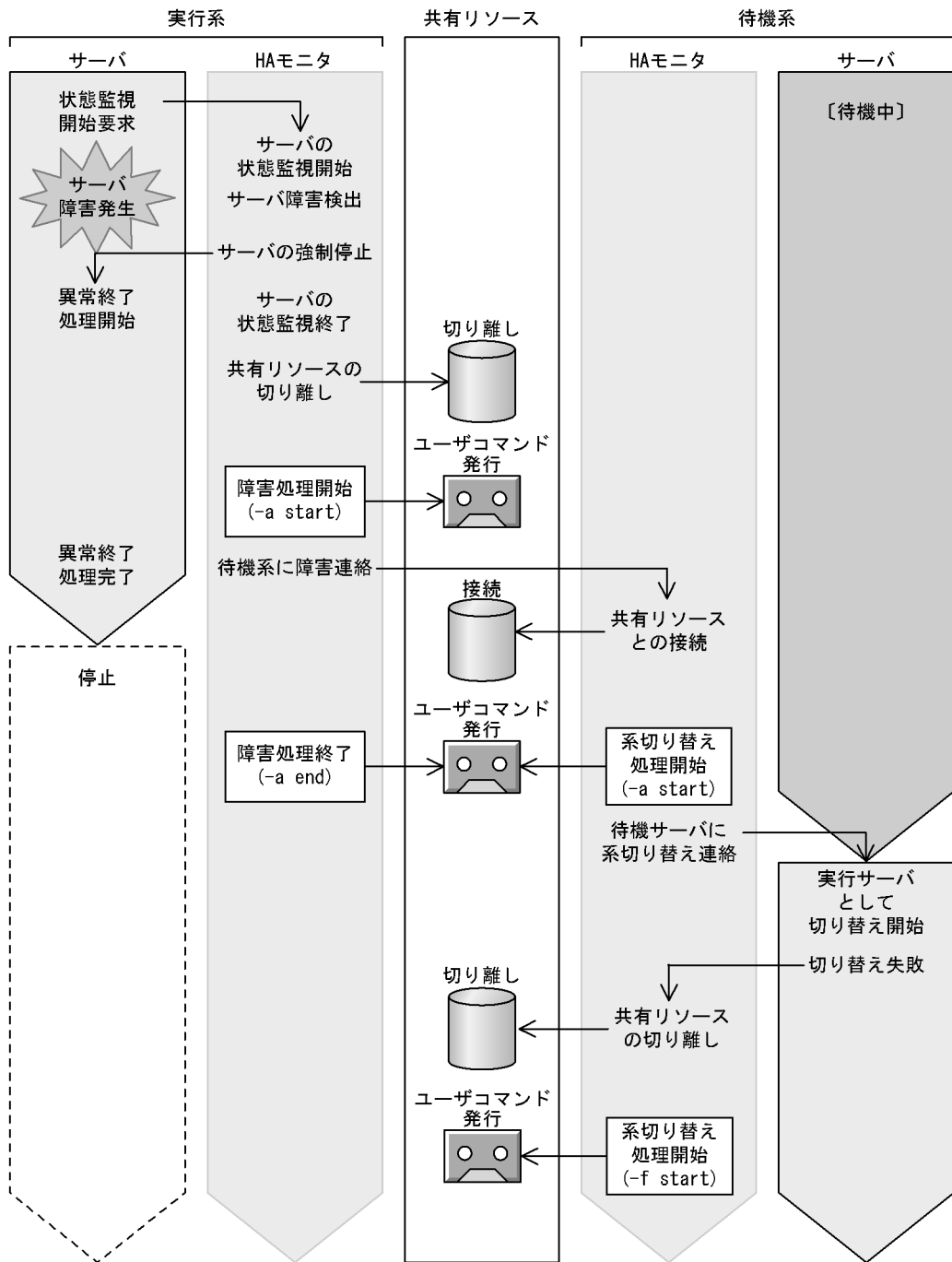
図 6-19 系切り替え失敗時に渡されるパラメタと発行タイミング
