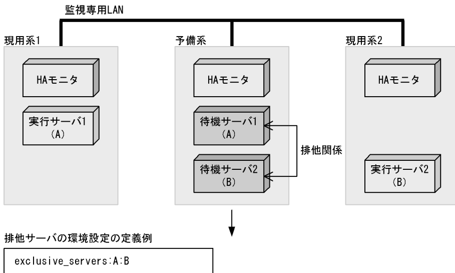
図 8-12 サーバ単位に排他関係にある場合の環境設定の定義例
