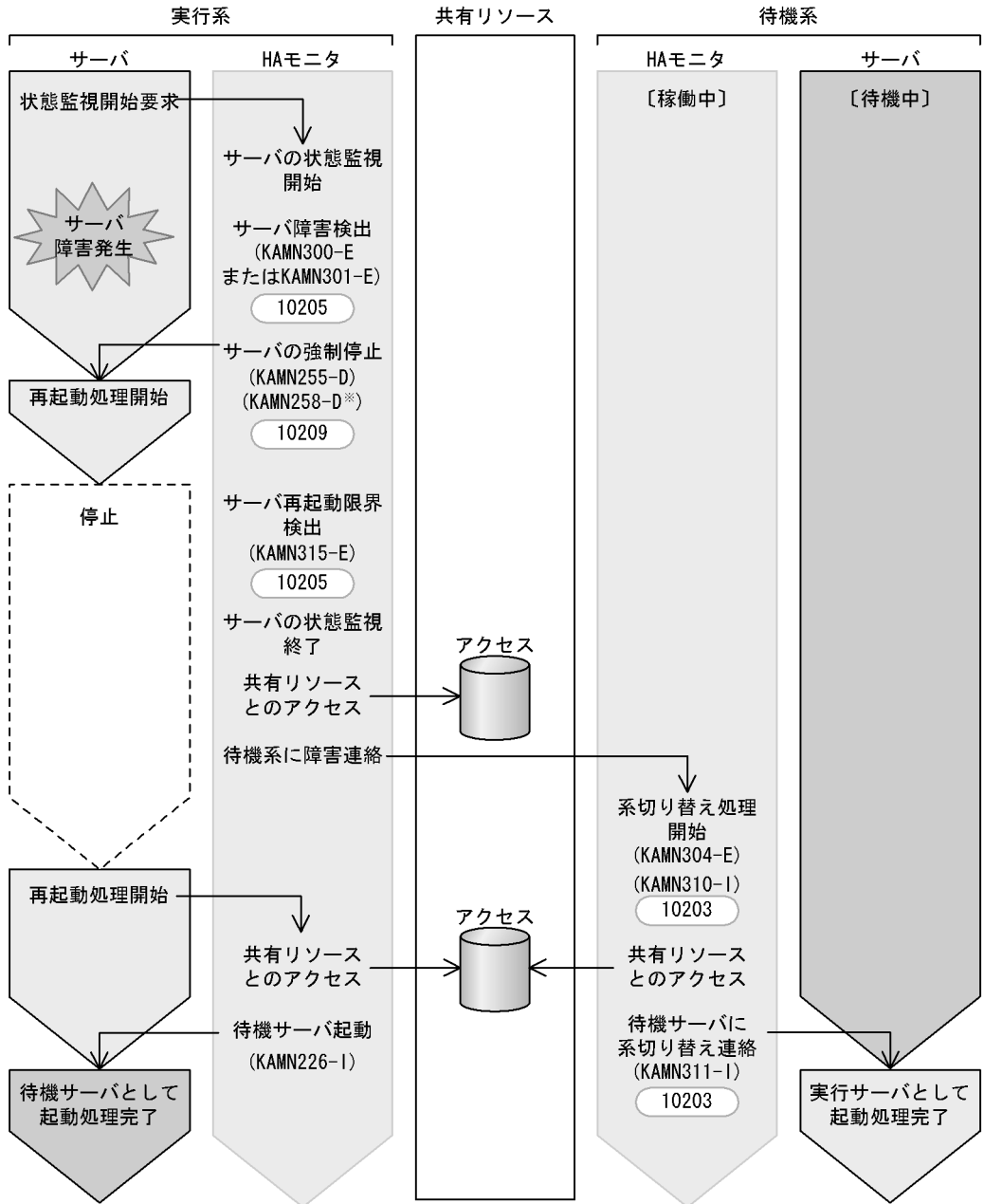
図 A-16 サーバ再起動限界時 ( switchtype = restart ) のイベント発行タイミング
