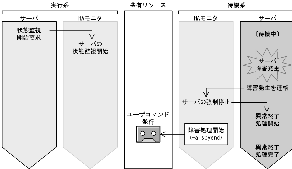
図 6-22 待機サーバ障害時に渡されるパラメタと発行タイミング
