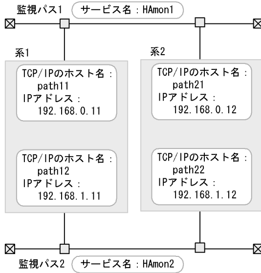
図 6-10 監視パスの構成例
