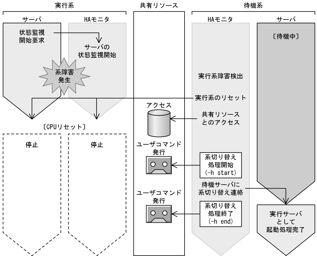
図 6-23 系障害時に渡されるパラメタと発行タイミング
