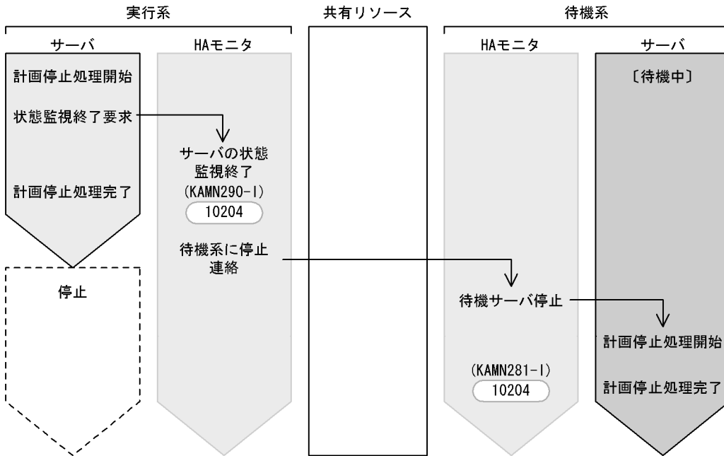
図 A-11 サーバ計画停止時のイベント発行タイミング
