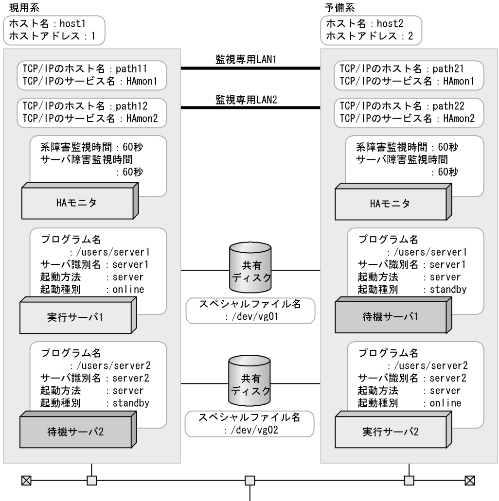
図 8-4 相互系切り替え構成時のシステム構成
