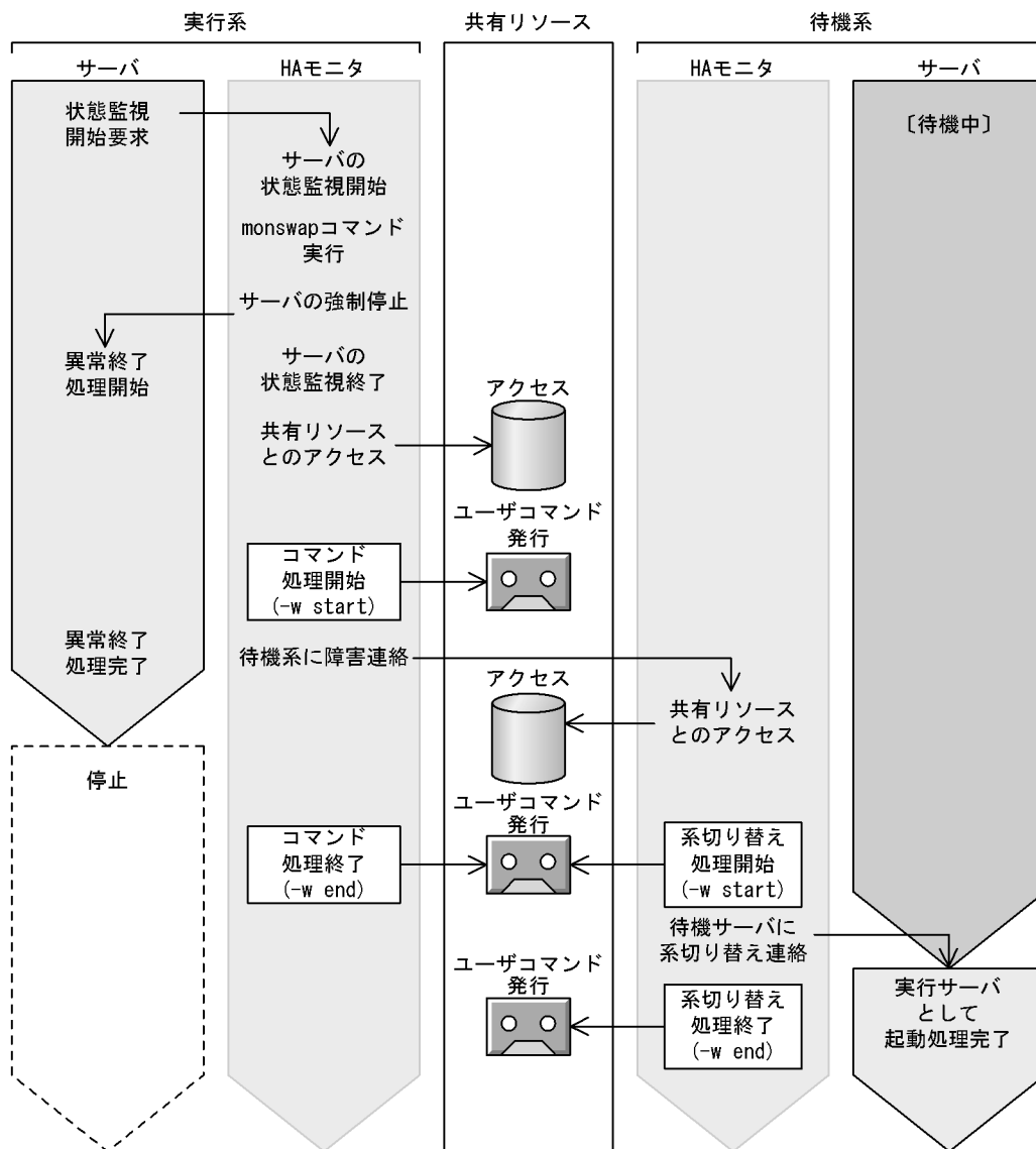
図 6-24 計画系切り替え時に渡されるパラメタと発行タイミング
