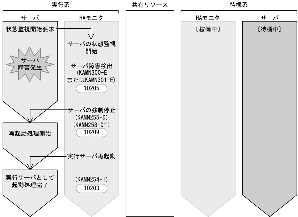
図 A-14 サーバ障害時 ( switchtype = restart ) のイベント発行タイミング
