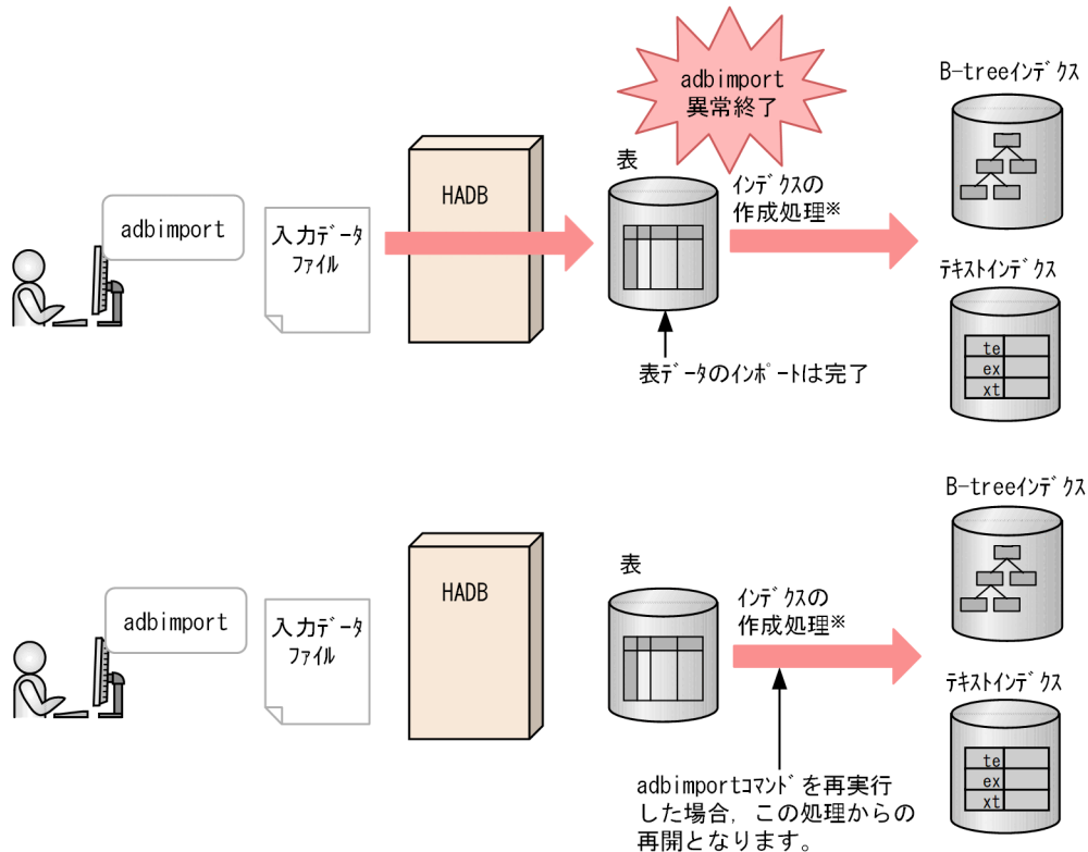
図 17-3 B-tree インデクスとテキストインデクス作成処理からの再実行機能
