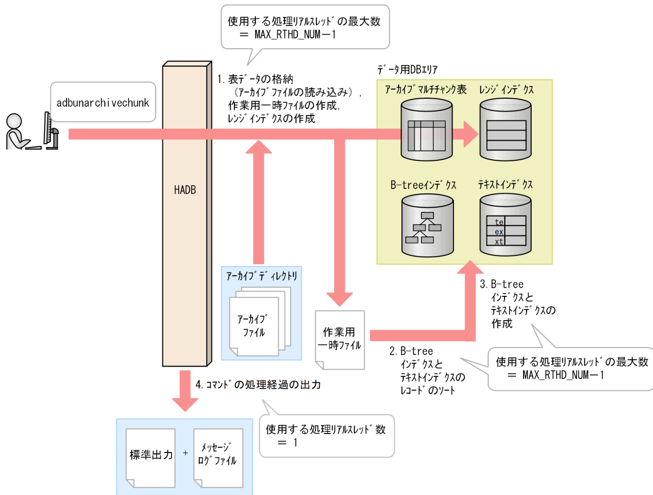
図 47-2 adbunarchivechunk コマンドが処理リアルスレッドを使用する処理
