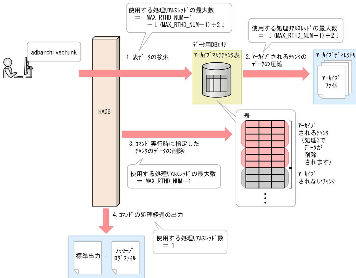
図 2-2 adbarchivechunk コマンドが処理リアルスレッドを使用する処理
