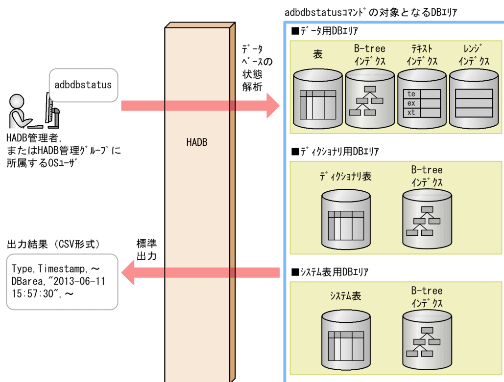
図 13-1 adbdstatus コマンドの概要
