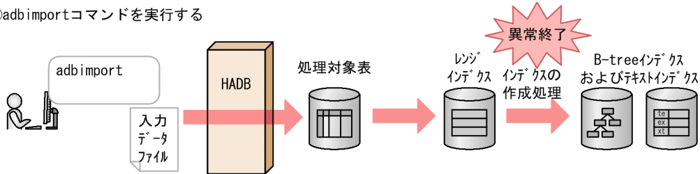
図 16-7 adbimport コマンドからのインデクス作成処理の引き継ぎ (--create-temp-file オプションを指定する場合)
