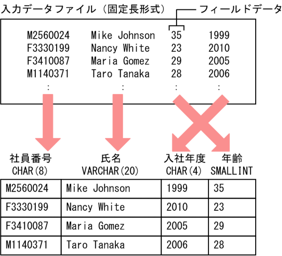
図 17-17 固定長形式の例
