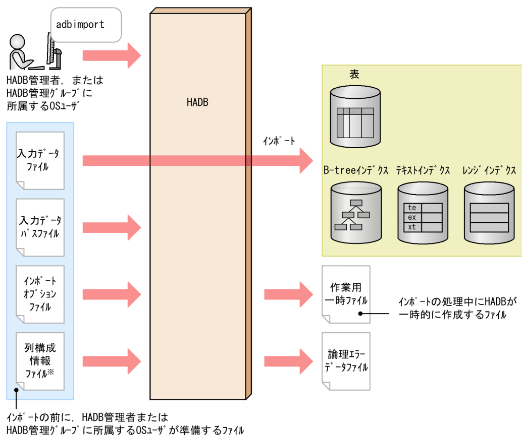
図 17-1 データインポート処理の概要
