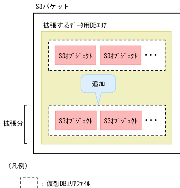
図 37-11 データ用 DB エリアの拡張 (AWS 環境または Amazon S3 互換オブジェクトストレージ環境でクラウドストレージ機能を使用している場合)
