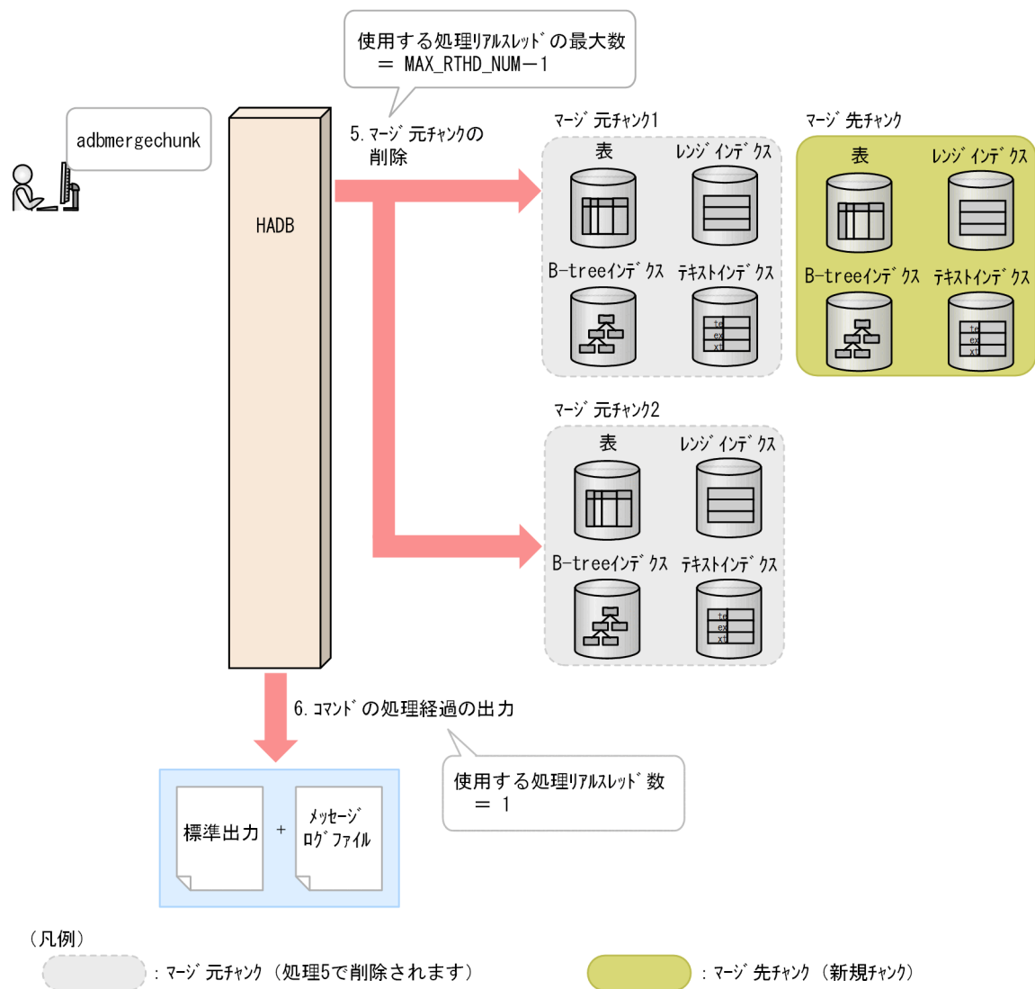
図 35-3 adbmergechunk コマンドが処理リアルスレッドを使用する処理（その 2）
