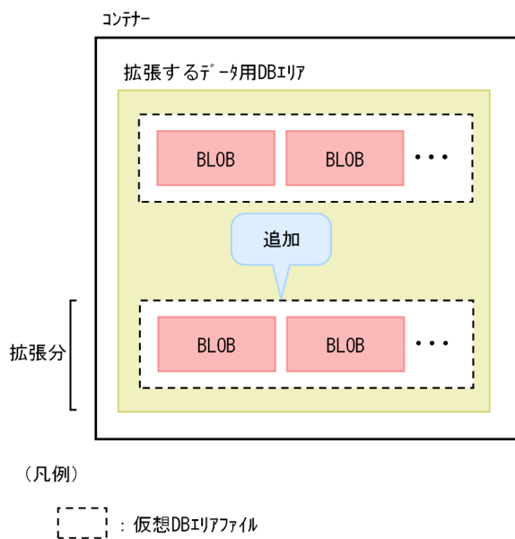
図 37-12 データ用 DB エリアの拡張 (Azure 環境でクラウドストレージ機能を使用している場合)
