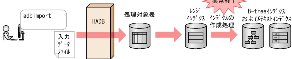
図 16-8 adbimport コマンドからのインデクス作成処理の引き継ぎ (--force オプションを指定する場合)
