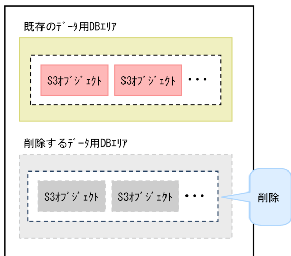
図 37-7 データ用 DB エリアの削除（AWS 環境または Amazon S3 互換オブジェクトストレージ環境でクラウドストレージ機能を使用している場合）
