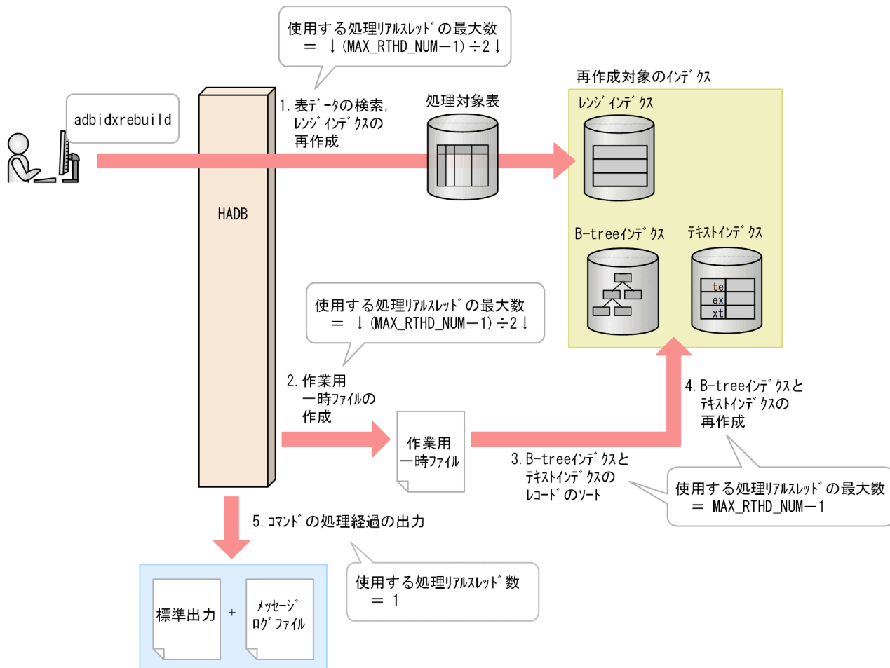
図 16-9 adbidxrebuild コマンドが処理リアルスレッドを使用する処理
