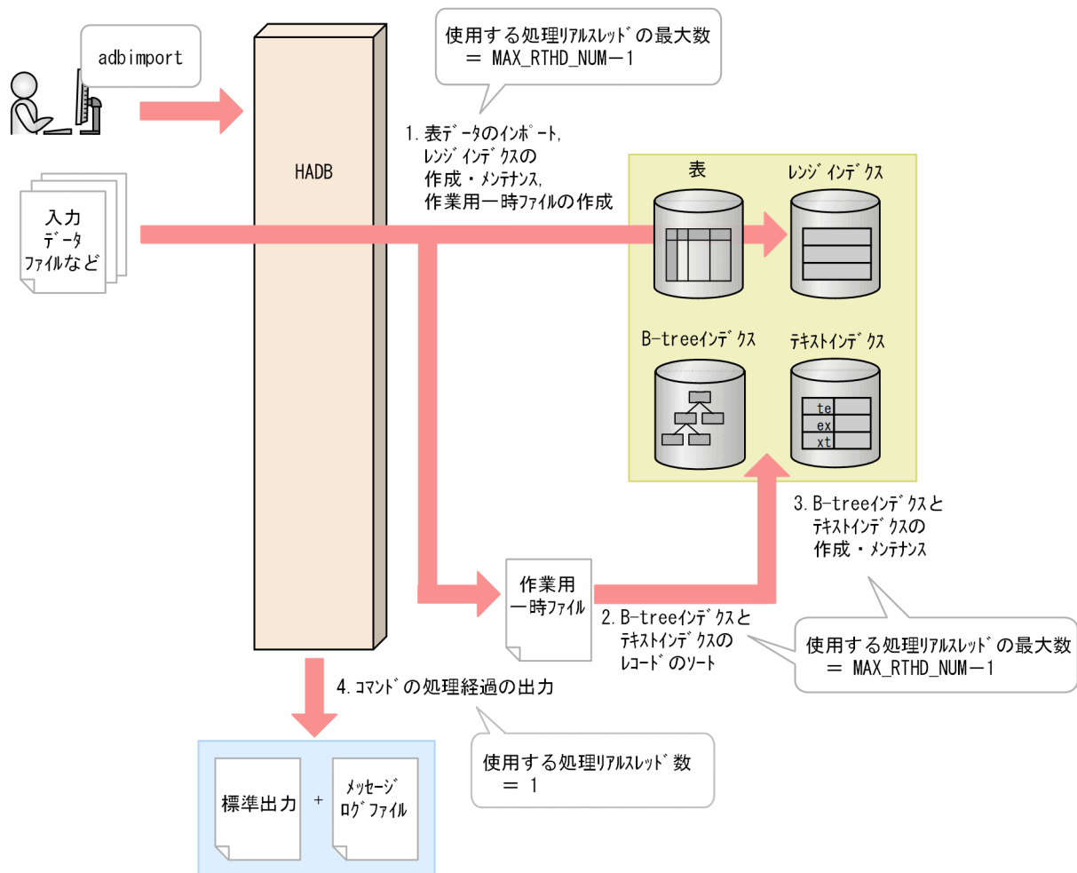
図 17-5 adbimport コマンドが処理リアルスレッドを使用する処理
