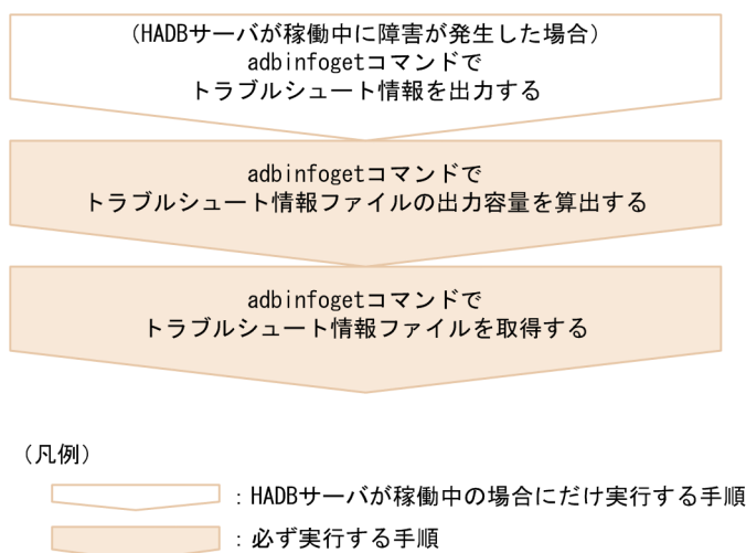
図 18-1 adbinfoget コマンドでトラブルシューティング情報ファイルを取得する際の流れ
