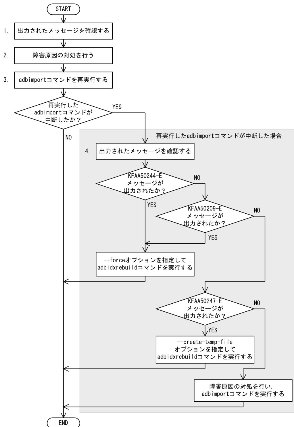
図 17-19 adbimport コマンドが異常終了したときの対処手順
