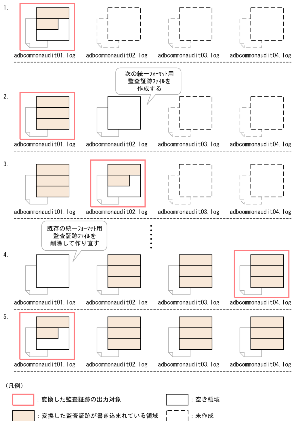
図 12-2 統一フォーマット用監査証跡ファイルの切り替え
