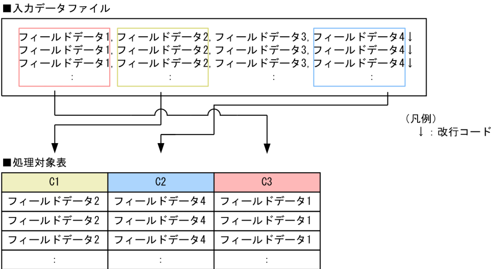
図 17-9 入力データファイルのフィールドデータの数処理対象表の列定義数より多い場合
