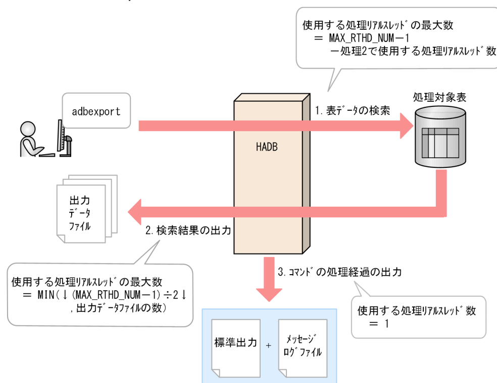
図 14-2 adbexport コマンドが処理リアルスレッドを使用する処理
