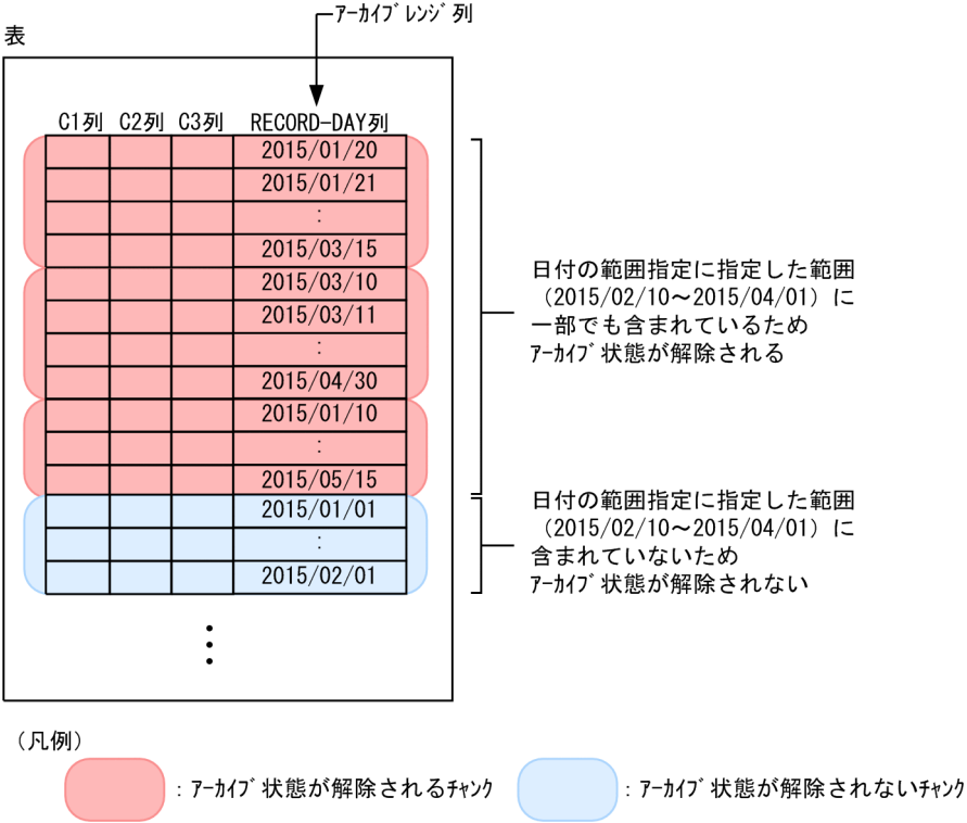
図 47-4 日付の範囲指定の内容とアーカイブ状態が解除されるチャンクの関係
