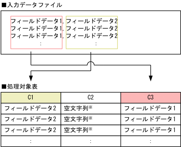
図 17-8 入力データファイルのフィールドデータの数処理対象表の列定義数より少ない場合
