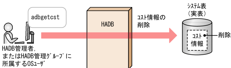
図 15-2 コスト情報の削除
