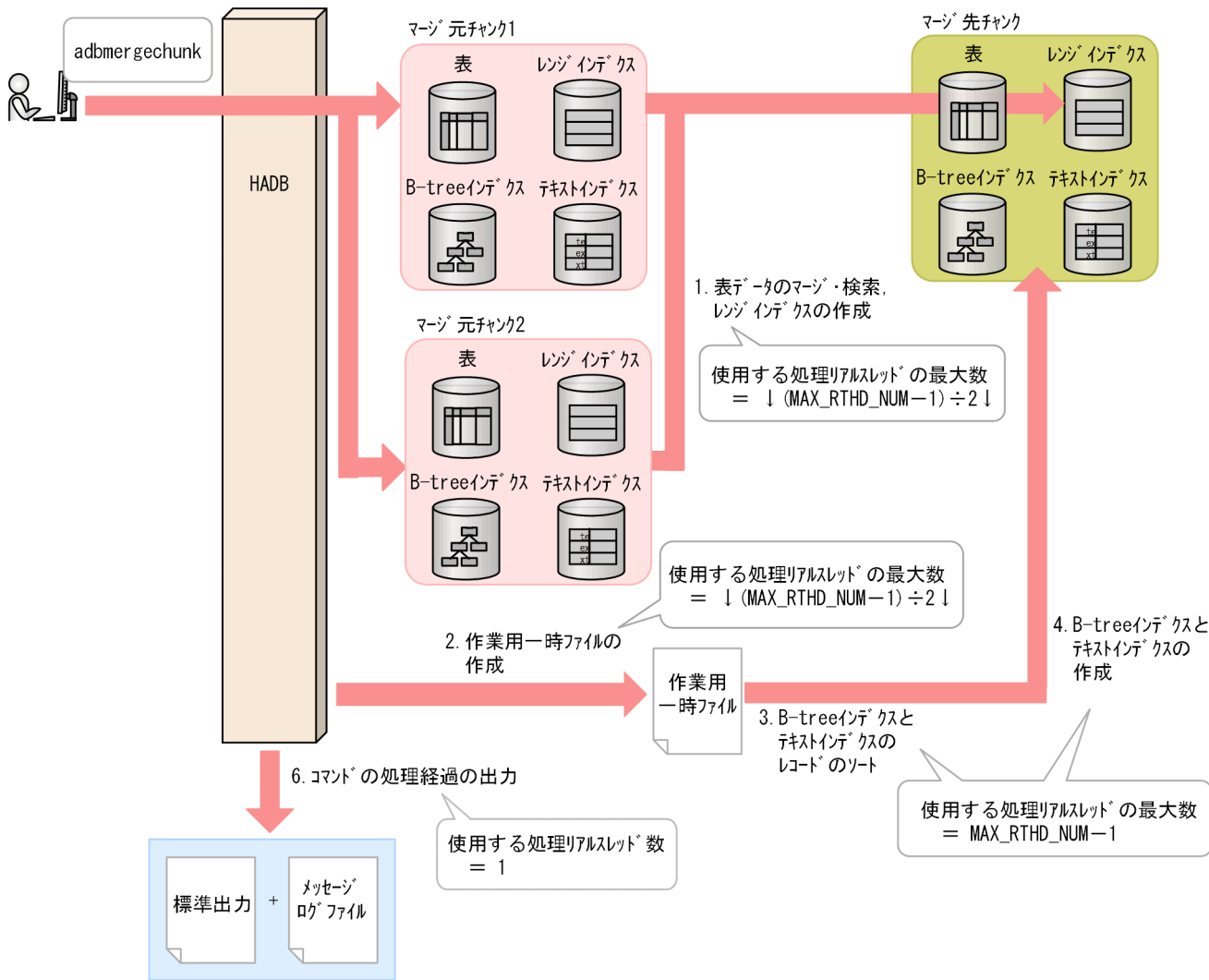
図 35-2 adbmergechunk コマンドが処理リアルスレッドを使用する処理（その 1）
