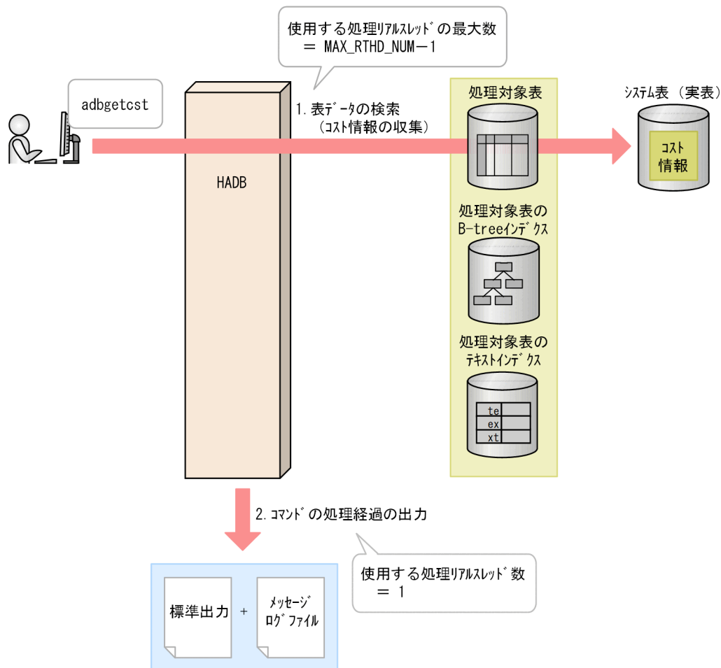
図 15-3 adbgetcst コマンドが処理リアルスレッドを使用する処理
