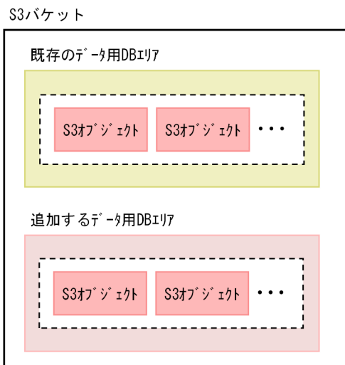
図 37-3 データ用 DB エリアの追加 (AWS 環境または Amazon S3 互換オブジェクトストレージ環境でクラウドストレージ機能を使用している場合)
