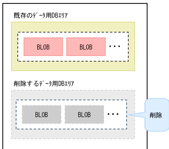
図 37-8 データ用 DB エリアの削除（Azure 環境でクラウドストレージ機能を使用している場合）
