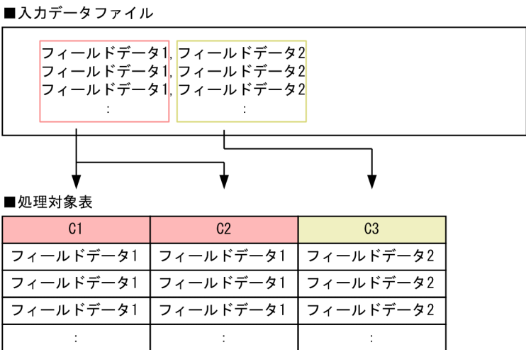
図 17-10 入力データファイルの特定のフィールドデータを処理対象表の複数列に格納する場合
