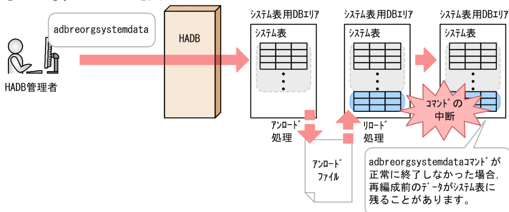
図 41-2 再編成前データの削除機能の概要
