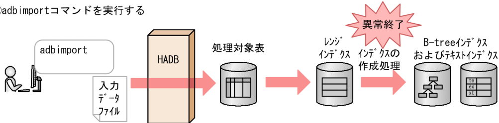
図 16-8 adbimport コマンドからのインデクス作成処理の引き継ぎ (--force オプションを指定する場合)
