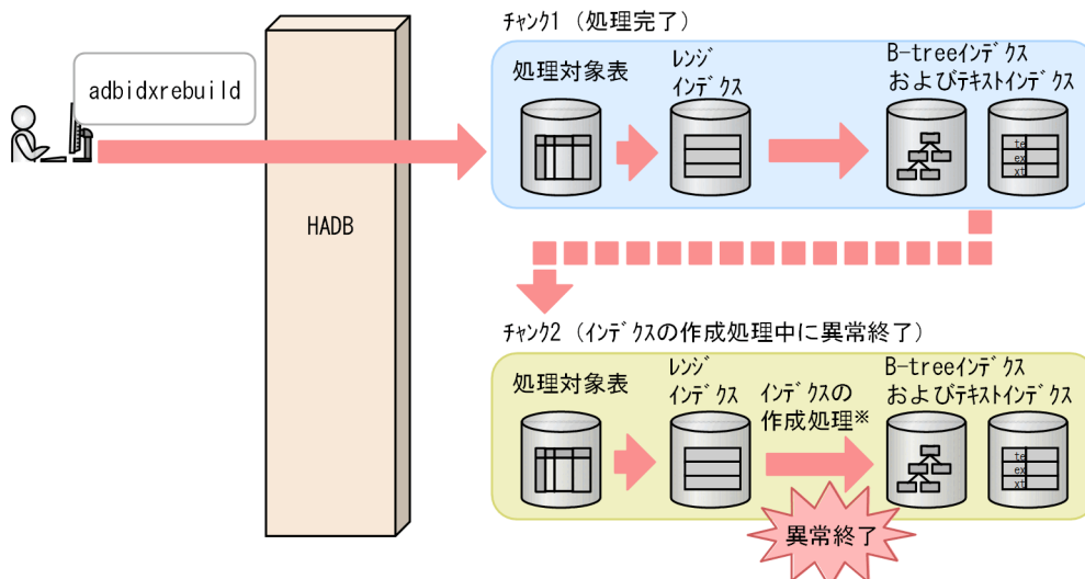
図 16-6 処理が中断したチャンクのB-tree インデクスおよびテキストインデクスの作成処理からの再実行
