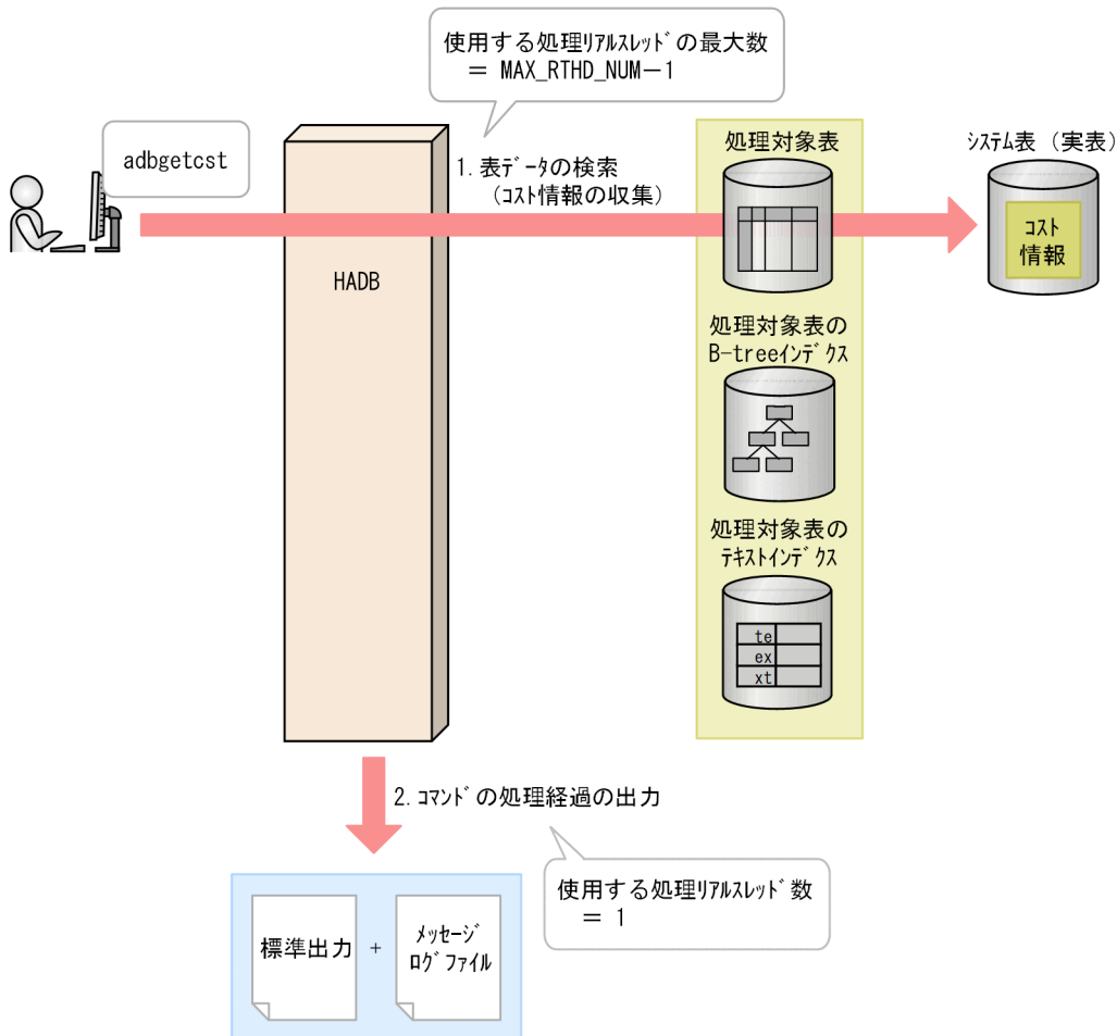
図 15-3 adbgetcst コマンドが処理リアルスレッドを使用する処理
