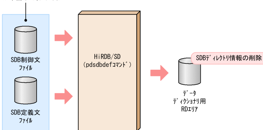
図 11-8 SDB ディレクトリ情報の削除
