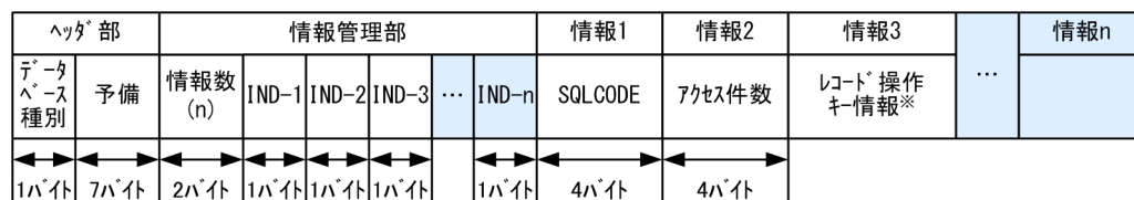
図 7-16 レコード操作出力情報の形式
