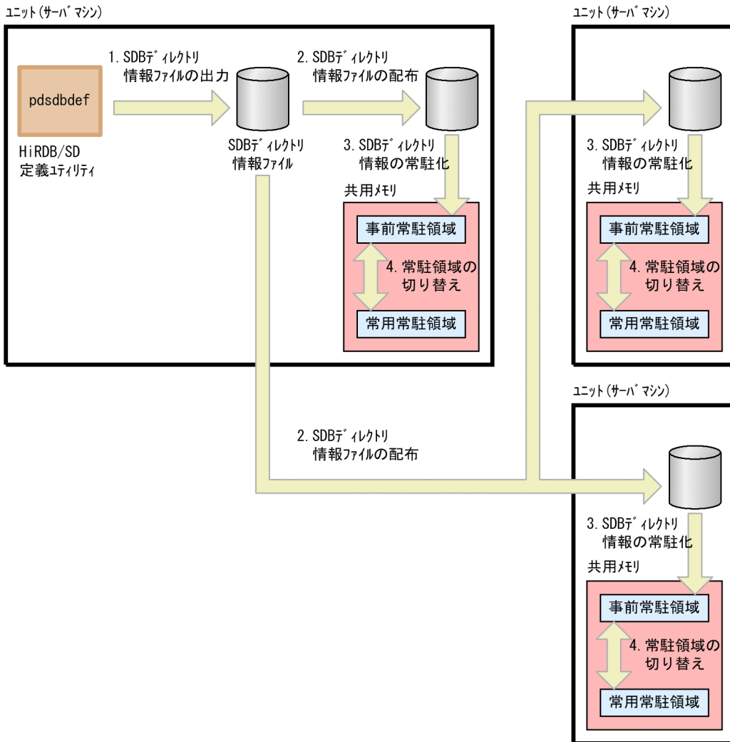
図 2-25 SDB ディレクトリ情報の常駐化コマンド (pdsdbarc コマンド) による SDB ディレクトリ情報の共用メモリ上への常駐化
