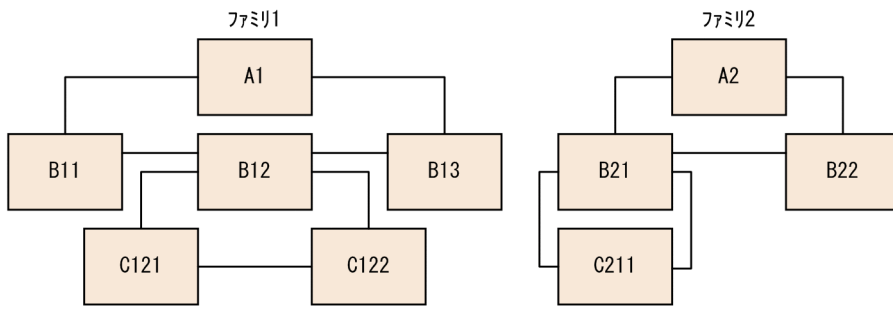
図 2-70 事前ページ割り当て機能を適用している場合の、サブページ間の関連づけとファミリー内接続サブページの例
