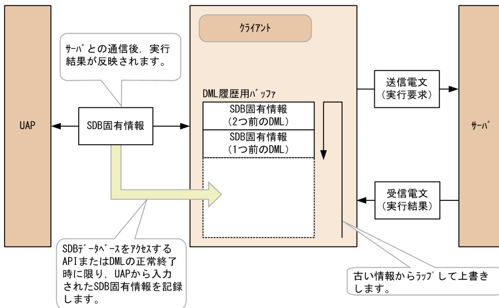
図 16-5 DML 履歴用バッファの記録イメージ
