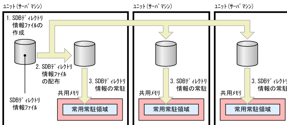
図 5-1 SDB ディレクトリ情報を変更する際の流れ
