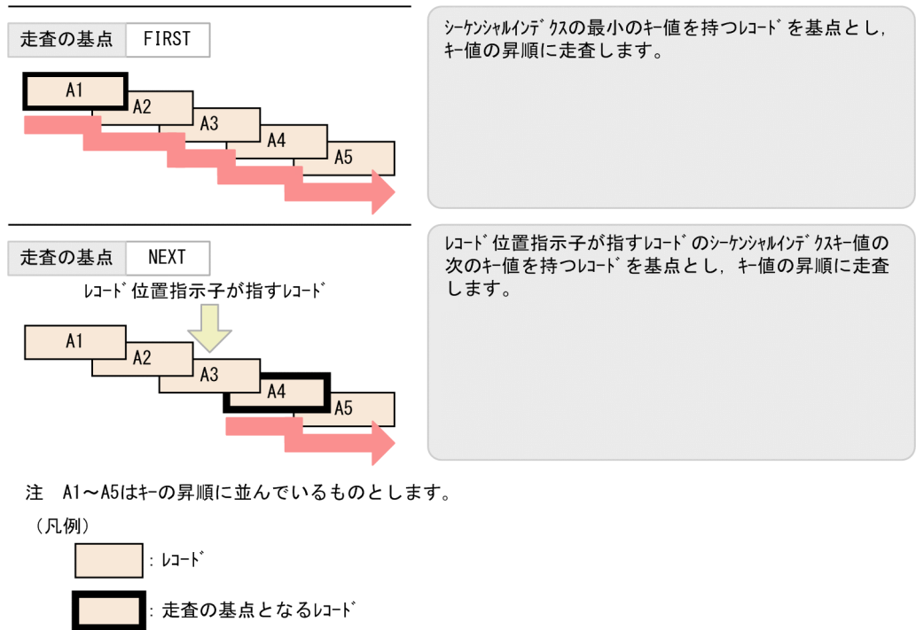
図 2-32 走査の基点となるレコードと走査の方向と走査範囲
