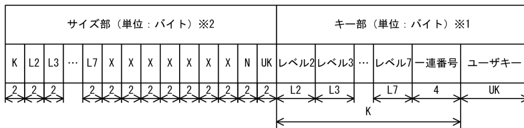
図 7-18 レコード操作キー情報の形式 (4V AFM の SDB データベースの場合)
