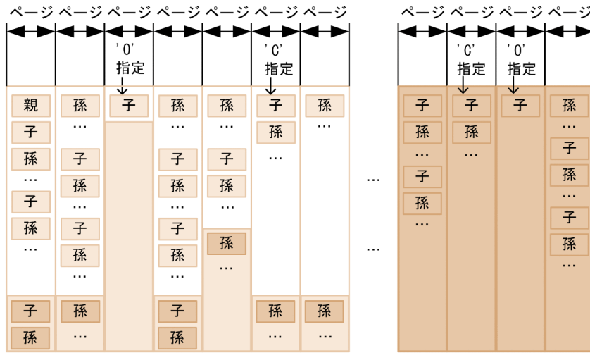
図 3-11 見積もり例に従った格納状態のイメージ
