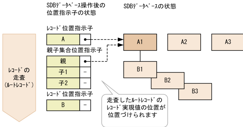
図 2-39 ルートレコードの走査
