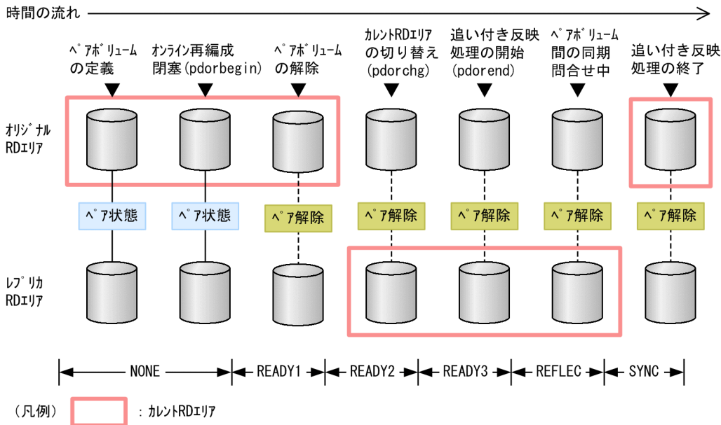
図 5-20 更新可能なオンライン再編成の障害発生時点
