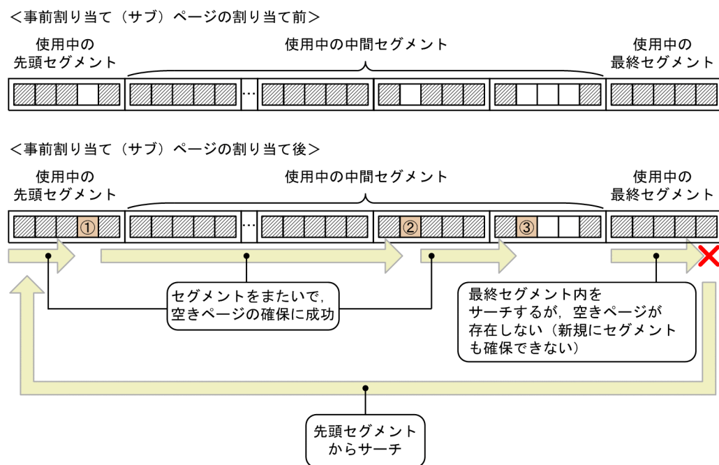
図 2-63 空きページのサーチ例
