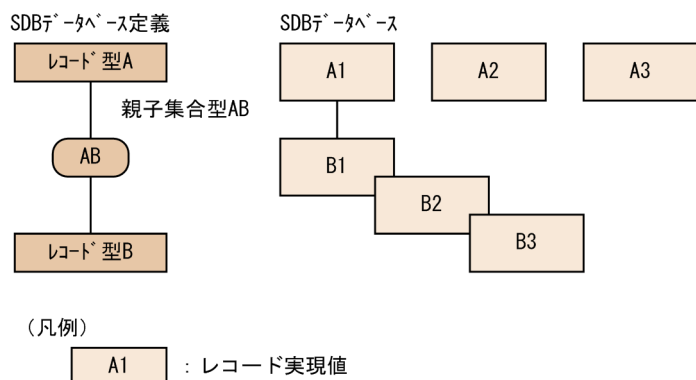
図 2-35 SDB データベースの操作と位置指示子の関係の説明で使用する SDB データベース
