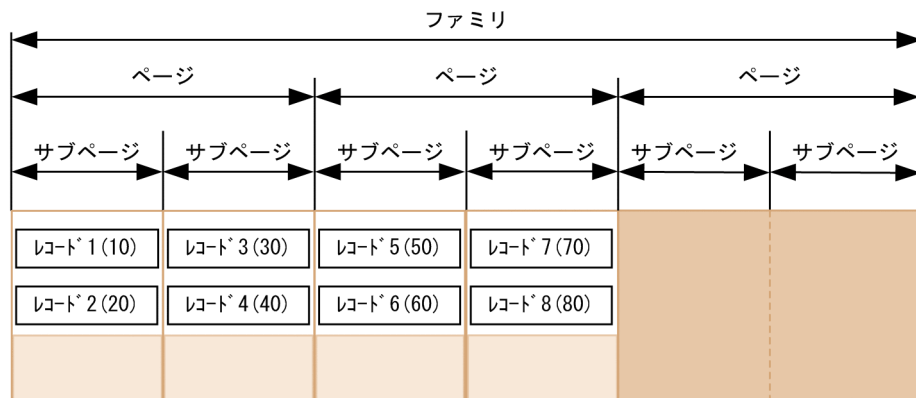
図 3-16 見積もりで想定するレコード格納状態
