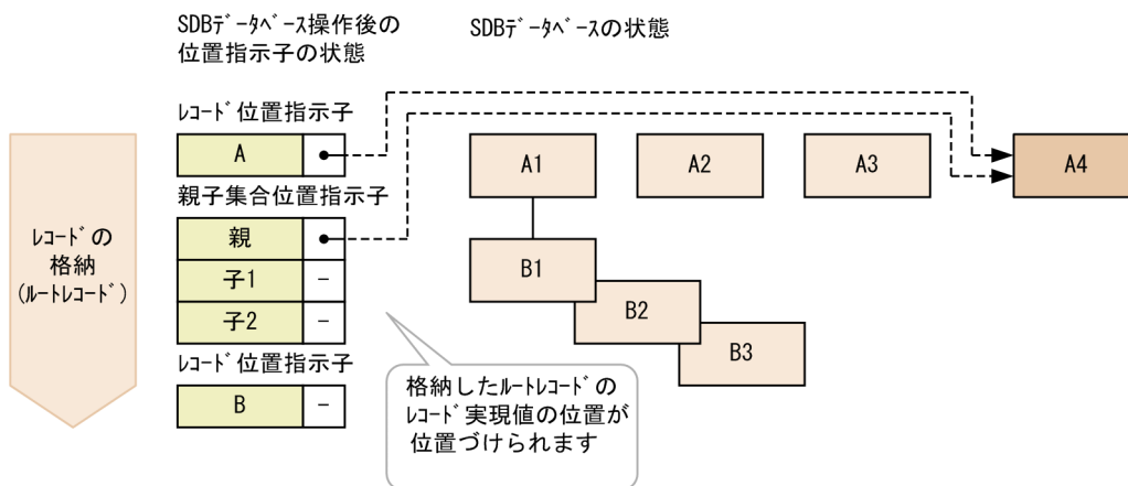
図 2-40 ルートレコードの格納 (ルートレコードの追加)
