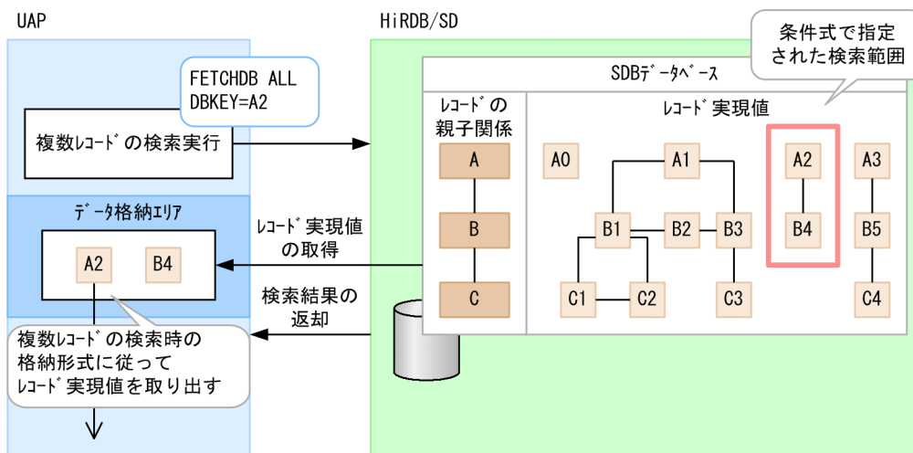
図 2-34 複数レコードの検索の概要
