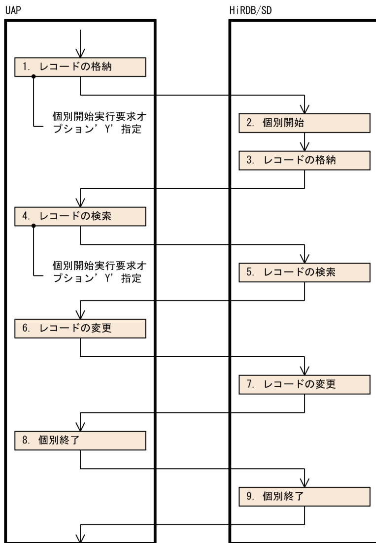
図 2-47 SDB データベースを操作する処理の流れ（個別開始実行要求オプションを指定する場合）
