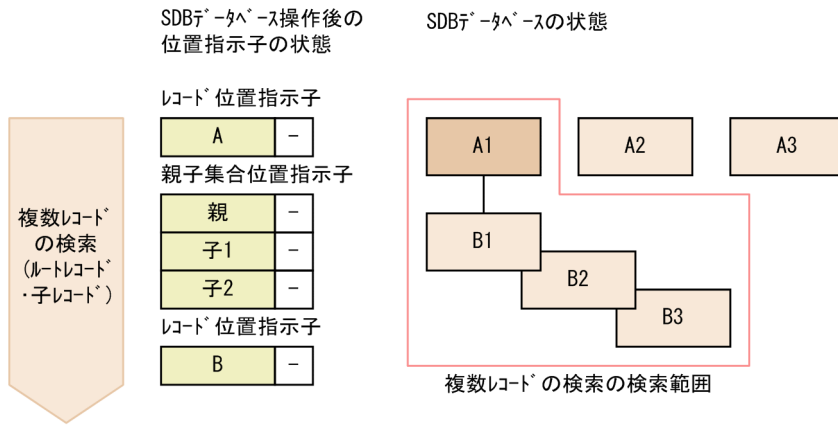
図 2-45 複数レコードの検索
