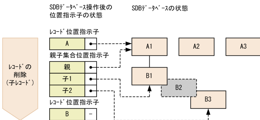
図 2-44 子レコードの削除
