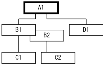
図 2-28 4V FMB または SD FMB の SDB データベースのアクセス順序の概要
