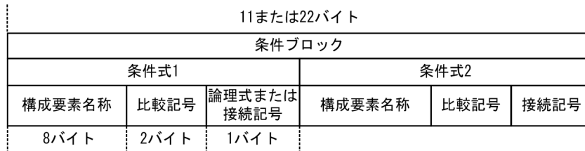
図 7-12 キーの条件の条件ブロックの形式
