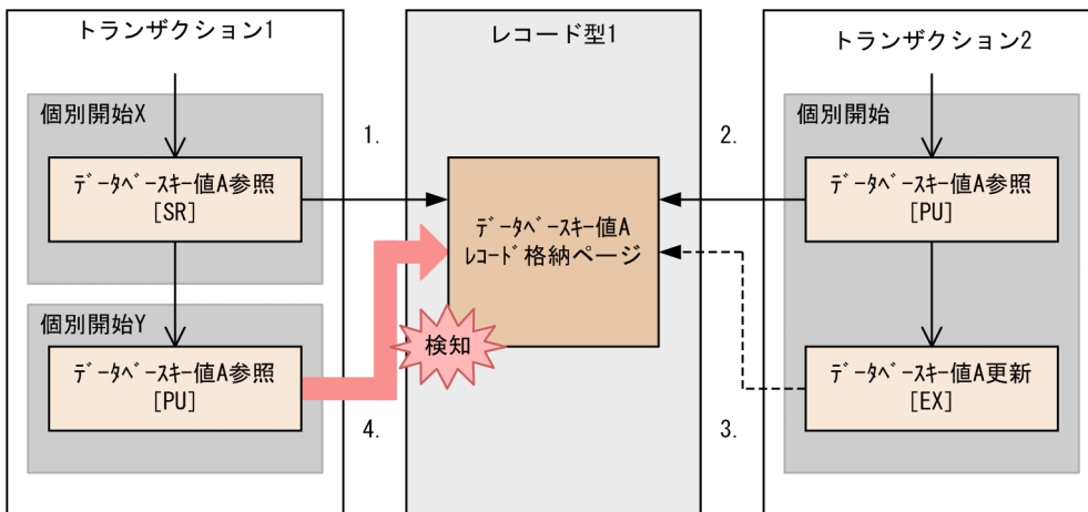
図 2-89 排他モード 1 の指定が異なる検索が混在するトランザクションと、ほかのトランザクションが同じレコード（同じページ）に対してアクセスした場合の、デッドロックの例
