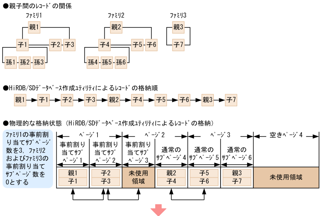
図 2-82 事前ページ割り当て機能の適用有無の違いによるファミリの格納例（サブページ分割をする場合）
