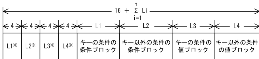
図 7-11 アクセス条件の形式
