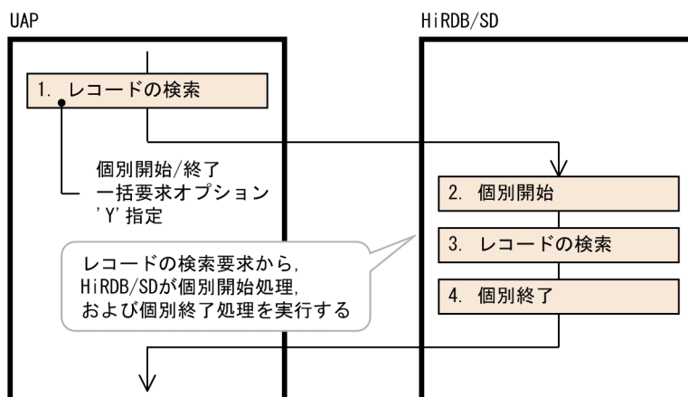
図 2-30 レコードの検索処理の流れ（個別開始/終了一括要求オプションを指定した場合）
