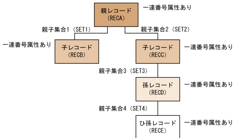
図 11-24 作成する SD FMB の SDB データベースの階層構造
