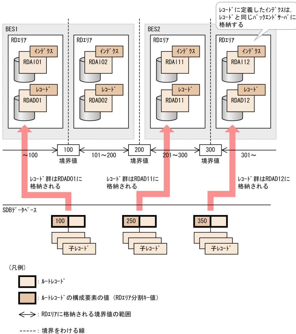
図 2-17 境界値指定の例
