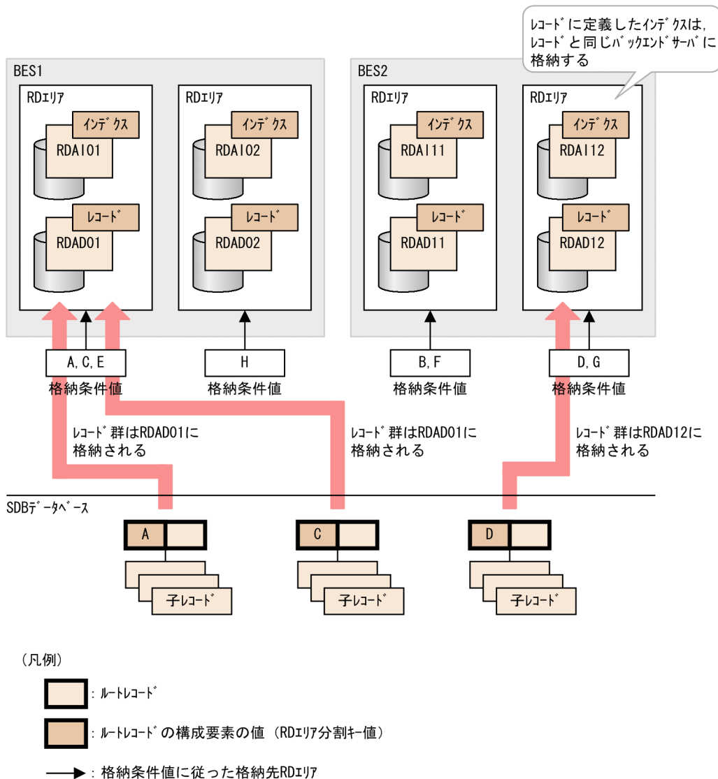
図 2-16 格納条件指定の例
