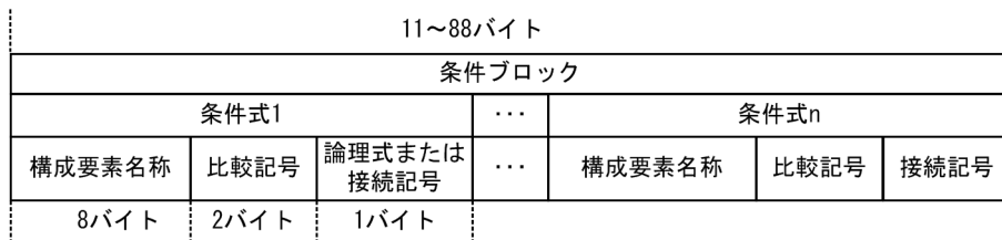
図 7-13 キー以外の条件の条件ブロックの形式
