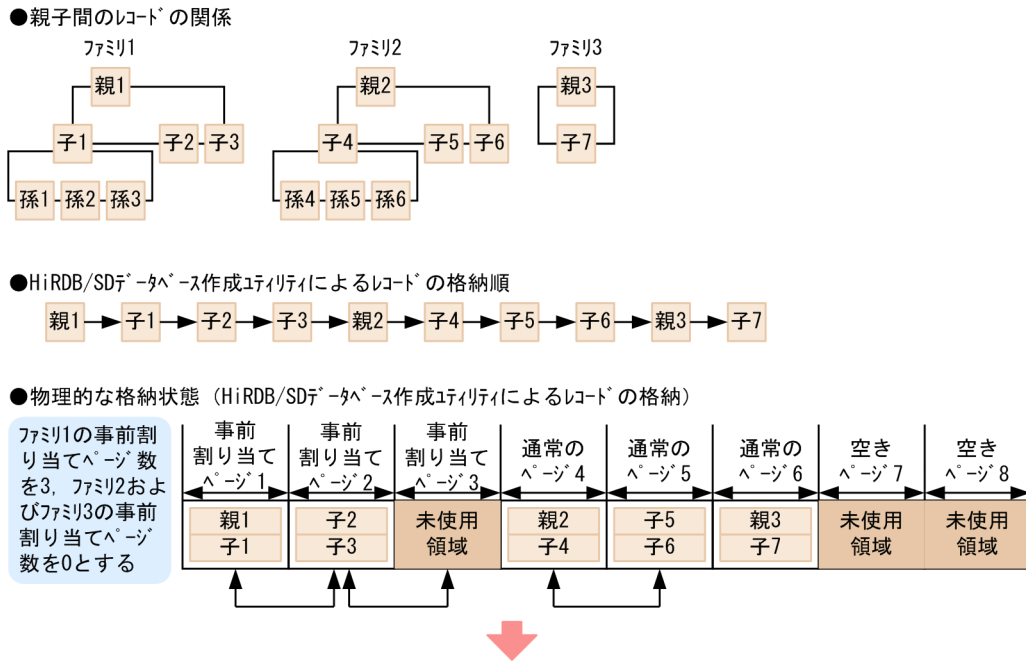
図 2-65 事前ページ割り当て機能の適用有無の違いによるファミリの格納例（サブページ分割をしない場合）
