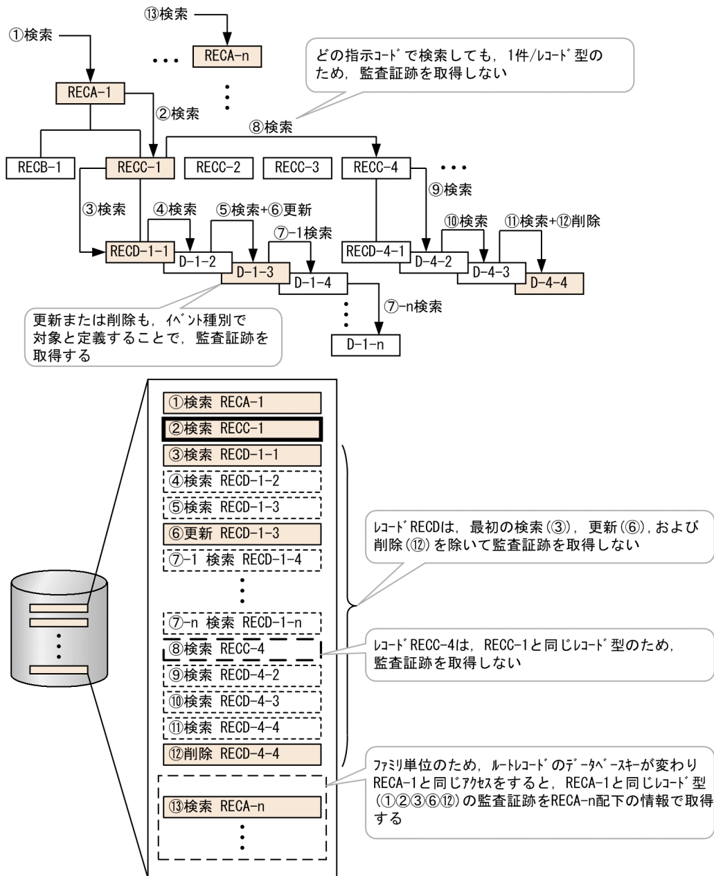
図 7-10 SDB データベースの操作時に取得される監査証跡の関連
