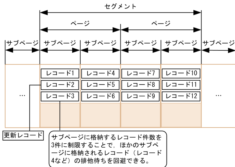
図 3-15 サブページに格納するレコード件数を制限する例
