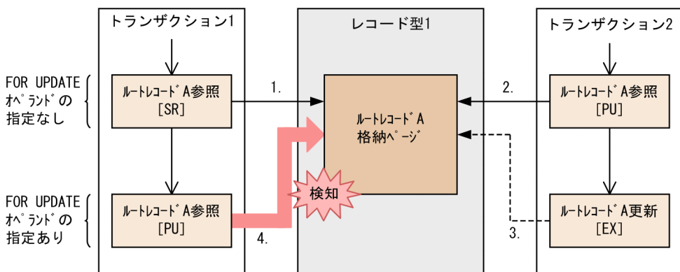
図 2-90 FOR UPDATE オペランドの指定の有無が異なる検索が混在するトランザクションと、ほかのトランザクションが同じレコード（同じページ）に対してアクセスした場合の、デッドロックの例
