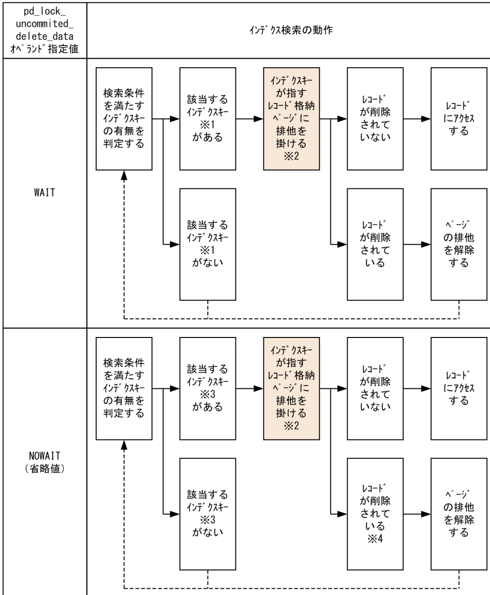
図 2-92 pd_lock_uncommitted_delete_data オペランド指定によるインデックス検索の動作の違い
