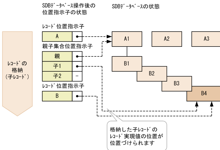
図 2-41 子レコードの格納（子レコードの追加）
