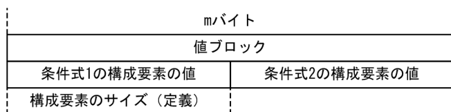
図 7-14 キーの条件の値ブロックの形式
