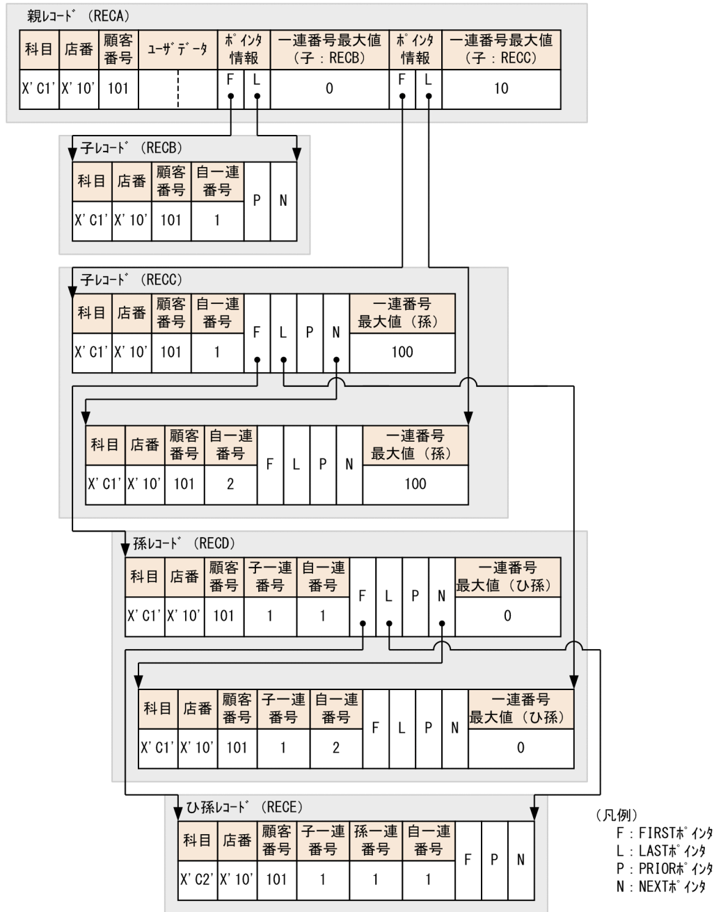
図 11-25 作成する SD FMB の SDB データベースの格納構造
