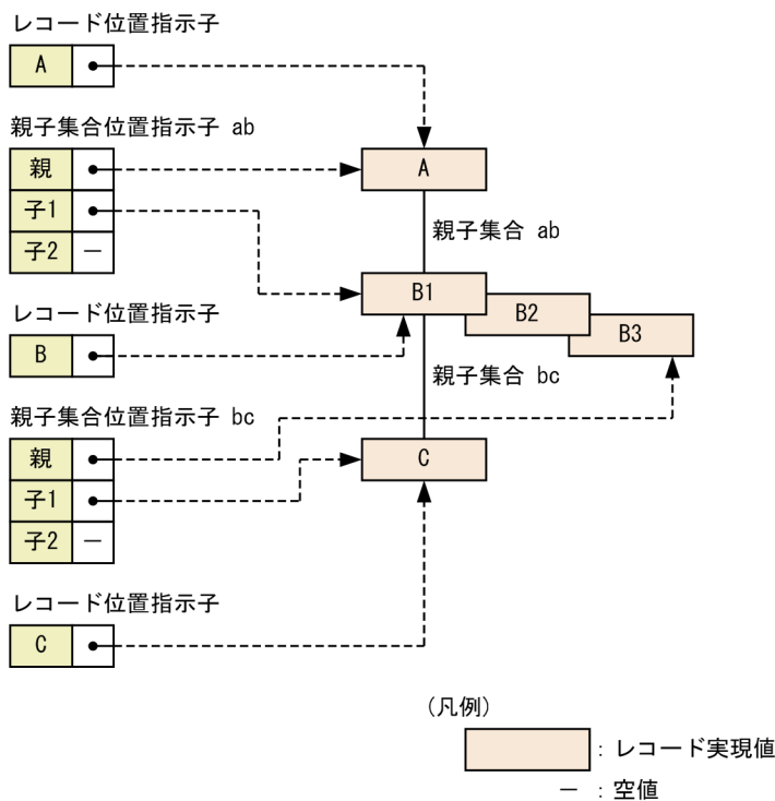
図 2-26 レコード位置指示子と親子集合位置指示子
