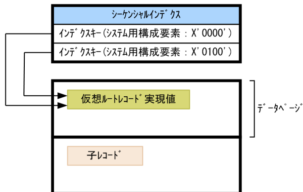
図 2-19 仮想ルートレコード型に定義したシーケンシャルインデックスの物理構造（配下に有効な子レコードが存在する場合）
