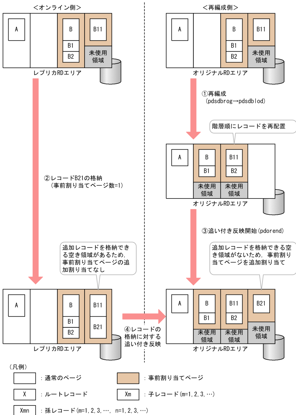
図 2-64 更新可能なオンライン再編成の追い付き反映処理での事前割り当てページ数の引き継ぎ例
