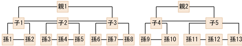
図 2-77 論理的に関連するレコードの格納位置をまとめる例
