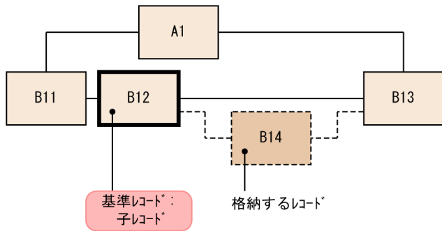
図 2-50 基準ページへの格納の例
