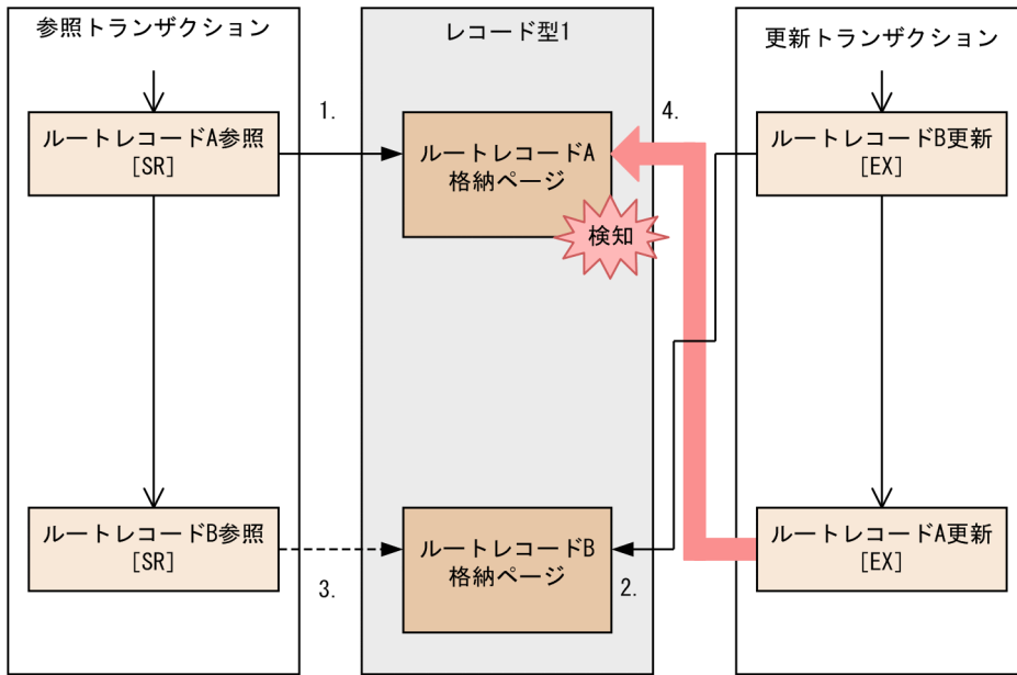
図 2-86 ルートレコードを格納しているページ間のデッドロックの例
