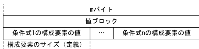
図 7-15 キー以外の条件の値ブロック形式
