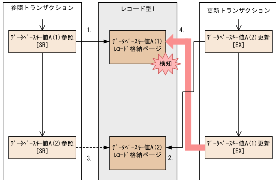
図 2-87 子レコードを格納しているページ間のデッドロックの例
