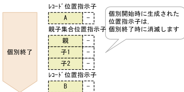
図 2-46 個別終了およびトランザクションの終了
