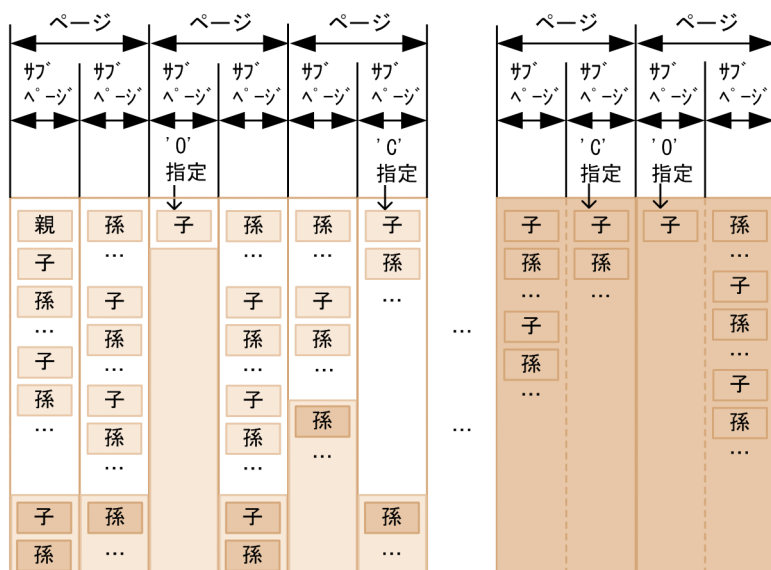
図 3-17 見積もり例に従った格納状態のイメージ
