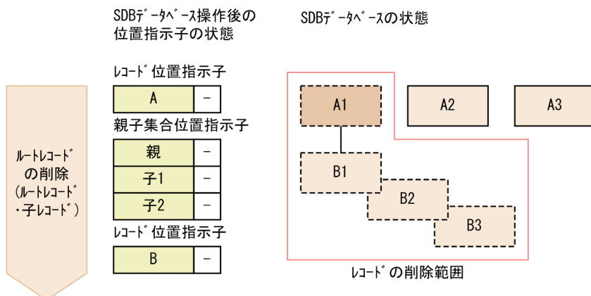
図 2-43 ルートレコード A1 を削除した場合の例
