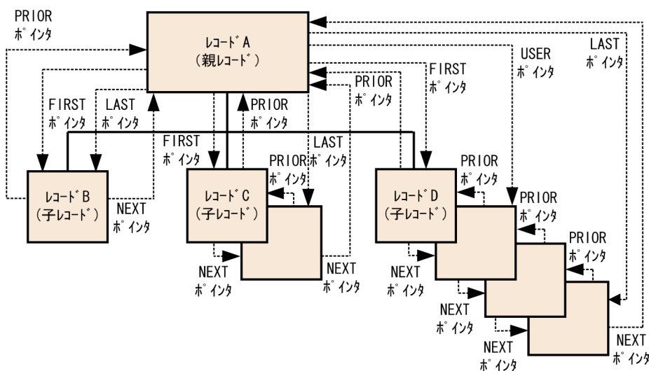
図 2-14 レコードとポインタの関係
