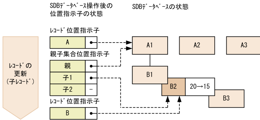
図 2-42 子レコードの更新
