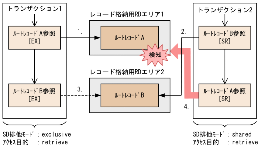
図 2-91 レコード格納用 RD エリア間のデッドロックの例
