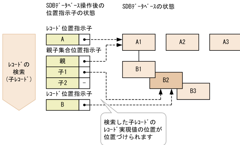
図 2-38 子レコードの検索
