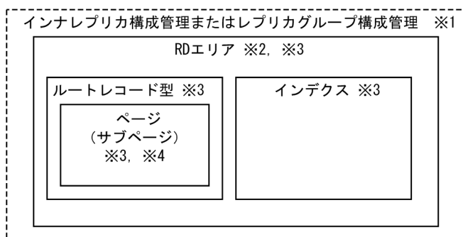
図 2-85 SDB データベースの排他資源とその包含関係
