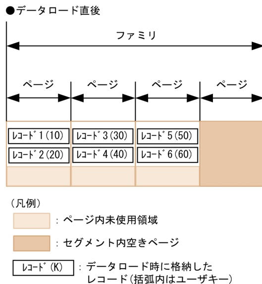
図 3-10 見積もりで想定するレコード格納状態
