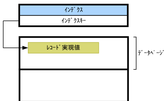
図 2-21 仮想ルートレコード型に定義したシーケンシャルインデックス以外のインデックスの物理構造
