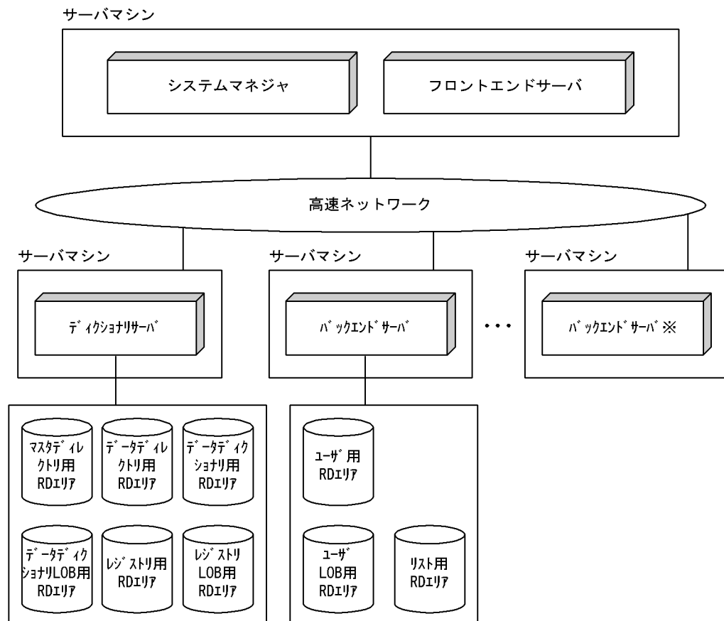
図 10-1 HiRDB/パラレルサーバのシステム構成例
