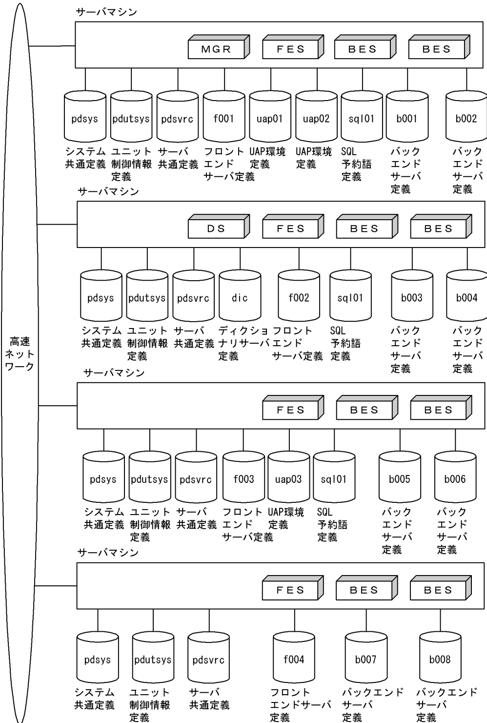
図 5-3 HiRDB システム定義ファイルの構成例 (HiRDB/パラレルサーバの場合)
