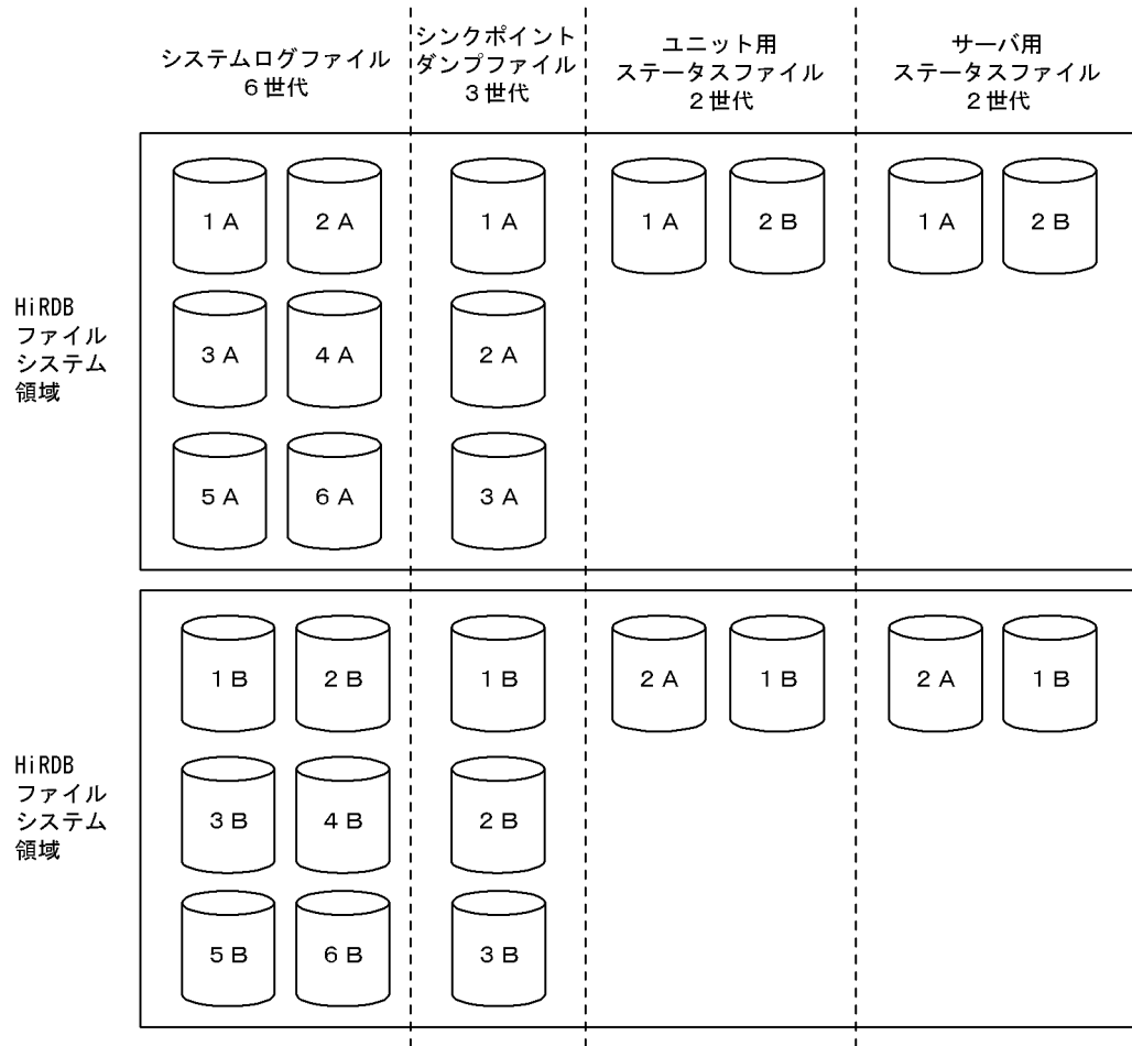
図 4-2 HiRDB が作成するシステムファイルの構成 (2 個指定した場合)
