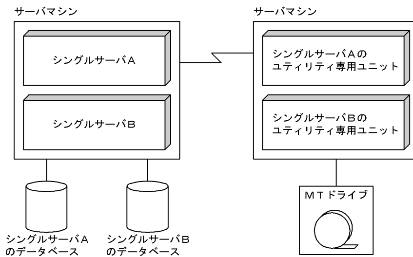
図 11-1 マルチ HiRDB でのユティリティ専用ユニットの設置例 (HiRDB ごとにユティリティ専用ユニットを持つシステム構成)
