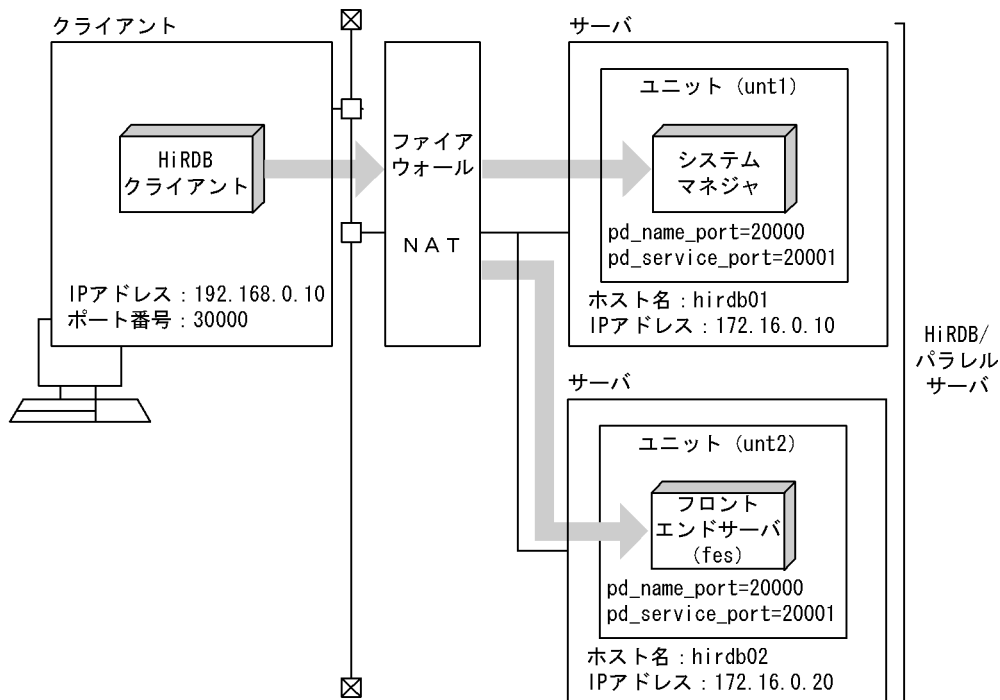
図 25-11 ファイアウォールと NAT が HiRDB/パラレルサーバ側に設置されているネットワーク構成例
