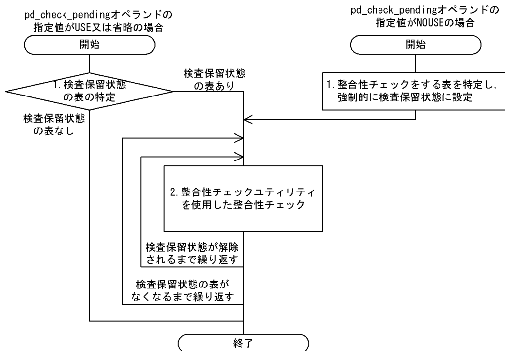
図 13-37 データの整合性確認手順の概要（参照制約）
