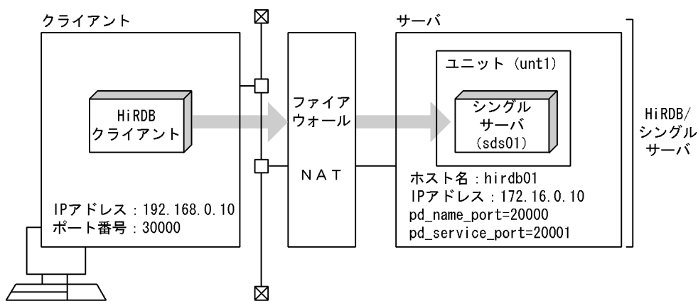
図 25-9 ファイアウォールと NAT が HiRDB/シングルサーバ側に設置されているネットワーク構成例
