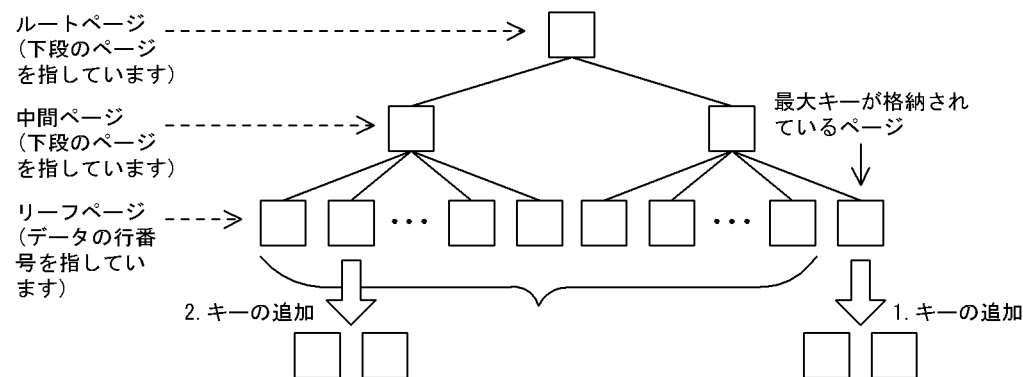
図 18-1 インデクスページスプリットの場合
