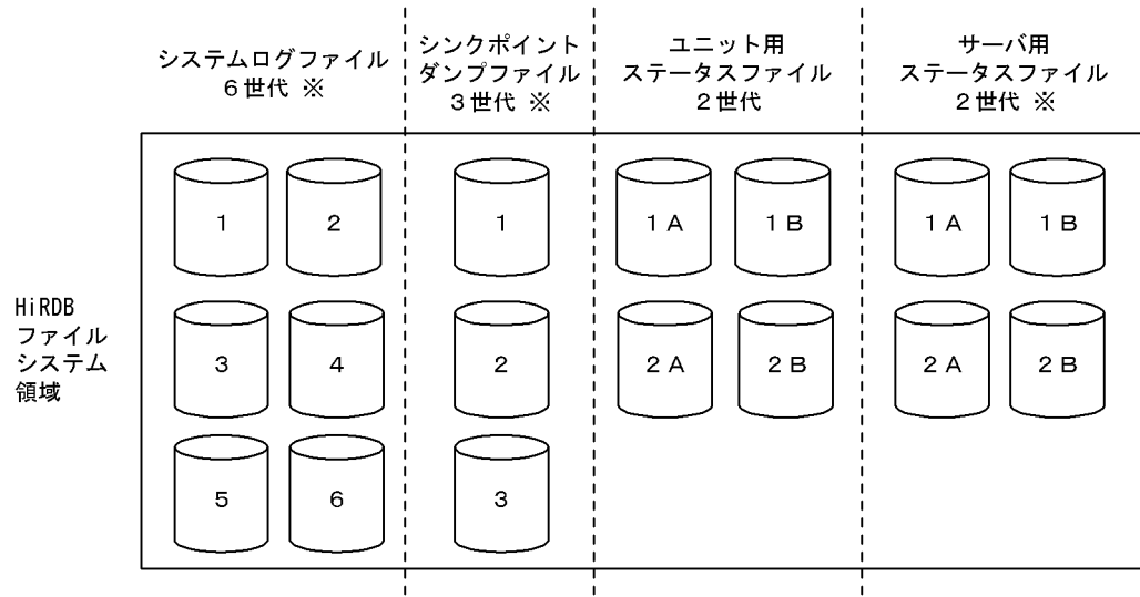
図 4-6 HiRDB が作成するシステムファイルの構成 (1 個指定した場合)
