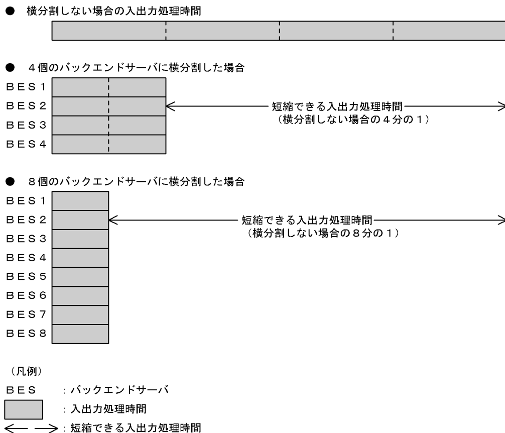
図 13-12 表を横分割するバックエンドサーバの数に伴う入出力処理性能の概要
