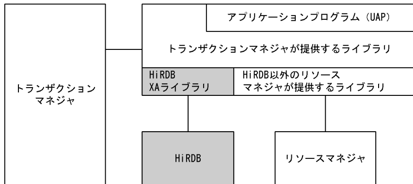
図 8-1 X/Open DTP モデルでの HiRDB の位置づけ
