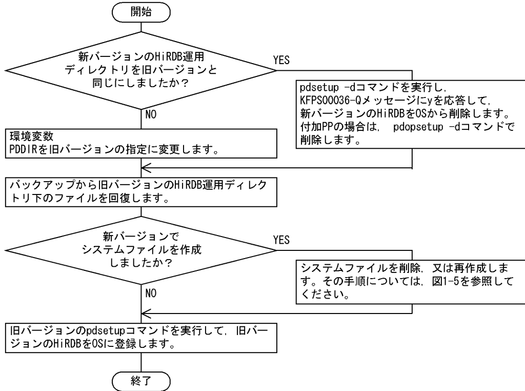
図 1-4 HiRDB を旧バージョンに戻す手順 (バージョンアップに失敗した場合)
