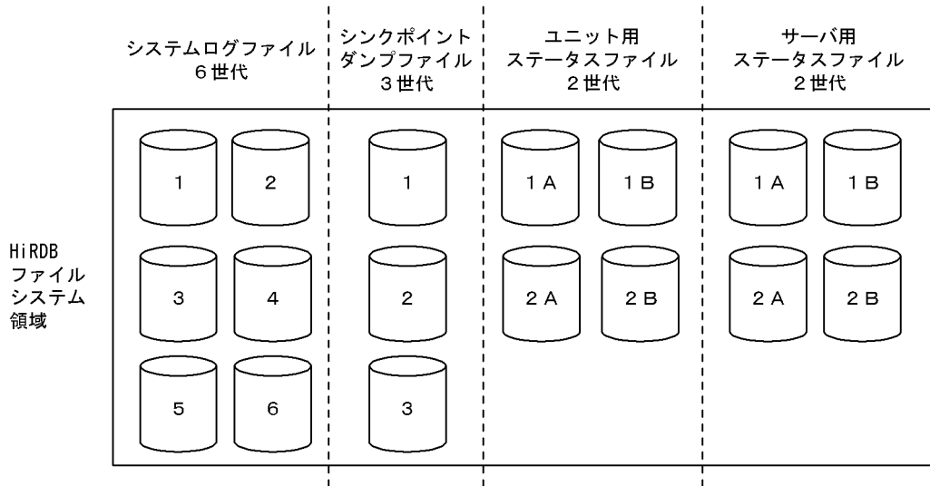
図 4-3 HiRDB が作成するシステムファイルの構成 (1 個指定した場合)
