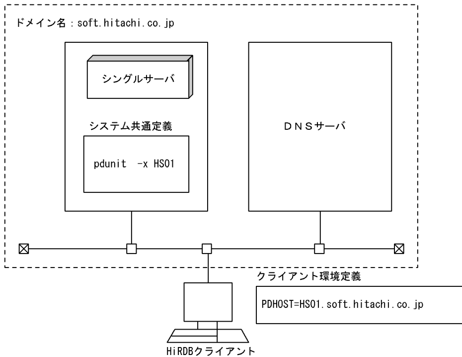
図 25-1 FQDN を指定して HiRDB サーバへ接続する場合のネットワーク構成例と定義例
