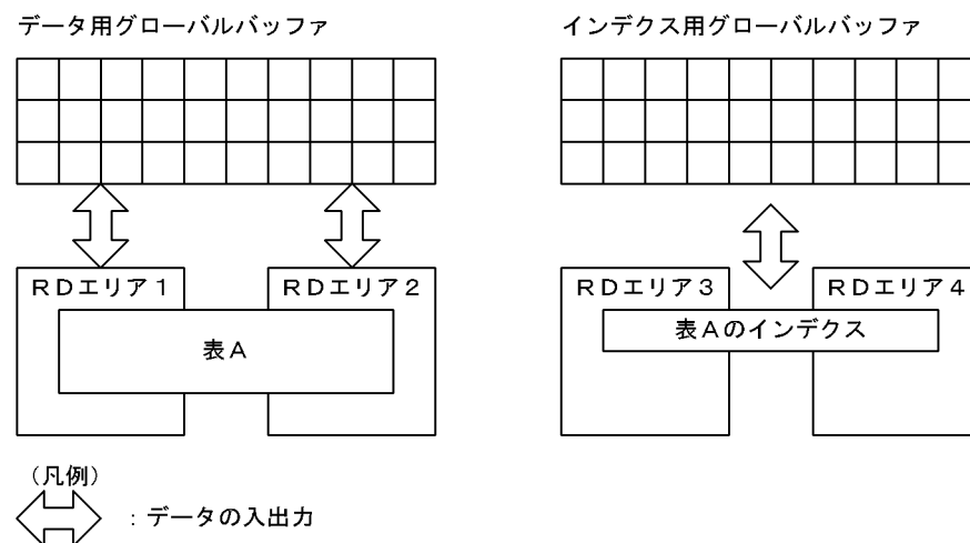
図 12-1 インデクス用グローバルバッファの概要
