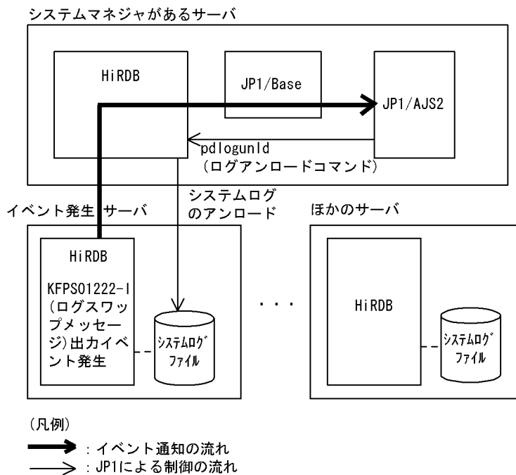
図 8-8 JP1 との連携によるシステムログファイルのアンロード時の自動制御
