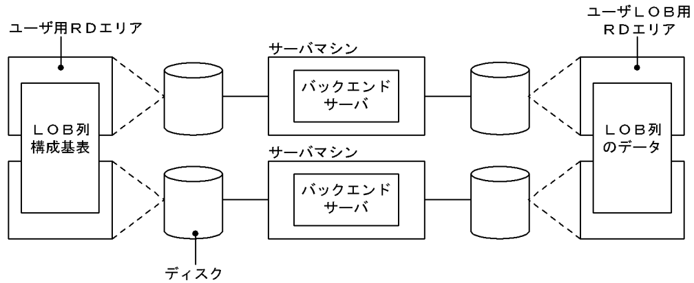
図 10-11 ユーザ LOB 用 RD エリアの配置例 (HiRDB/パラレルサーバの場合)
