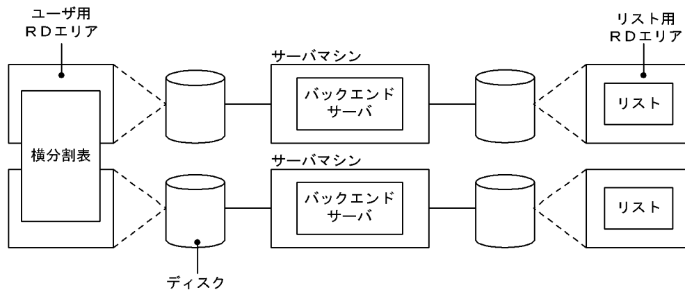
図 10-12 リスト用 RD エリアの配置例 (HiRDB/パラレルサーバの場合)
