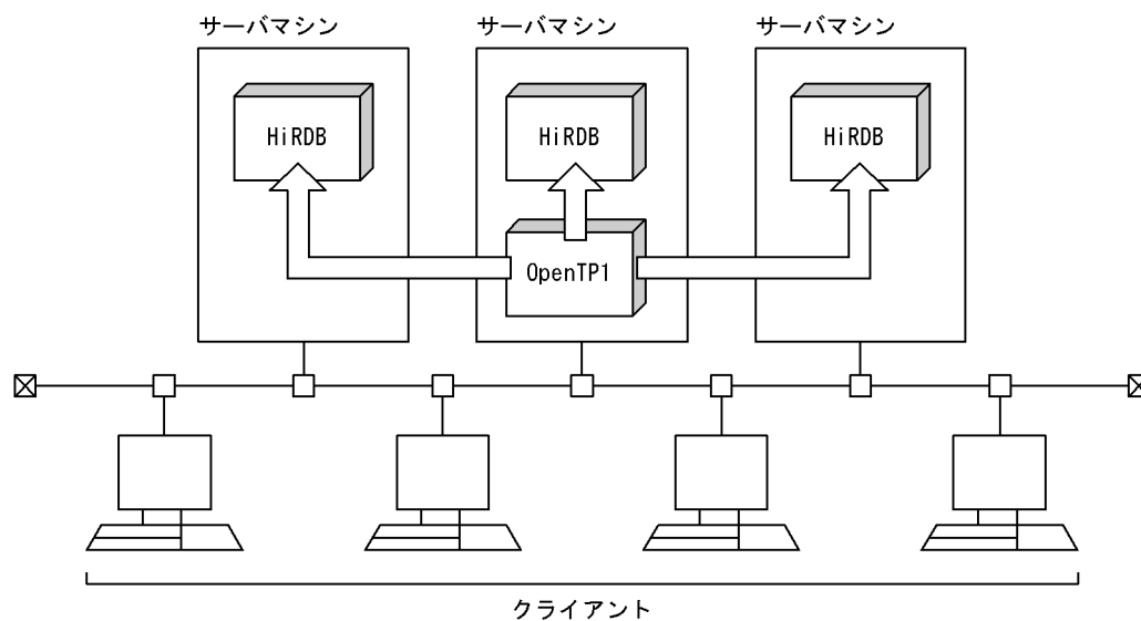
図 8-5 一つの OLTP (OpenTP1) と複数の HiRDB との連携
