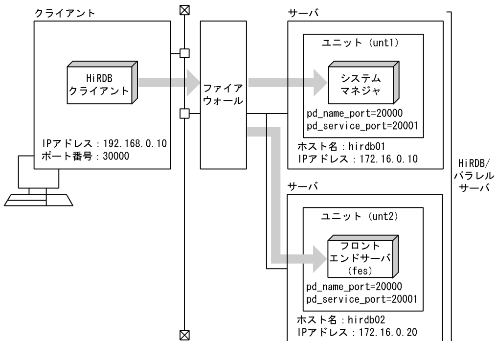
図 25-10 ファイアウォールが HiRDB/パラレルサーバ側に設置されているネットワーク構成例
