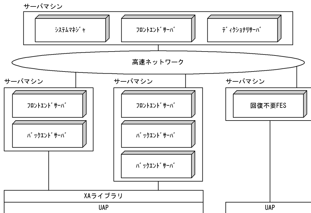
図 10-4 回復不要 FES を使用したシステムの構成例
