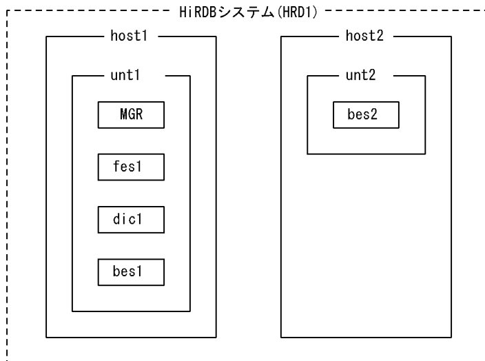
図 24-3 HiRDB/パラレルサーバの場合の構成
