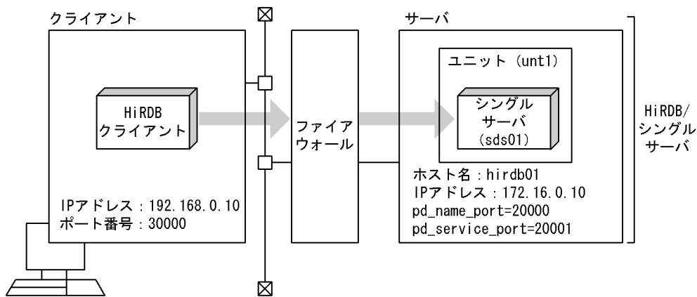
図 25-8 ファイアウォールが HiRDB/シングルサーバ側に設置されているネットワーク構成例
