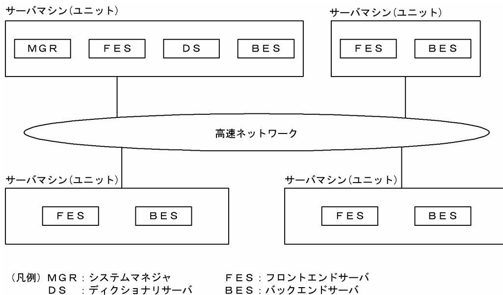
図 4-7 システムジェネレータが作成するシステム構成例
