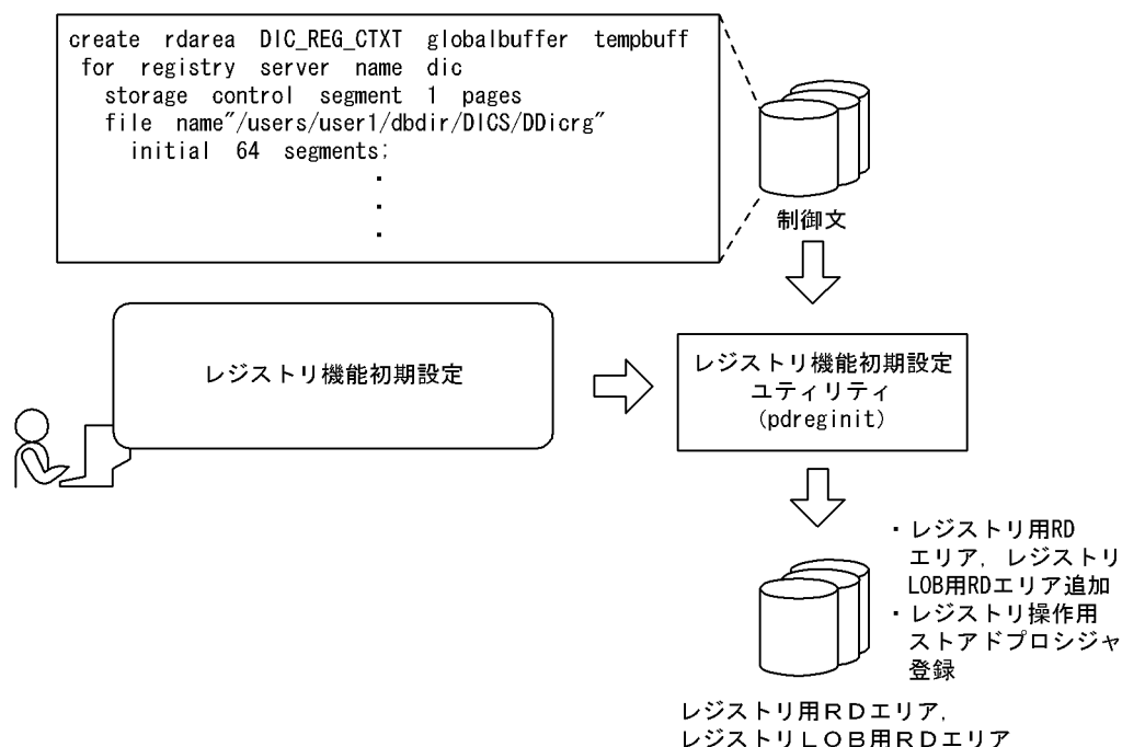
図 6-3 レジストリ用 RD エリア、レジストリ LOB 用 RD エリアの作成の手順
