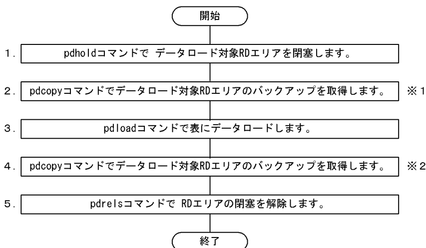
図 7-2 データベースの更新ログ取得方式による運用方法の違い (データロード)
