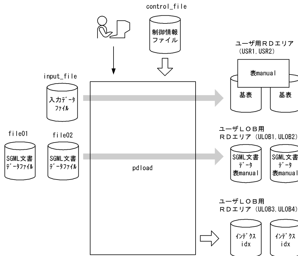
図 23-4 pdload の概要
