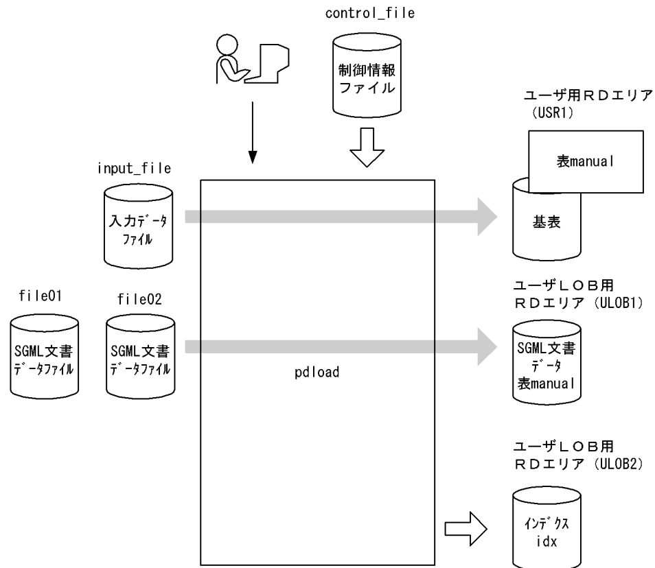
図 22-4 pdload の概要
