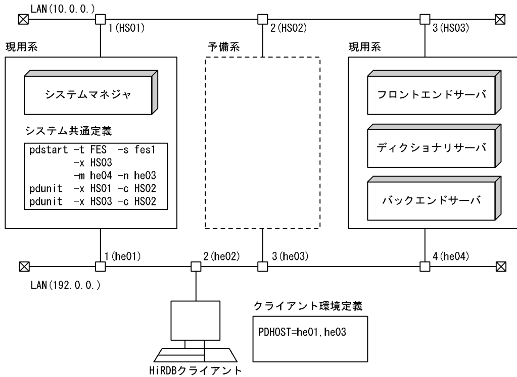
図 25-5 ネットワーク構成例と定義例 (IP アドレスを引き継がない系切り替えをする場合)
