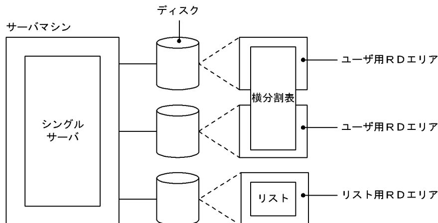
図 9-10 リスト用RDエリアの配置例 (HiRDB/シングルサーバの場合)
