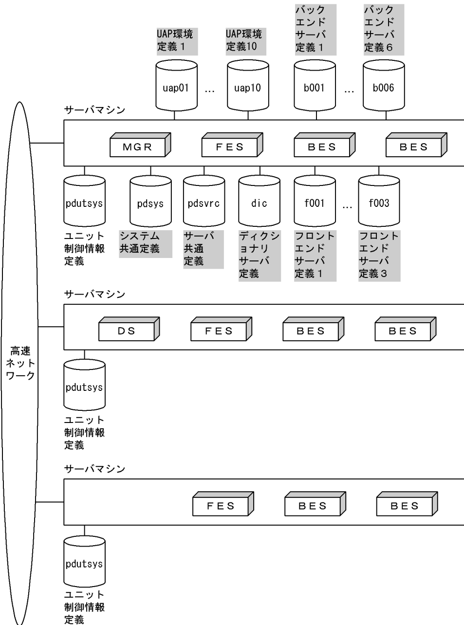
図 5-5 HiRDB システム定義ファイルの共用化
