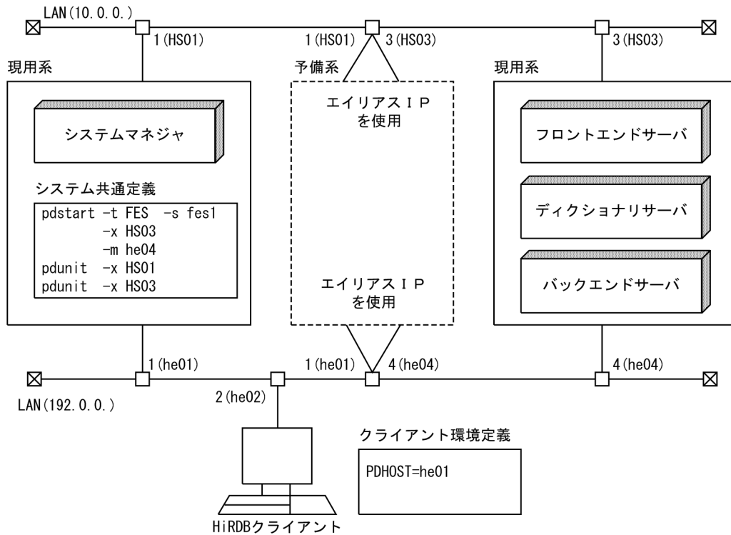
図 25-4 ネットワーク構成例と定義例 (IP アドレスを引き継ぐ系切り替えをする場合)
