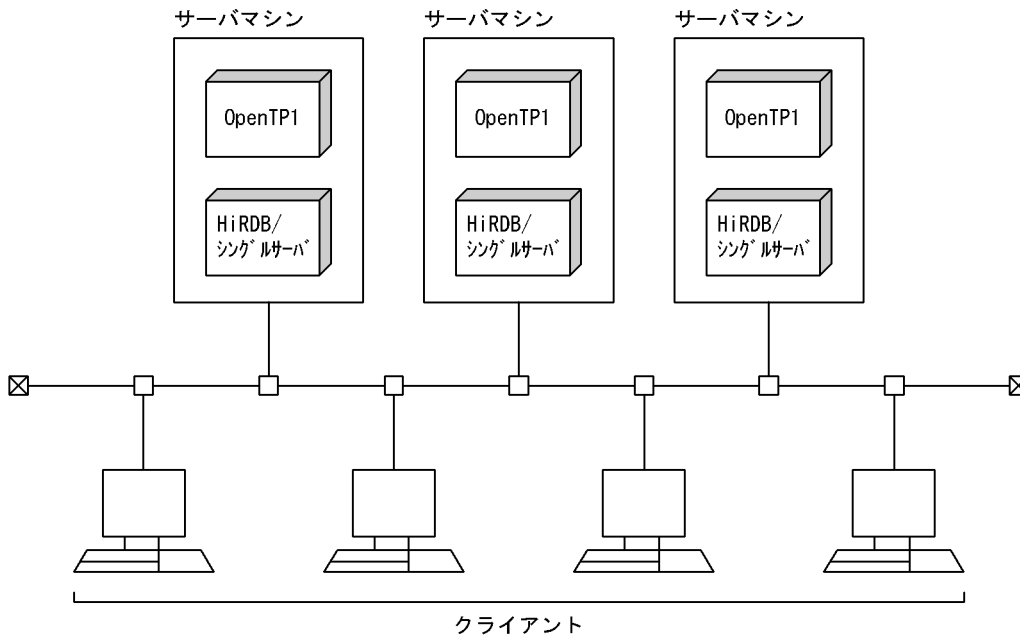
図 8-2 HiRDB/シングルサーバと OLTP (OpenTP1) との連携
