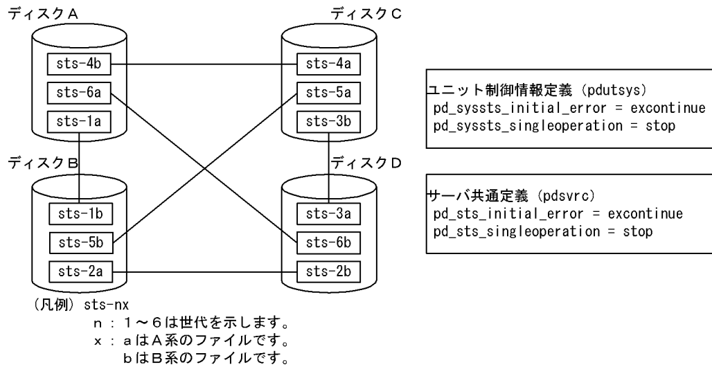
図 10-7 四つのディスクに 6 組のステータスファイルを配置する例
