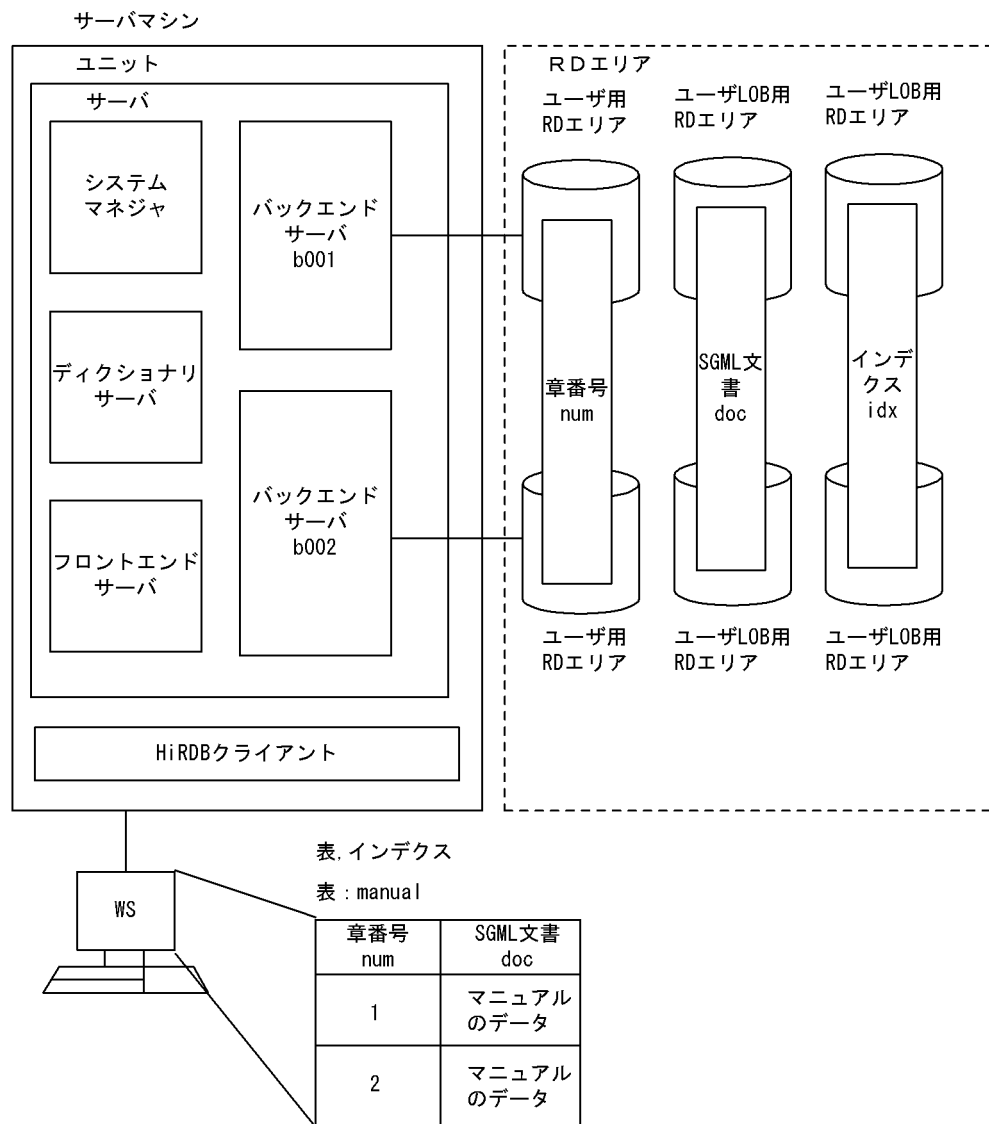
図 23-1 簡易導入で構築する HiRDB の構成
