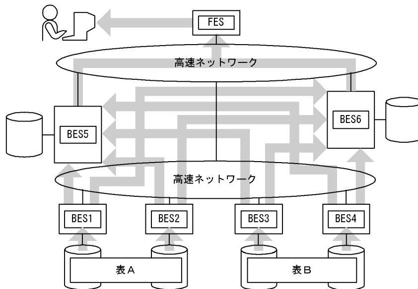
図 13-29 共用表を使用しない結合処理
