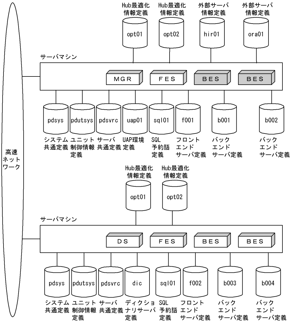
図 5-4 HiRDB システム定義ファイルの構成例 (HiRDB External Data Access 機能を使用する場合)
