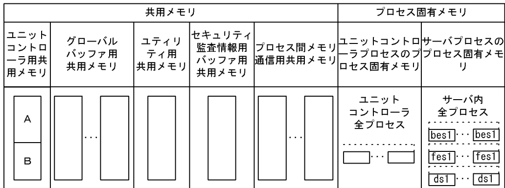
図 16-2 HiRDB/パラレルサーバの各ユニットのメモリ配置
