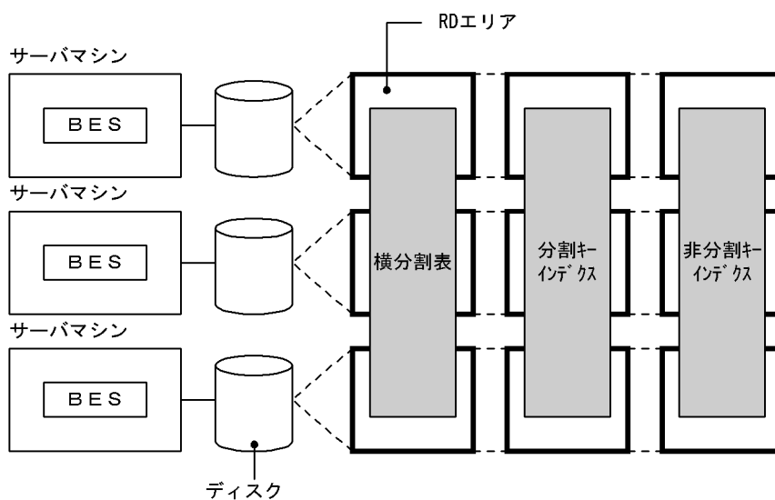
図 14-5 インデクスの横分割の例（サーバ間横分割の場合）
