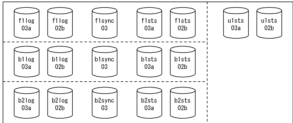
HiRDBファイルシステム領域 (/sysarea03)
