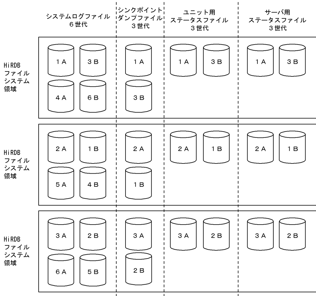
図 4-1 HiRDB が作成するシステムファイルの構成 (3 個指定した場合)
