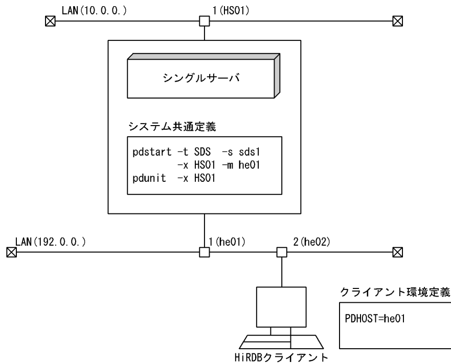
図 25-2 ネットワーク構成例と定義例 (HiRDB/シングルサーバの場合)
