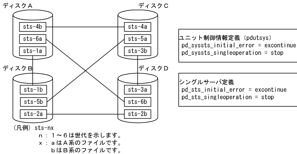
図 9-5 四つのディスクに 6 組のステータスファイルを配置する例
