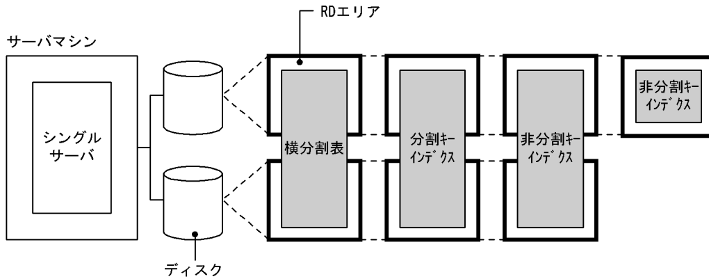
図 14-3 インデクスの横分割の例 (HiRDB/シングルサーバの場合)
