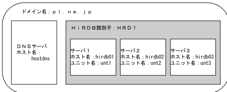
図 25-6 同一ドメインのシステム構成例
