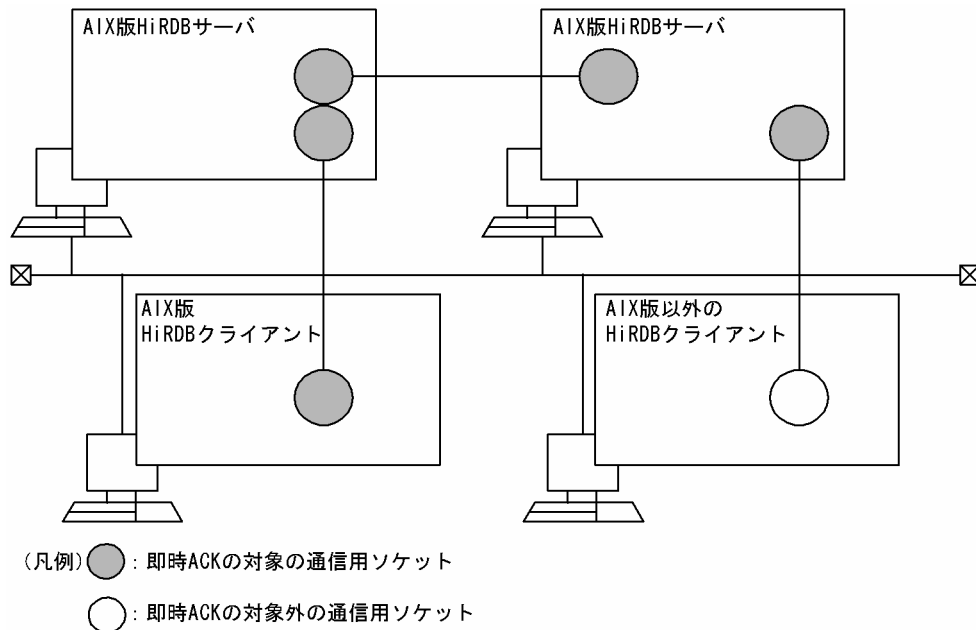
図 25-12 即時 ACK の対象
