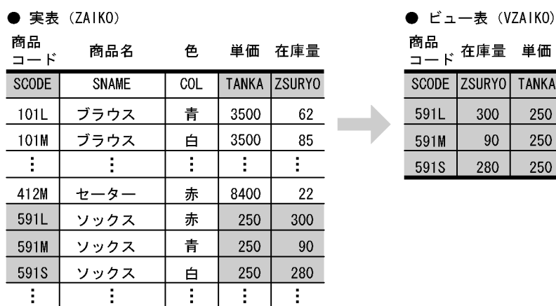
図 13-18 実表とビュー表の関係
