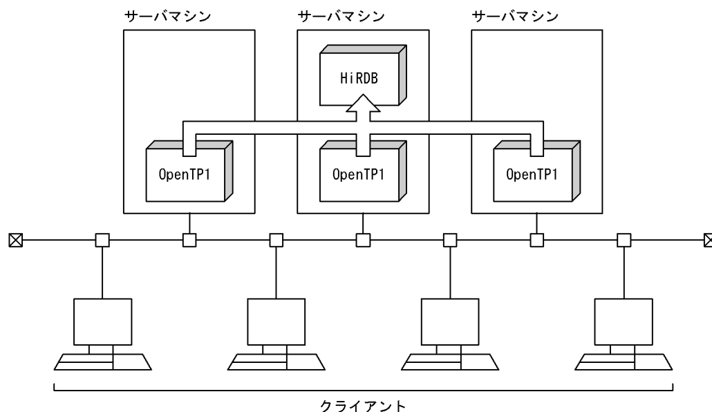
図 8-4 複数の OLTP (OpenTP1) と HiRDB との連携
