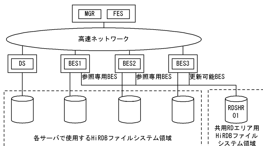
図 15-5 共用 RD エリアの概要
