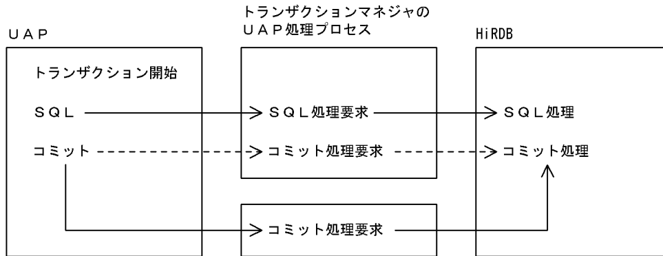
図 8-6 トランザクションの移行の概要
