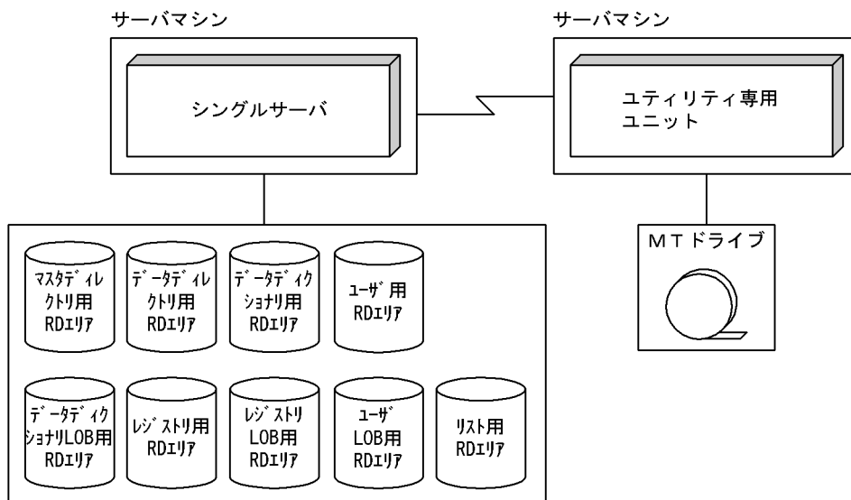
図 9-2 HiRDB/シングルサーバのシステム構成 (ユーティリティ専用ユニットを設置する場合)
