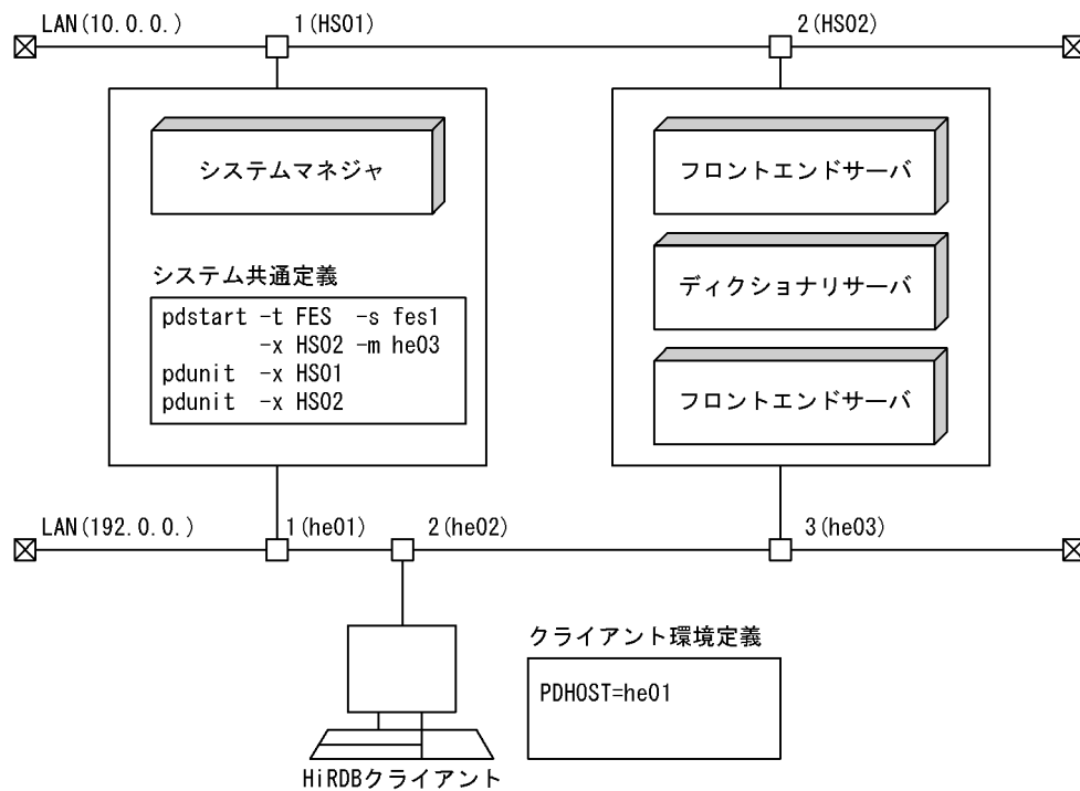
図 25-3 ネットワーク構成例と定義例 (HiRDB/パラレルサーバの場合)
