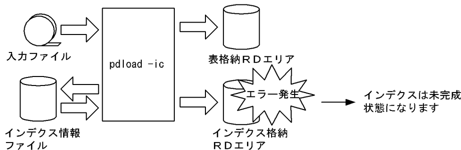
図 7-5 データベース作成ユーティリティ (pdload) でインデクス一括作成中にエラーが発生した場合のインデクスの状態
