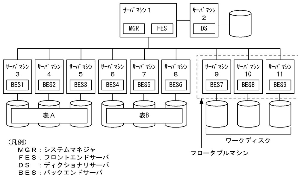
図 13-14 複雑な検索処理を考慮した横分割のシステム構成
