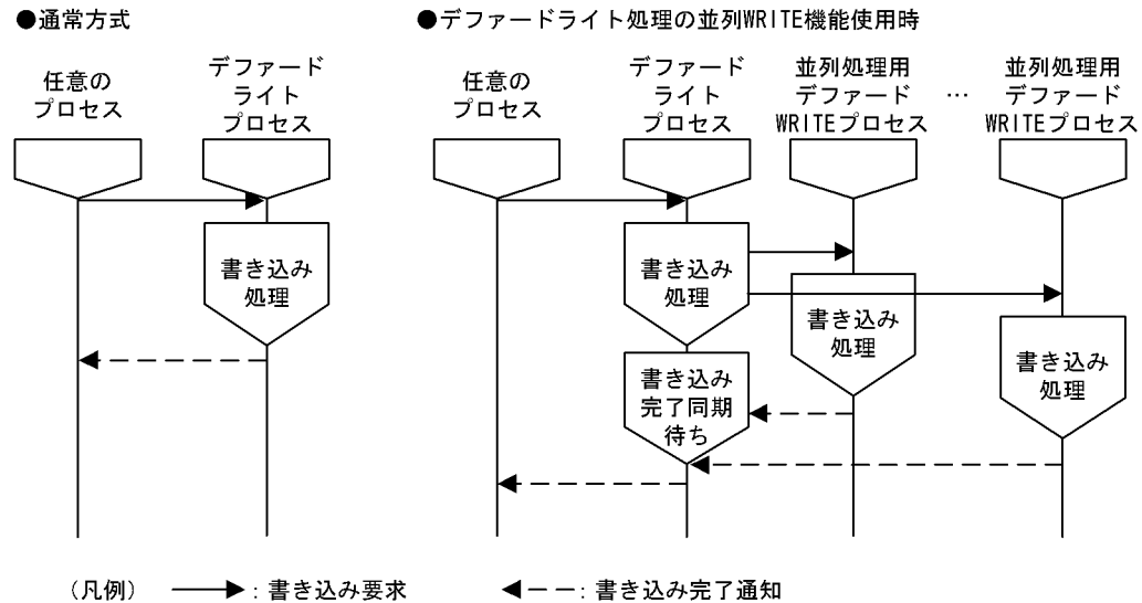
図 12-3 デファードライト処理の並列 WRITE 機能の概要
