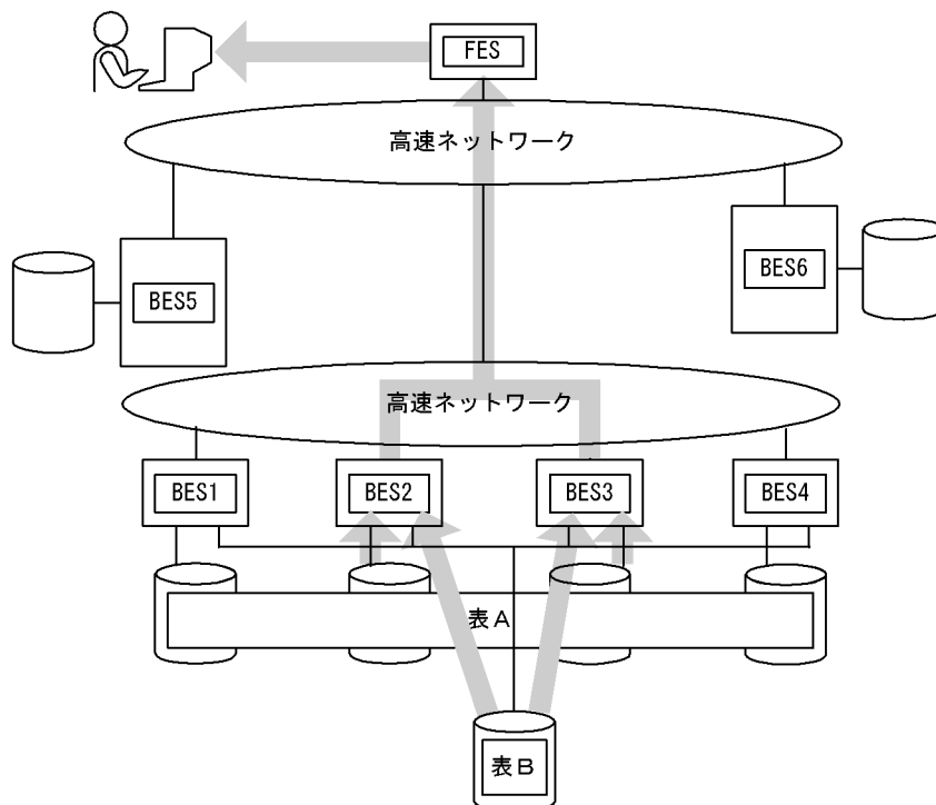
図 13-30 共用表を使用した結合処理
