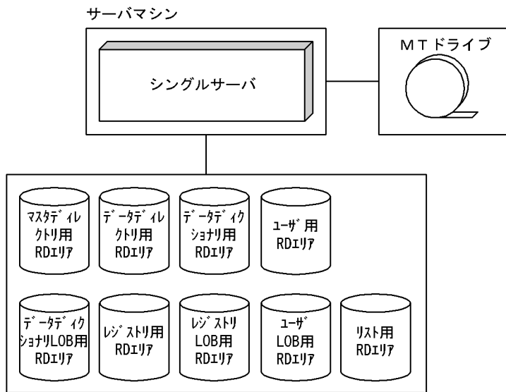
図 9-2 HiRDB/シングルサーバのシステム構成 (ユーティリティ専用ユニットを設置する場合)
