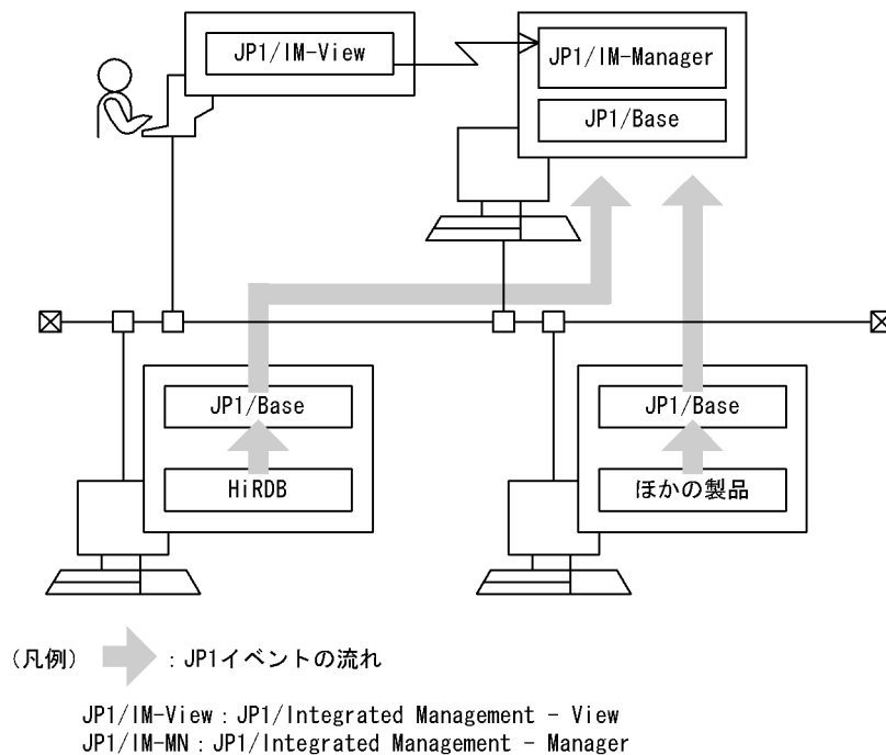
図 8-7 JP1/IM によるイベント監視の概要
