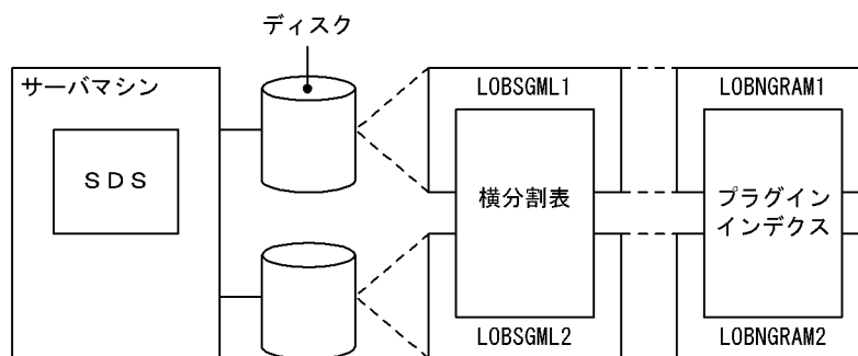
図14-6 プラグインインデクスの横分割の形態 (HiRDB/シングルサーバの場合)
