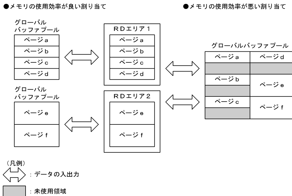
図 12-2 グローバルバッファの割り当ての例
