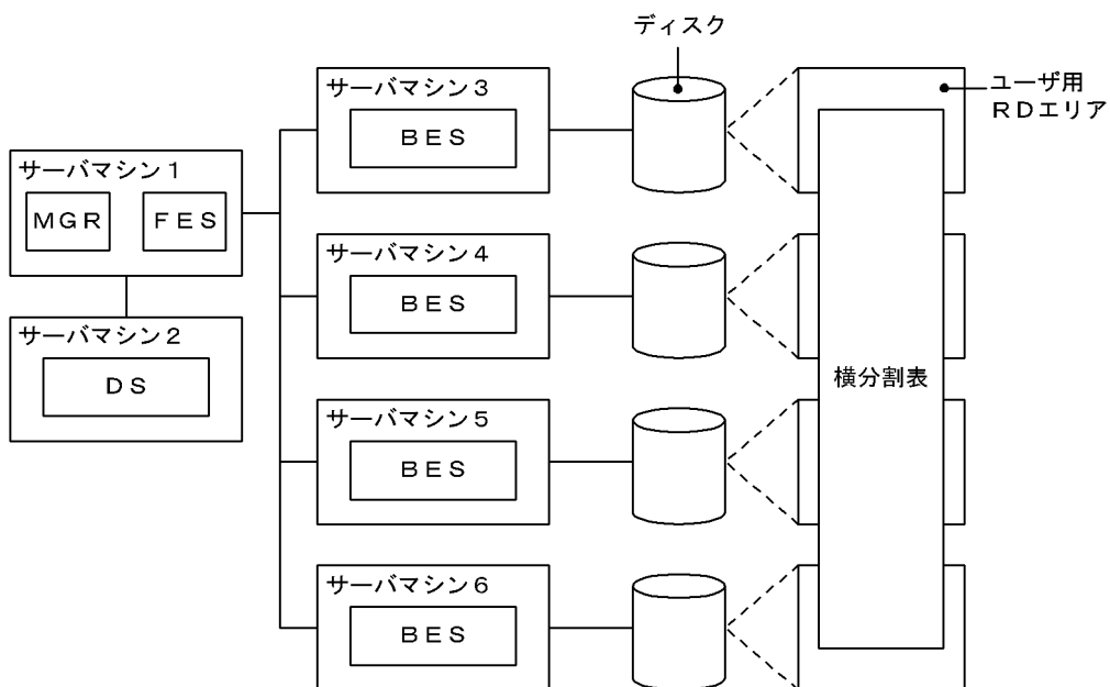
図 13-9 表の横分割の形態 (HiRDB/パラレルサーバの場合)
