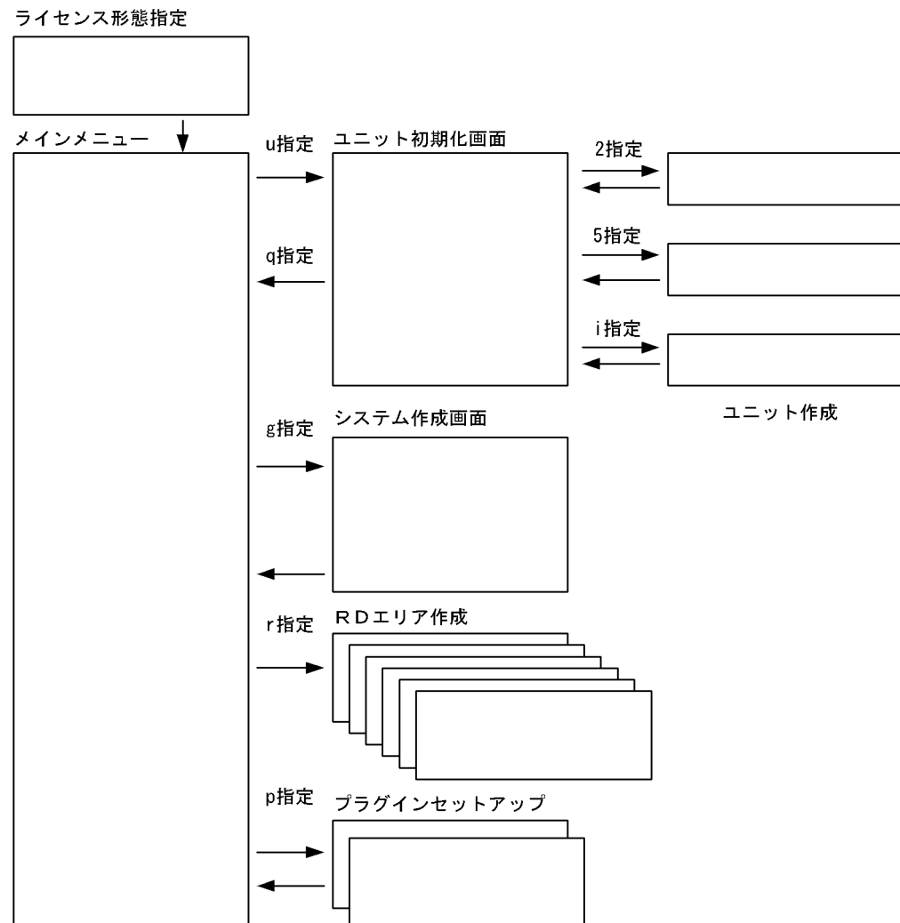
図 23-2 画面の遷移
