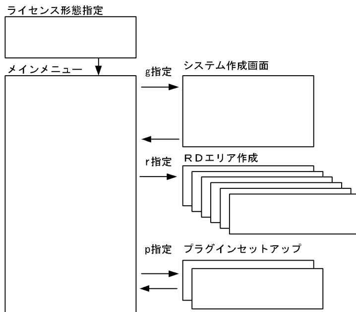
図 22-2 画面の遷移
