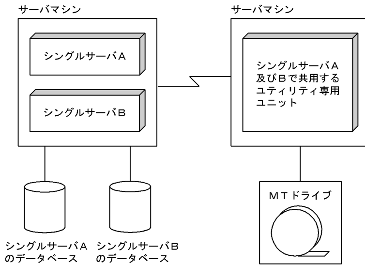
図 11-2 マルチ HiRDB でのユーティリティ専用ユニットの設置例（複数の HiRDB でユーティリティ専用ユニットを共有するシステム構成）
