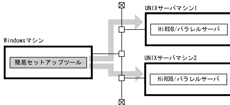
図 3-4 簡易セットアップツールを使用した UNIX 版 HiRDB の環境設定の概要 (HiRDB/パラレルサーバの場合)
