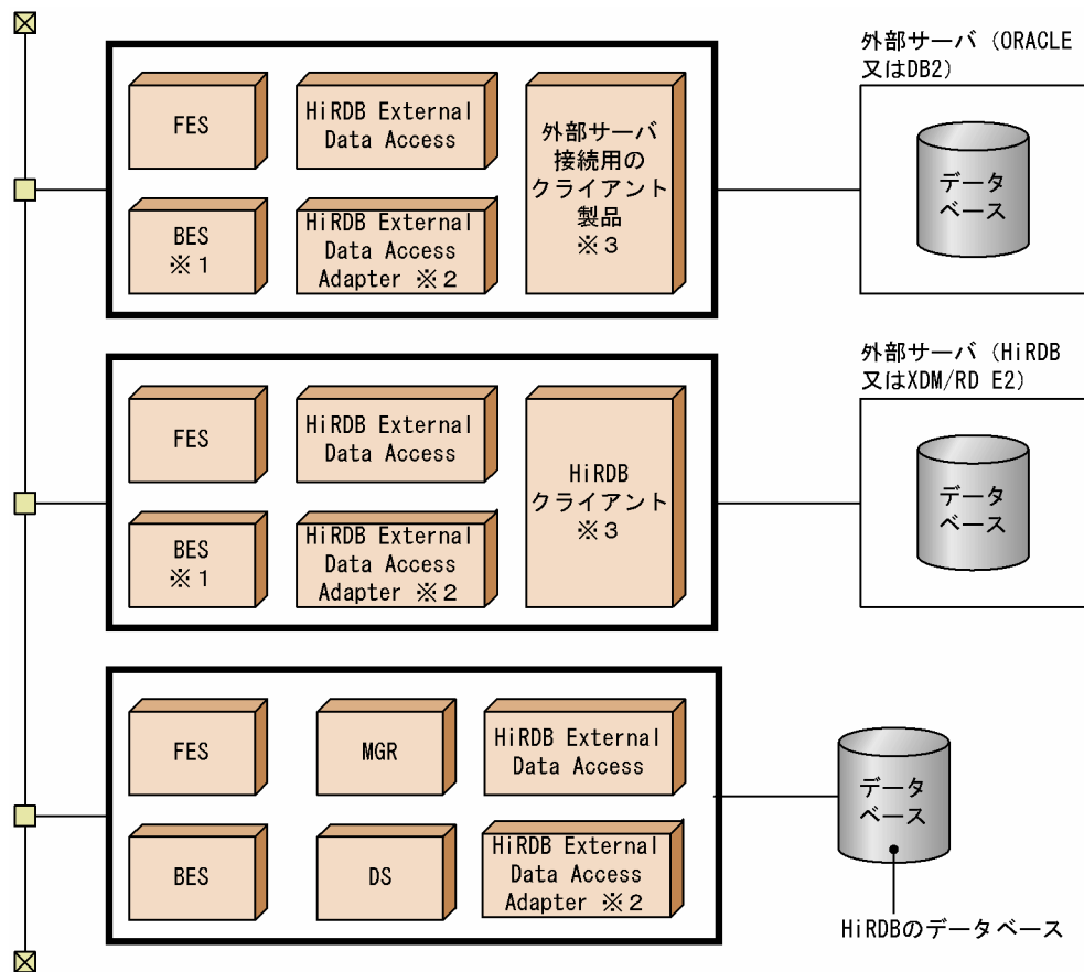
図 2-6 HiRDB External Data Access 機能使用時のシステム構成例
