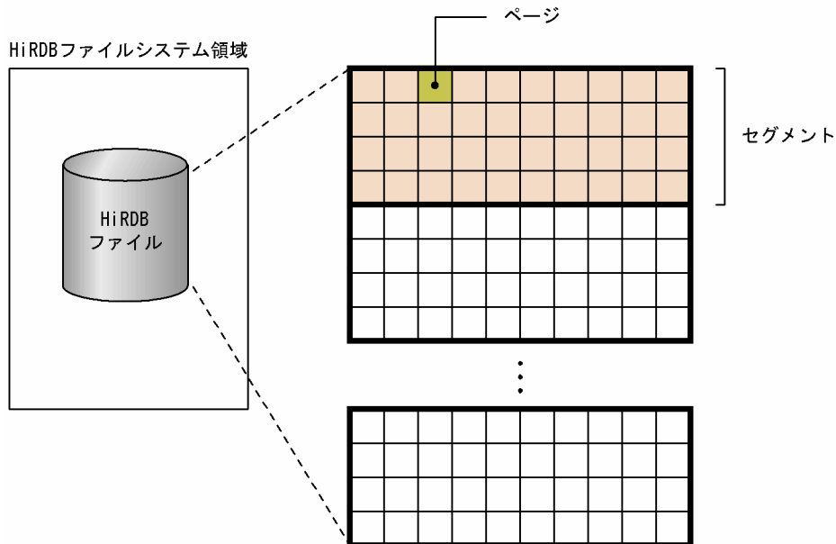
図 4-1 データベースの物理構造
