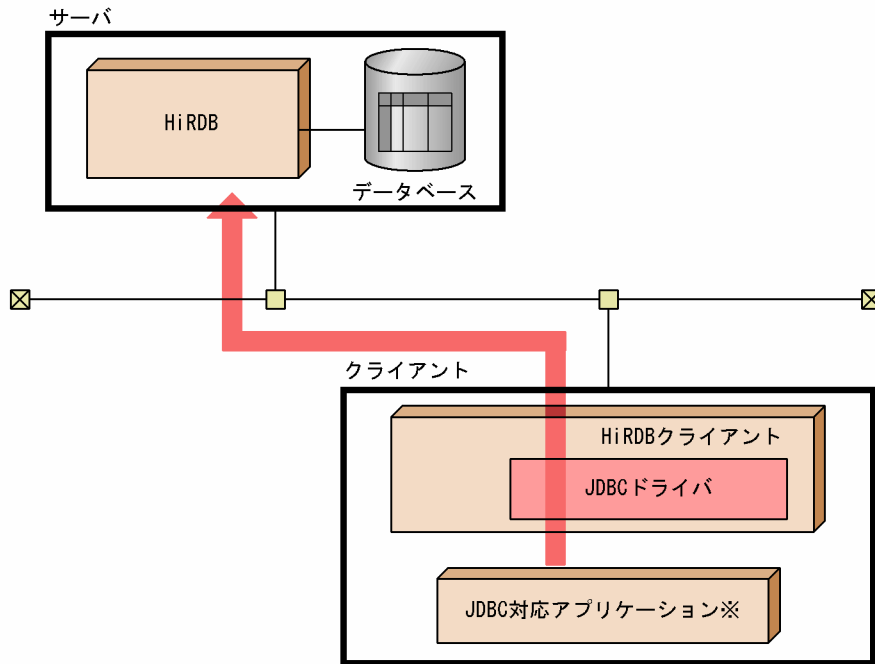
図 1-14 JDBC 対応のアプリケーションからデータベースにアクセスする形態
