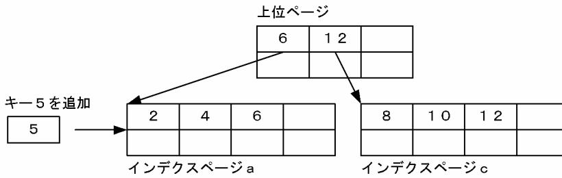
図 3-28 均等に分割するインデクスページスプリットの例
