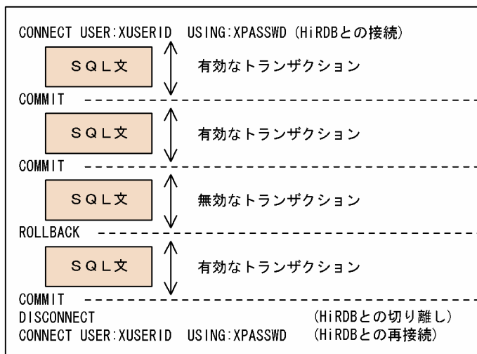
図 6-23 トランザクションの開始と終了の例
