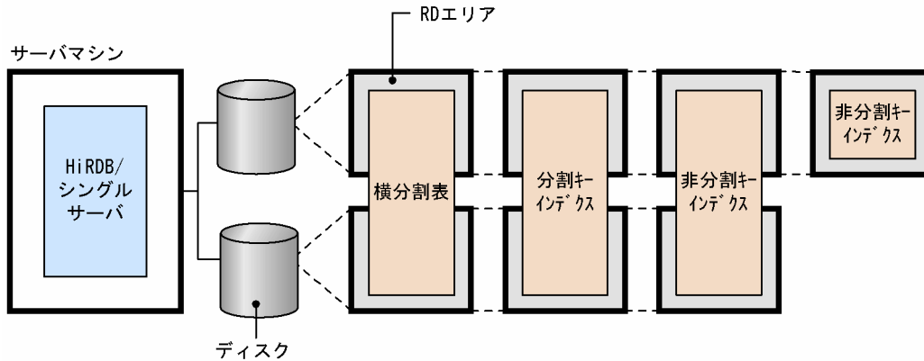
図 3-23 インデクスの横分割の例 (HiRDB/シングルサーバの場合)
