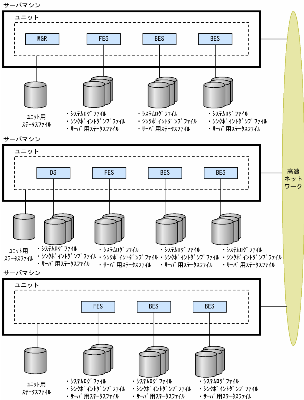
図 6-6 システムファイルの構成 (HiRDB/パラレルサーバの場合)
