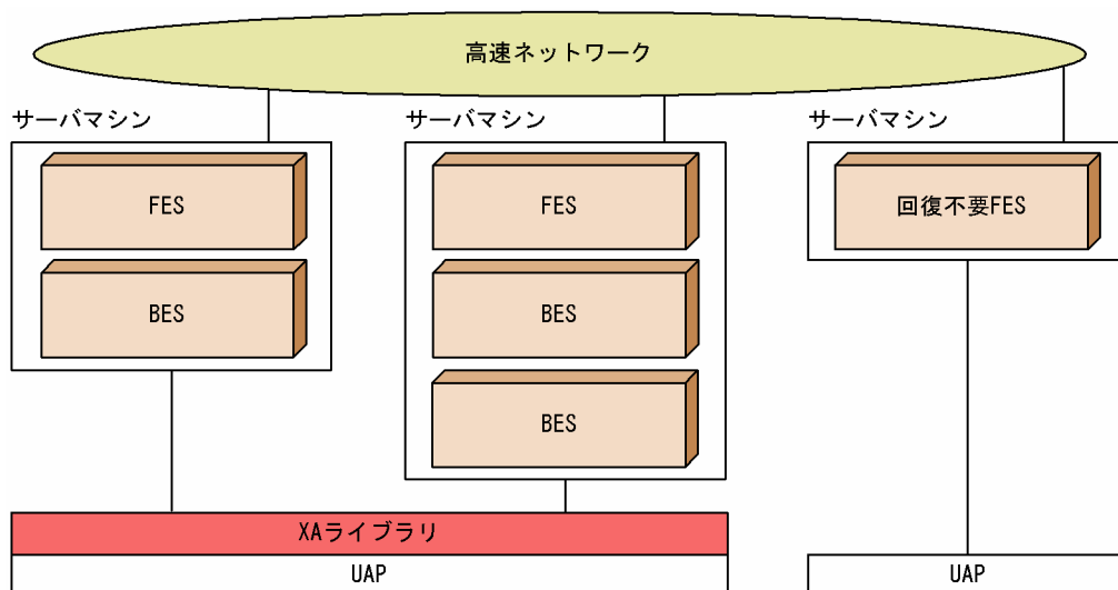
図 8-14 回復不要 FES を使用したシステムの構成例
