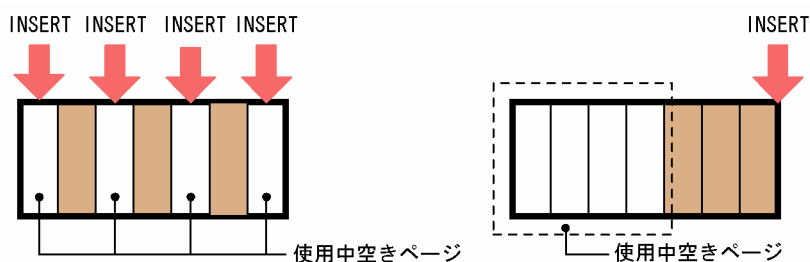
図 7-16 インデクスページに使用中空きページが作成される処理
