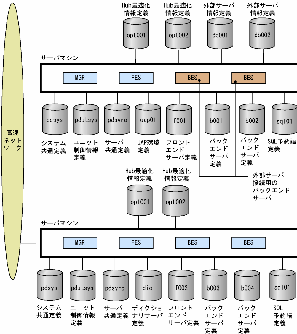
図 6-9 HiRDB システム定義ファイルの構成例 (HiRDB External Data Access 機能を使用する場合)
