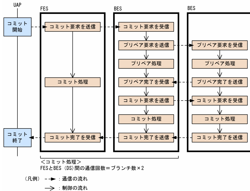
図 6-24 一相コミットの処理方式
