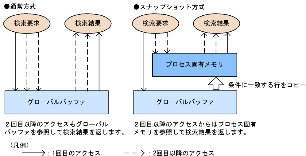
図 6-13 スナップショット方式の概要
