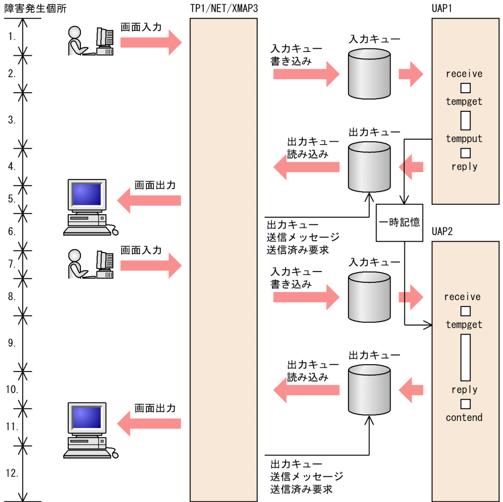
図 11-4 継続問い合わせ応答形態の障害
