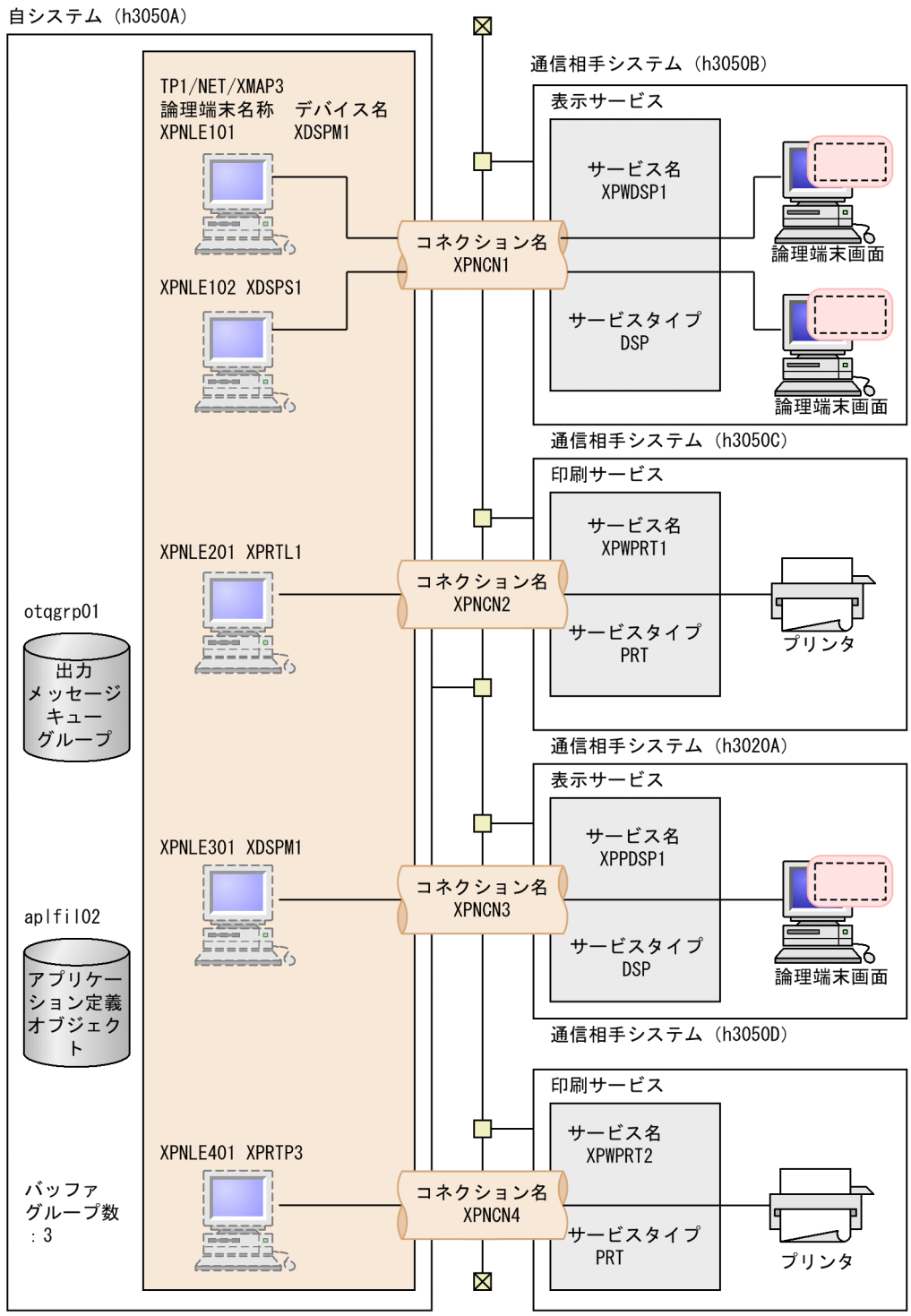
図 7-4 TP1/NET/XMAP3 システム構成例
