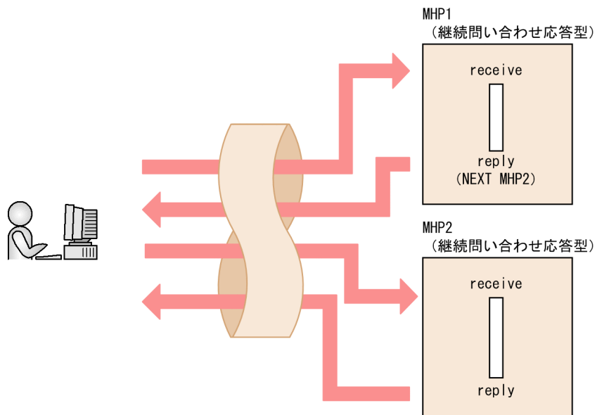
図 2-13 次起動アプリケーションの予約
