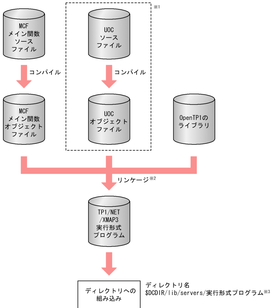
図 10-3 MCF メイン関数のディレクトリへの組み込み方法
