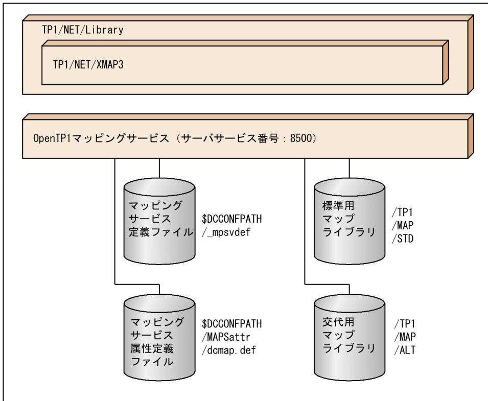
図 6-2 マッピングサービス機能のシステム構成例
