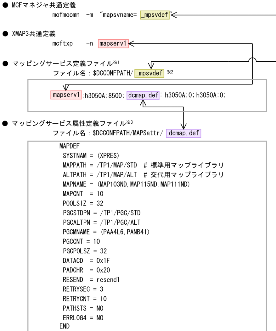
図 6-3 マッピングサービス機能の定義例
