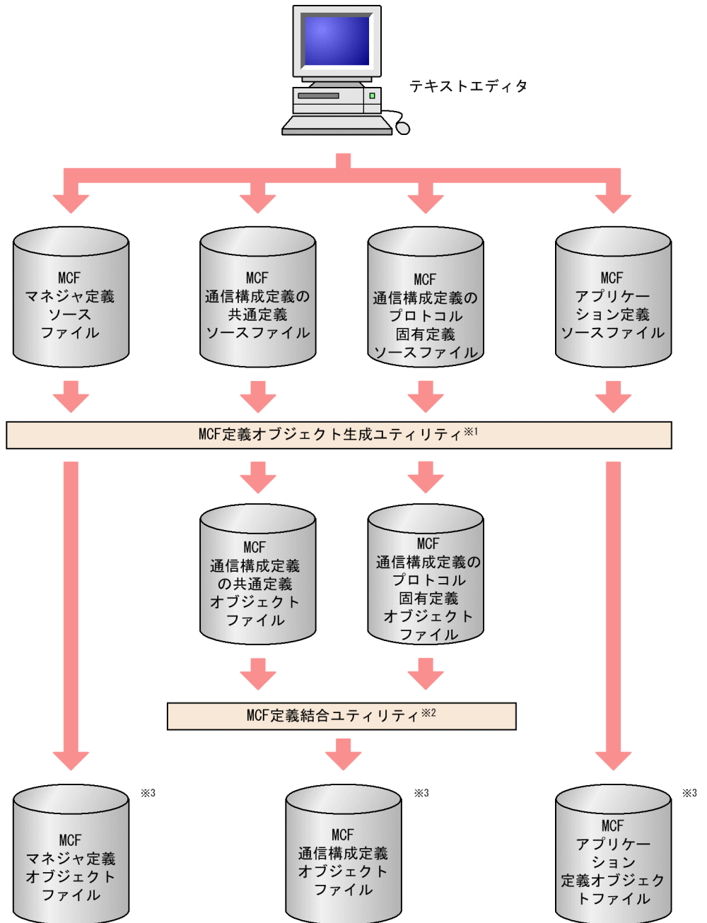
図 10-4 定義オブジェクトファイルの作成方法の概要
