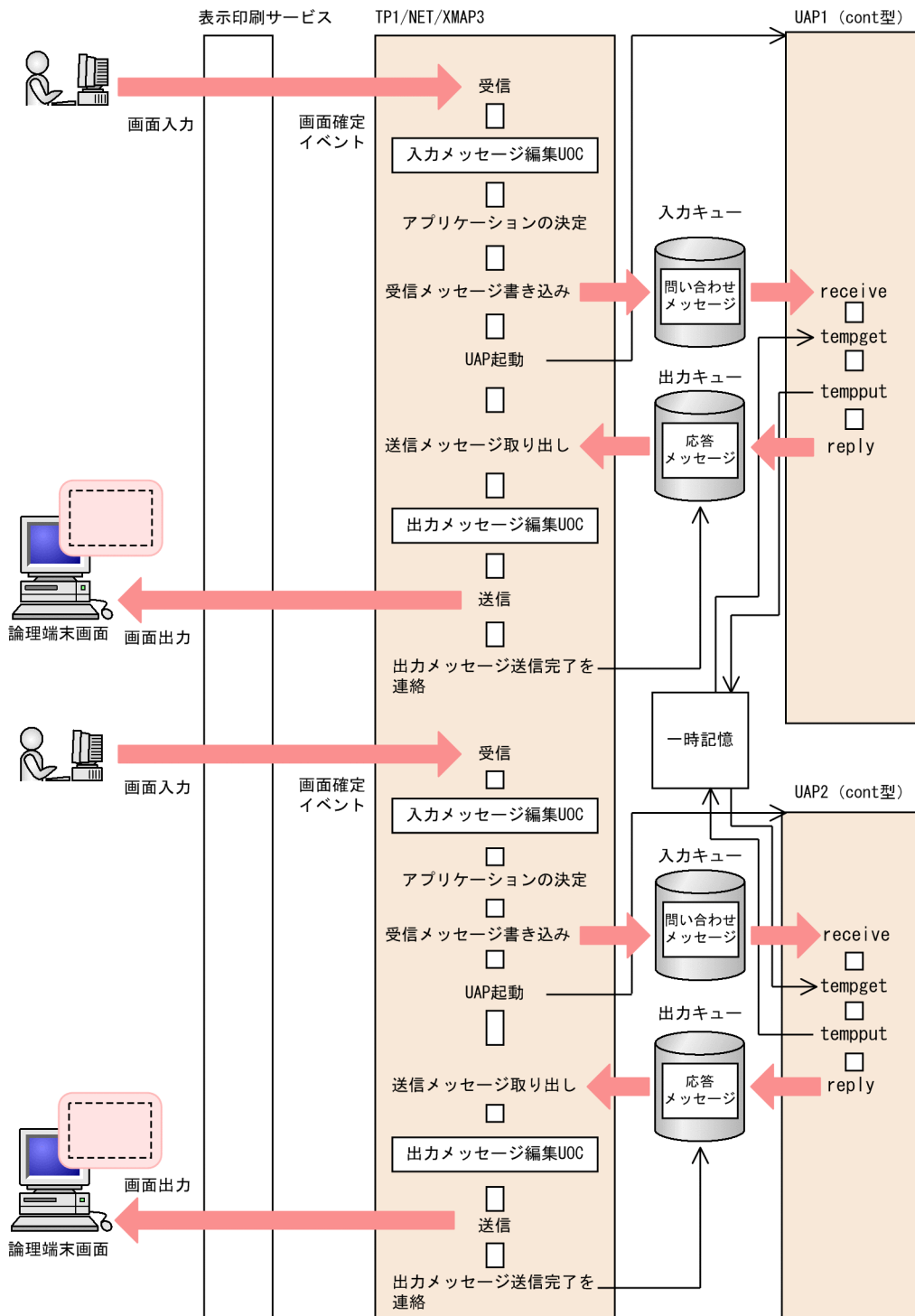
図 2-12 継続問い合わせ応答形態
