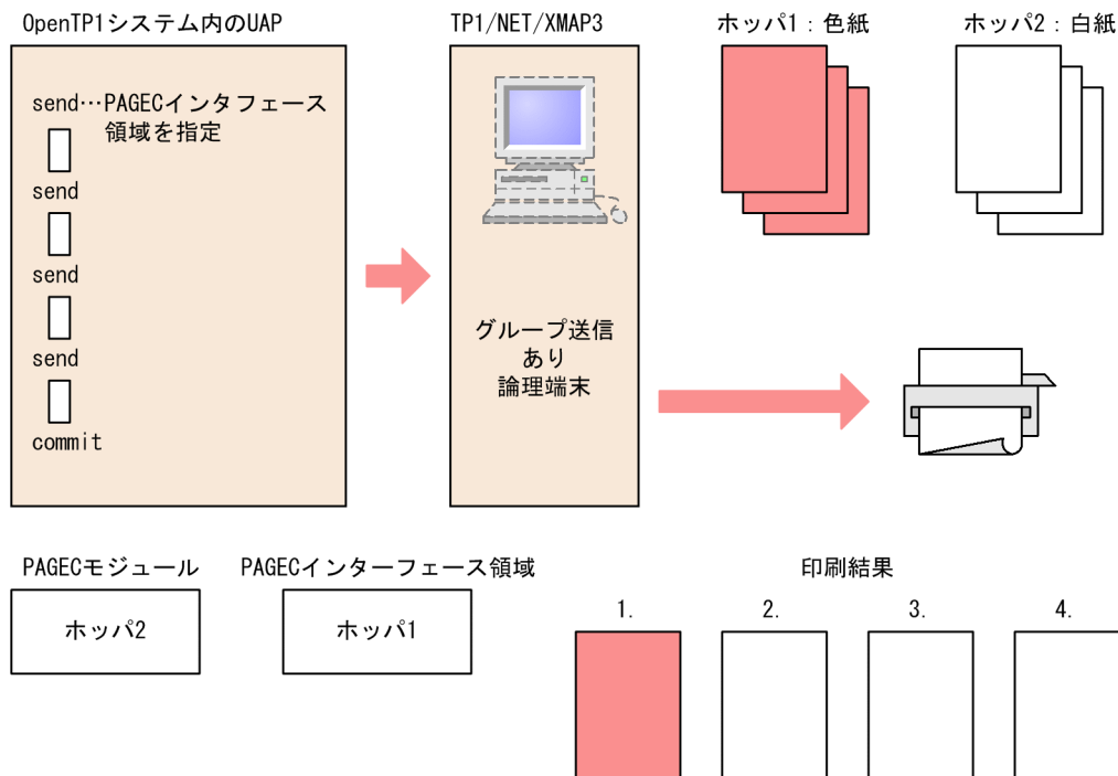
図 2-22 ページ制御機能を利用した印刷
