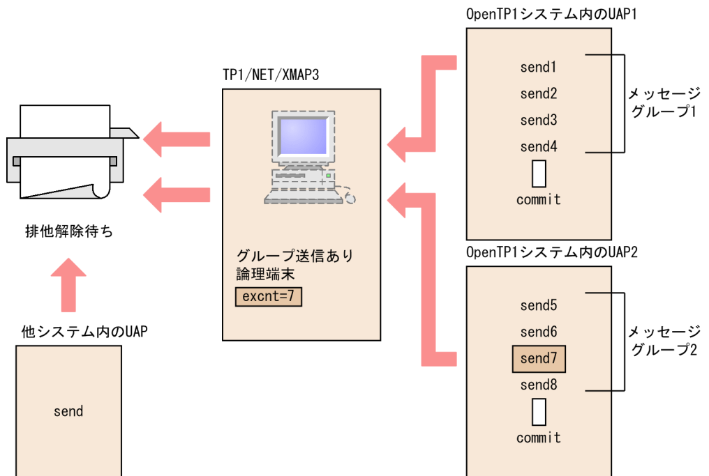
図 2-21 プリンタの連続使用
