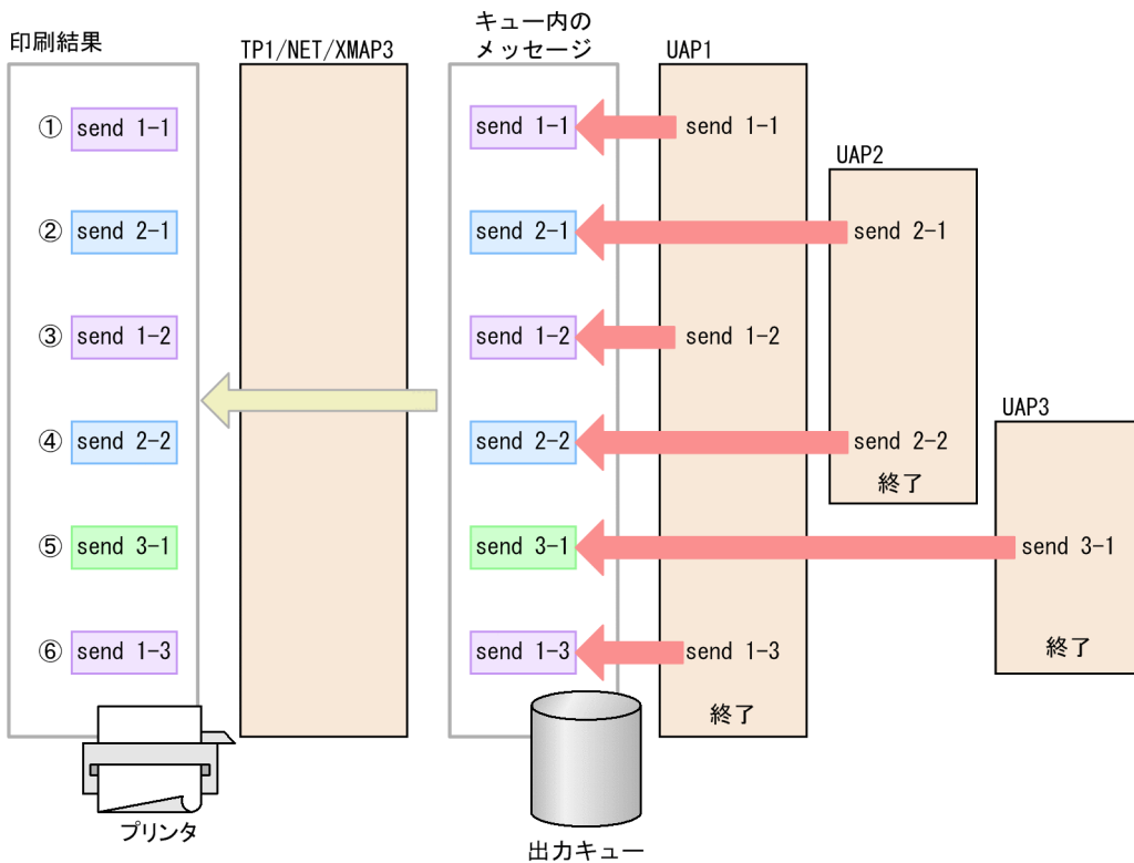
図 2-18 メッセージグループ送信機能を使用しない場合の印刷結果
