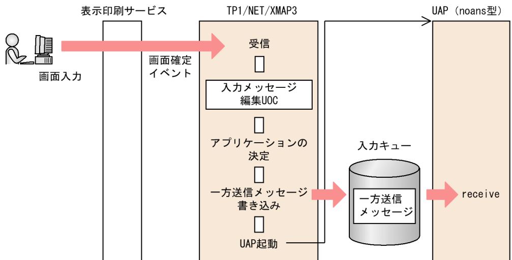
図 2-8 非問い合わせ応答形態
