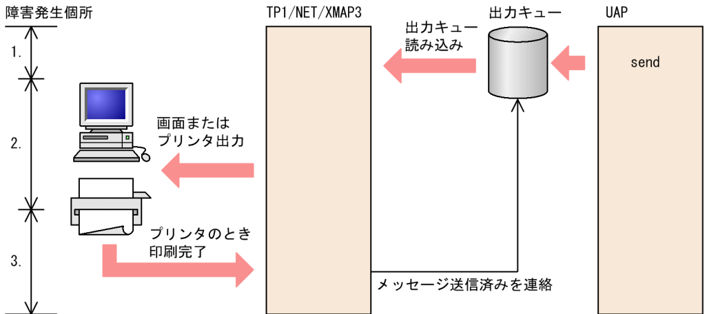
図 11-2 分岐送信形態の障害
