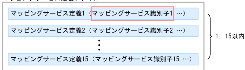
図 7-3 マッピングサービス定義と TP1/NET/XMAP3 固有の定義の関係
