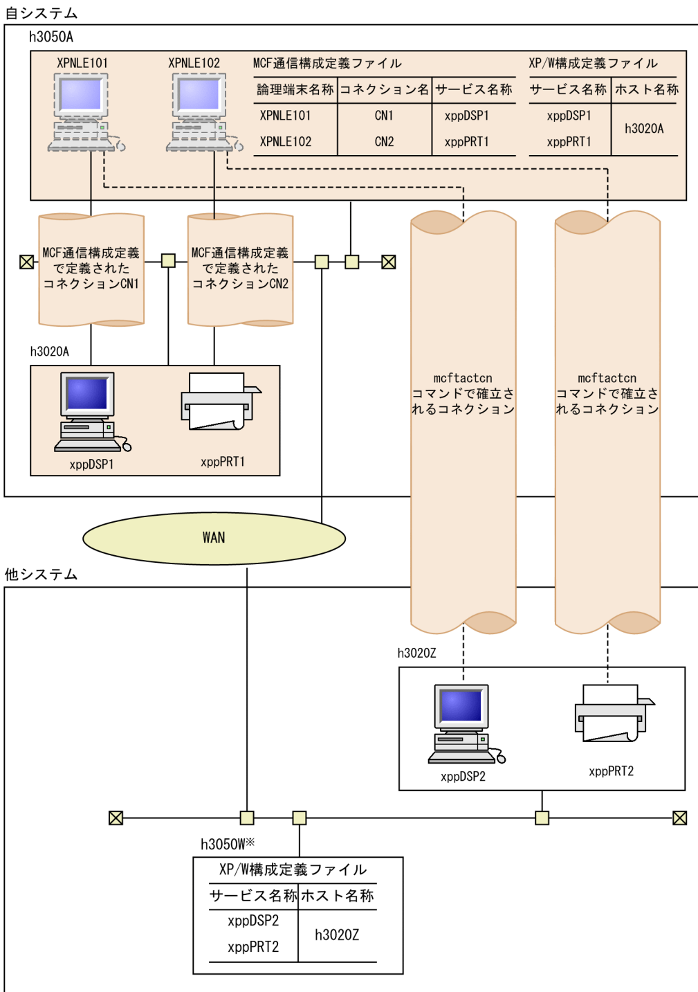
図 2-3 他システムとの接続
