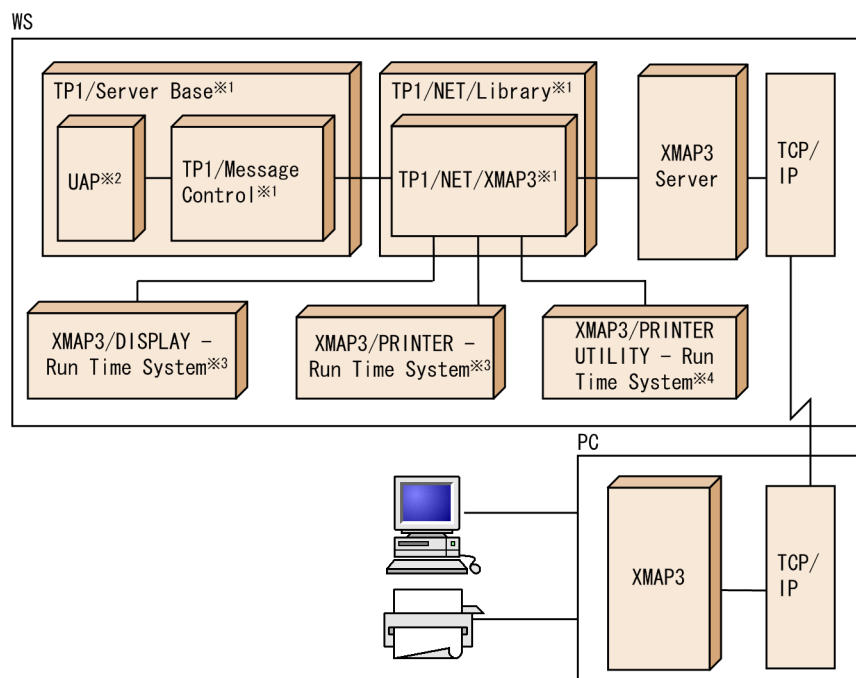
図 1-4 TP1/NET/XMAP3 を組み込んだソフトウェア構成の例
