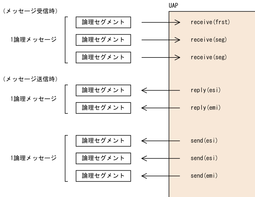
図 2-15 複数セグメントのメッセージ関数の使用方法
