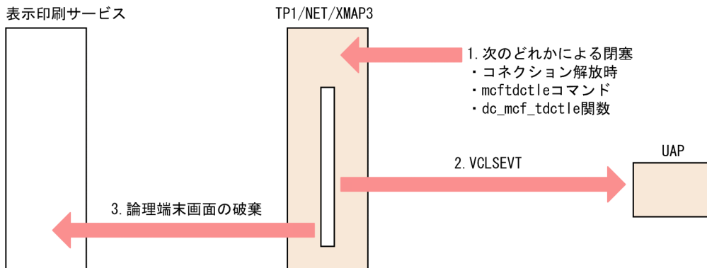
図 2-6 画面属性の端末状態の閉塞処理
