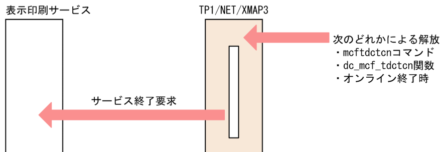
図 2-2 コネクションの解放の流れ
