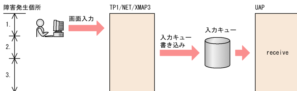
図 11-1 非問い合わせ応答形態の障害
