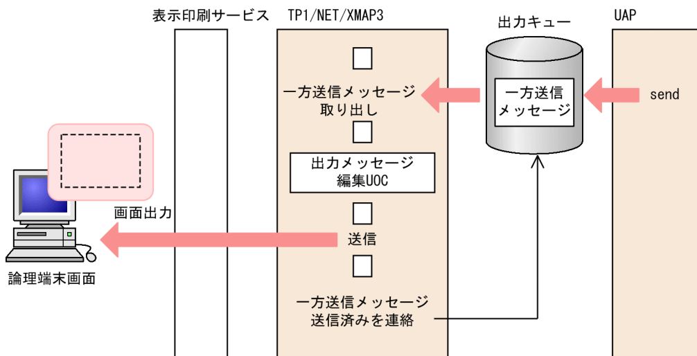
図 2-9 画面に対する分岐送信形態
