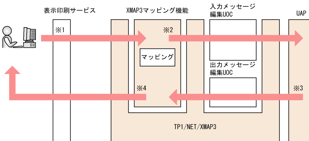
図 2-16 マッピングによるメッセージ編集の流れ
