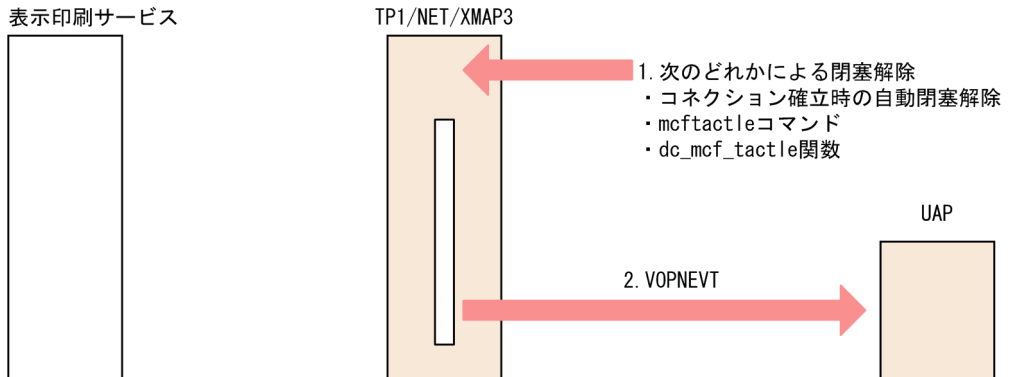
図 2-5 プリンタ属性の端末状態の閉塞解除処理
