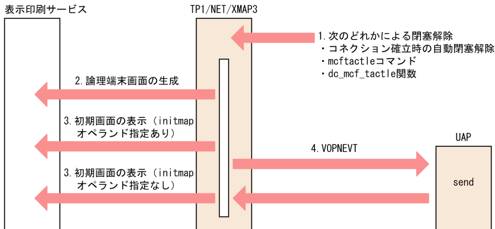
図 2-4 画面属性の端末状態の閉塞解除処理
