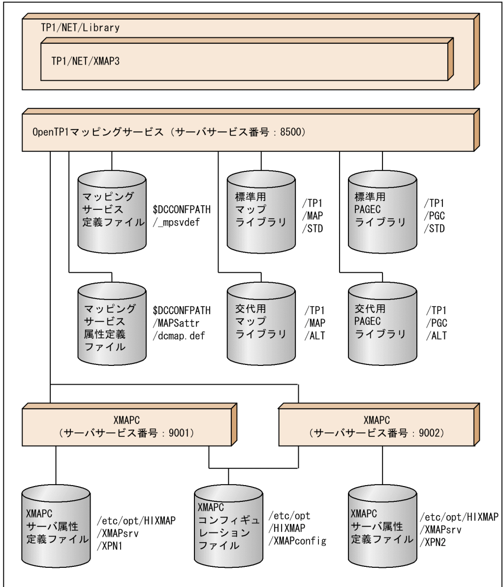
図 F-1 マッピングサービス機能のシステム構成例 (PAGEC 機能を使用する場合)
