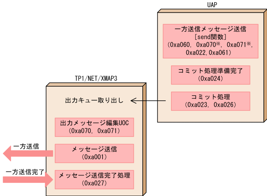
図 C-2 一方送信メッセージ送信時の MCF 性能検証用トレースの取得タイミング
