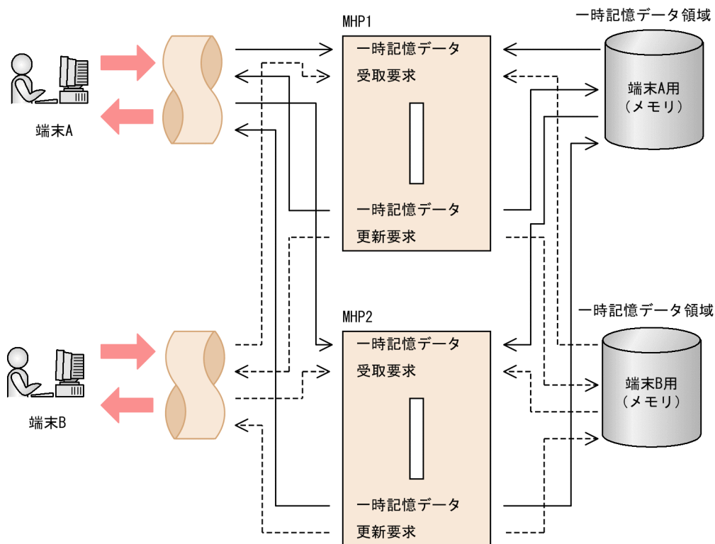
図 2-14 一時記憶データの使用形態
