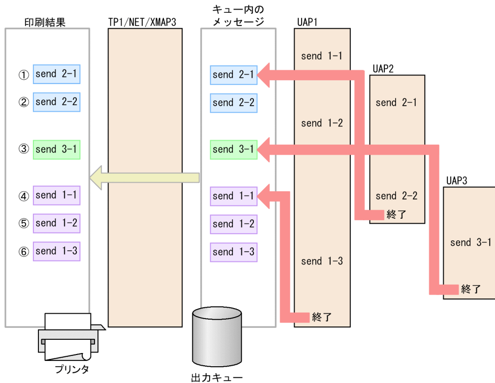
図 2-19 メッセージグループ送信機能を使用する場合の印刷結果
