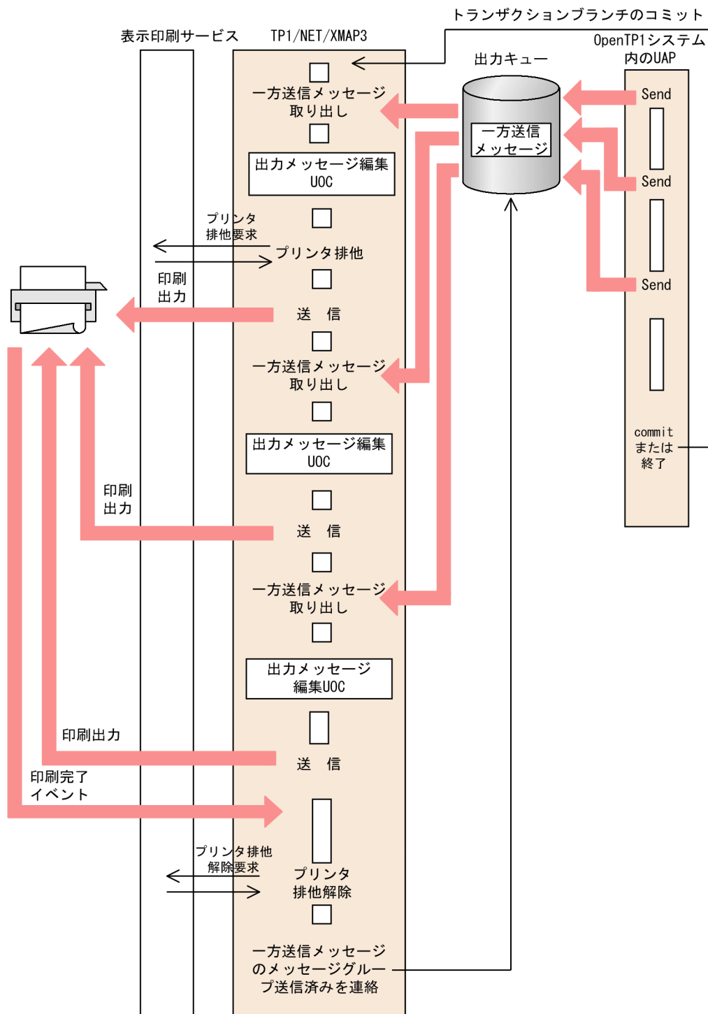
図 2-20 メッセージグループ送信の流れ
