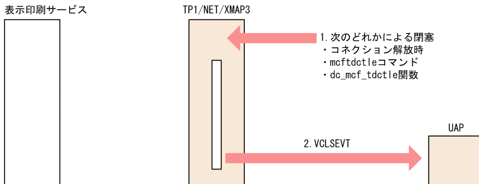
図 2-7 プリンタ属性の端末状態の閉塞処理
