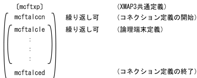
図 7-1 TP1/NET/XMAP3 のプロトコル固有定義コマンドの指定順序
