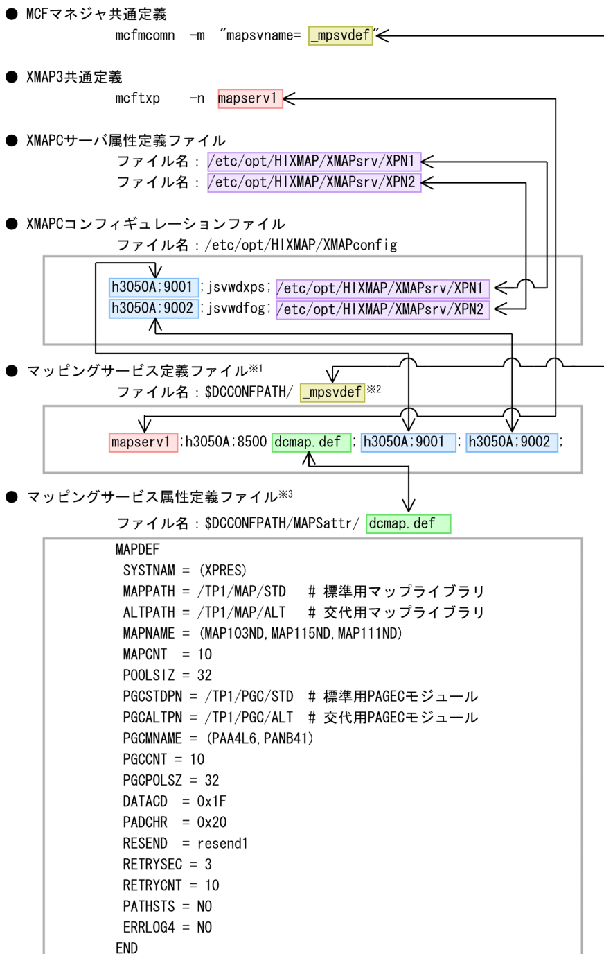
図 F-2 マッピングサービス機能の定義例 (PAGEC 機能を使用する場合)
