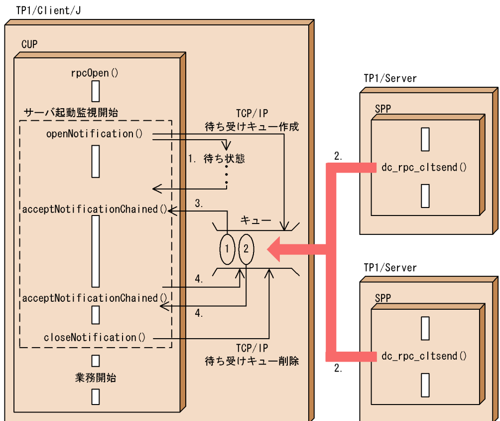
図 2-23 一方通知連続受信機能の処理の流れ
