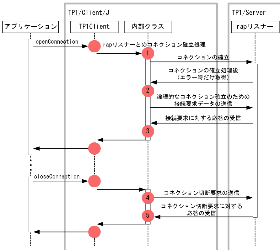
図 2-33 rap リスナーとのコネクション確立、切断処理でのトレース取得ポイント
