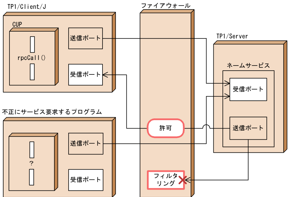
図 2-42 受信ポート固定機能を使用する場合（ネームサービスを使用した RPC）
