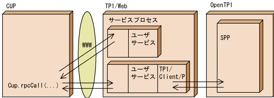
図 2-29 DC_JUSR サービスセットを使用した場合にサービスが実行される流れ
