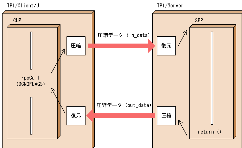
図 2-37 データ圧縮機能の概要
