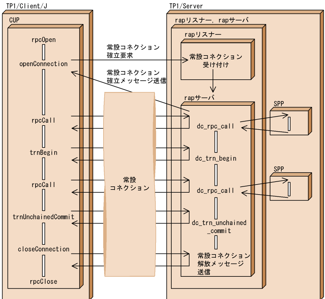
図 2-1 常設コネクションの確立・解放処理
