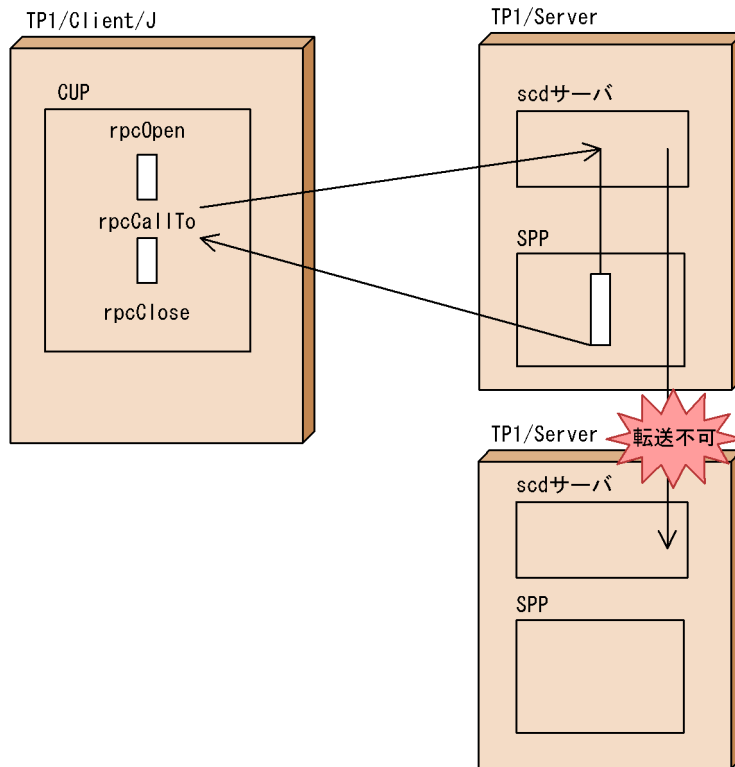
図 2-9 通信先指定 RPC を使用したサービス要求の流れ
