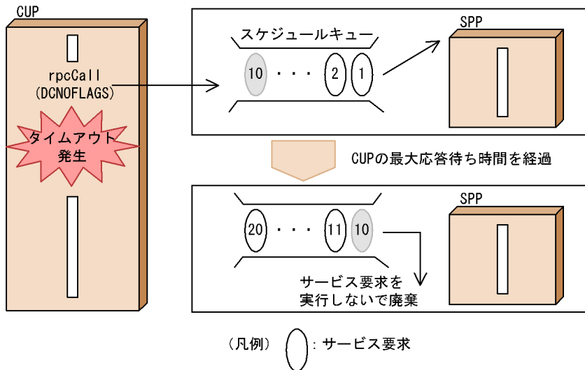
図 2-10 同期応答型 RPC タイムアウト時のサーバ負荷軽減機能の処理概要
