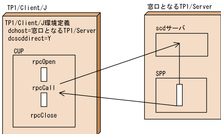
図 2-6 スケジューラダイレクト機能を使用した RPC のサービス要求の流れ
