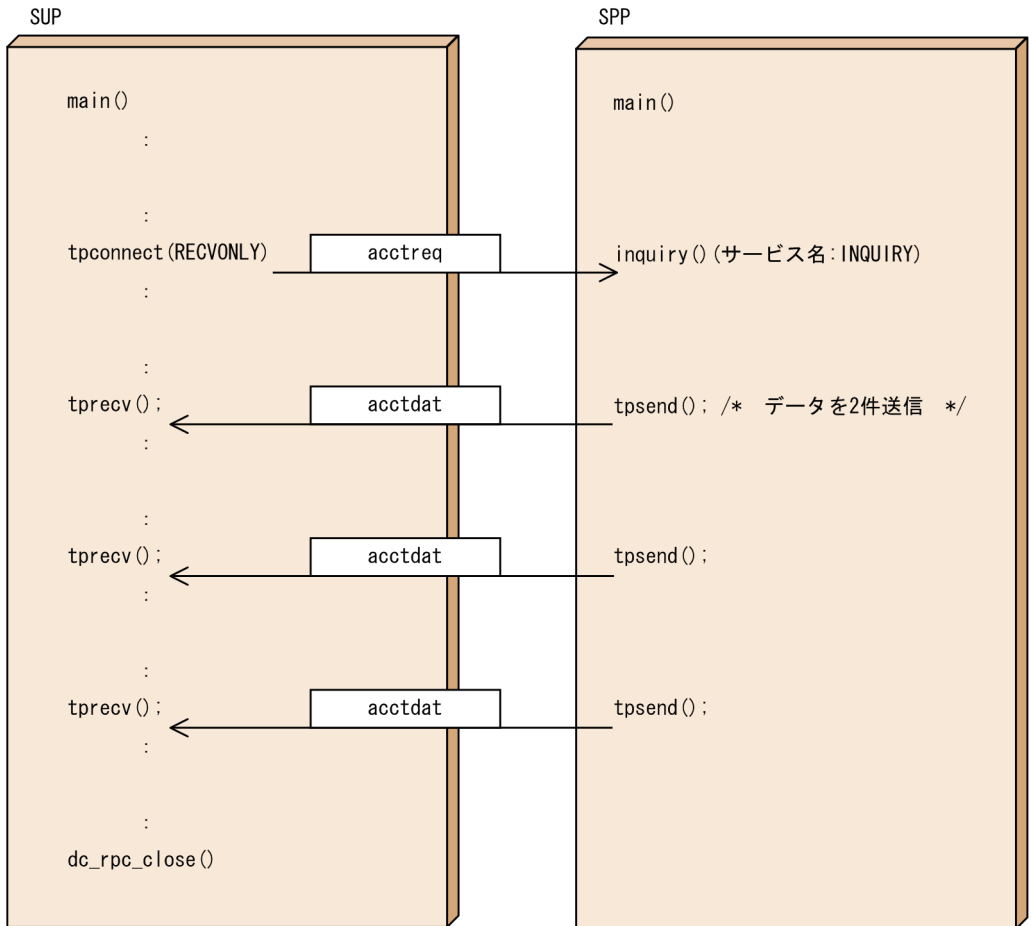
図 6-5 会話型サービスの通信形態
