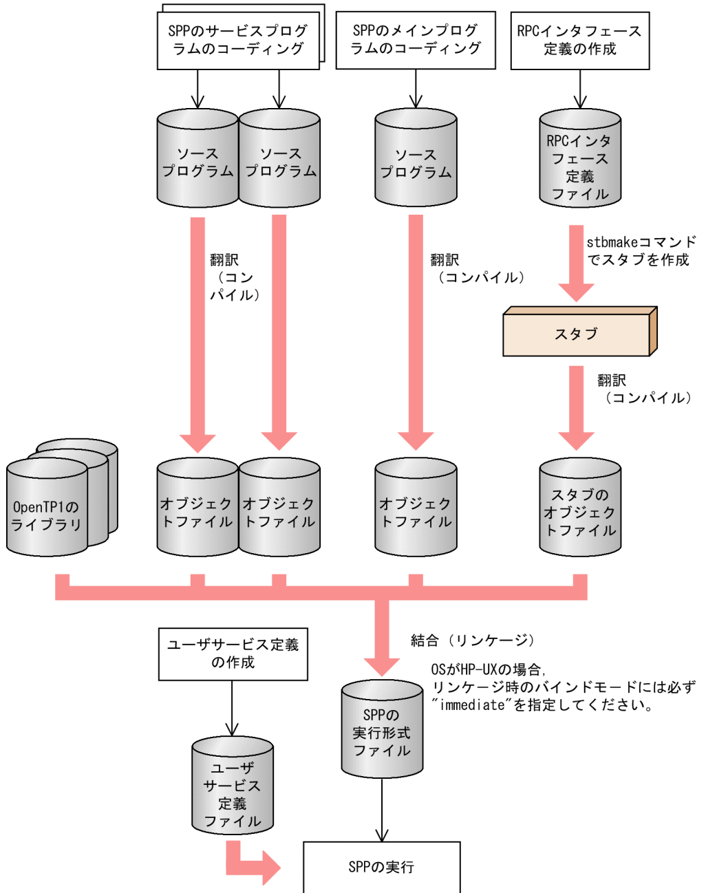
(b) SPP の作成手順 (サービス関数動的ローディング機能使用時)
