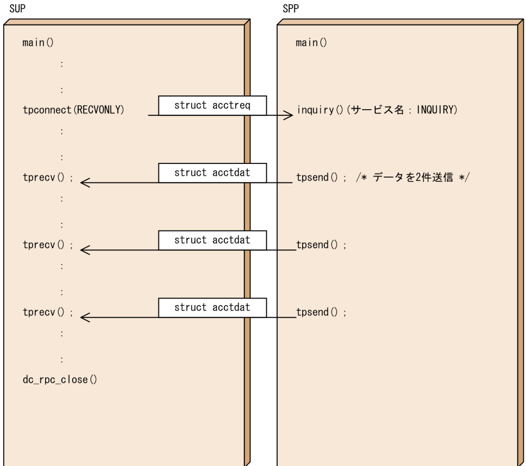
図 7-5 会話型サービスの通信形態
