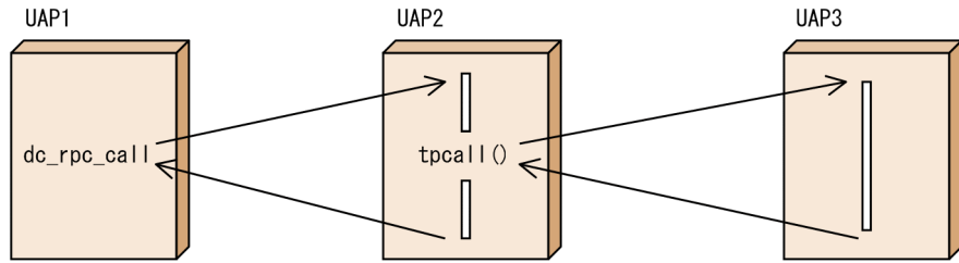
図 A-1 通信を併用する形態と必要なインタフェース定義
