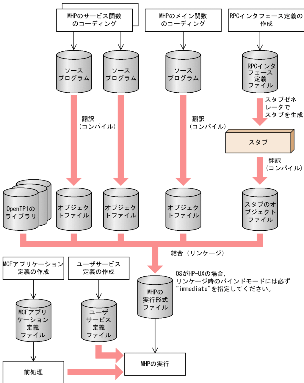
(b) MHP の作成手順 (サービス関数動的ローディング機能使用時)
