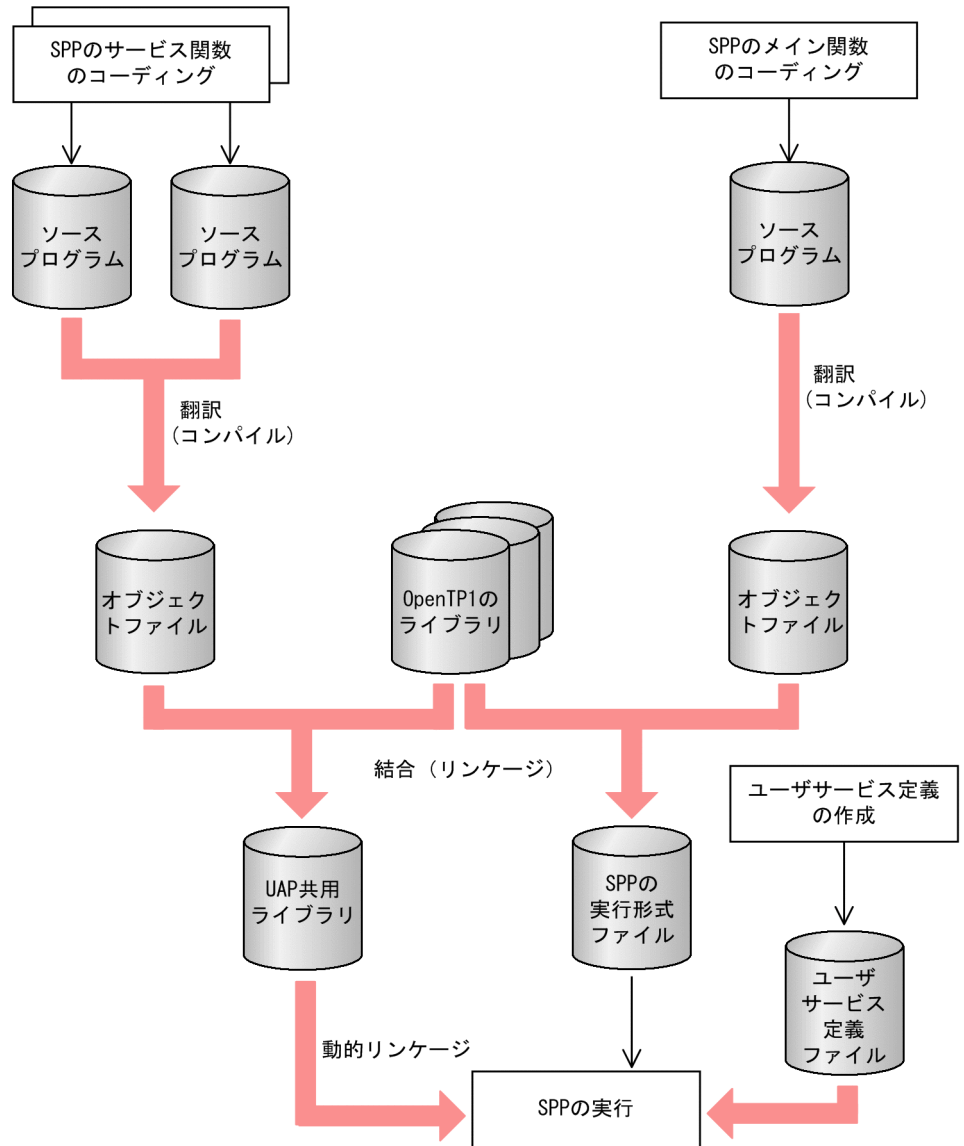
図 1-3 SPP の作成手順（サービス関数動的ローディング機能使用時）
