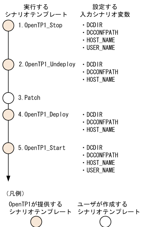
図 3-50 ローリングアップデートの実行順序
