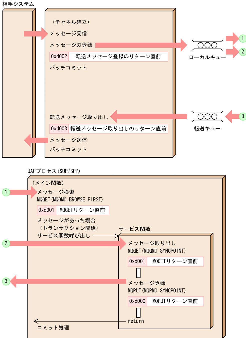
図 L-4 TP1/Message Queue の性能検証用トレースの取得例
