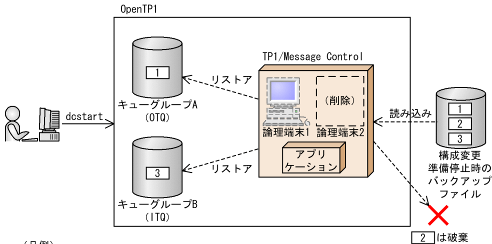
図 5-10 削除した論理端末がある場合のメッセージのリストアの流れ
