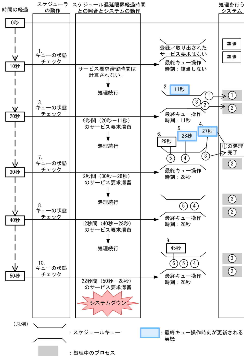
図 3-2 スケジュールキューの監視の例 (schedule_delay_limit=15, schedule_delay_abort=Y の場合)
