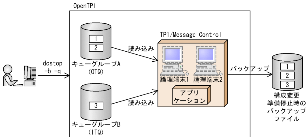
図 5-7 未処理受信メッセージまたは未送信メッセージのバックアップの流れ
