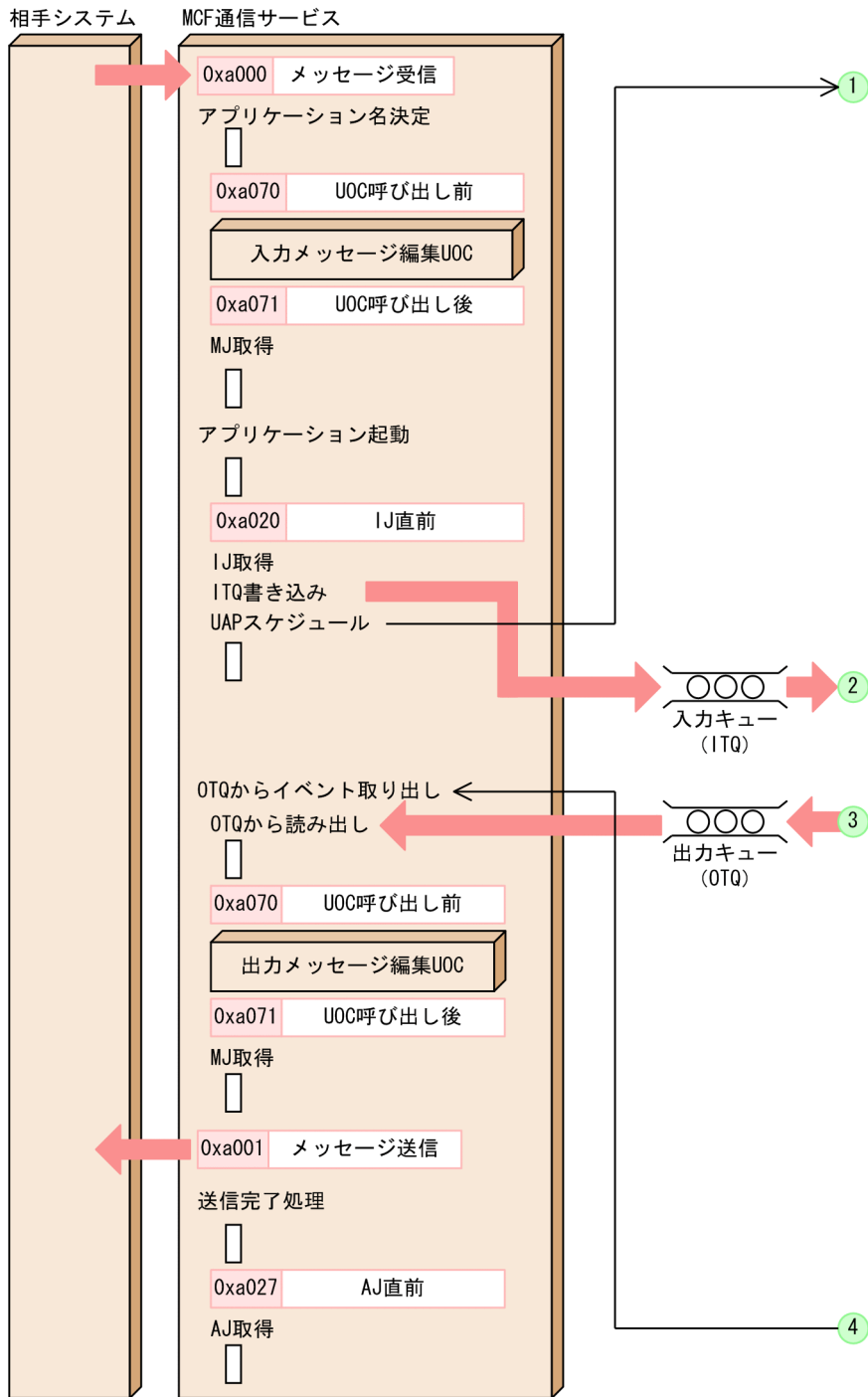
図 L-3 TP1/Message Control の性能検証用トレースの取得例
