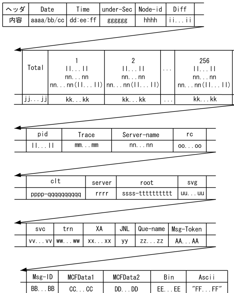
図 13-2 性能検証用トレースファイルの出力形式 (表計算ソフトで表示)
