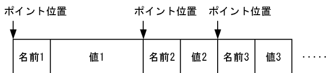
図 25-4 CGI リストの構造
