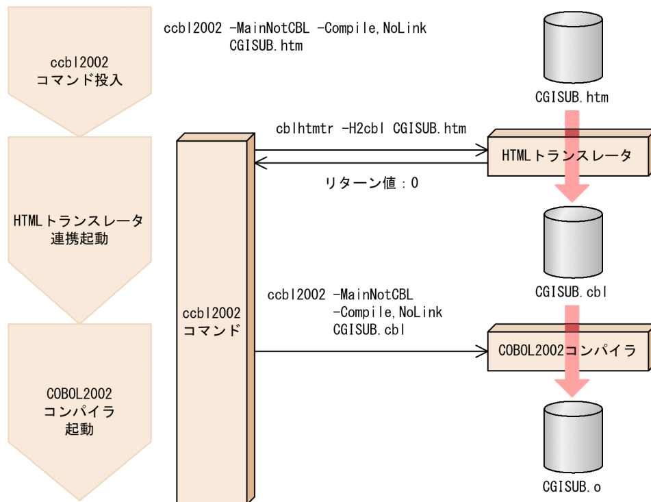
図 25-5 ccb12002 コマンドで HTML ファイルをコンパイルするときの流れ
