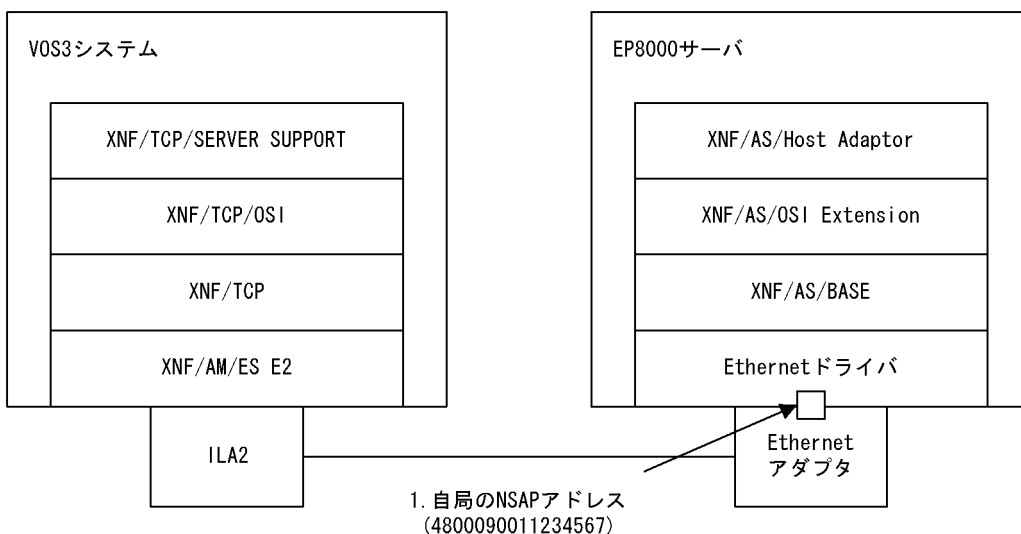
図 4-22 エンドシステムで OSI 拡張高信頼化機能を使用して接続する場合の構成例
