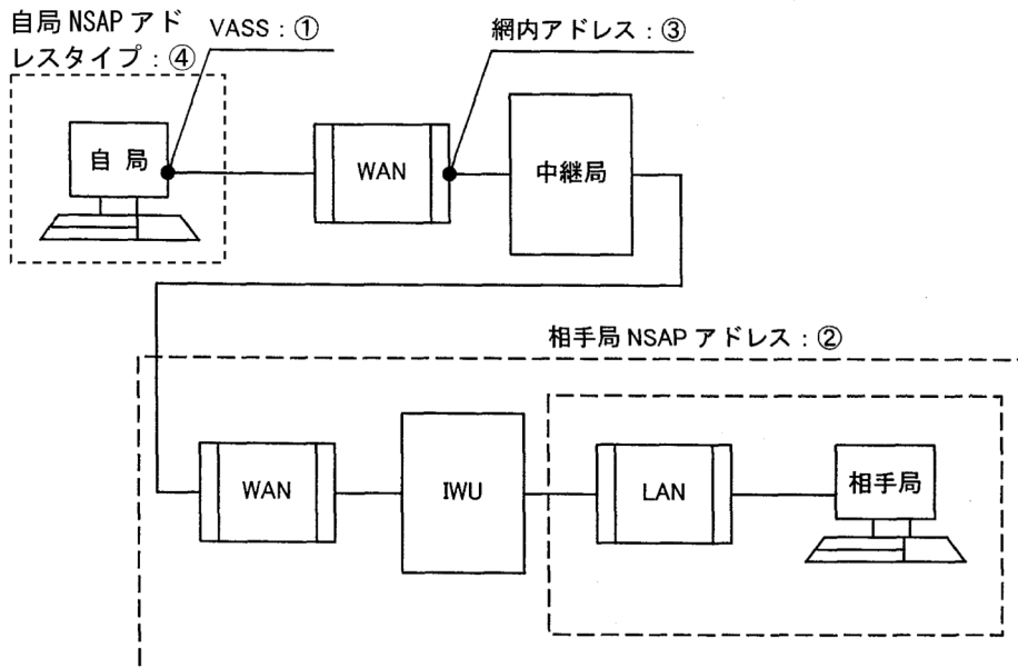
図 2-6 WAN 接続から IWU 経由による LAN 接続の場合のネットワークモデル
