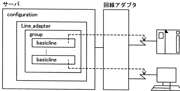
図 1-4 定義文とハードウェア資源との対応（ベーシック手順の場合）
