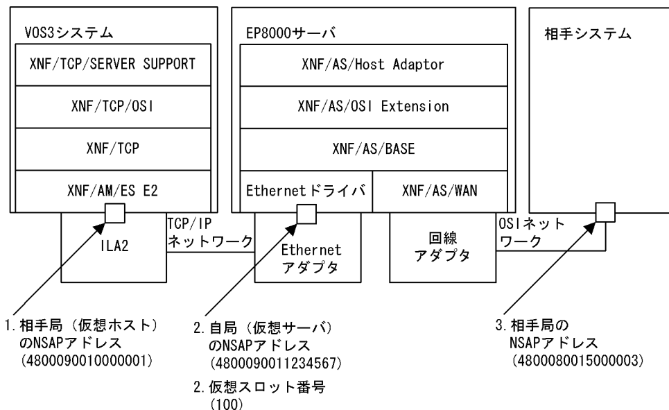
図 4-23 ゲートウェイシステムで OSI 拡張高信頼化機能を使用して接続する場合の構成例
