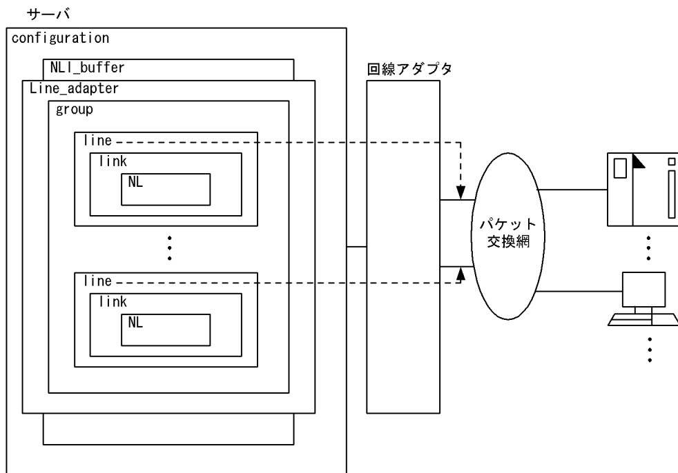
図 1-9 定義文とハードウェア資源との対応 (X.25 パススルーの場合)
