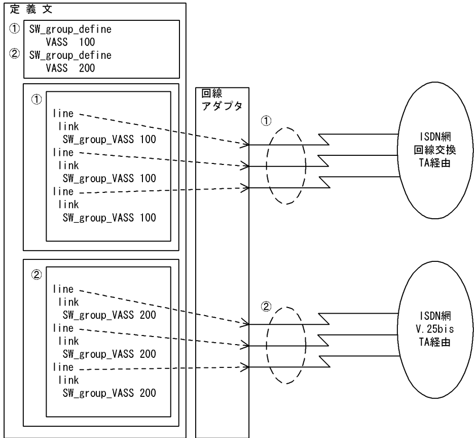
図 2-8 HNA 公衆回線のグループ指定を行った場合の定義文と回線接続構成の関係
