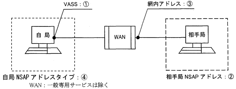
図 2-7 INTAP V2.0 新形式の NSAP アドレスを使用する場合のネットワークモデル
