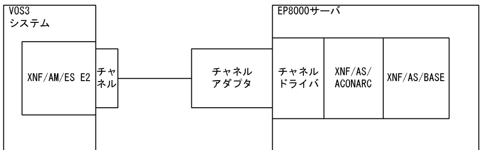
図 4-20 1 台の EP8000 と 1 台の VOS3 ホストを接続する場合の構成例
