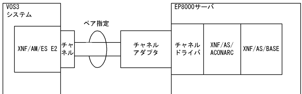
図4-21 1台のEP8000と1台のVOS3ホストをペア指定した二つのチャンネルラインで接続する場合の構成例
