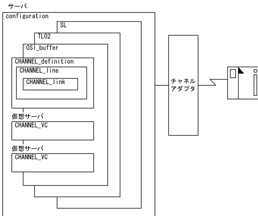
図 1-8 定義文とハードウェア資源との対応 (チャンネル接続の場合)
