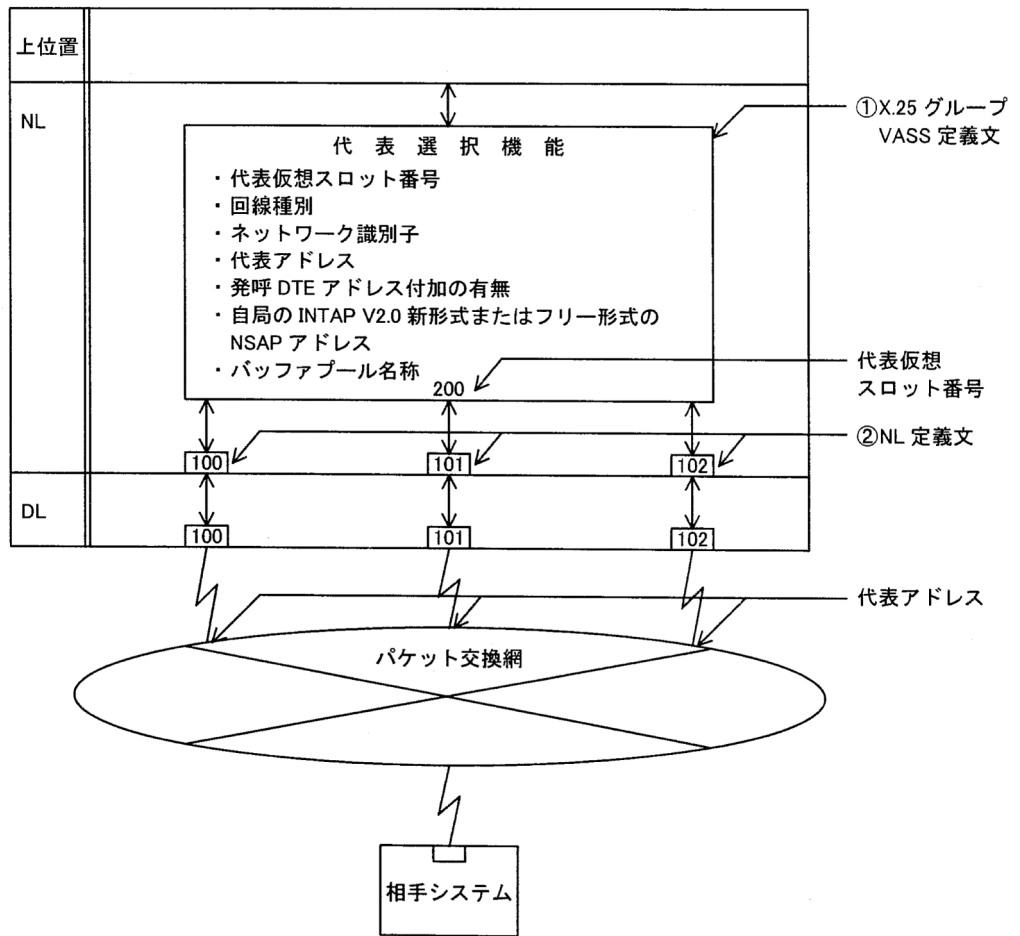
図 4-9 X.25 の代表選択機能を使用する場合の構成例
